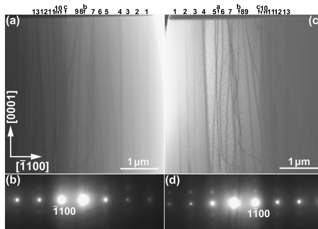
図 2 (a) 楔形 GaN 単結晶膜中の貫通転位の BF-STEM 像(1 MV)と (b) SAED 図形 ( g = \bar{1}100 )。画像右端が試料端(試料厚さ 0.5 \mu\text{m} )、左に向かって試料厚さが増加する(左端で厚さ 2.5 \mu\text{m} )。画像上部の数字は転位線を表す番号を示す。(c), (d) 同一試料の裏面からの観察結果(楔形試料の表裏を逆にして観察)。画像の左から右にかけて試料が厚くなる。転位線を示す番号は (a) と対応している。(c) BF-STEM 像, (d) SAED 図形 ( g = \bar{1}100 )。文献(18)を改変引用。
