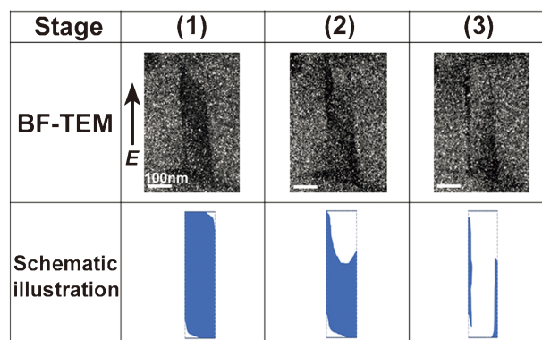
図9 その場観察から得られた分極反転過程でのBF-TEM像(上段)とドメイン形態変化を表す模式図(下段)。文献(29)を改変引用。
