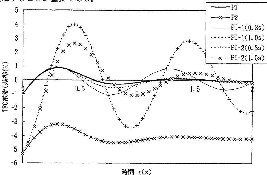
図8. 6 フラットトップ制御時のケースごとの特性比較
