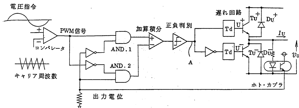
図3. 13 T_d 補正回路の基本構成(1相分)
