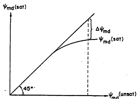
(b) 主磁束(d軸:本論文の \gamma 軸)方向の飽和特性
