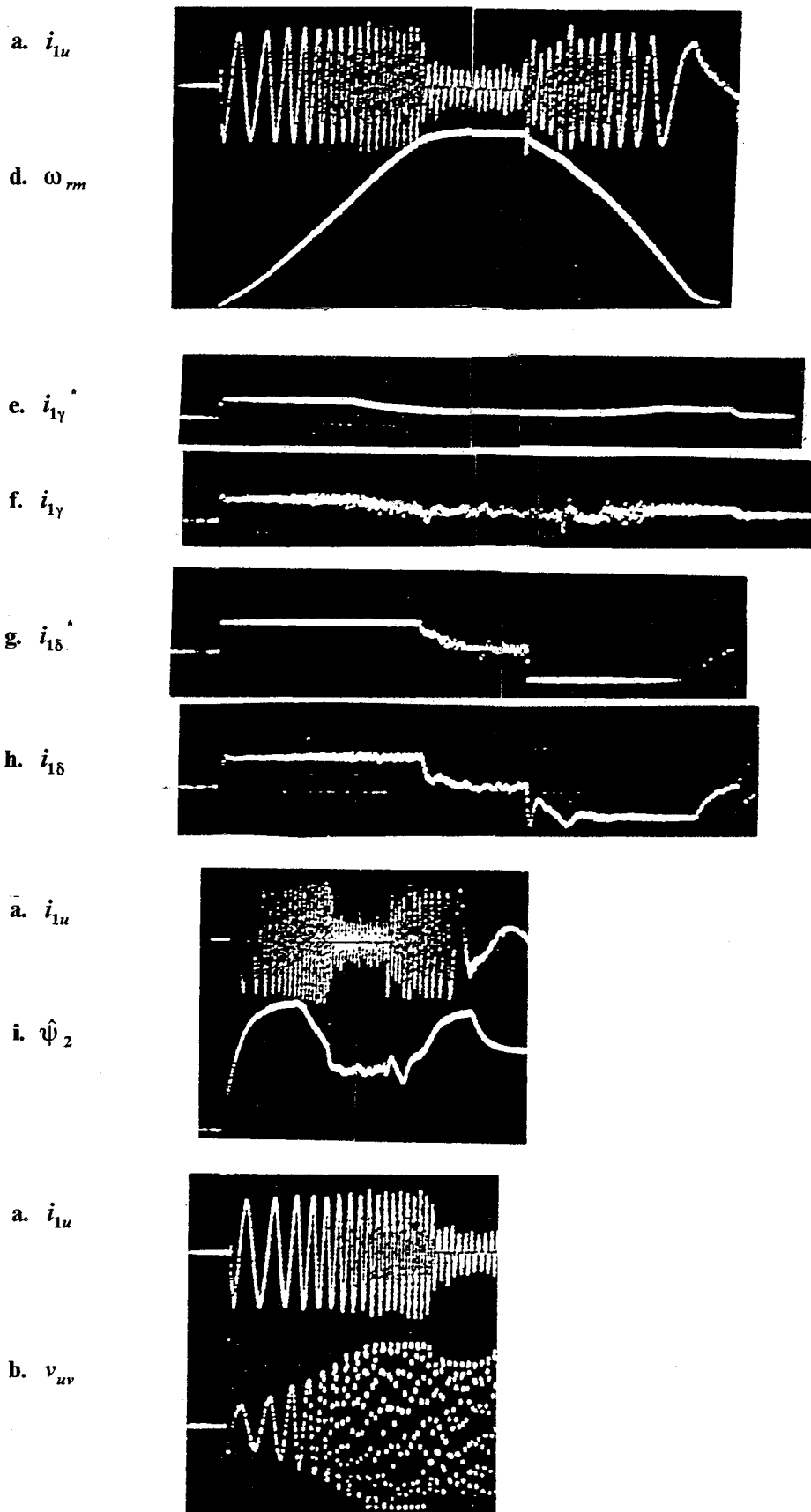
図6. 13 加速特性Ⅱ(慣性負荷, モータ回転数 4000 rpm, T_d 補正あり) (実験結果... f_s = 1.6\text{kHz} , f_c = 1.6\text{kHz} )
