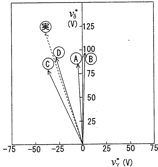
図6. 12 試験結果およびシミュレーション結果(SH, DT考慮の可否の違いによる case A～case D)対する v_{\gamma}^* , v_{\delta}^* の関係を示すベクトル図
