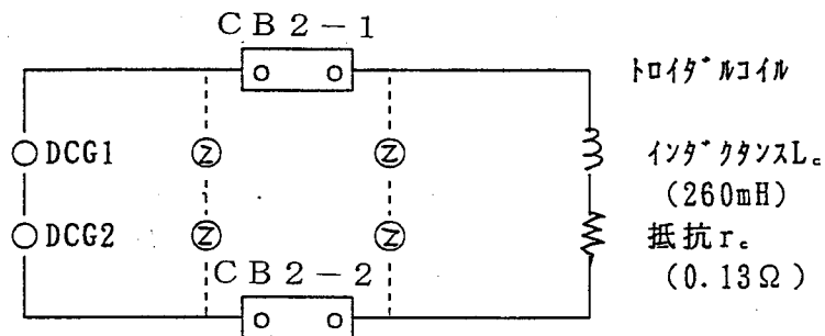
(a) 主回路通電時
