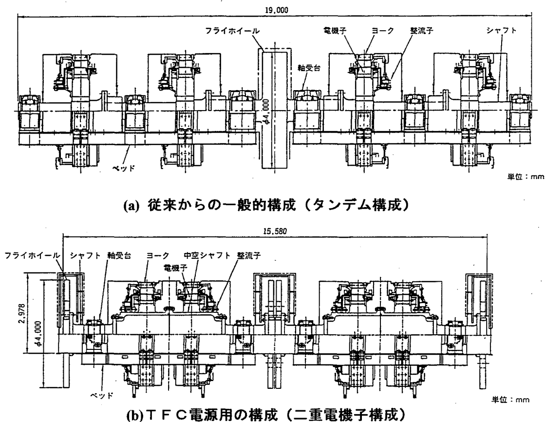
図7. 5 フライホイール付DCGの構成
