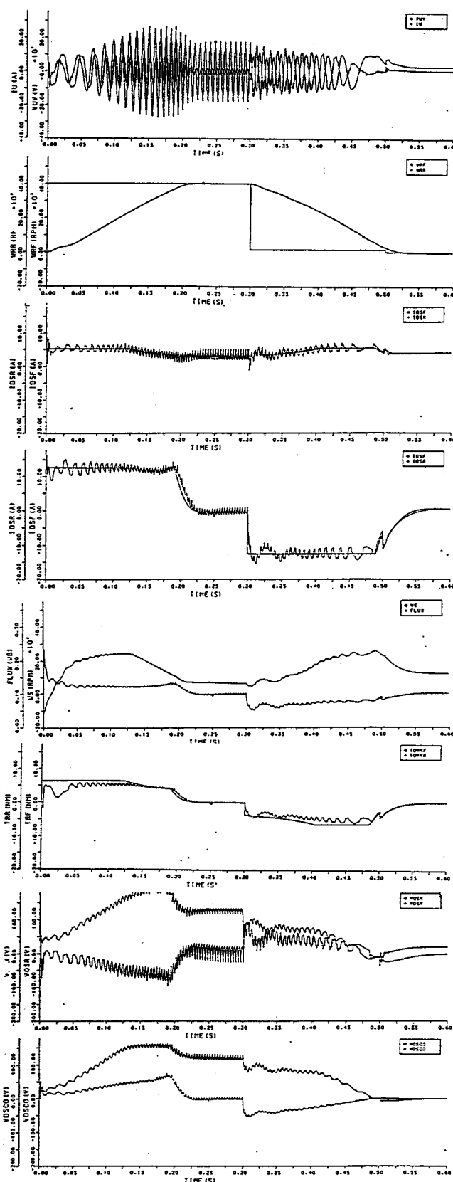
図6. 17 加速特性Ⅱ(慣性負荷, モータ回転数 4000 rpm, T_d 補正なし) (シミュレーション結果 Case 1 \cdots f_s = 1.6kHz , f_c = 1.6kHz )
