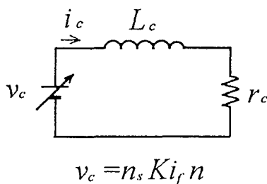
図8.8 発電制動時の過渡特性を表す等価回路
