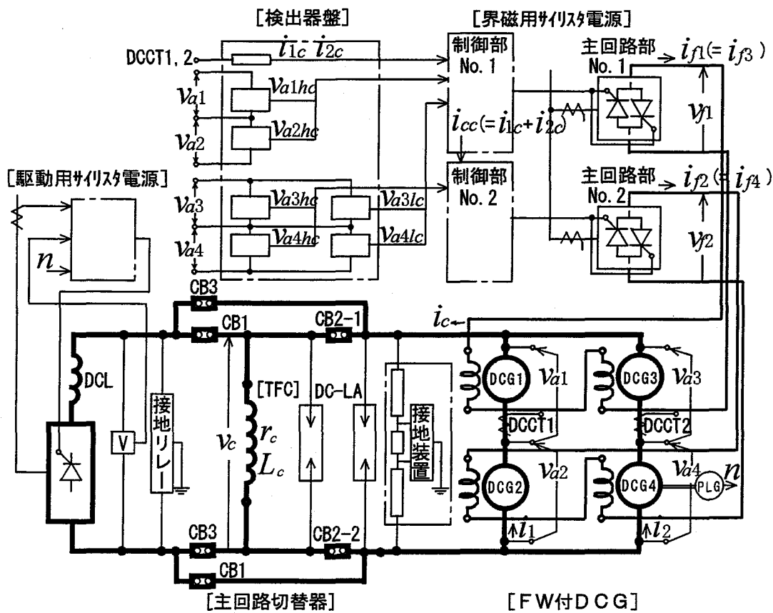
图 7. 7 主回路構成
