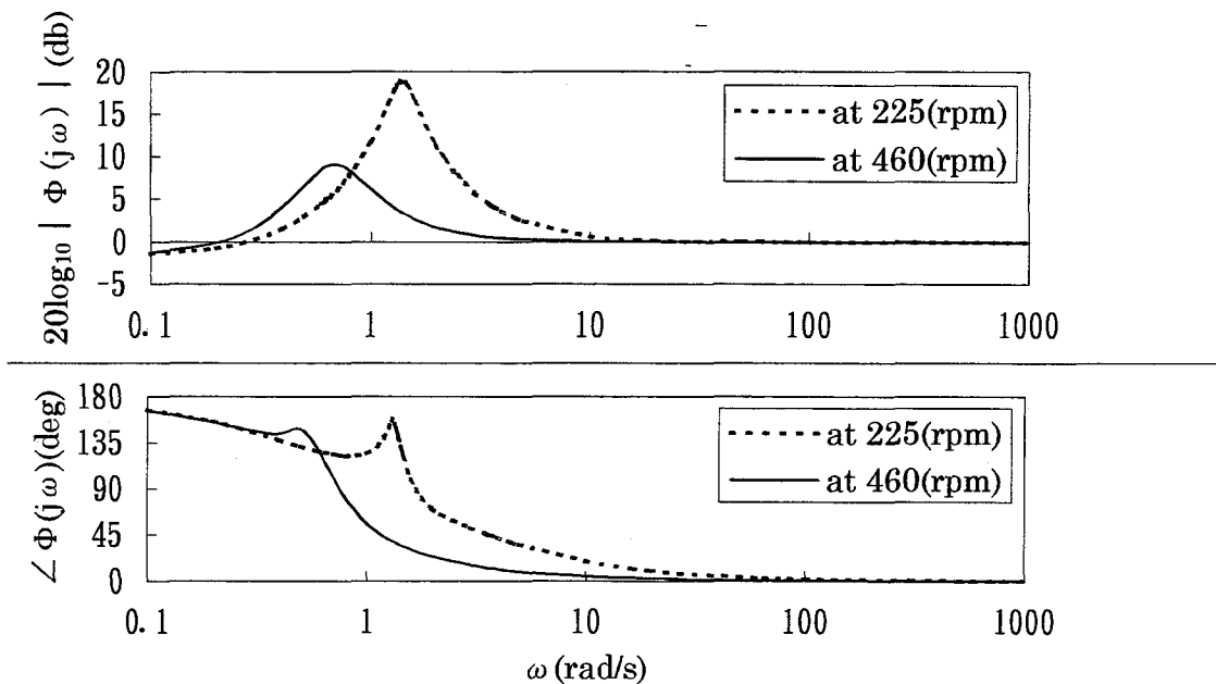
図 8. 2 |\Theta(j\omega)| , \angle\Theta(j\omega) の周波数特性
