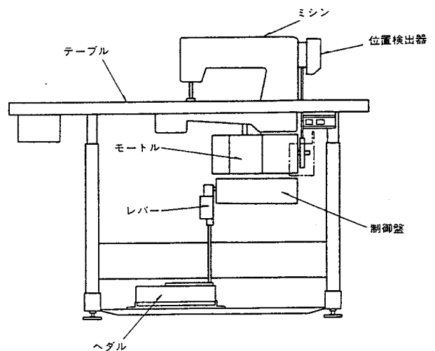
図6. 1 一般工業用マシンの構成
