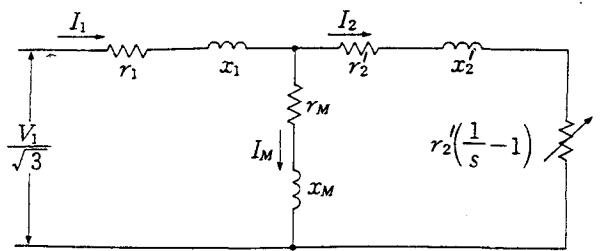
図 2. 2 T形等価回路
