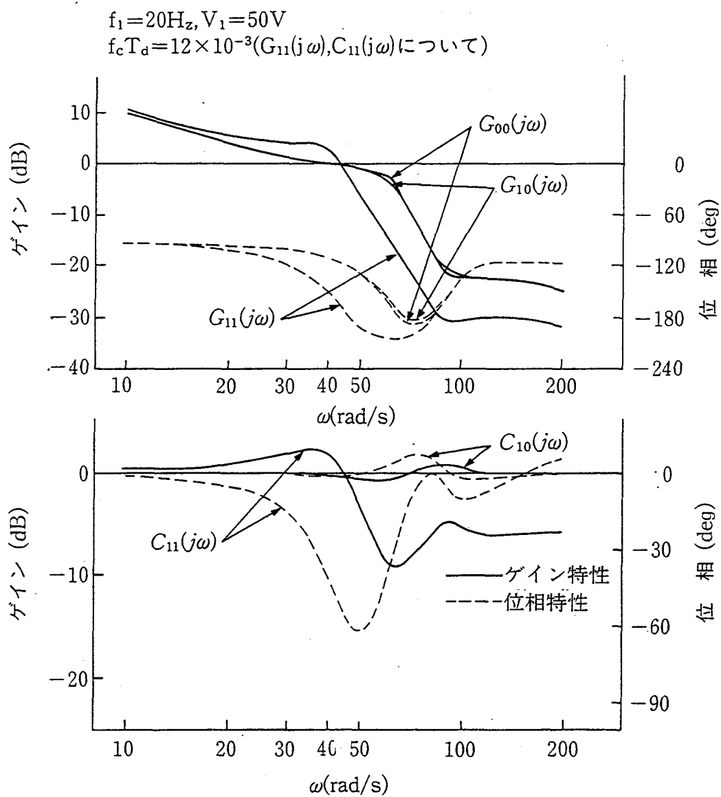
(b) 磁気飽和を考慮しない場合の影響 (A 点)
