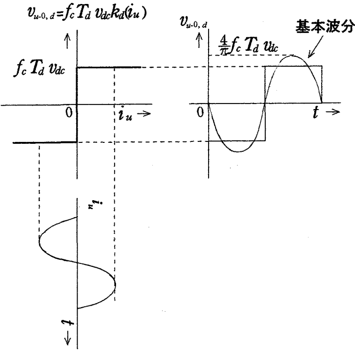
図 3. 7 T_d の影響による方形波電圧の発生と基本波成分
