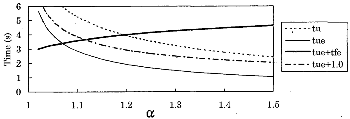
(a) \alpha に対する t_u , t_{ue} , t_{ue}+t_{fe} , t_{ue}+1 の関係
