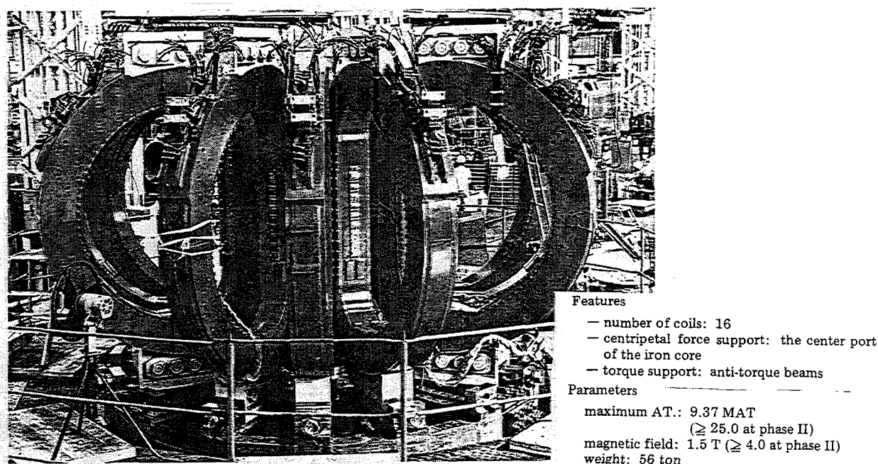
図7. 8 電源装置の負荷となるTFCの外観
