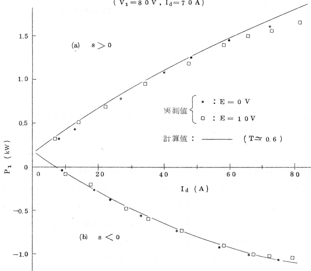
図 1. 5. 1 4 入力と直流電流の関係 ( 供試機 D )
