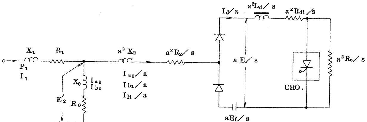
図 1. 5. 2 1 チョップパ方式の等価回路
