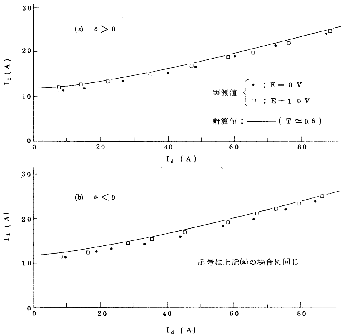
図 1. 5. 1 5 1 次電流と直流電流の関係 ( 供試機 D )
