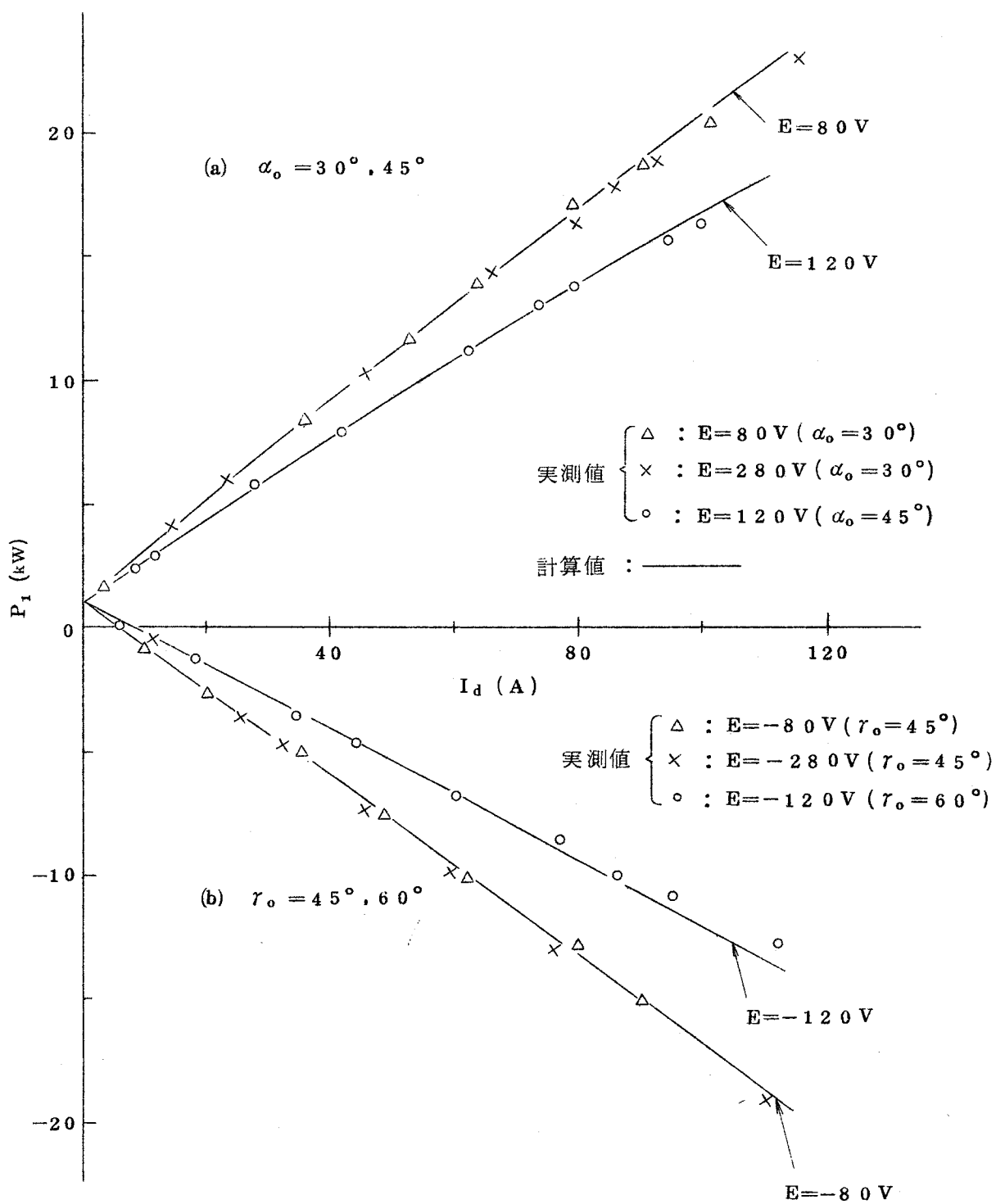
図 1.4.5 入力と直流電流の関係
