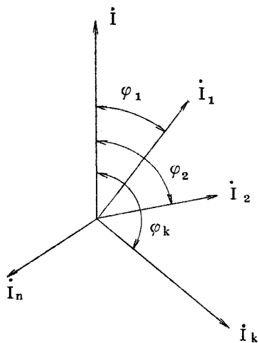
図 1.7.6 励磁電流
