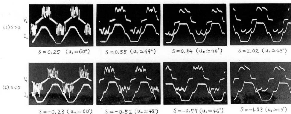
図 1.5.6 定格負荷時における 2 次電圧，電流波形 (供試機 D)
