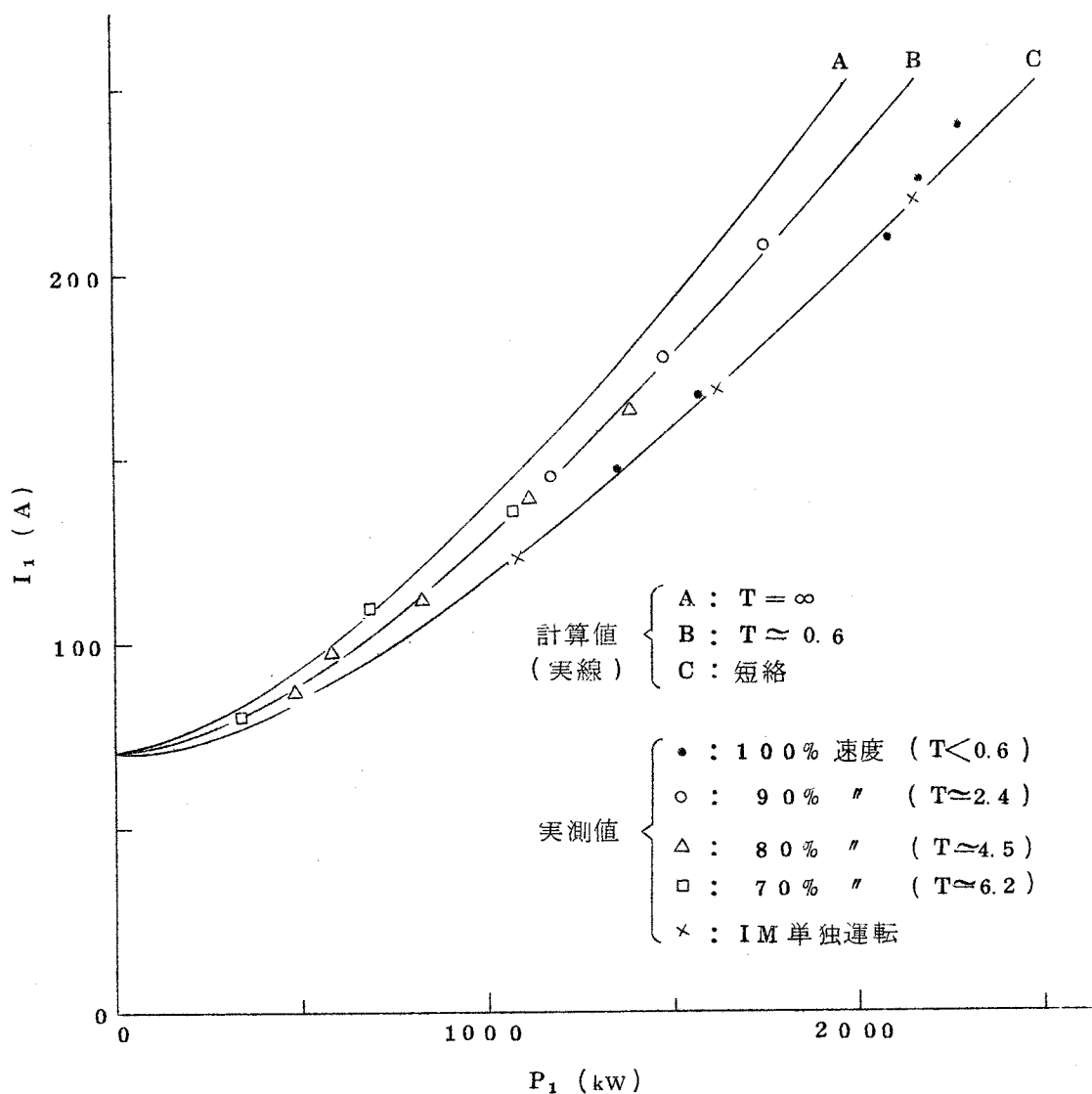
図 1.5.17 2100 kW 機における 1 次電流と入力との関係
