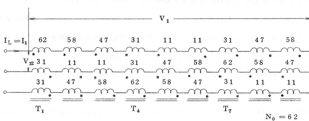
(a) 1 次巻線
