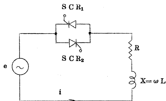
図 2.2.3 逆並列接続したサイリスタをもつR-L直列回路
