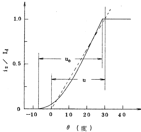
図 1.3.9 i_2/I_d と \theta の関係 ( T = 0.6 , u_0 = 35^\circ )
