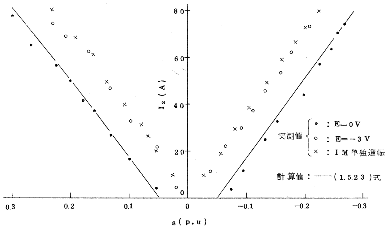
図 1. 5. 1 0 2 次電流とすべりの関係 ( 供試機 D )
