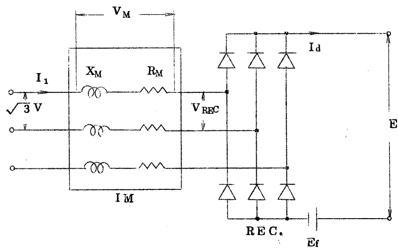
図 2.3.3 中性点分離整流方式における誘導電動機の等価回路
