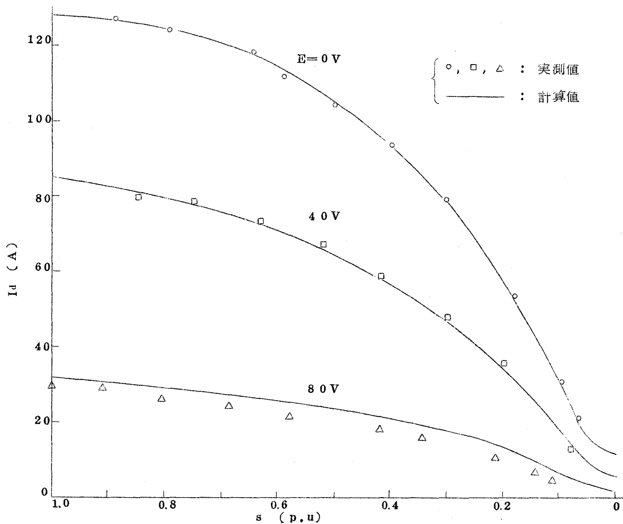
図 2.3.11 直流電流とすべりの関係
