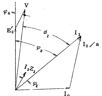
図 1.4.7 1 次側のベクトル図
