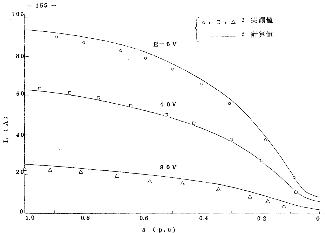
図 2.3.10 1 次電流とすべりの関係
