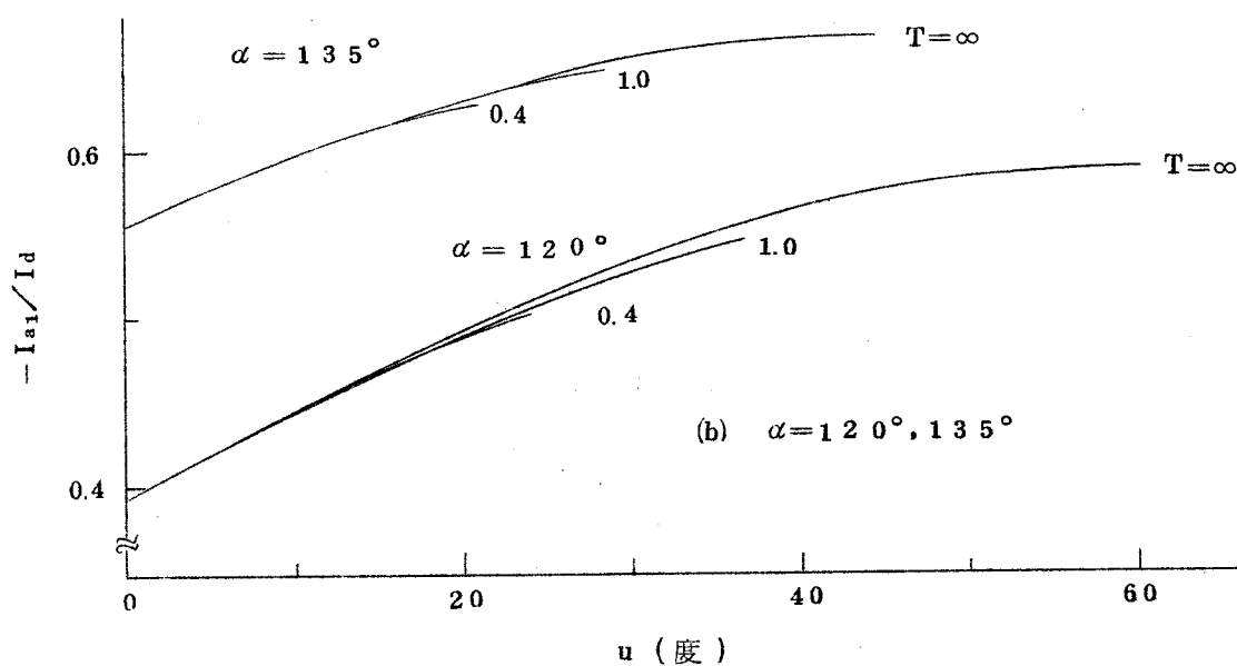
図 1. 3. 4 I_{a1}/I_d と u の関係
