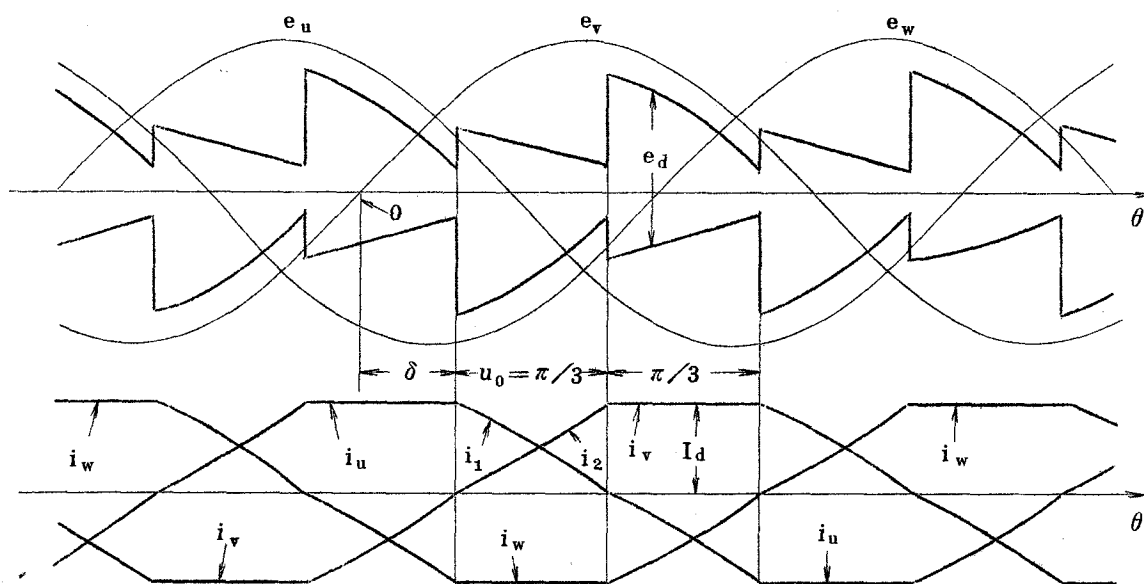
(a) 第 2 モードにおける電圧, 電流の位相関係
