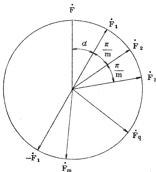
図 1. 7. 5 起磁力
