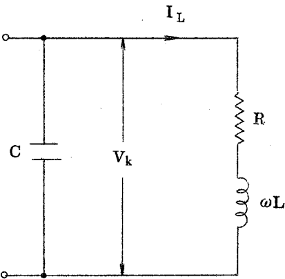
図 1. 7. 1 0 通倍器の等価回路
