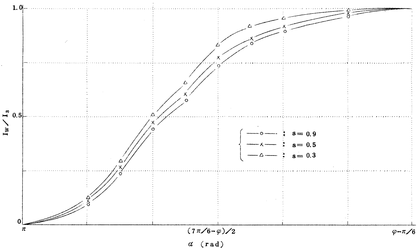
図 2.2.19 2 相制御における W 相電流と点弧角の関係
