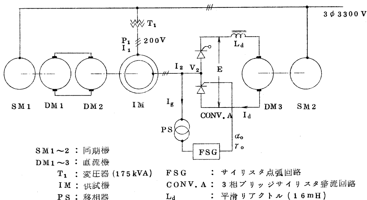
図 1.4.2 実験回路
