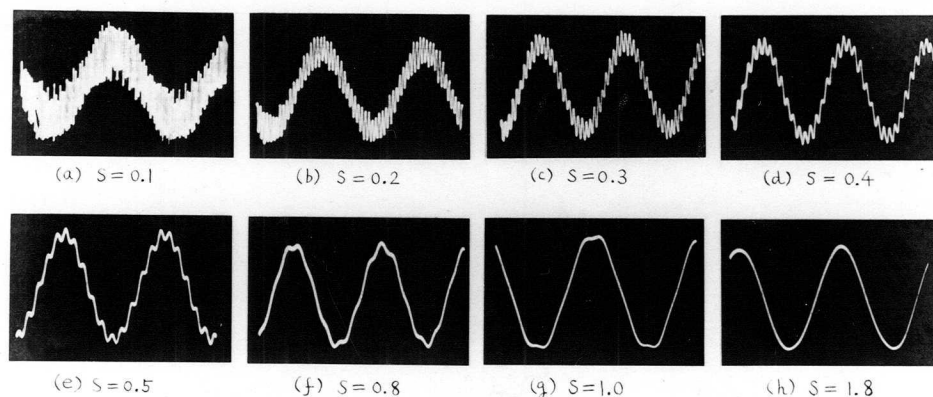
図 1. 4. 1 3 2 次誘起電圧波形 ( 供試機 B )
