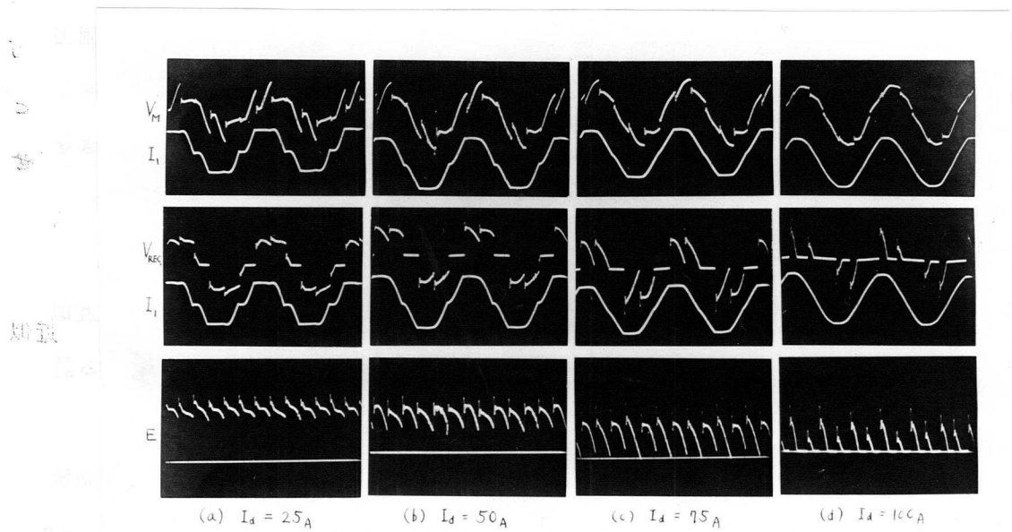
図 2. 3. 5 整流回路の動作モードが変わる境界値
