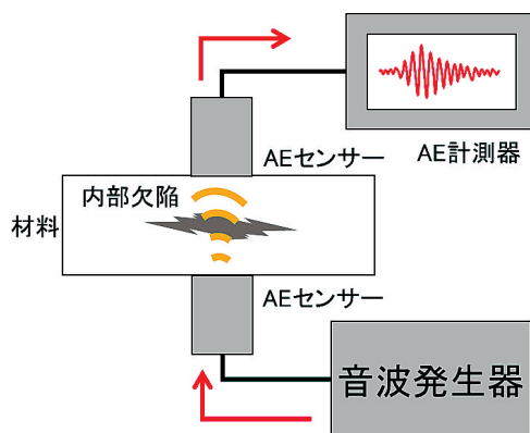
図5 新規評価法（アクティブ AE 法）の原理 音波発生器によって振動波を加振した AE センサーから振動波を発生させ、材料を介することで変化した振動波を従来型 AE 法としての AE センサーで検知し、AE 計測器にて記録する。
