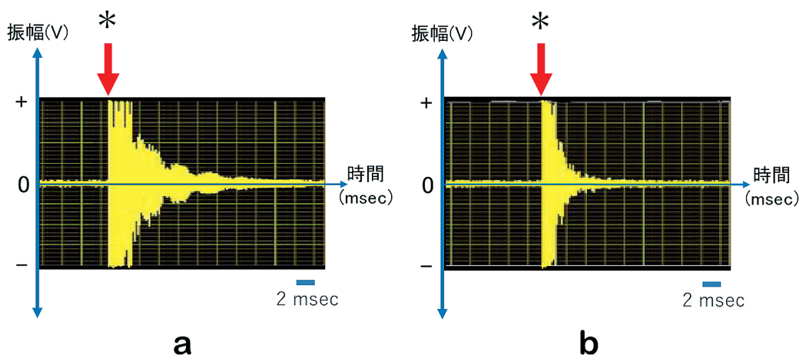
図10 AE法を用いたジルコニアボール衝突試験によって得られた振動波形
