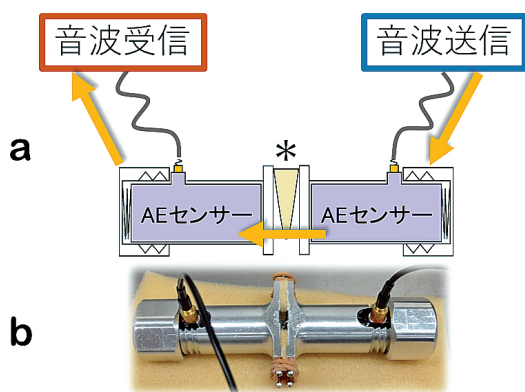
図6 アクティブ AE 法の模式図
