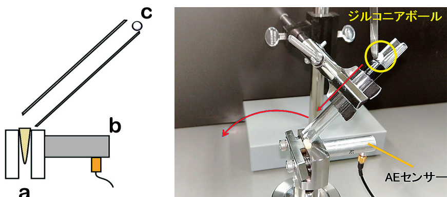
図4 ジルコニアボール衝突試験（左：イラスト，右：実際の写真）
