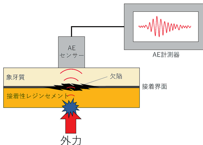
図3 従来型 AE 法の原理
