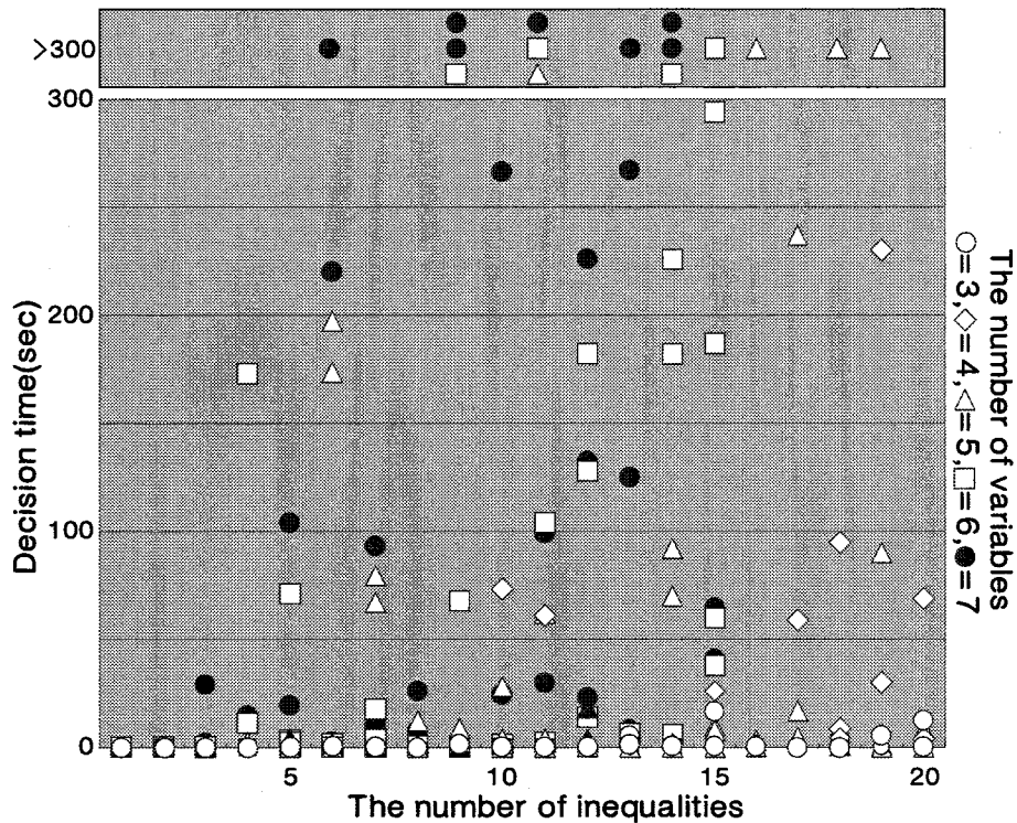
図 15 測定結果 2
