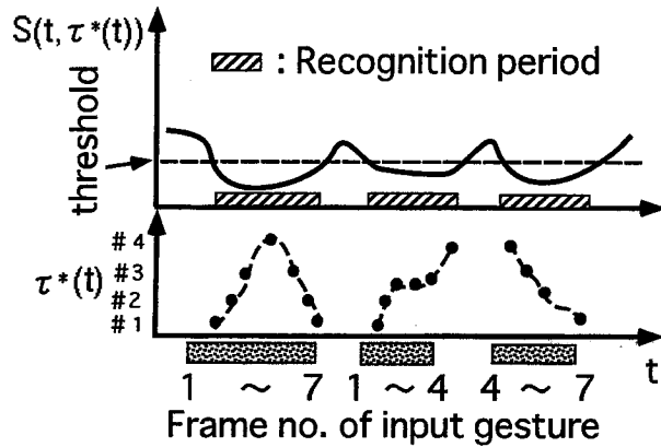
標準パターンは図 4.3 のフレーム # 1 ~ # 4
