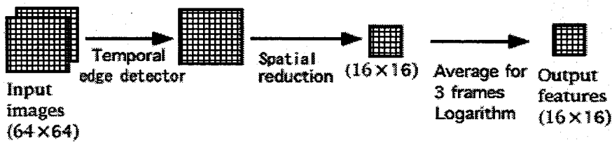
図 2.1 従来の特徴抽出法
