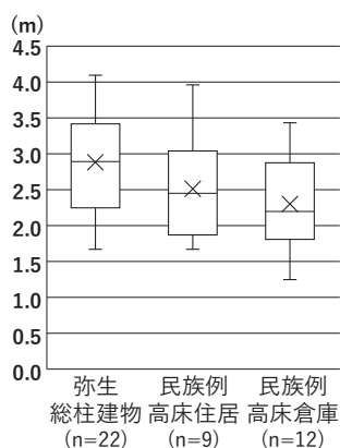
図 1 高床建物の梁行柱間距離
