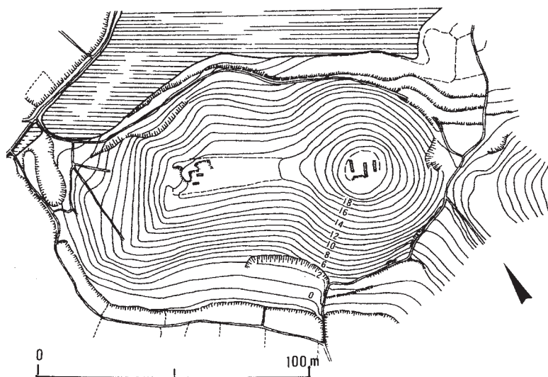
図4 安土瓢箪山古墳の墳丘
