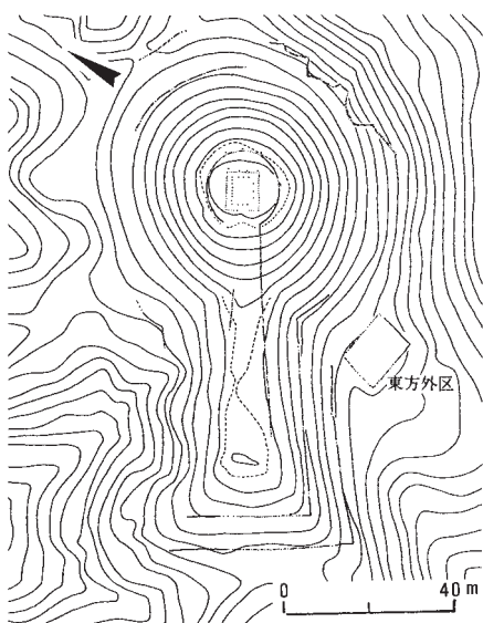
図 14 石山古墳の墳丘
