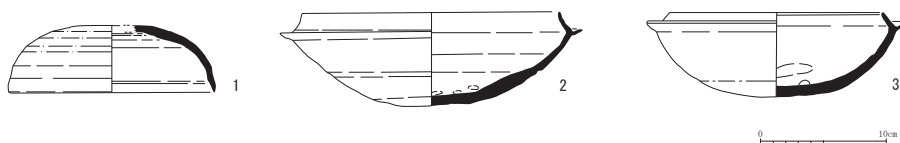
図4 定留鬼塚遺跡と周辺遺跡出土の坏H大型品（S=1/6）
