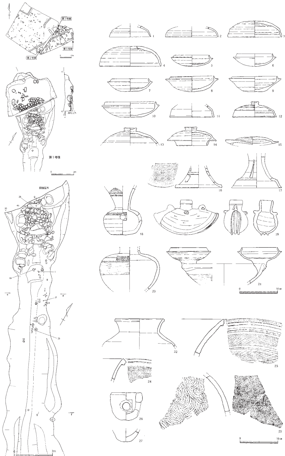
図1 定留鬼塚遺跡1号墳遺構平面図（左上 S=1/1000、左中 S=1/200、左下 S=1/120）・出土遺物（S=1/6）
