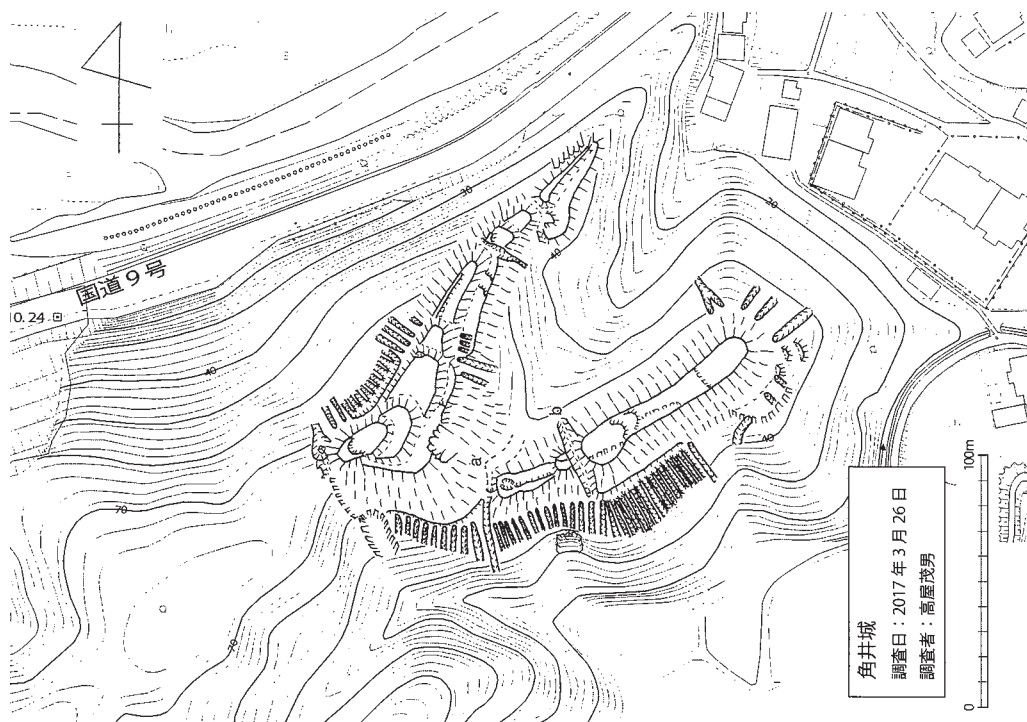
図3 角井城縄張り図（中四国地方で最も堅堀本数が多い）（高屋編 2017）
