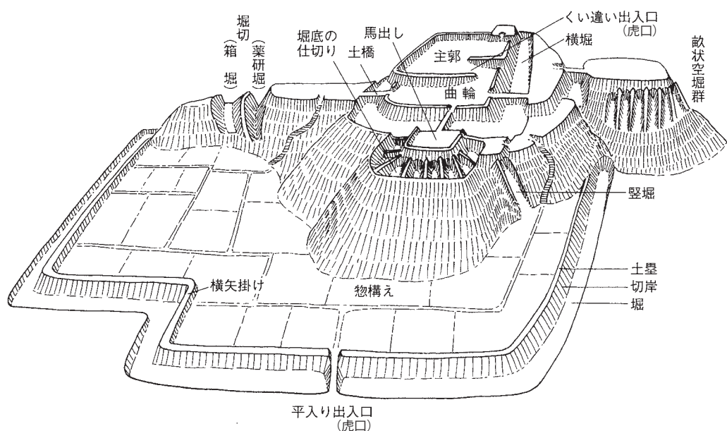
図1 中世山城の遺構模式図（文化庁 2013）
