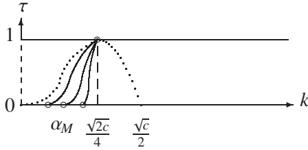
Fig. 12. \mathcal{F}_2^-
