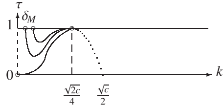
Fig. 13. \mathcal{F}_2^+
