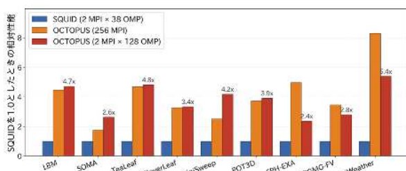
図 7 : SPEchpc 2021 ベンチマーク (tiny サイズ) による SQUID と OCTOPUS の実測性能比較 (縦軸は SQUID を 1.0 としたときの相対性能)
