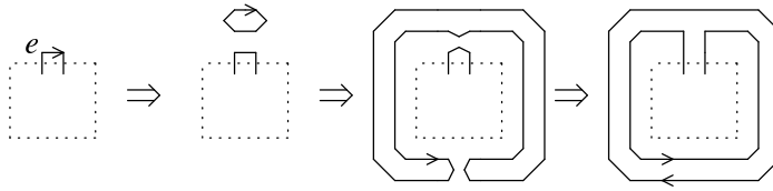
Fig. 5. Turning edge over
