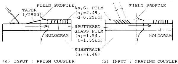
図5.1 作成した導波路ホログラムの構造
