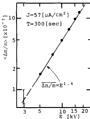
図 4.15 平均屈折率変化量と電子ビーム電圧の関係
