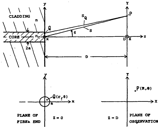
図 2.2 ファイバ端面と観測面の定義
