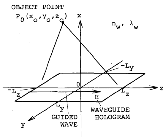
図 3.7 導波路ホログラムの平面ホログラム的取扱
