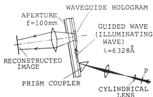
図 5.5 再生(直接波)のための光学系
