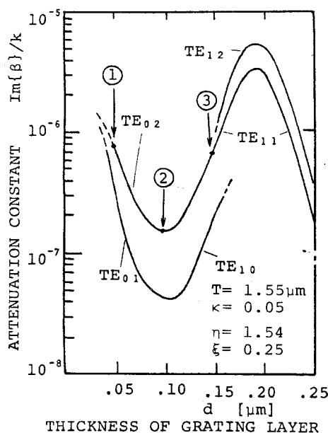
図 6.4 伝搬定数虚数部の記録材料層膜厚への依存性
