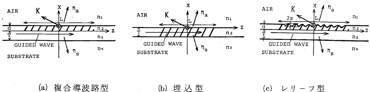
図6.1 高効率導波路ホログラムの構造
