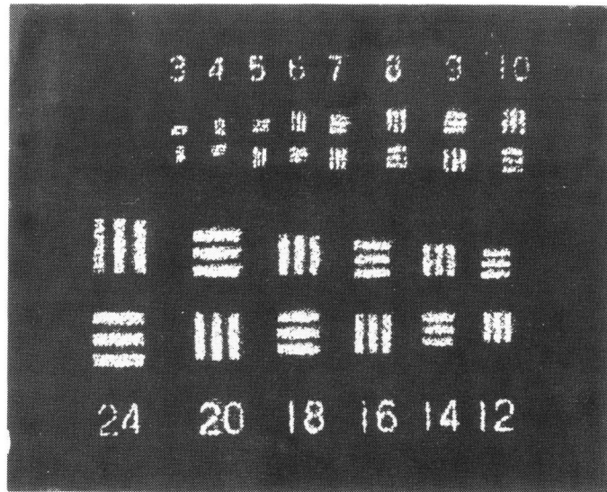
図 4.1 0 ホログラム再生像 ( \text{As}_2\text{S}_3 , T=1.3\mu\text{m} , 4\text{mm}\phi )
