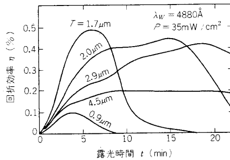
図 4.7 回折効率の時間的变化 ( \text{As}_{40}\text{Se}_{25}\text{S}_{25}\text{Ge}_{10} , V=1 )
