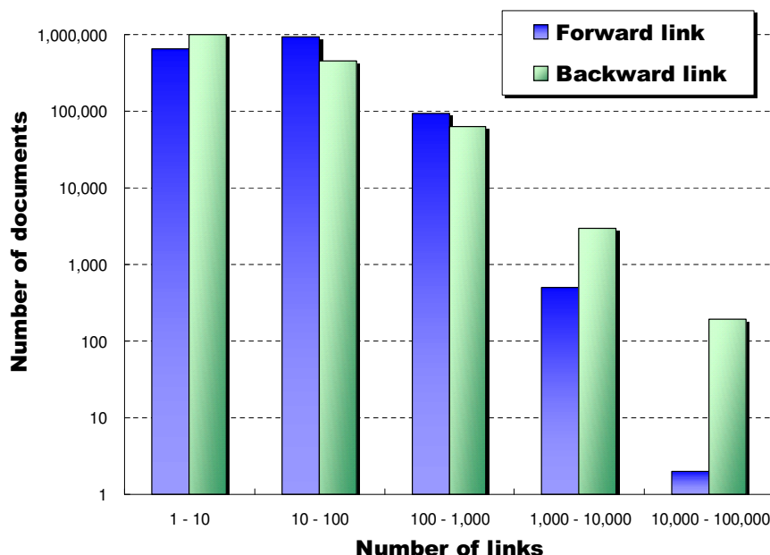
図 1.1: リンク数の分布
