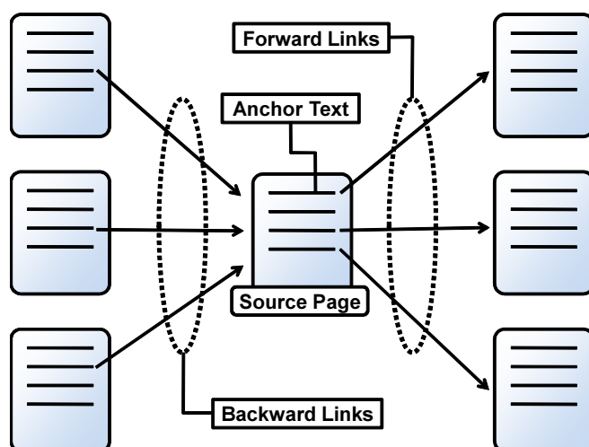
図 1.5: リンクの概念
