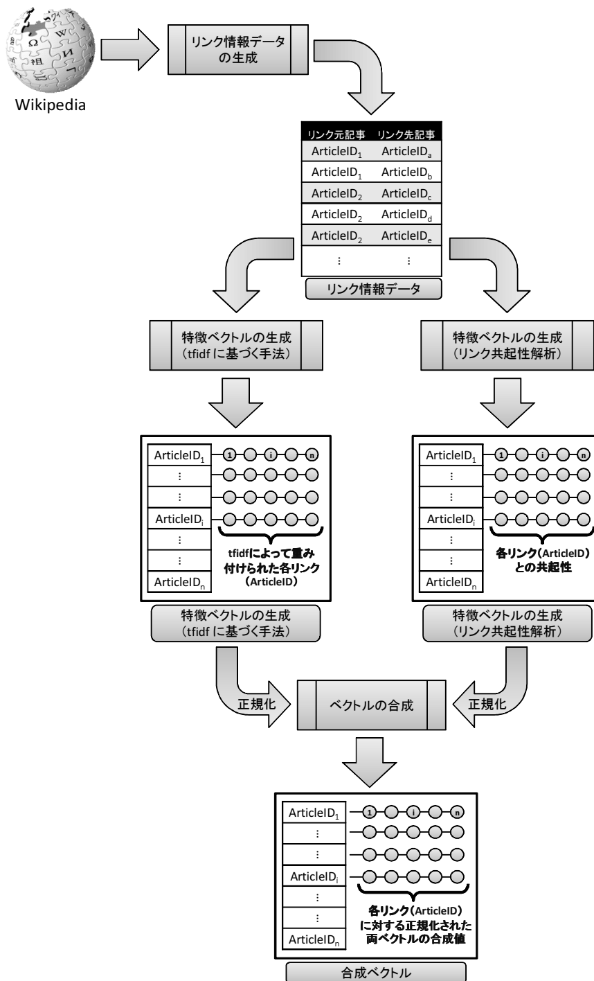
図 3.1: 処理の流れ：ベクトルの生成
