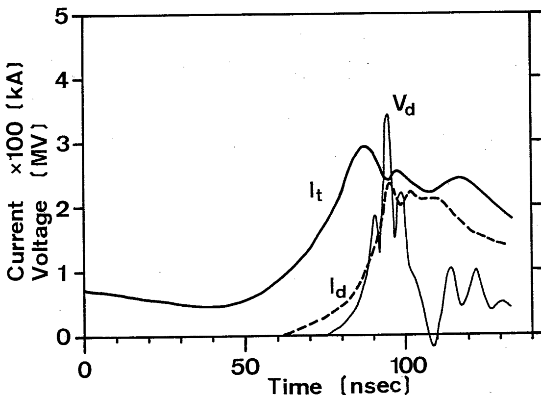
第 2-9 図 1 \Omega モードにおける電圧・電流波形
