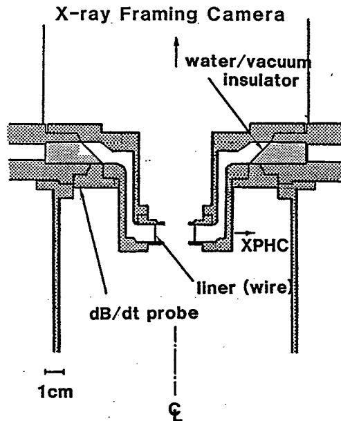
第5-1図 ライナー実験配置
