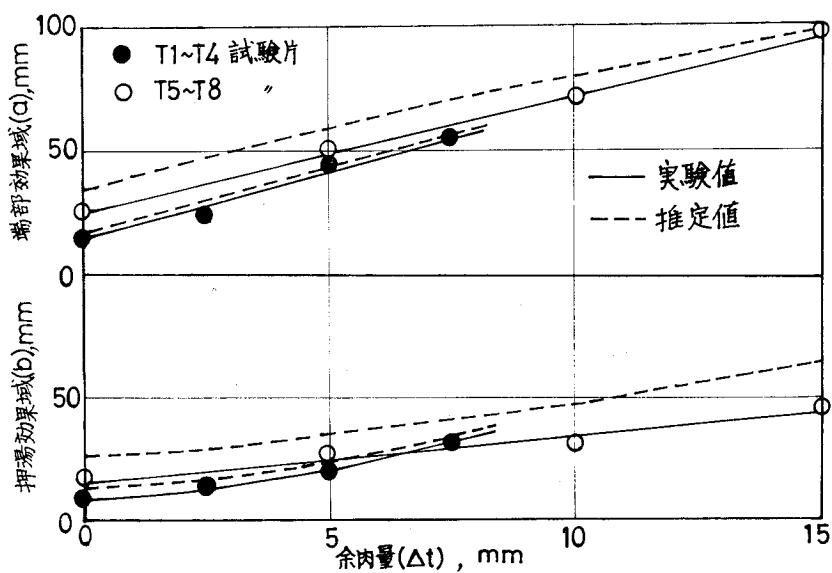
図 4 - 10 No. T1~T8 縦姿勢試験片における余肉量 ( \Delta t ) と 端部効果域 (a) および押湯効果域 (b) の関係
