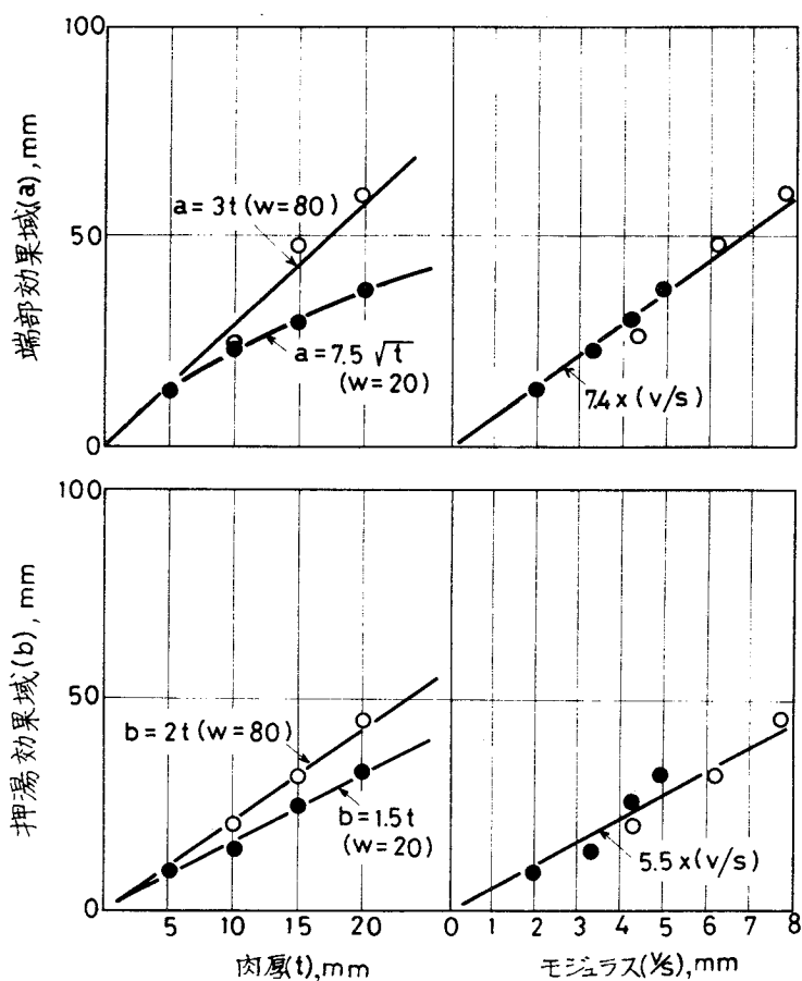
図2-5. 板形状試験片での肉厚 ( t ), モジュラス ( v/s )と 端部効果域 ( a ), 押湯効果域 ( b )との関係 (標準条件: \alpha = 1.4 , T_m = 1600^\circ\text{C} )
