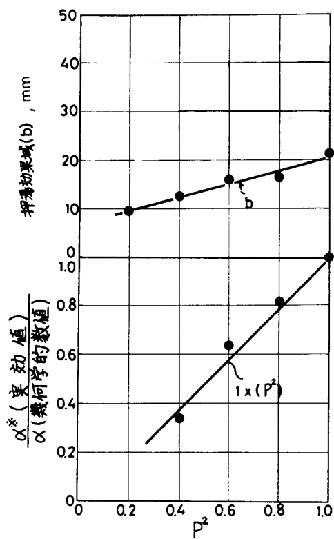
図 2 - 12 板状試験片におけるネック付き押湯での P^2 と 押湯効果域(b), \alpha^*/\alpha との関係 ( \alpha = 2.0 , T_m = 1600^\circ\text{C} )
