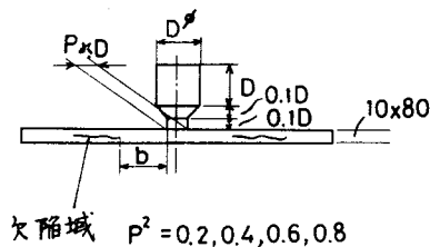
(3) ネック付押湯試験片
