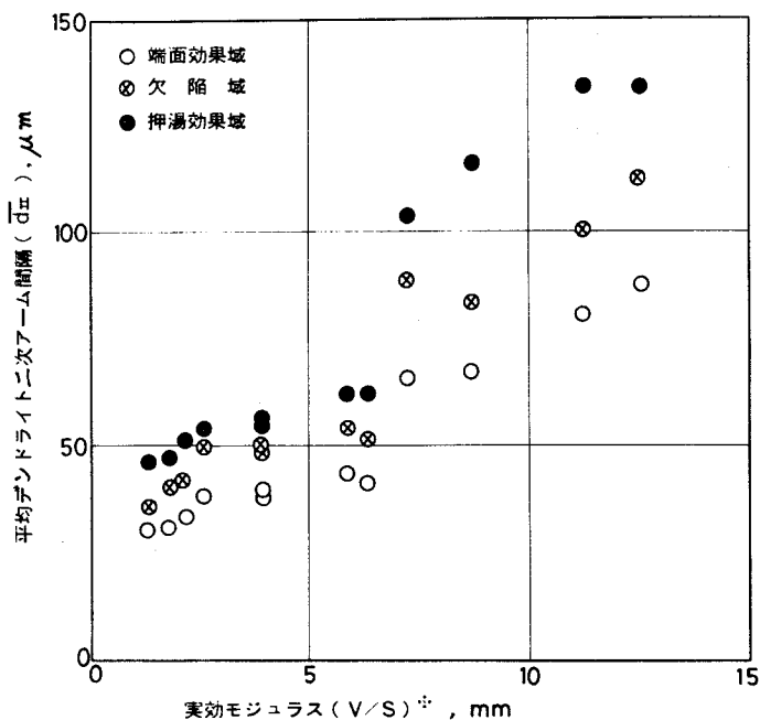
図 5-9 各領域での実効モジュラス ( v/s ) * と平均デンドライト二次アーム間隔 ( \overline{d_{II}} ) の関係
