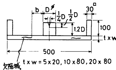
(2) 盲押湯試験片
