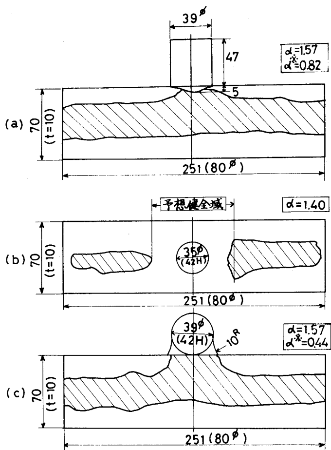
図2-15 各種円筒試験片（展開図）での欠陥発生状況 ( T_m = 1600^\circ\text{C} )
