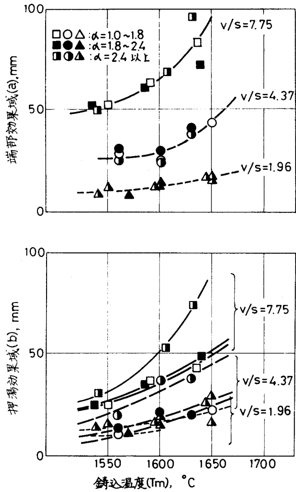
図 2 - 8 板状試験片での鋳込温度 ( T_m ) と端部効果域 (a), 押湯効果域 (b) との関係
