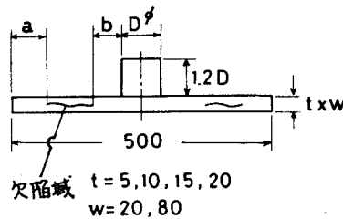
(1) 標準試験片
