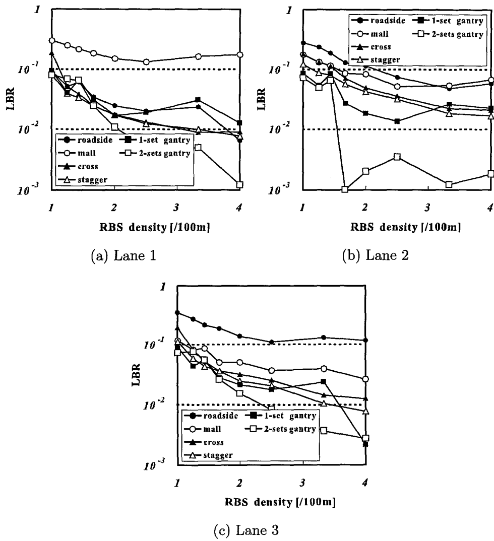
図 4.9 RBS 密度に対する通信遮断率 (Congested flow, h_b=6\text{m} )
