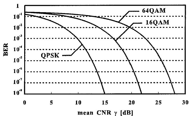
図 3.3 直交振幅変調方式の BER
