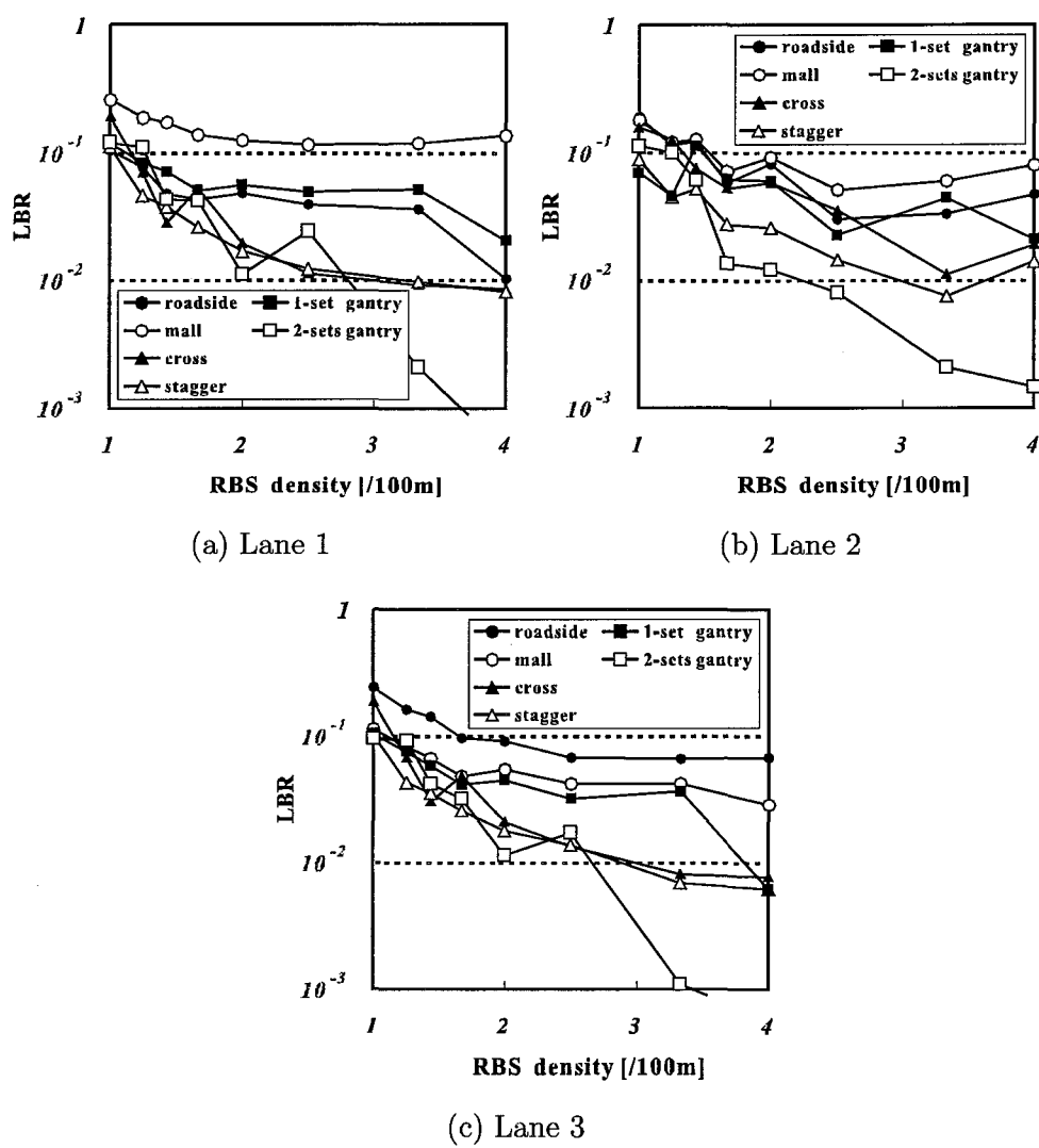
図 4.6 RBS 密度に対する通信遮断率 (Free flow, h_b=6\text{m} )
