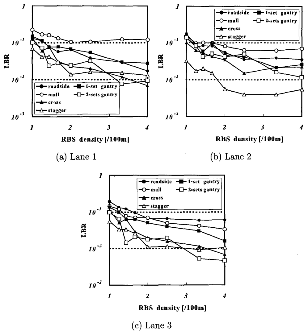
図 4.7 RBS 密度に対する通信遮断率 (Free flow, h_b=12\text{m} )
