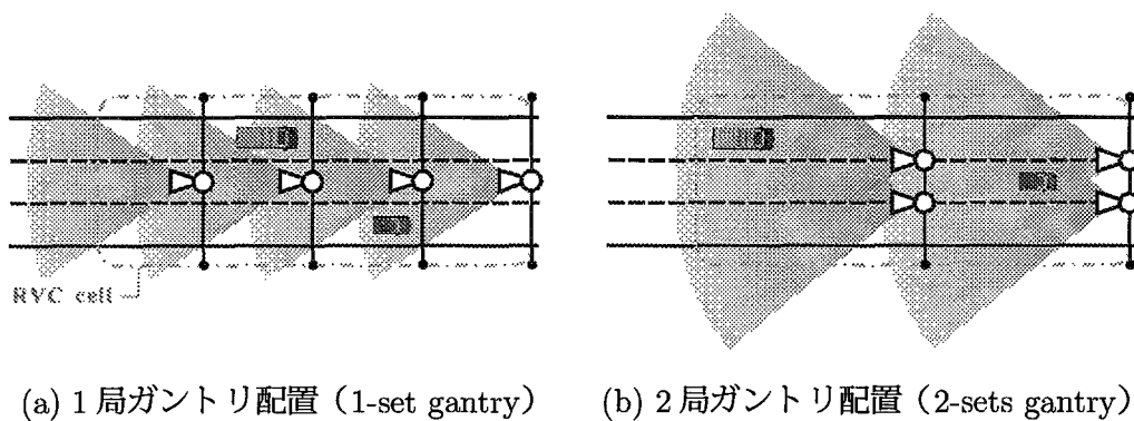
図 4.4 ガントリ RBS 配置
