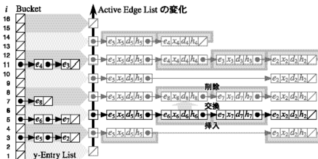
図 2.5 Active Edge List の作成
