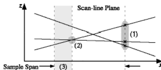
図 4.5 サンプルスパンの分割
