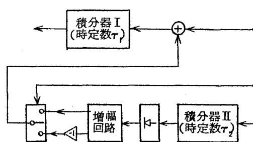
図2.9 改良2重積分形定差変調の局部復号回路の構成図
