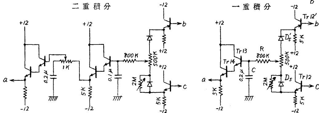
図 3 . 1 1 定差標本化変調試作装置の回路図
