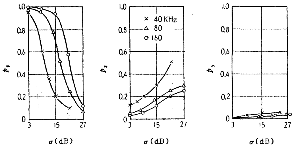
図5.5 擬似音声信号に対する遷移確率
