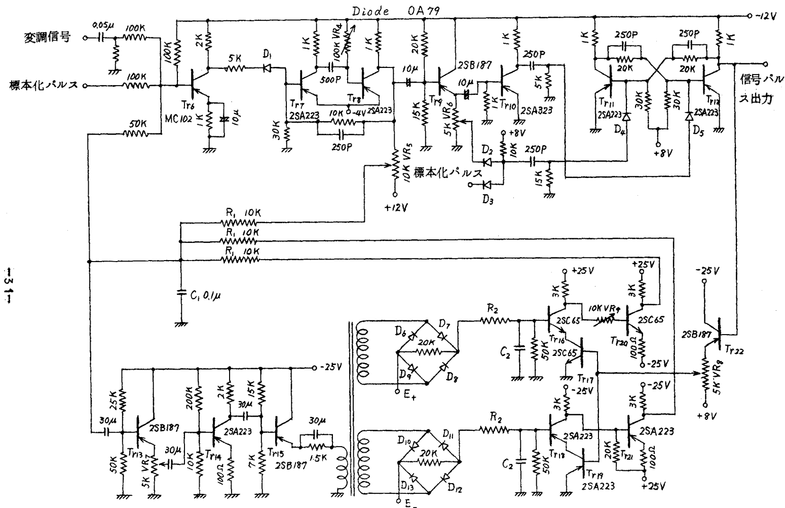
図 2 . 1 9 (b) 圧伸定差変調試作装置の回路図
