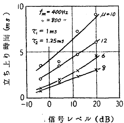
図 2.18 シュミレーションによる過渡特性
