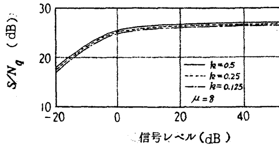
図 2.15 合成信号に対する S/N 比特性
