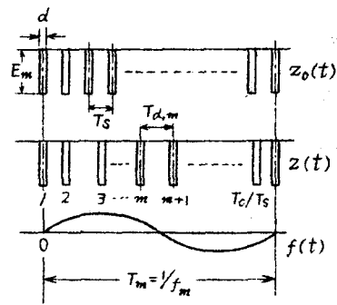
図4.5 PIM波と変調信号との 関係
