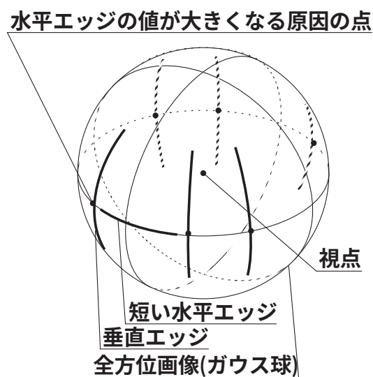
図 5.25: エッジの間違った偏り
