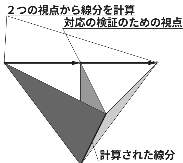
図 5.26: 線分の三次元再構築の基本原理
