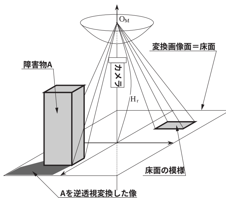
図 4.1: 床面方向への変換
