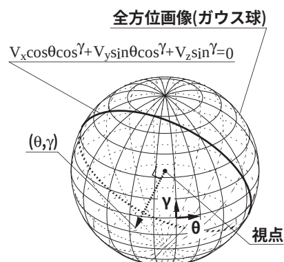
図 5.20: 極座標
