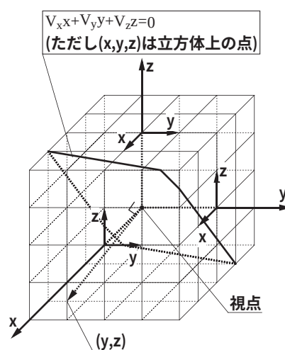
図 5.22: 立方体座標
