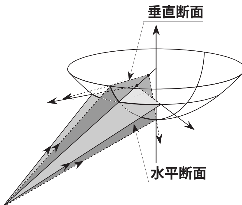
図 2.7: 非点収差
