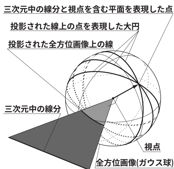
図 5.18: 大円の交点
