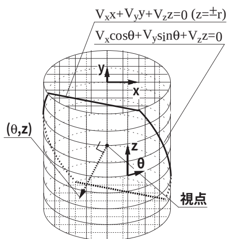
図 5.21: 円柱座標
