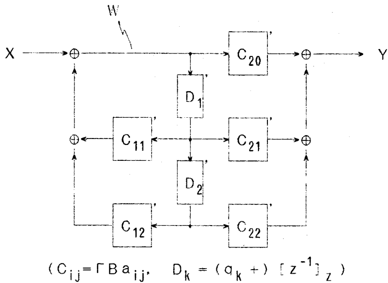
(a) 原回路
