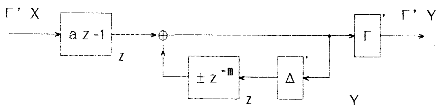
(b) 等価回路
