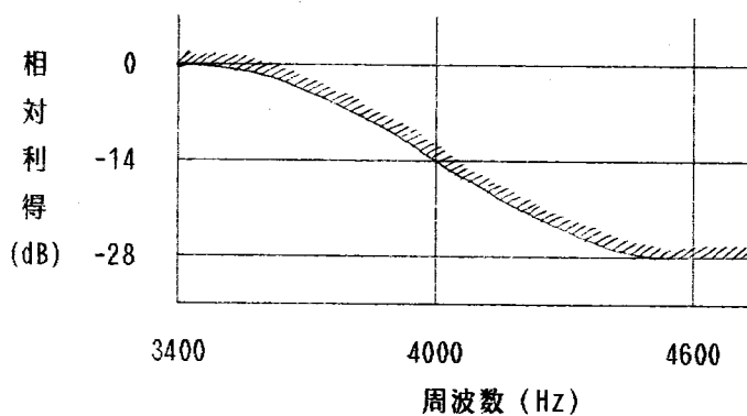
(b) 帯域内伝送特性
