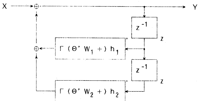
(a) 直接形
