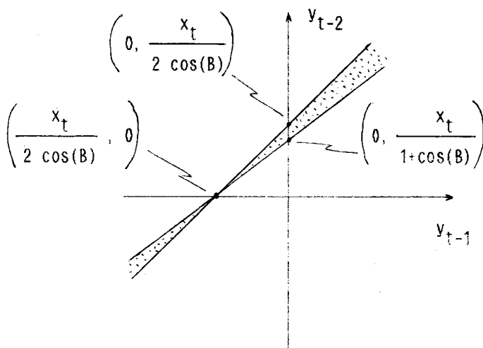
図3. 15 出力の勾配による量子化切換えで蓄積エネルギーが増加する領域（定数入力）
