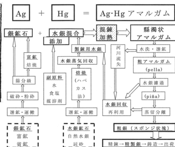
図 5 ポトシ鉱山の銀製錬プロセスの工程図
