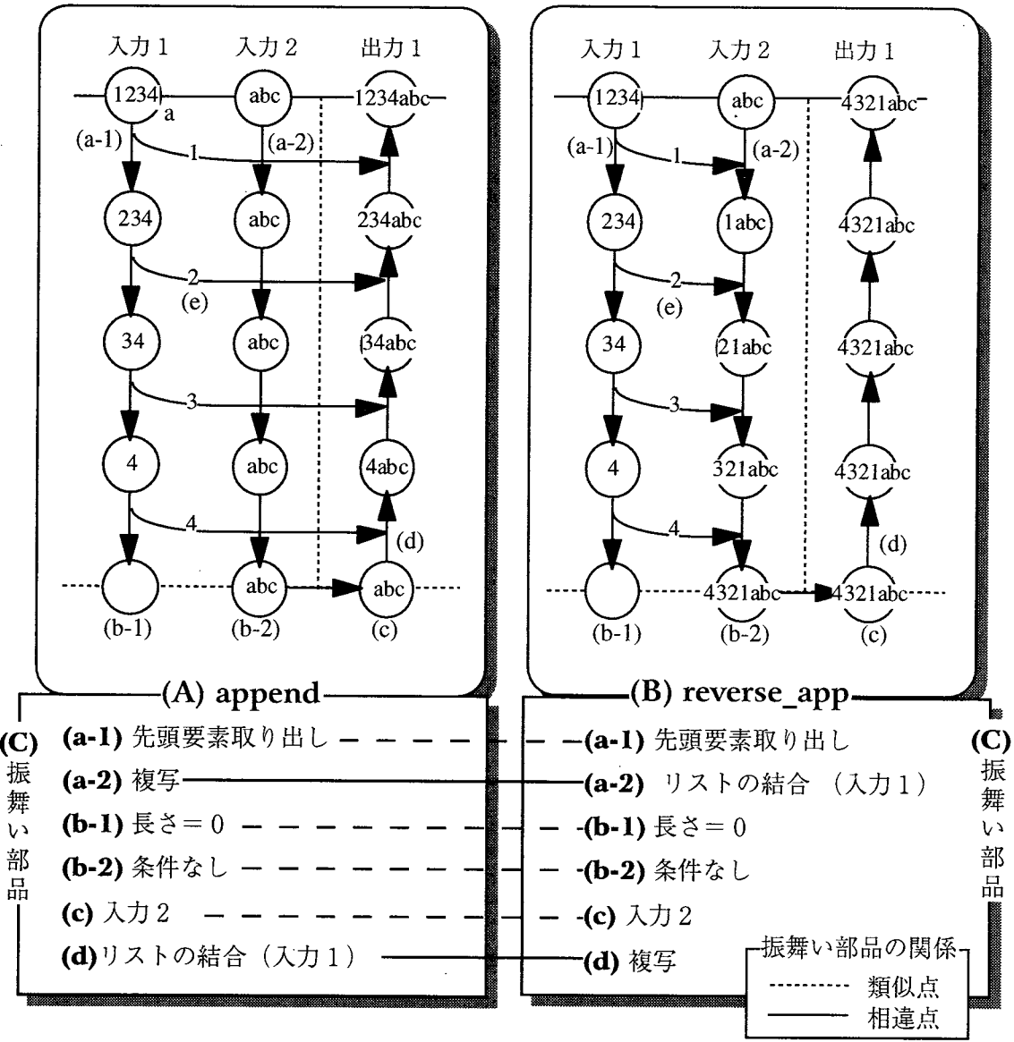
図 3.3 append と reverse_app の U-behavior における類似点・相違点
