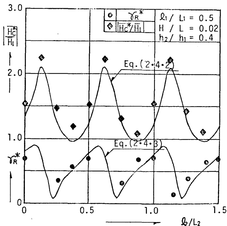
図-2.4.6 |\bar{H}_c^*/\bar{H}_l| と \gamma_R^* に及ぼす l_2/L_2 の効果 ( l_1/L_1 = 0.5 の場合)
