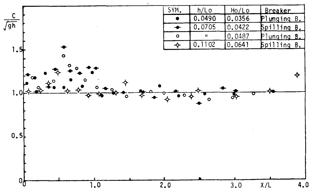
図-1・3・21 砕波後の波速（微小振幅波の波速との比較）
