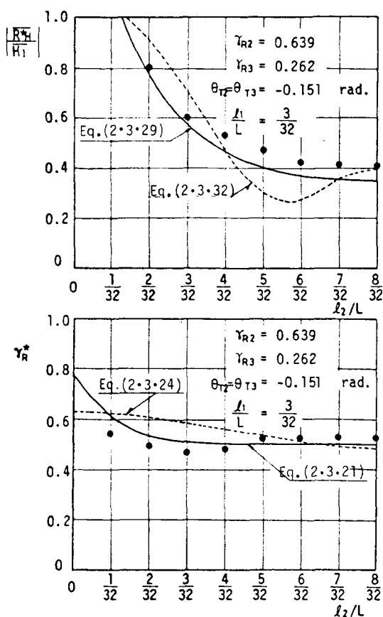
図-2.3.29 \gamma_R^* と |\bar{R}_H^*/\bar{H}_I| と l_2/L の関係 ( l_1/L = 3/32 の場合)
