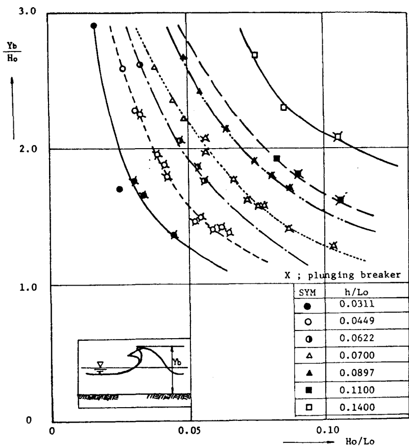
図-1・3・8 砕波峰高
