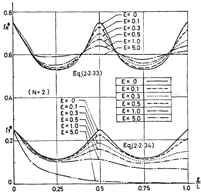
図-2.2.20 \gamma_R^* と \gamma_T^* に及ぼす l/L の効果
