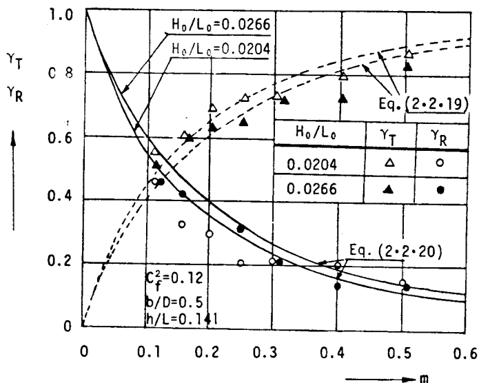
図-2・2・11 \gamma_R と \gamma_T に及ぼす m と H_0/L_0 の効果 ( h/L = 0.141 の場合)
