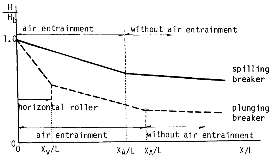
図－１・３・３５ 碎波後の波高減衰の模式図
