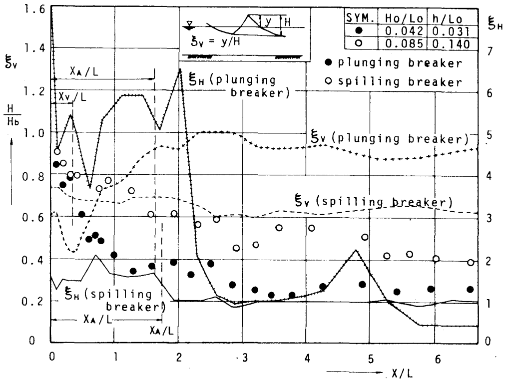
図－１・３・１５ 砕波後の波形変化と波高変化
