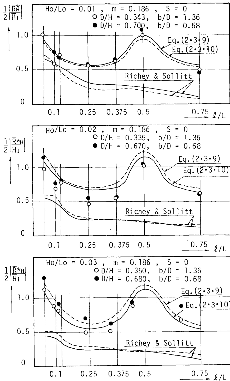
図-2.3.26 不透過壁面での水位変動
