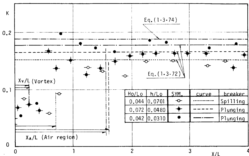
図-1・3・56 平均水位変動の計算値と実験値の比較
