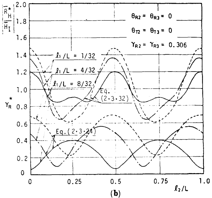
※図-2.3.8 \gamma_R^* と |\bar{R}_H^*/\bar{H}_I| に及ぼす l_2/L の効果 ( r_{R2} = r_{R3} = 0.306 の場合)
