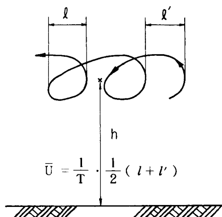
図-1・3・19 残留速度 \bar{U} の定義
