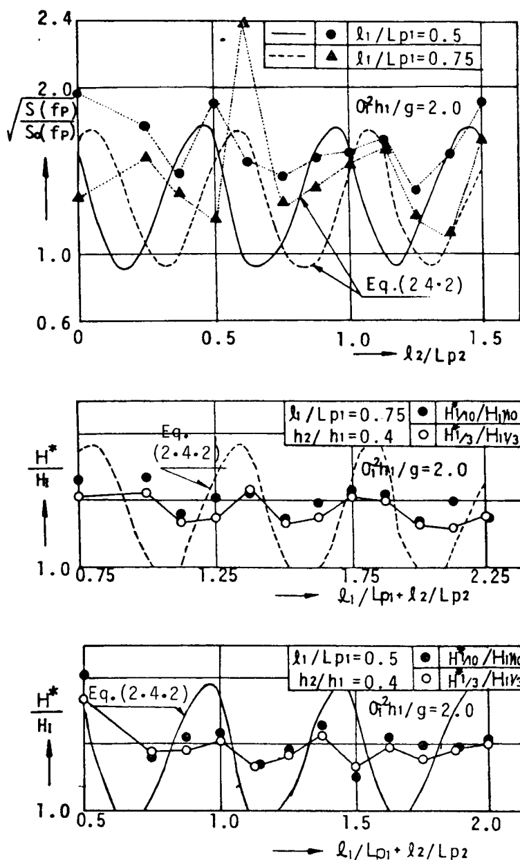
図-2.4.11 海岸堤防前面波高に及ぼす離岸堤の設置距離 ( l_1/L_1 + l_2/L_2 ) の効果 (不規則波の場合)
