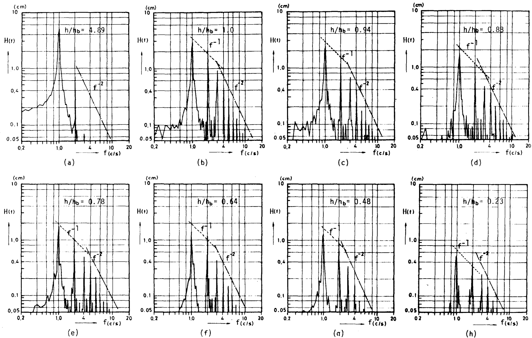
図-1・3・30 成分波高スペクトルの変化 ( S = 1/40 , H_0/L_0 = 0.049 , T = 1.0 \text{ sec} の場合)
