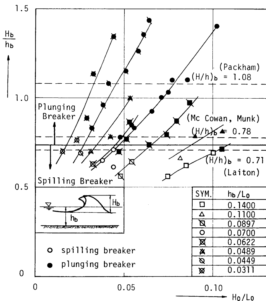
図-1.3.7 碎波波高
