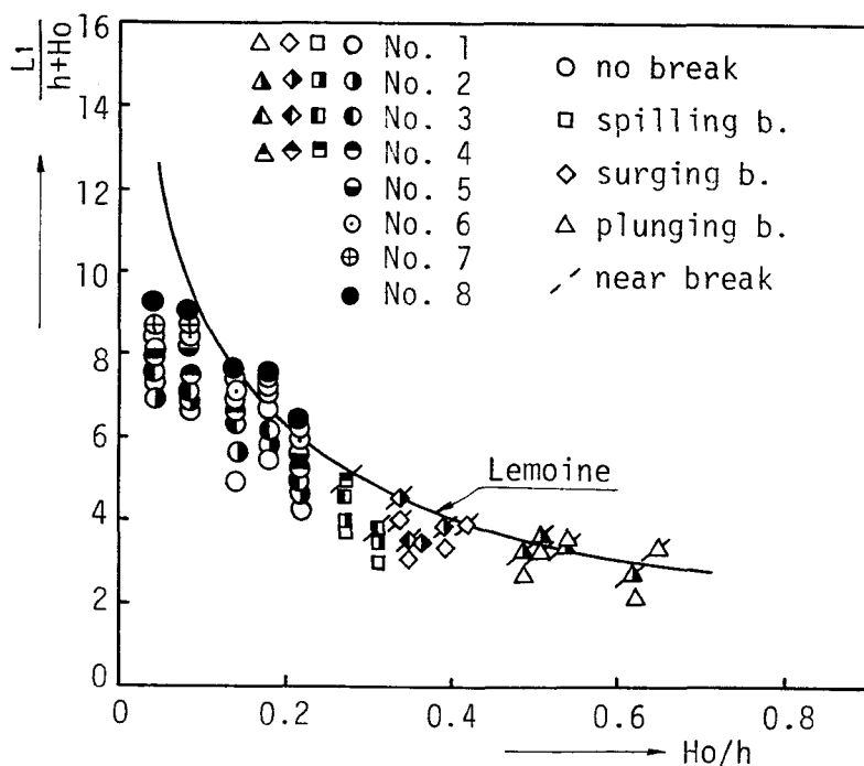
図-1・2・14 分散波の波長と段波波高との関係
