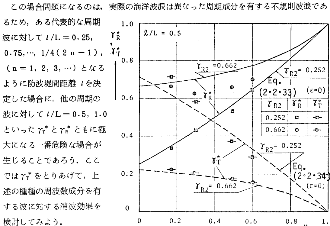
図-2・2・27 \gamma_T^* と \gamma_R^* に及ぼす \gamma_{R1} の効果 ( l/L = 0.5 , \gamma_{R2} = 0.252, = 0.662 の場合)
