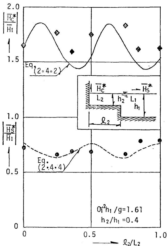
図-2.4.4 |\bar{H}_C^*/\bar{H}_1| と |\bar{H}_S^*/\bar{H}_1| に及ぼす l_2/L_2 の効果
