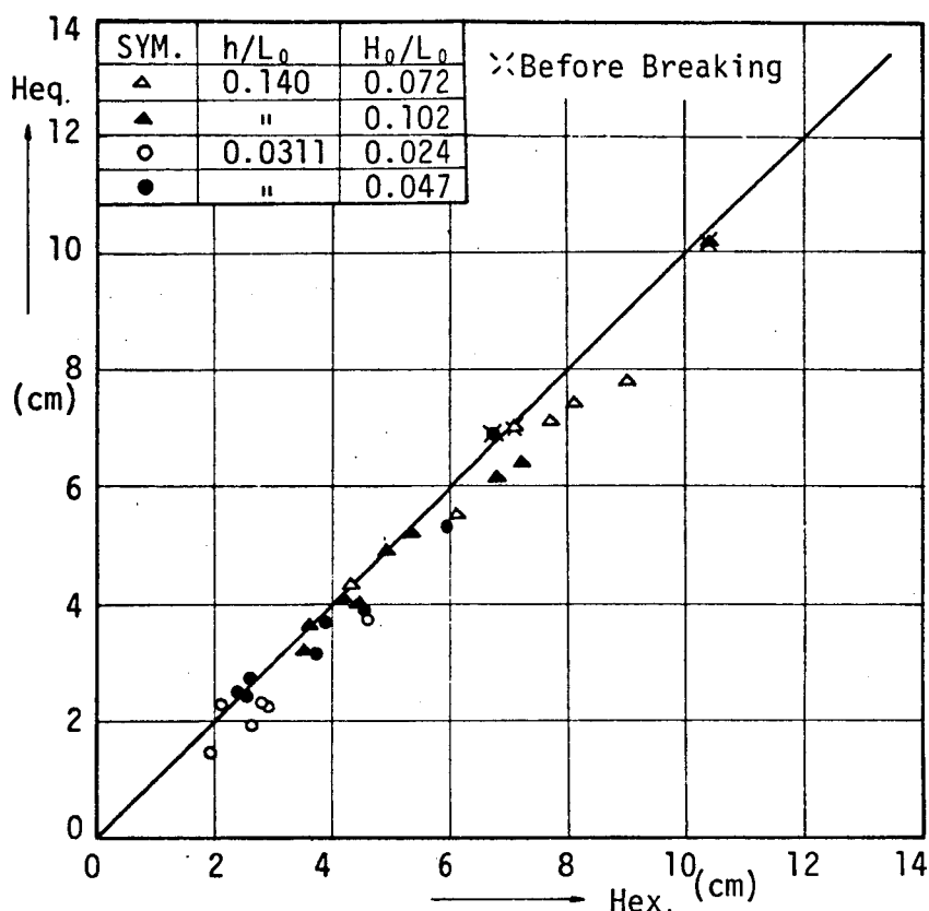
図-1・3・34 H_{eq.} と H_{ex.} の関係
