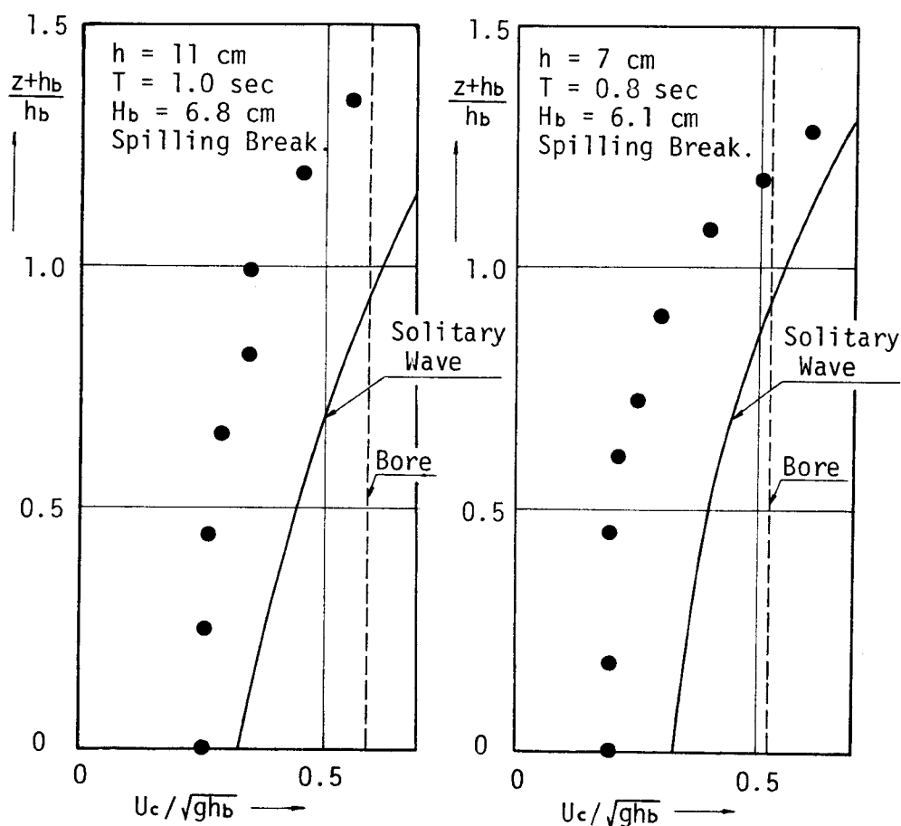
図- 1.3.16 砕波時の水粒子の水平方向流速（波峰）
