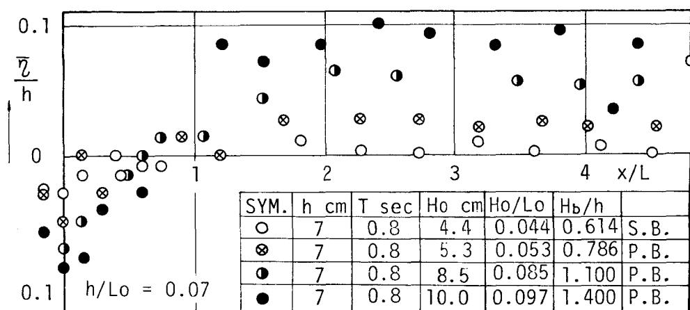
図-1.3.9 波の伝播に伴う \bar{\eta}/h の値の変化
