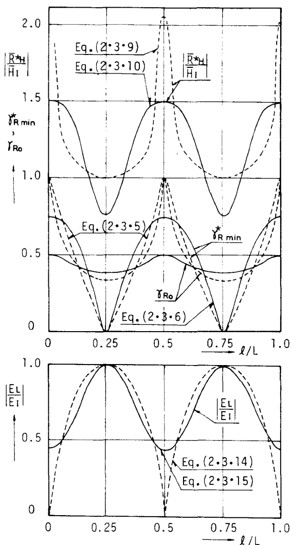
図-2.3.16 r_{R0} の値と (\gamma_R^*)_{\min} , |\bar{R}_H^*/\bar{H}_I| , E_L/E_I の関係 ( \epsilon = 0 , \theta_T = 0 の場合)
