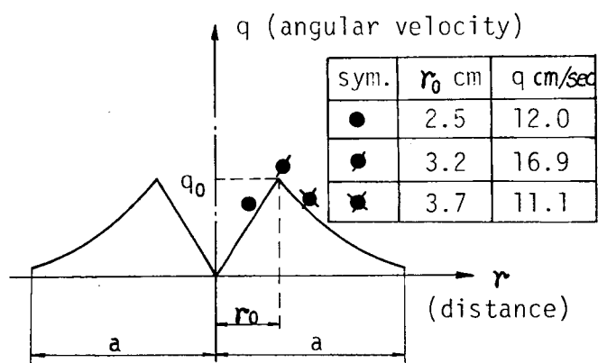
図-1.3.37 horizontal roller の回転角速度
