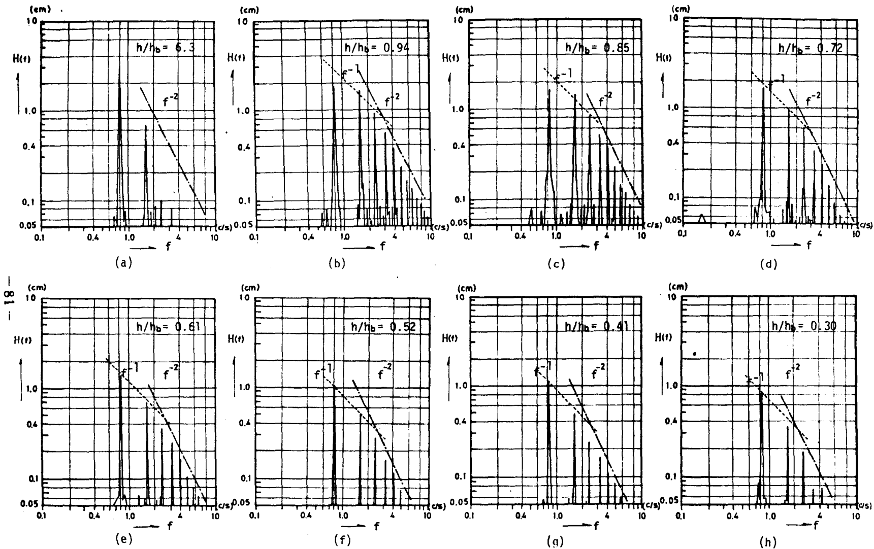
図-1・3・29 成分波高スペクトル ( S=1/25 , H_0/L_0=0.015 , T=1.22\text{sec} の場合)
