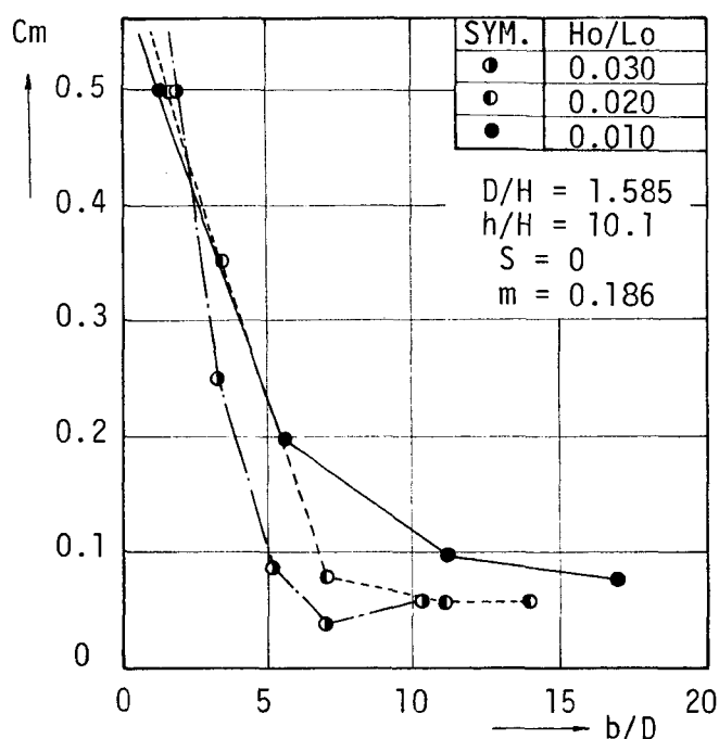
図-2・2・5 b/D の変化に伴う C_m の変化
