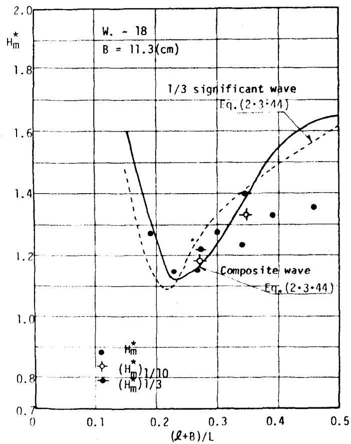
図-2.3.53 H_m^* と R_m^* と (l+B)/L あるいは l/L との関係 (W. = 18 の不規則波)
