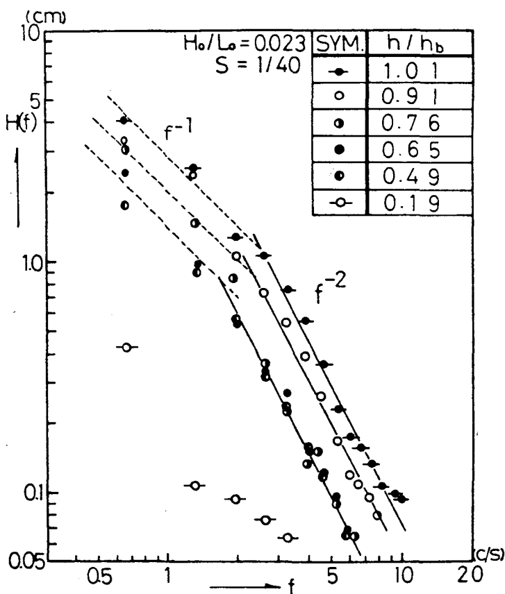
図-1・3・32 成分波高スペクトル(卓越成分波)
