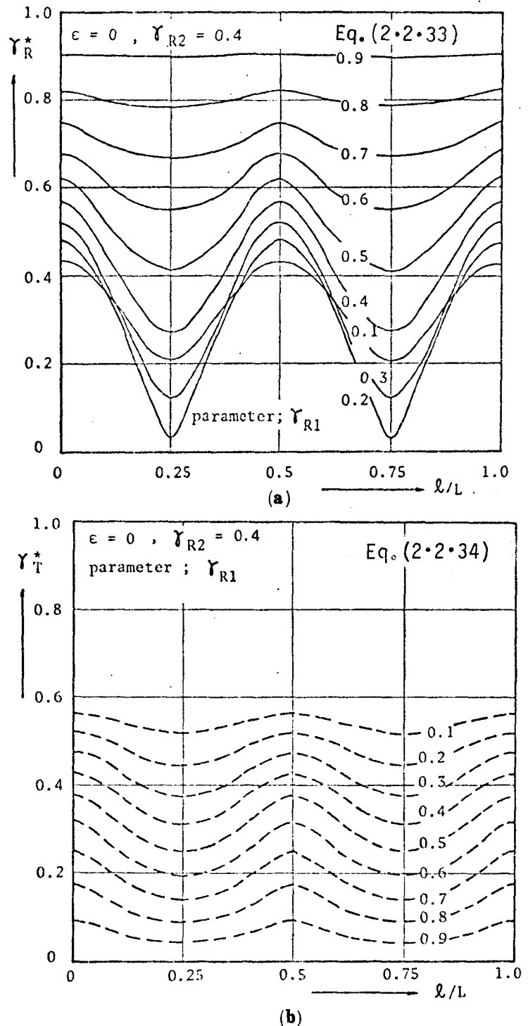
図-2.2.19 \gamma_R^* と l/L の関係 ( \gamma_{R2}=0.4 の場合)
