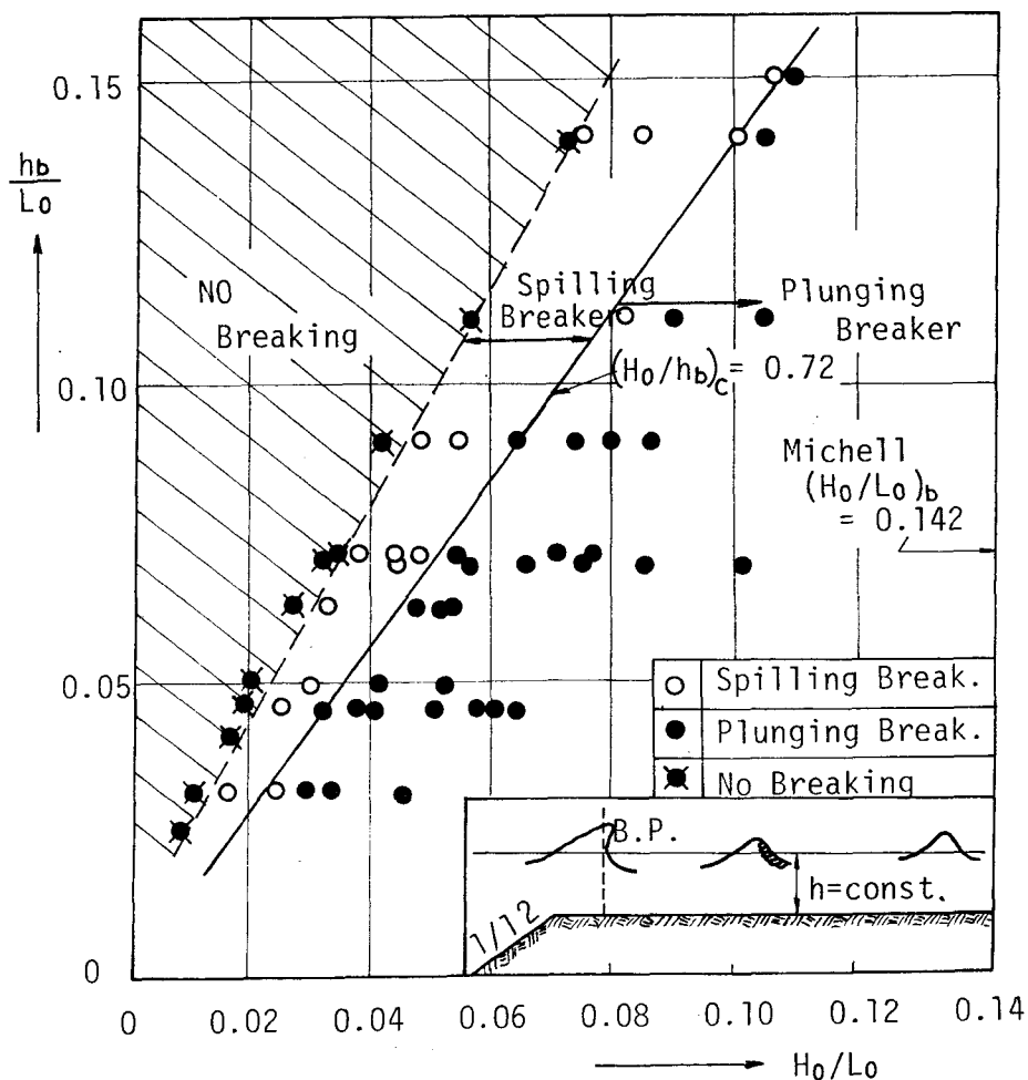
図-1.3.2 砕波型式 ( S = 0 の場合)
