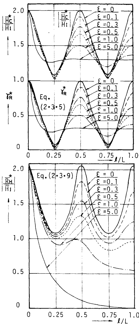
図-2.3.2 l/L に伴う |\bar{H}_c^*/\bar{H}_i| , \gamma_R^* , |\bar{R}_h^*/\bar{H}_i| の変化 (無限の繰返し, r_R = 0.3 , r_T = 0.7 の場合)
