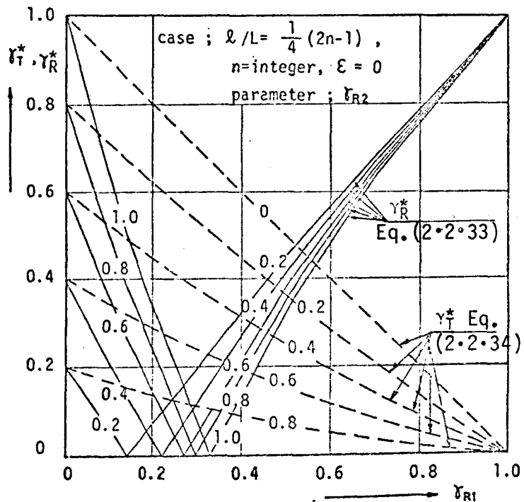
図-2.2.21 \gamma_R^* と \gamma_T^* に及ぼす \gamma_{R1} と \gamma_{R2} の効果
