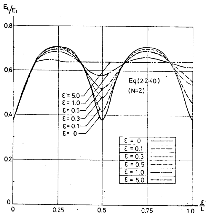
図- 2.2.22 E_L/E_I に及ぼす l/L の効果について ( n=2 、 \gamma_R=\gamma_{R2}=0.6 、 \gamma_T=\gamma_{T2}=0.4 の場合)
