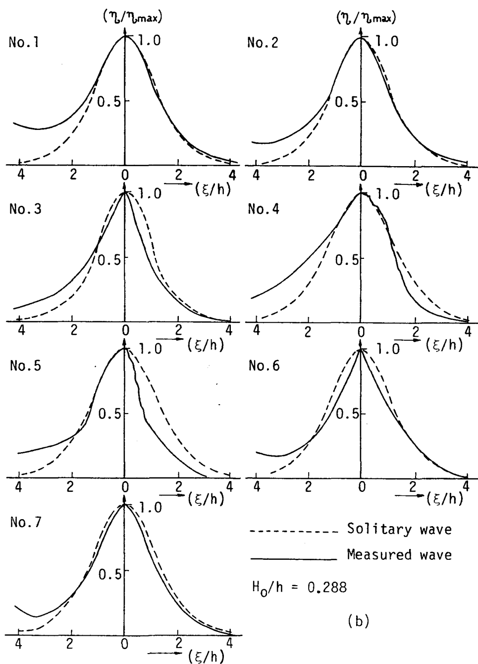
図-1.2.5(b) 計測波形と孤立波形の比較の一例
