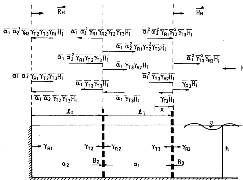
図-2.3.7 波の反復反射の状況
