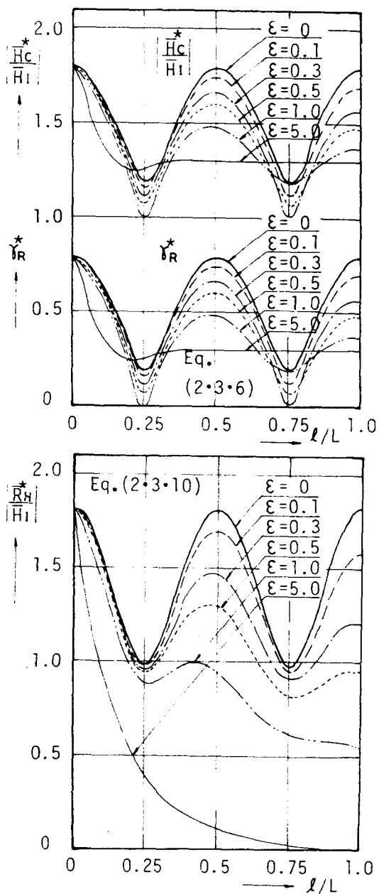
図-2.3.3 l/L に伴う |\bar{H}_c^*/\bar{H}_i| , \gamma_R^* , |\bar{R}_h^*/\bar{H}_i| の変化 (有限な繰返し, r_R = 0.3 , r_T = 0.7 の場合)
