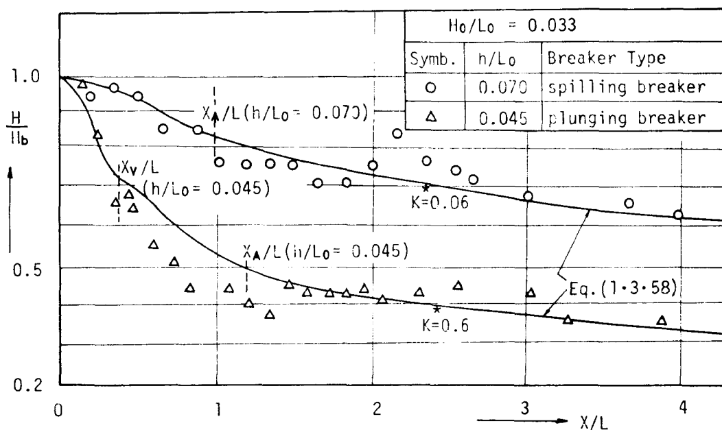
図－ 1・3・55 波高減衰の計算値と実測値の比較
