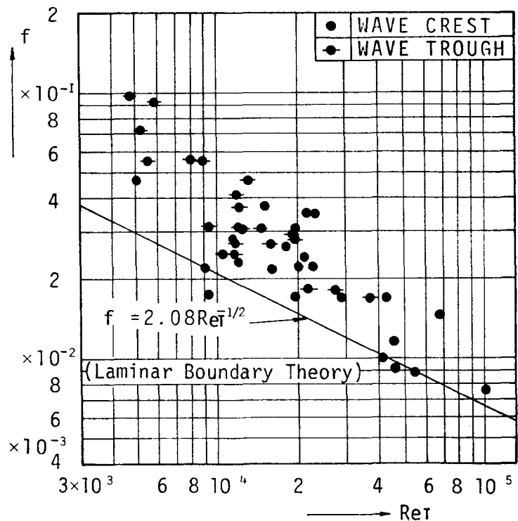
図-1.3.49 f と Re_T の関係
