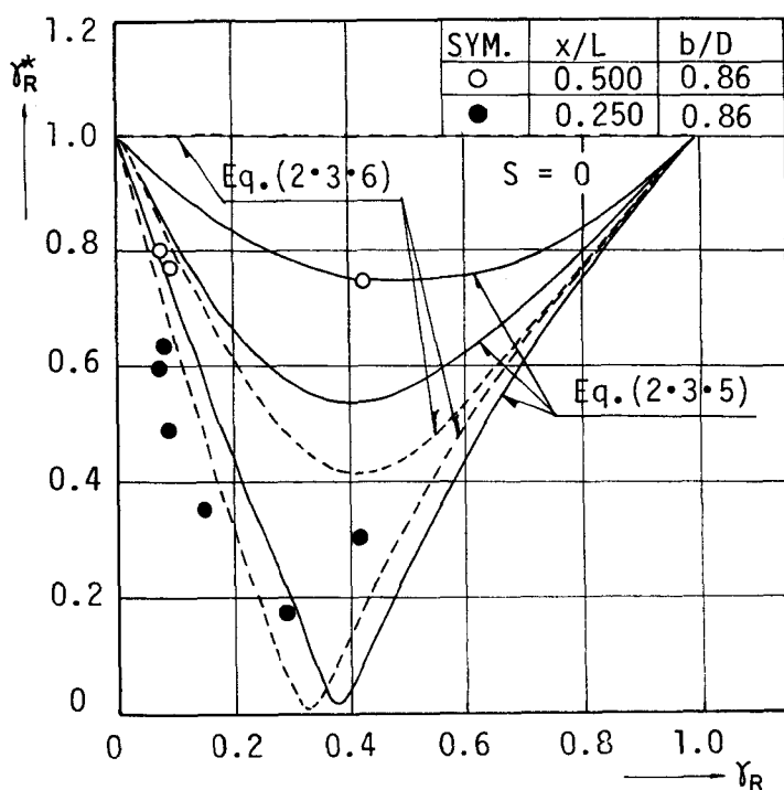
図-2-3-24 \gamma_R^* と r_R の関係 ( \bar{H}_1/L = 0.01, D/\bar{H} = 0.68, h/H = 10.1 の場合)
