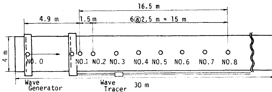
図-1・2・2 実験装置
