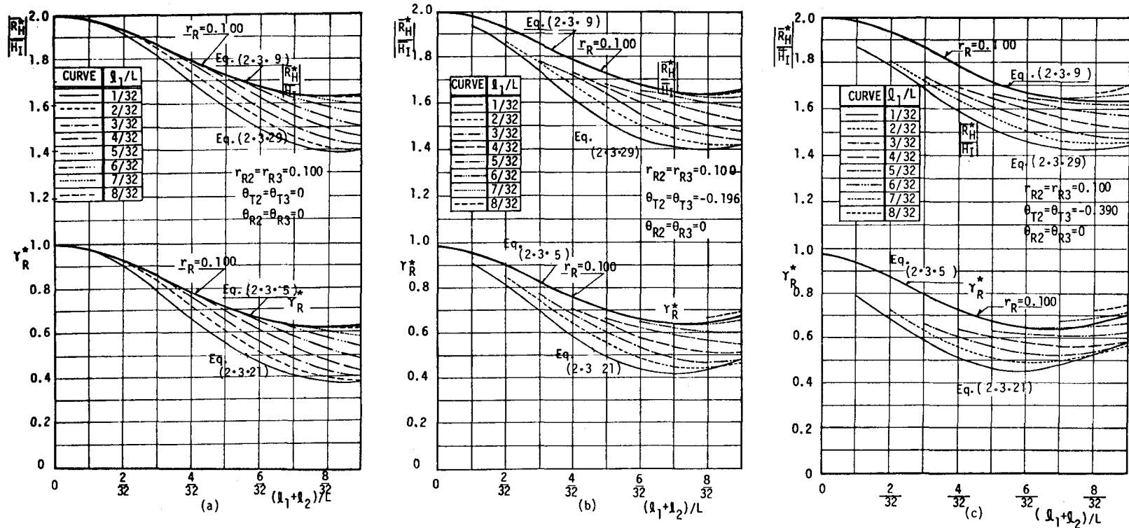
図-2.3.9 \gamma_R^* と |\bar{R}_H^* / \bar{H}_T| と (l_1 + l_2)/L の関係 ( r_{R2} = r_{R1} = 0.100 の場合)
