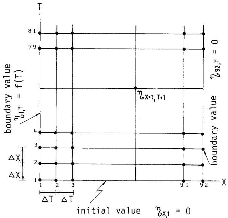
図－１・２・２０ 初期値、境界値と所要解
