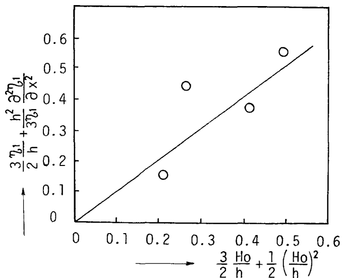
図-1・2・18 波高と曲率の関係
