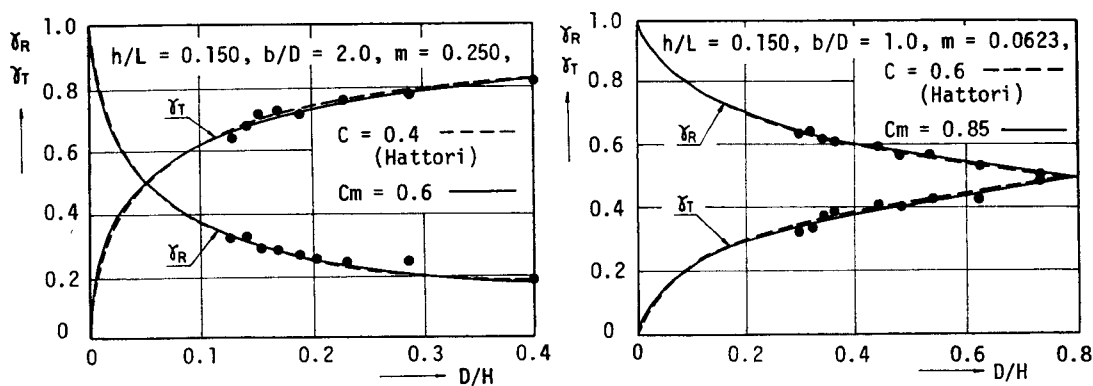
図-2.2.3 \gamma_T と \gamma_R に及ぼす D/H の効果
