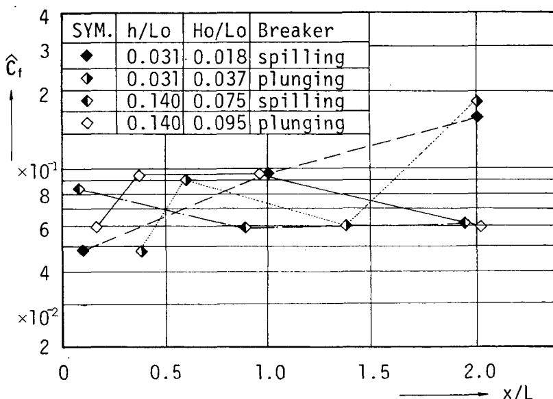
図-1・3・47 \hat{C}_f と x/L の関係
