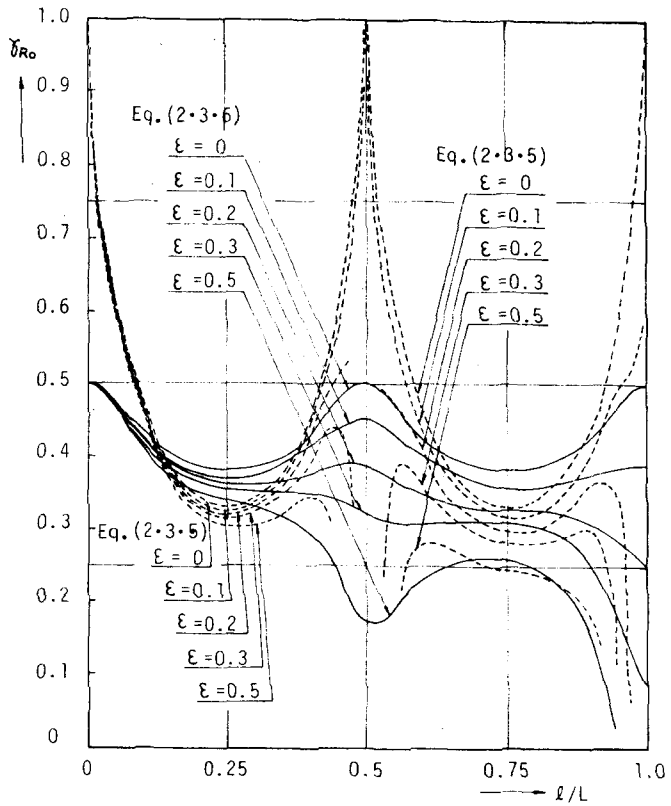
図-2・3・14 \gamma_{R0}^* を最小にする最適な r_{R0} の値 r_{R0} について( \theta_T = 0 の場合)
