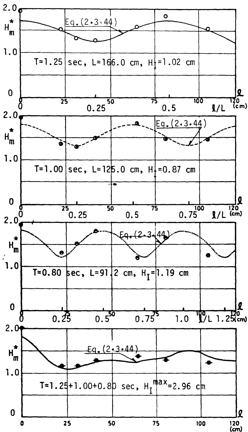
図-2.3.45 (a) H_m^* と l の関係 ( W. - 17 の 3 成分合成波の場合 )
