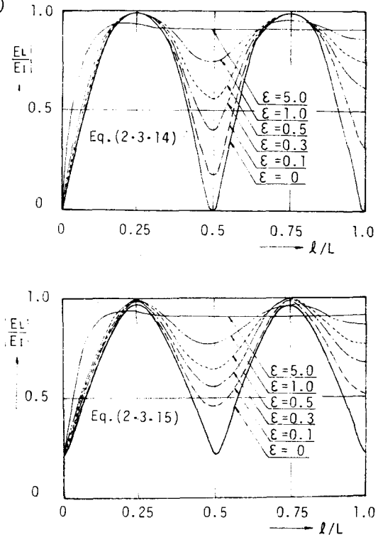
図-2.3.4 E_L/E_I と l/L の関係 ( r_R = 0.3 , r_T = 0.7 の場合)
