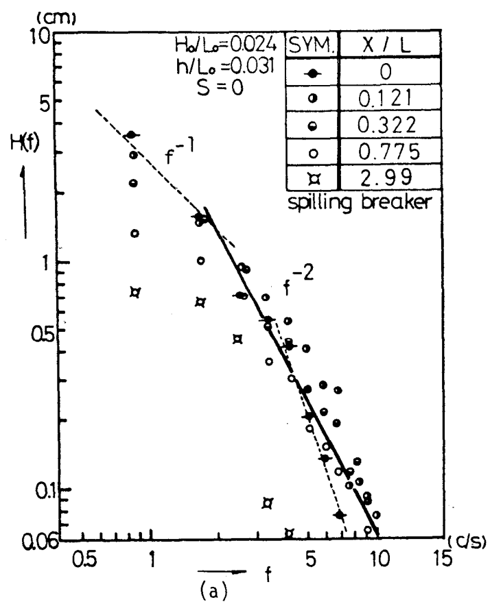
図-1・3・26 成分波高スペクトル(卓越成分波)
