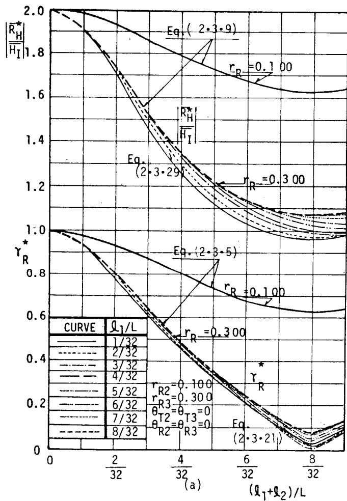
図-2.3.13 \gamma_R^* と |\bar{R}_H^*/\bar{H}_I| と (l_1+l_2)/L の関係, ( r_{R2}=0.100, r_{R3}=0.300 の場合)
