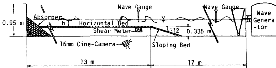
図-1・3・1 実験装置
