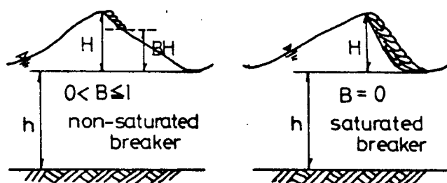
図-1.3.27 non-saturated breaker と saturated breaker の模式図
