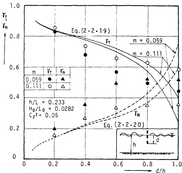
図-2.2.13 \gamma_R と \gamma_T に及ぼす d/h の効果 ( h/L = 0.233 の場合)
