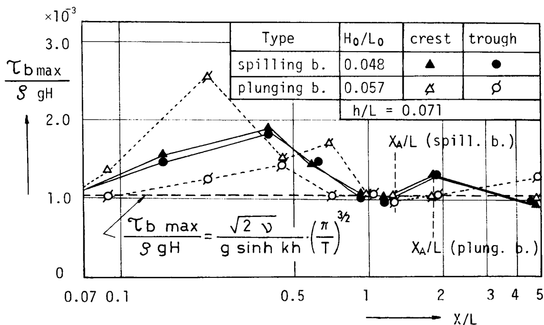
図-1・3・44 \frac{\tau_{b \max}}{\rho g H} と x/L の関係
