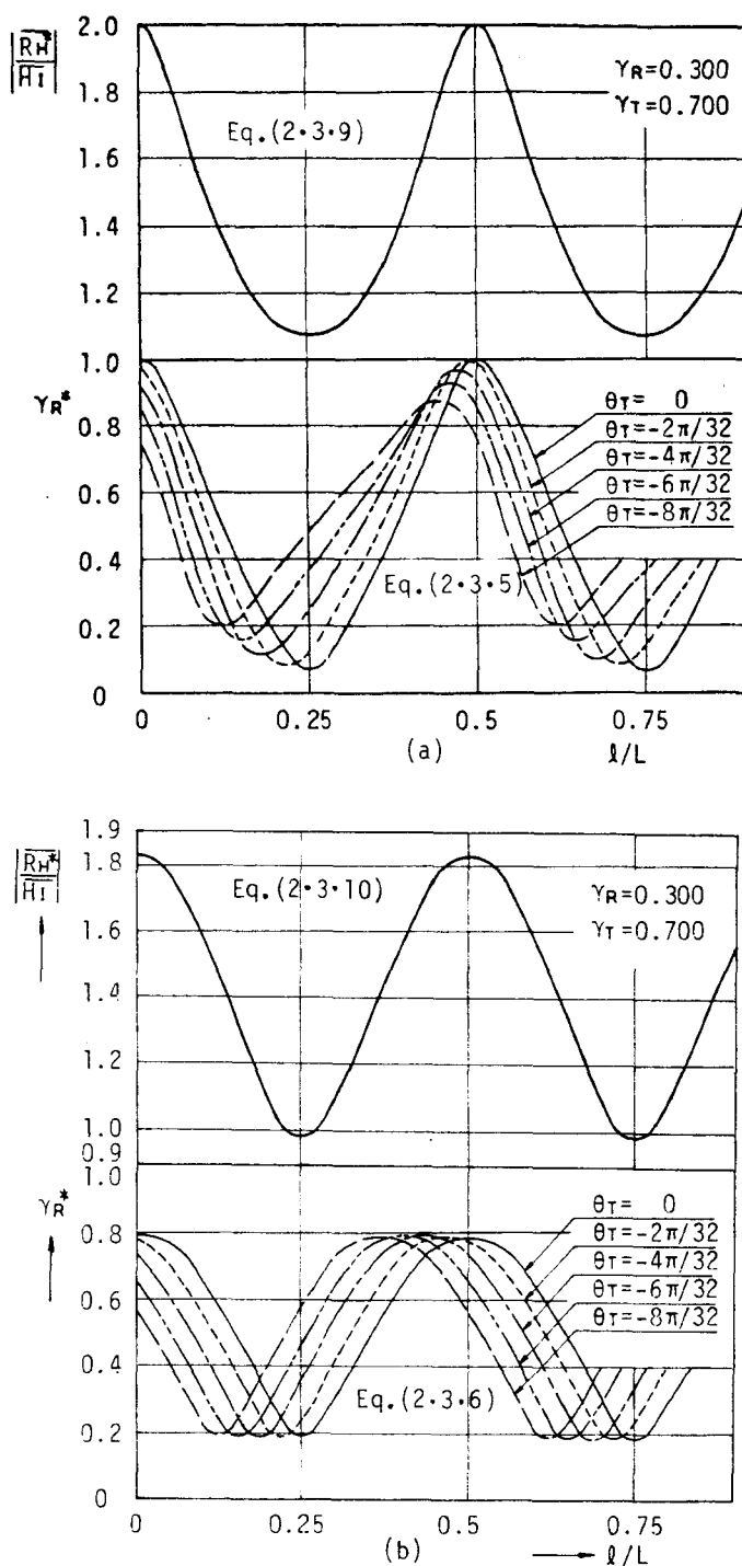
図- 2・3・5 \gamma_R^* と |\bar{R}_H^*/\bar{H}_I| に及ぼす \theta_T の効果 ( r_R = 0.3 , r_T = 0.7 の場合)
