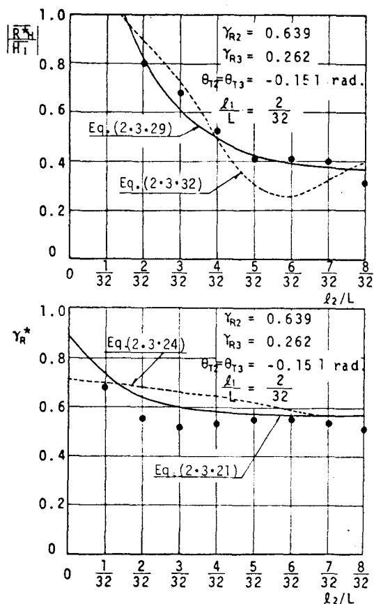
図-2.3.30 \gamma_R^* と |\bar{R}_H^*/\bar{H}_1| と l_2/L の 関係 ( l_1/L = 2/32 の場 合)
