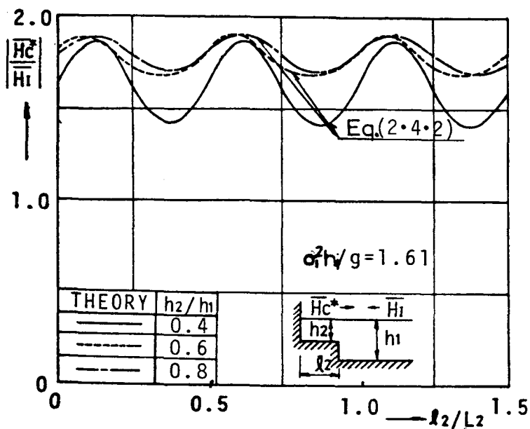
図-2.4.5 |\bar{H}_c^*/\bar{H}_l| に及ぼす h_2/h_1 と l_2/L_2 の効果
