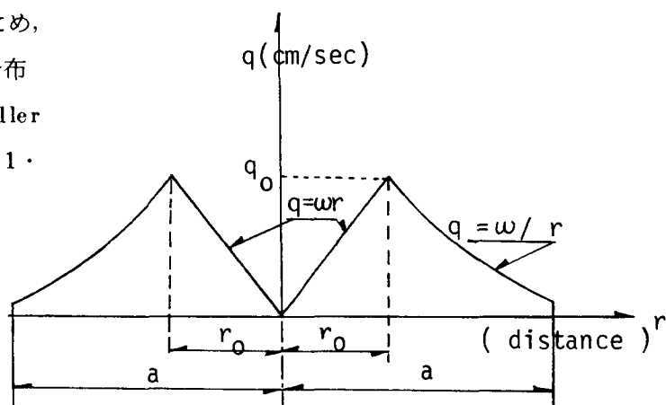
図-1.3.39 Rankine 型 vortex
