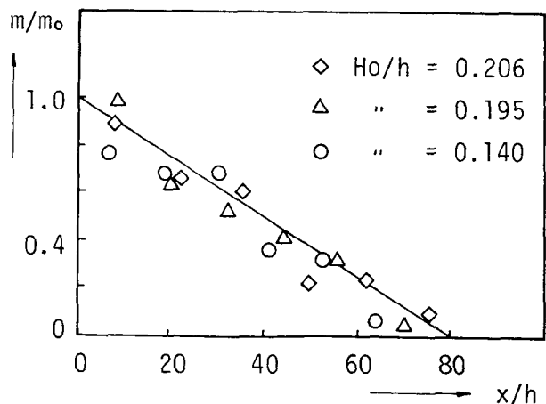
図-1・2・7 波の伝播にともなう m の変化
