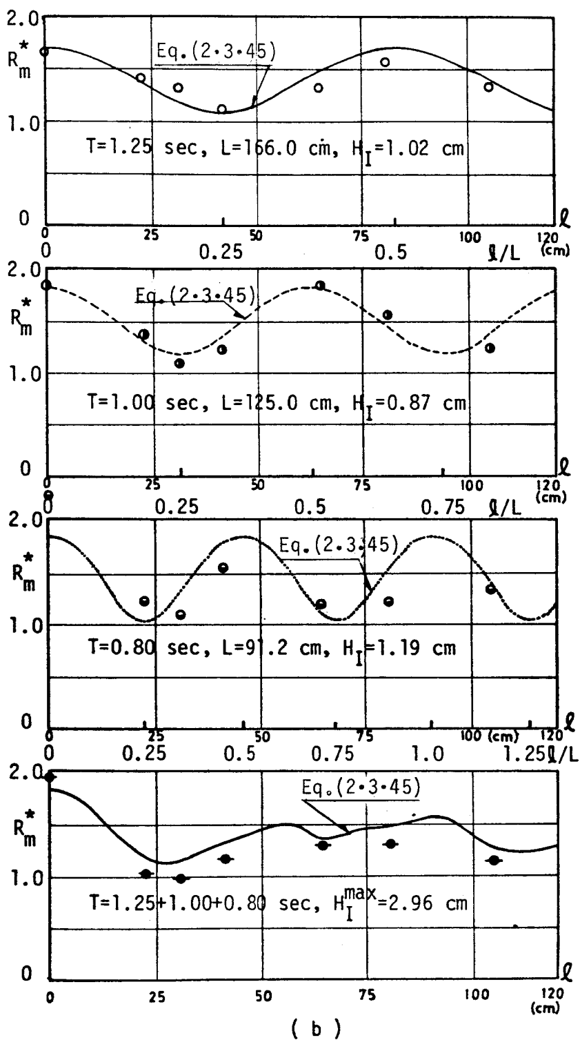
図-2.3.45(b) R_m^* と l の関係 (W.-17 の 3 成分合成波の場合)
