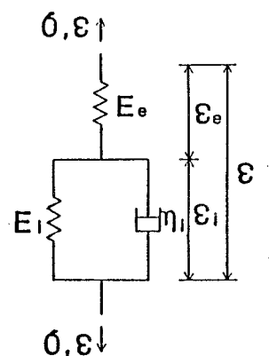
図 5-1 三要素粘弾性モデル
