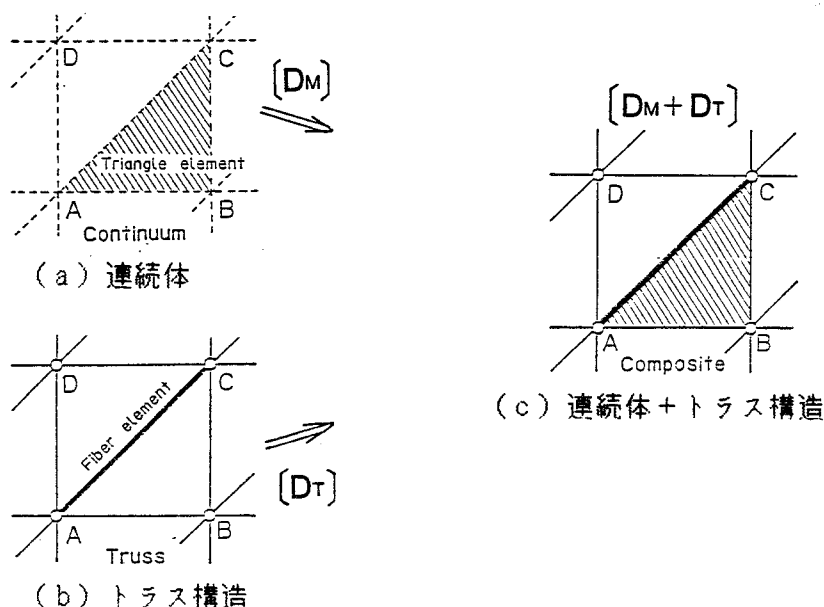
図 7-1 連続体とトラス構造の合成
