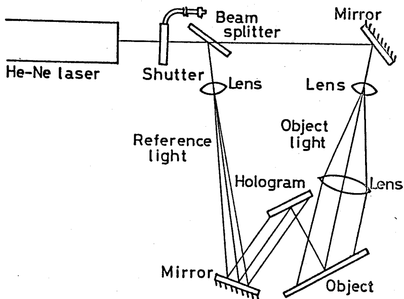
図 2-3-1 ホログラム撮影の光学系
