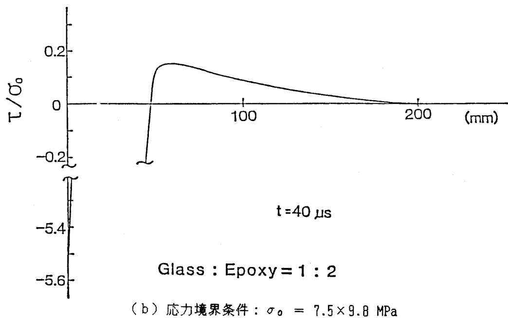
図 3-2 波頭展開法による層間のせん断応力分布
