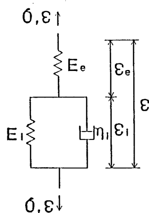
図 6-1 三要素粘弾性モデル
