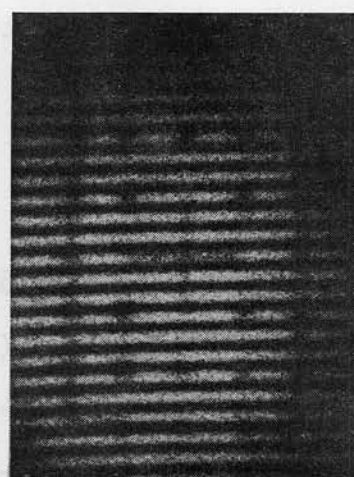
(b) 焦点：干渉じま 図 2-3-4 面内変位のホログラム再生像 ( u = 60 \mu\text{m} の場合)
