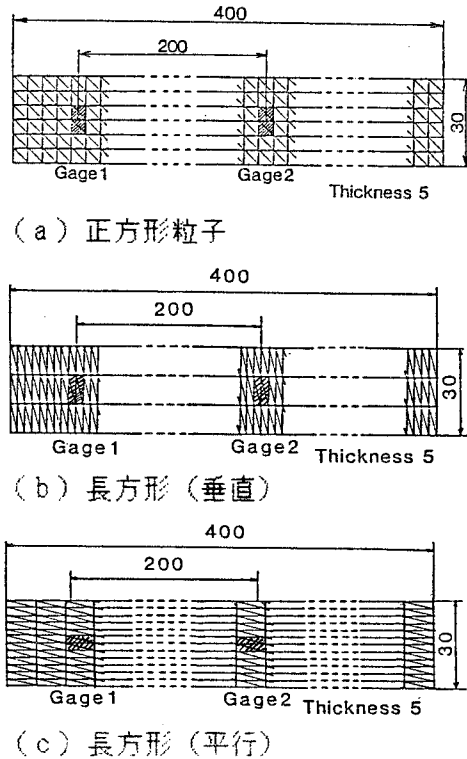
図 6-4 モデル分割
