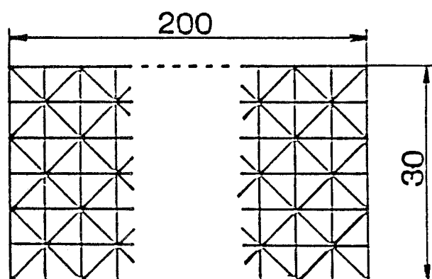
図 4-5 分割モデル
