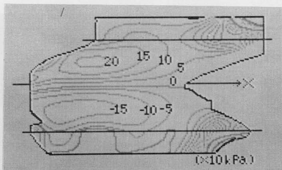
(b) せん断応力分布
