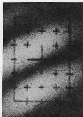
(b) 焦点：干渉じま 図 2-3-3 面内変位のホログラム再生像 ( u = 5 \mu\text{m} の場合)
