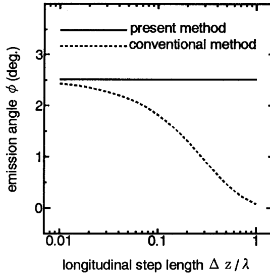
図 2.5 伝搬方向きざみ幅に対する空間ソリトンの放出角 ( P = 30\text{mW/mm} )
