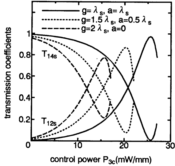
図 4.9 制御光パワに対する信号光の透過特性
