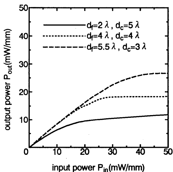
図 5.5 入出力特性
