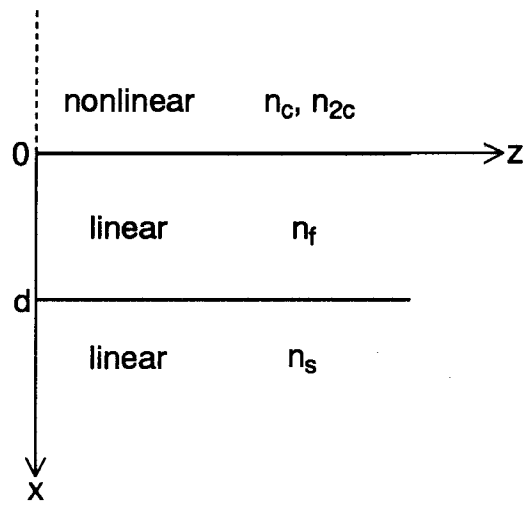
図 2.1 非線形スラブ導波路
