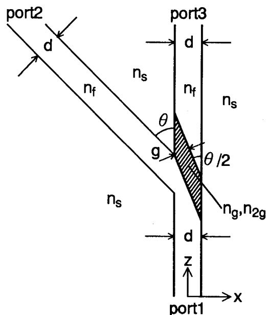
図 3.2 非線形誘電体部を有する非対称光 Y 分岐素子
