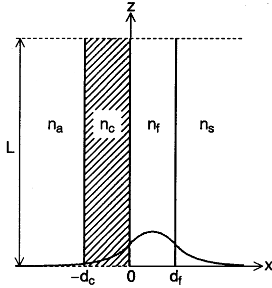
図 5.1 非線形誘電体層を有する導波路型光パワリミタ
