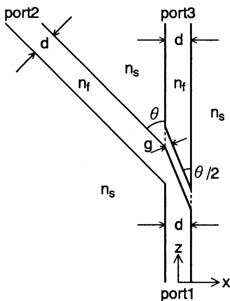
図 3.1 不連続部を有する非対称 Y 分岐線路
