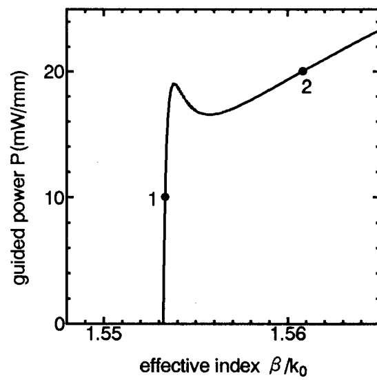
図 2.2 分散曲線
