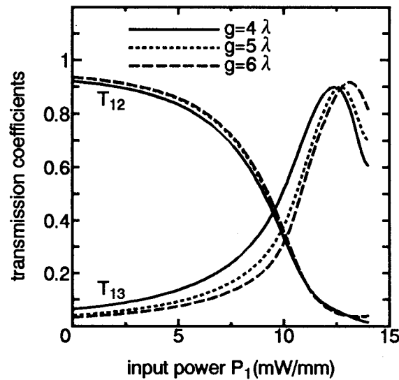
図 3.6 入力パワに対する透過特性
