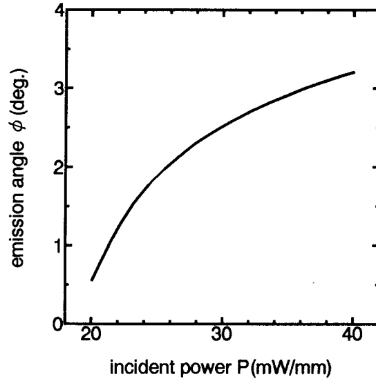
図 2.7 入射パワに対する空間ソリトンの放出角
