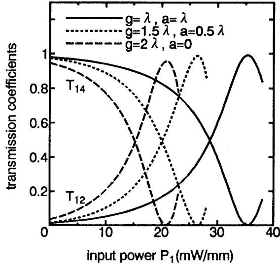
図 4.5 入力パワに対する透過特性
