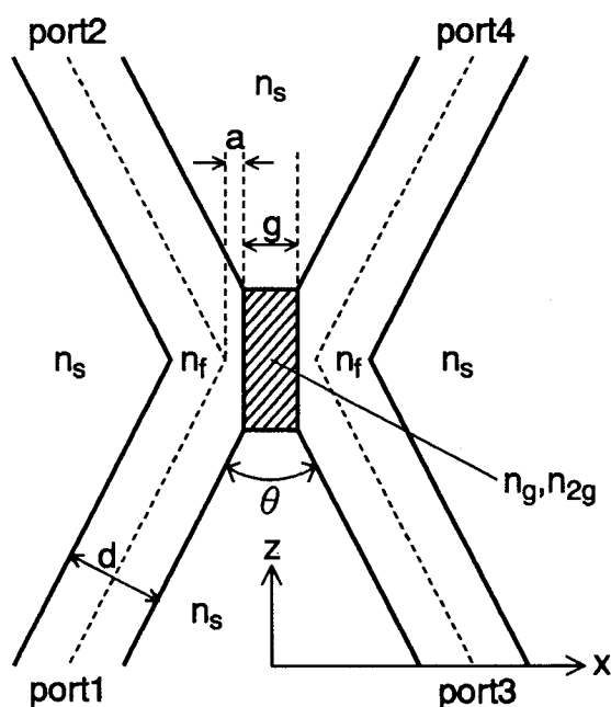
図 4.1 非線形誘電体部を有する X 形光カブラ
