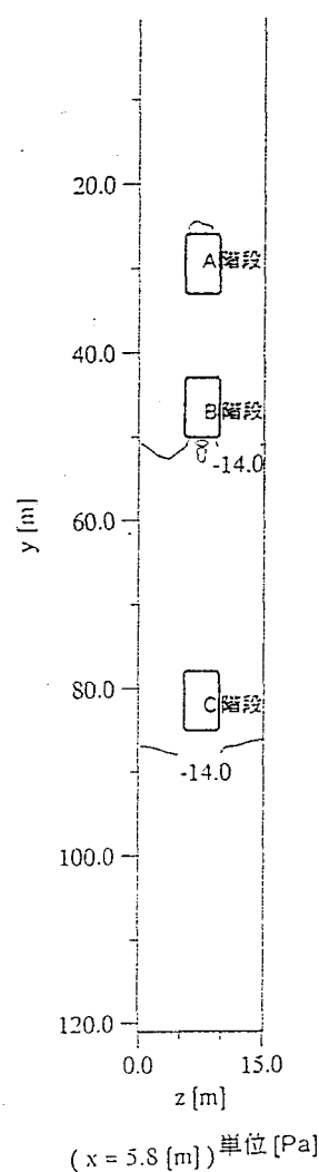
(b) 静圧分布
