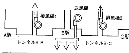
図-4.15 地下鉄系および換気機器の配置
