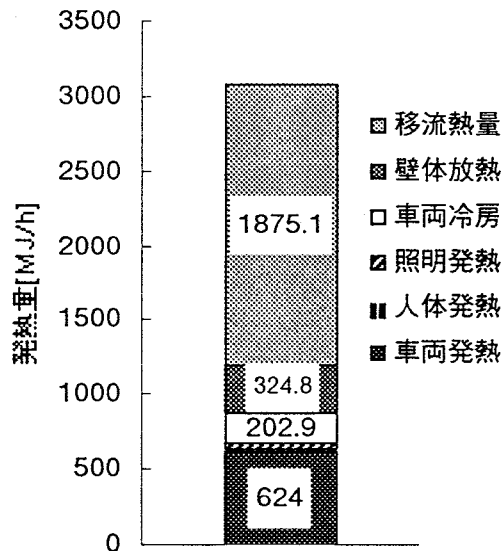
図-5.10 17時の冷房負荷
