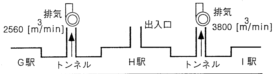
図-2.15 H駅および排風機の位置関係
