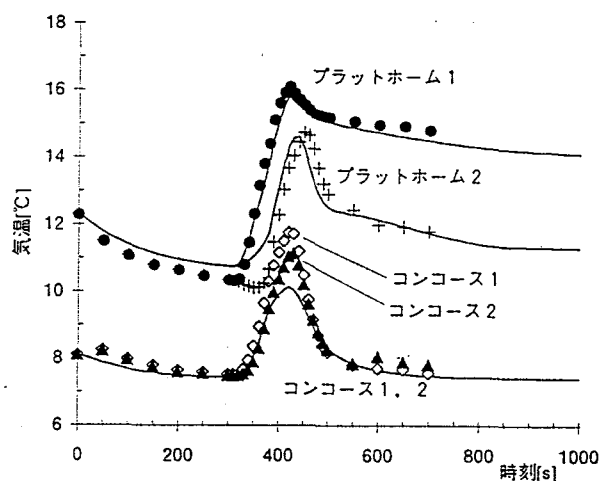
図-3.26 ミクロおよびマクロモデルによる簡易駅各部気温の変化
