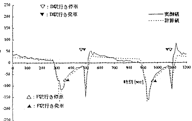
(d) F駅到着側トンネルの流量比較
