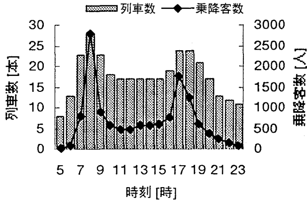
図-5.4 列車数と乗降客数
