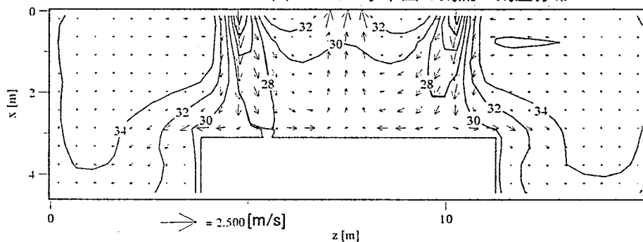
図-5.14 垂直断面の気流・気温分布
