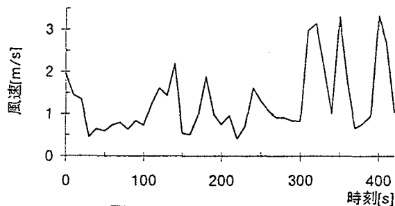
図-4.5 地上風速の変動
