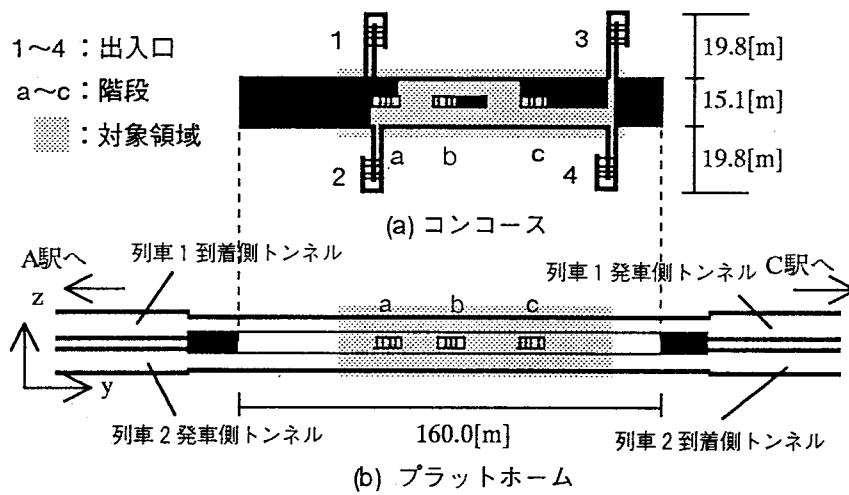
図ー5.1 地下鉄B駅平面図
