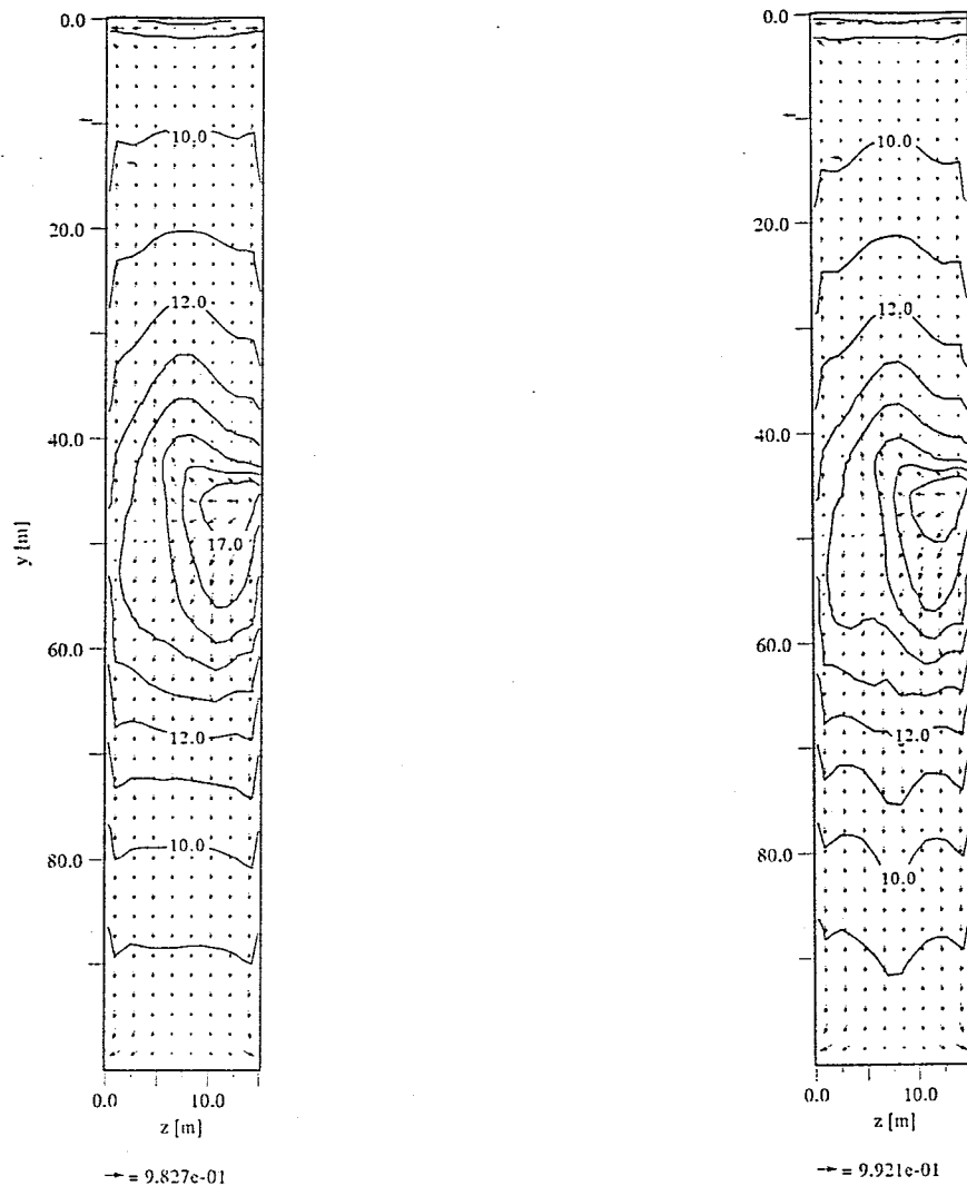
(c) one-way modelによる気流・気温分布 (x=1.5mの水平断面) (d) two-way modelによる気流・気温分布 (x=1.5mの水平断面)
