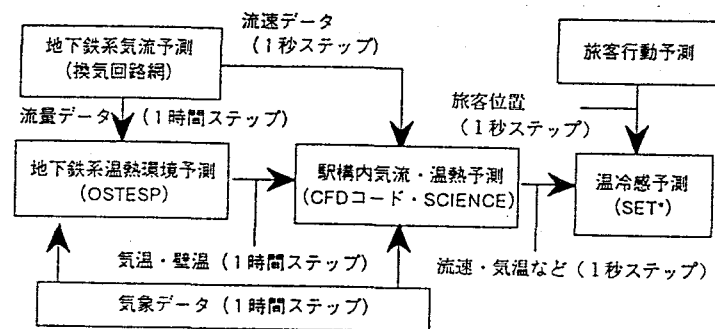
図-4.14 気流・温熱環境および温冷感予測の手順
