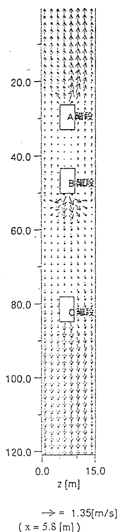
(a) 気流分布
