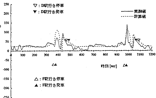
(b) F駅発車側トンネルの流量比較
