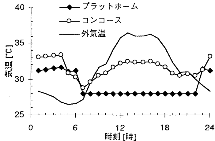
図-5.8 8月8日の気温変動
