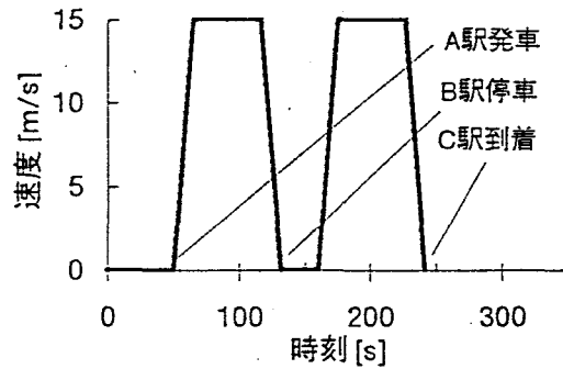
図-4.17 列車の走行曲線
