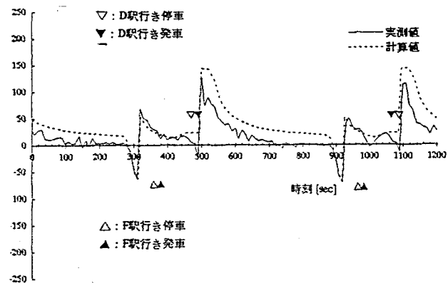
(a) D駅発車側トンネルの流量比較
