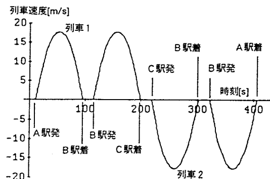
図-4.4 列車の走行曲線
