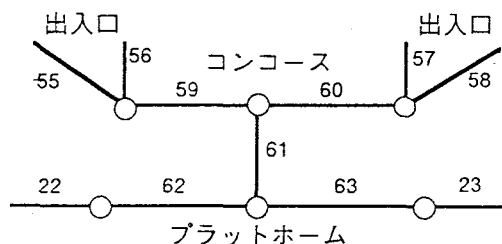
図ー3.18 換気回路網に置き換えた簡易駅
