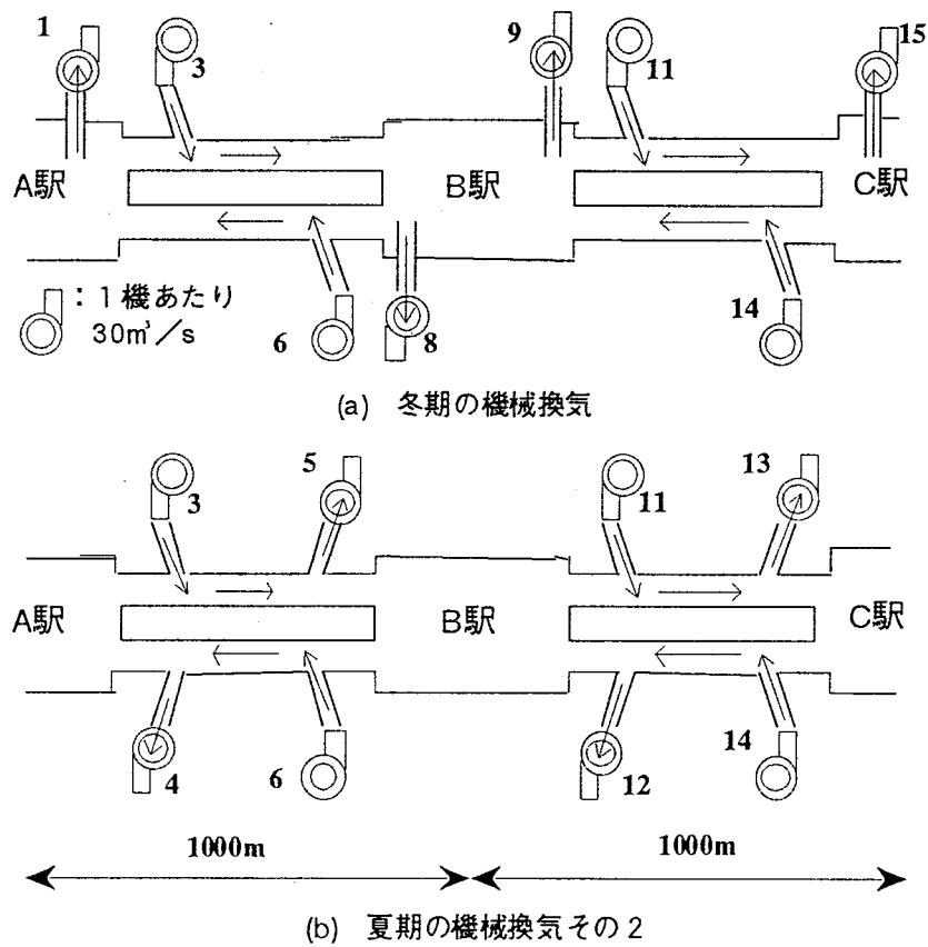
図ー5.2 地下鉄系の換気方式
