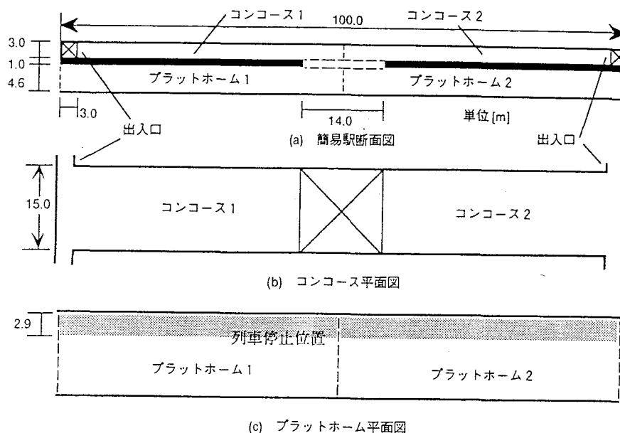
図ー3.17 簡易駅の構造
