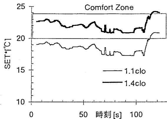
図-4.27 乗車客の温冷感
