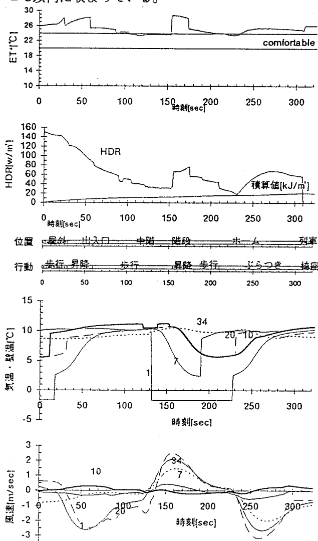
図-4.8 行動履歴1に対する温冷感および冬期の温熱環境
