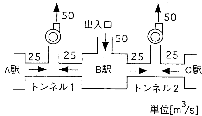
図一3.5 地下鉄系模式図
