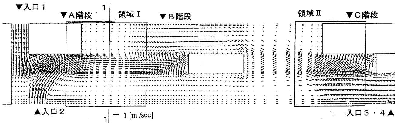
図-A.4 シミュレーションによるコンコースの気流分布
