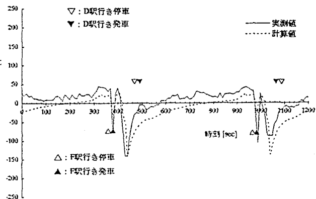
(c) D駅到着側トンネルの流量比較
