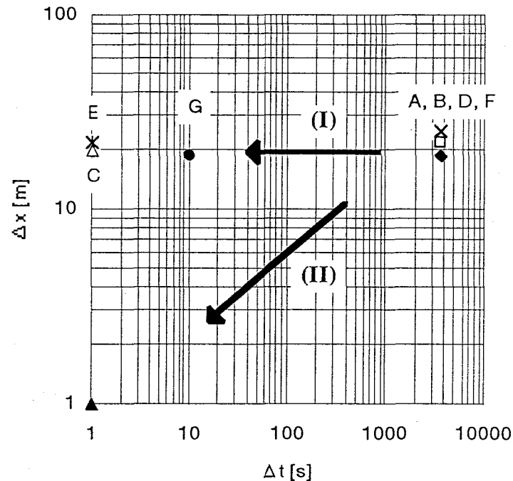
図-1.4 解析スケールの比較
