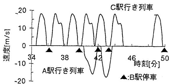
図-2.6 走行曲線
