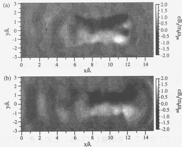
図 5.12 超高強度レーザーにより発生した定常磁場。(a)円偏向と(b)p 偏向のレーザーの場合について、 z 方向の磁場は同じ様なパターンになる。図は \omega_e t = 126 でプロットしたものであり、レーザー周期での平均をとり振動成分を落としてある。
