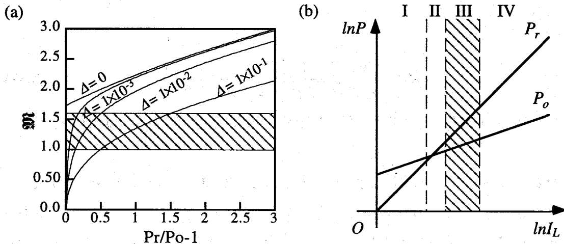
図 3.4 イオンの加速機構のレーザー強度依存性。(a)(3.32) 式を、粒子の反射率 \Delta を変えてプロットしたもの。マッハ数が1から1.6の範囲(図の斜線領域)に収まるためには、 P/P_0 に上限と下限がある。(b) P_r と P_o のレーザー強度依存性。Iの領域では、 P_r < P_o でありイオンの加速は起こらない。II、IVの領域で直接加速が起こり、IIIの領域では、マッハ数が 1 < M < 1.6 であり衝撃波加速になる。
