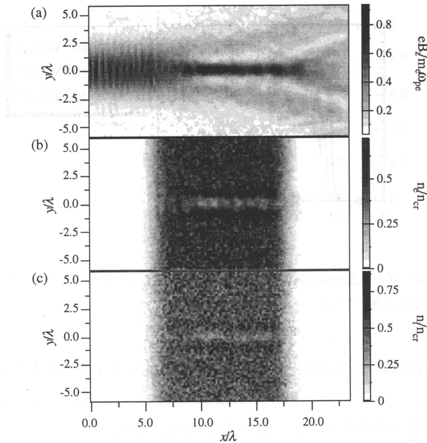
図 5.3 レーザー強度 1 \times 10^{18} \text{W/cm}^2 の時の図 5.2 と同様のプロット。
