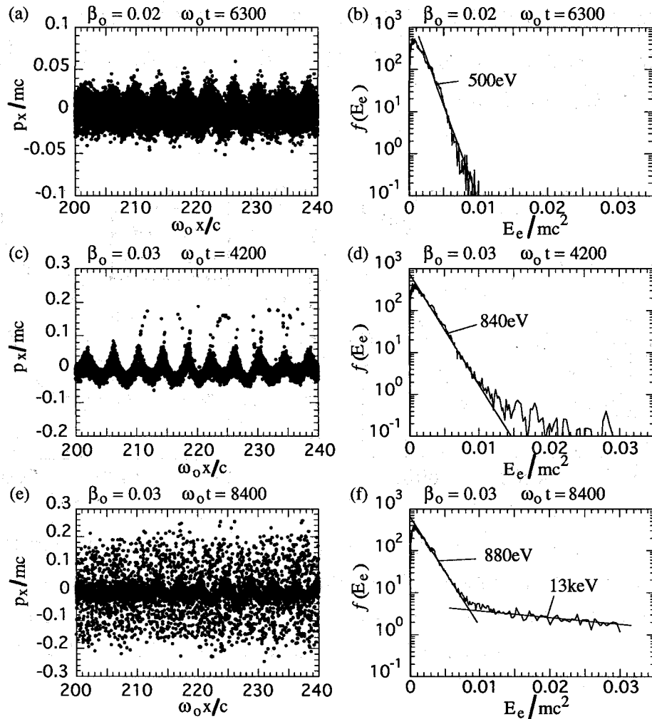
図 4.4 PIC シミュレーションによる位相空間プロット(a, c, e)とそのエネルギー分布関数(b, d, f)。レーザー強度が \beta_o = 0.02 と低いとき(a, b)は、位相のそろったプラズマ波が線形に成長し、プラズマの加熱は起こらない。強度が上がって \beta_o = 0.03 の時(c, d)には、プラズマ波のダイナミクスが非線形になり、電子が波に捕捉される。この捕捉電子は分布関数の裾野に見られるコブとして現われている。図(e) と(f)は \beta_o = 0.03 のプロットであるが、(c, d)よりも時間がたった後のプロットである。乱雑さが発展し、コヒーレントな部分とカオス的な部分両方が混在しているのが分かる。プラズマ波の崩壊により、分布関数に高温の裾野が現われ、全体的な加熱も起こっている。
