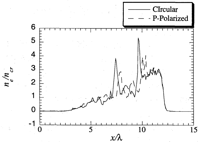
図 5.10 円偏向および p 偏向レーザー照射時の，レーザー軸上の電子密度分布。 \omega_0 t = 75.4 におけるプロット。
