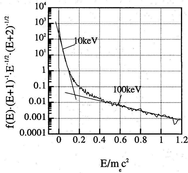
図 3.6 \omega_e t = 258 の時間での電子の分布関数。
