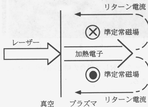
図 5.13 超高強度レーザーによる、準定常磁場の励起。レーザーにより加速された電子の電流で、定常磁場が作られる。また、リターン電流により、磁場はレーザーのスポット径の内側に閉じ込められる。
