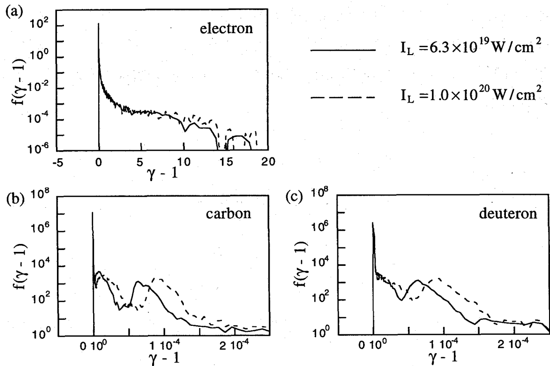
図 3.11 炭素(b), 重水素(c) の \omega_0 t = 283.5 (=0.16 \text{ psec}) におけるエネルギー分布関数。実線はレーザー強度 6.3 \times 10^{19} \text{ W/cm}^2 , 点線は 1 \times 10^{20} \text{ W/cm}^2 におけるプロット。
