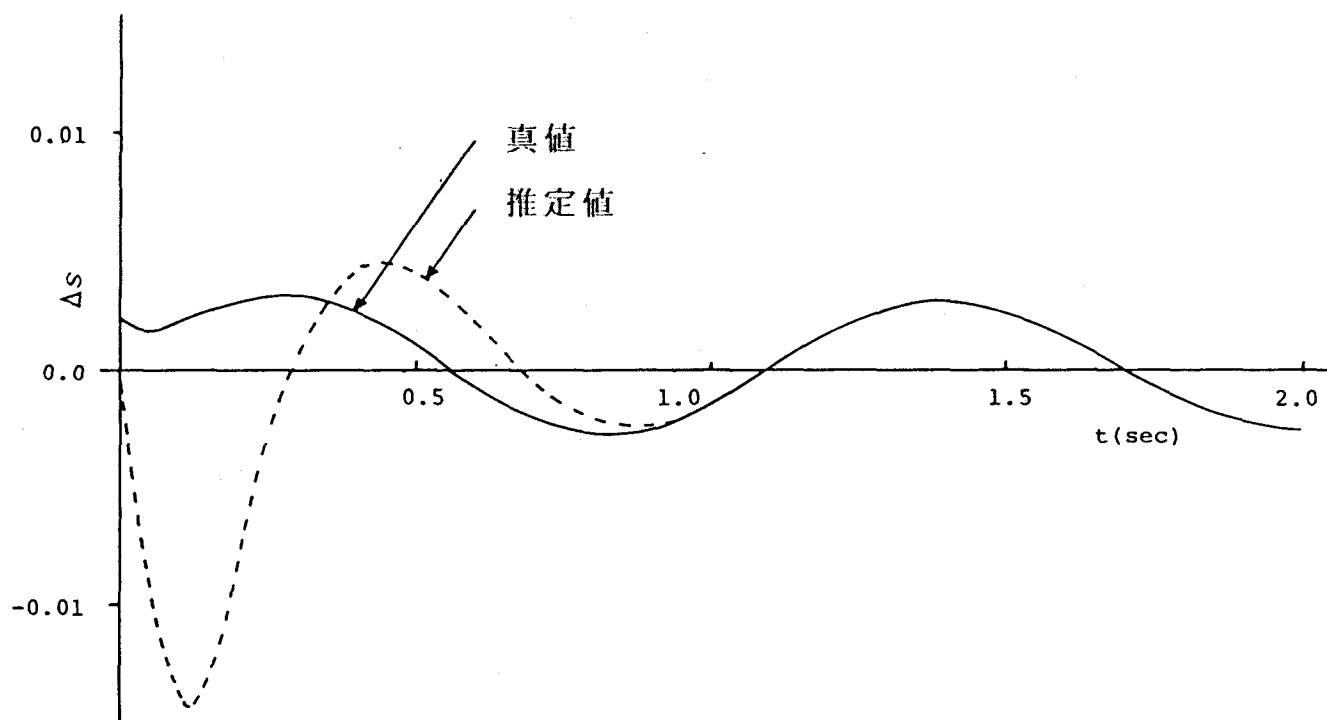
第 7. 5 図 \Delta s の時間応答
