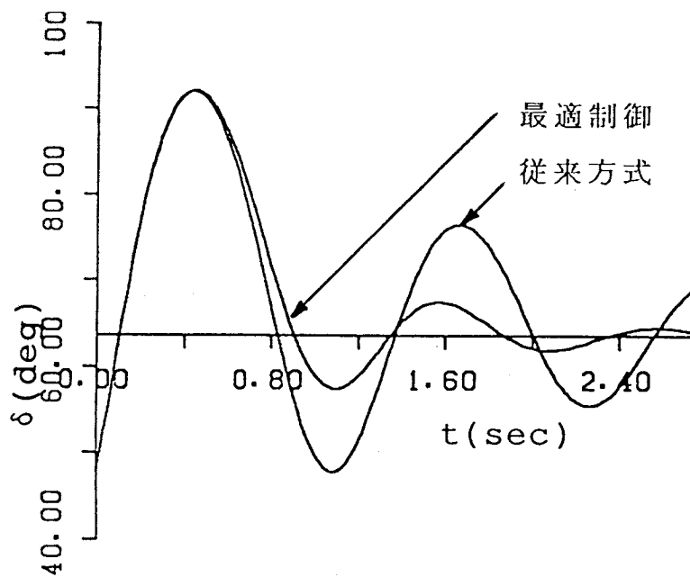
第 8 . 5 図 \delta の時間応答
