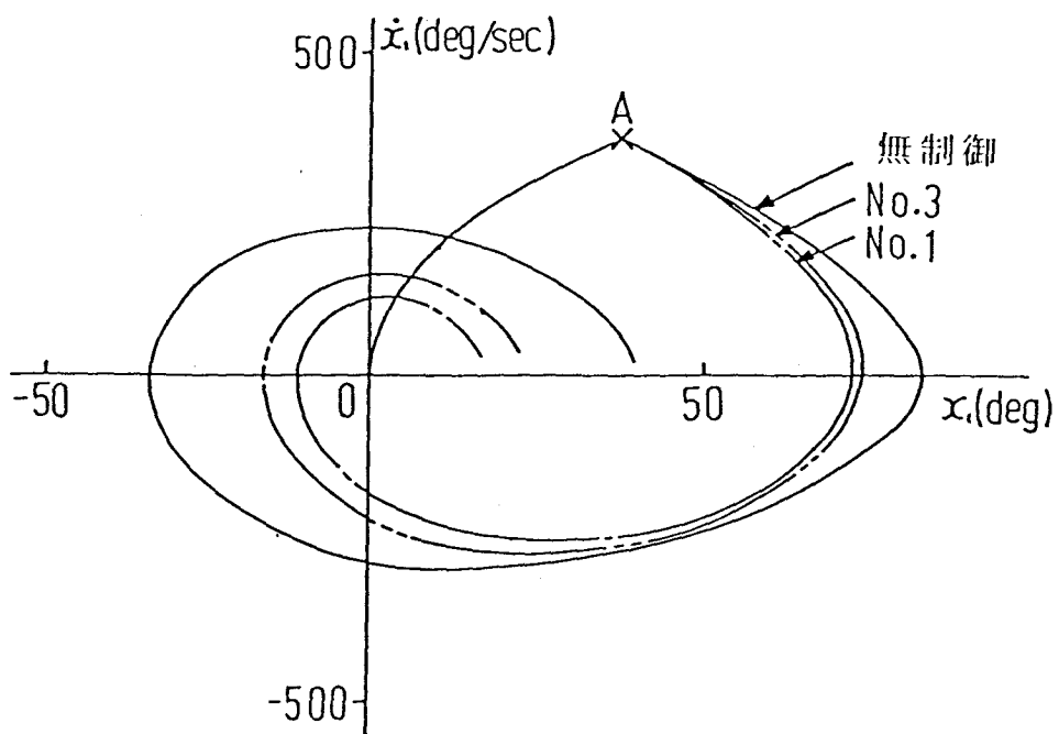
第 4 . 4 図 x_1 - \dot{x}_1 位相面軌道
