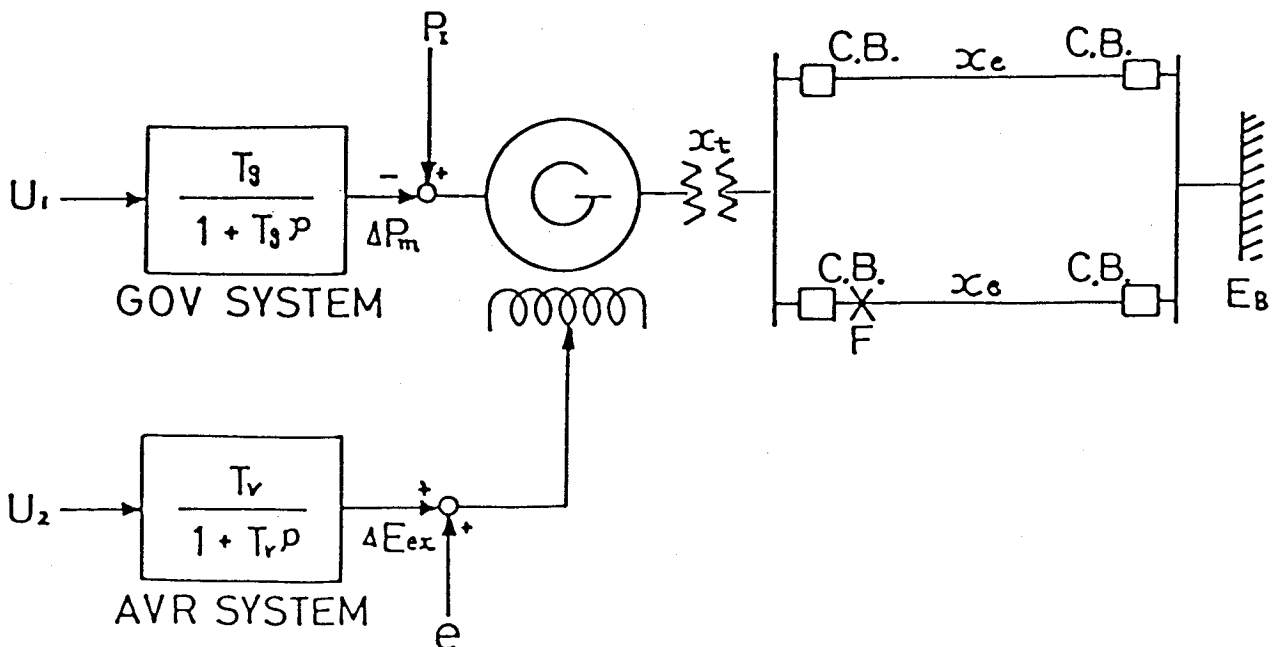
第 4. 1 図 調速機と A V R 制御系を含む一機一無限大母線系統
