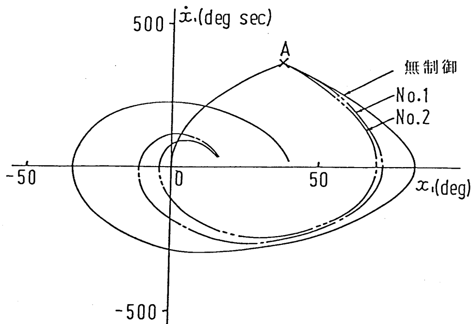
第 4 . 2 図 x_1 - \dot{x}_1 位相面軌道
