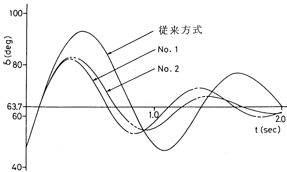
第 5 . 2 図 \delta の時間応答
