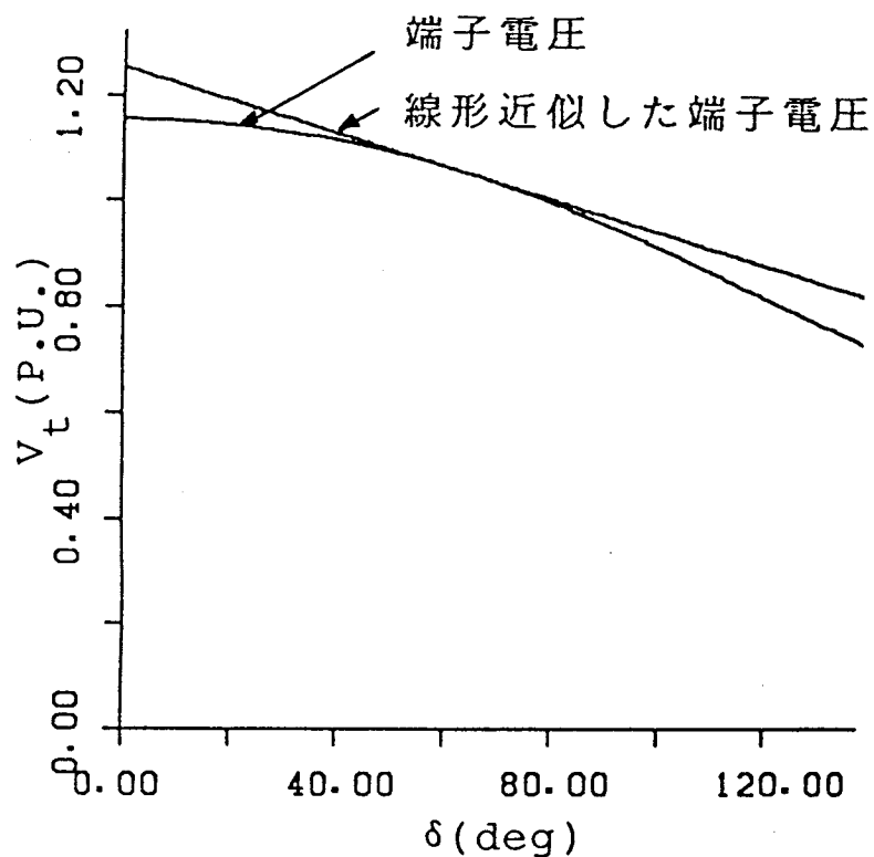
第 8. 1 図 位相角と端子電圧の関係
