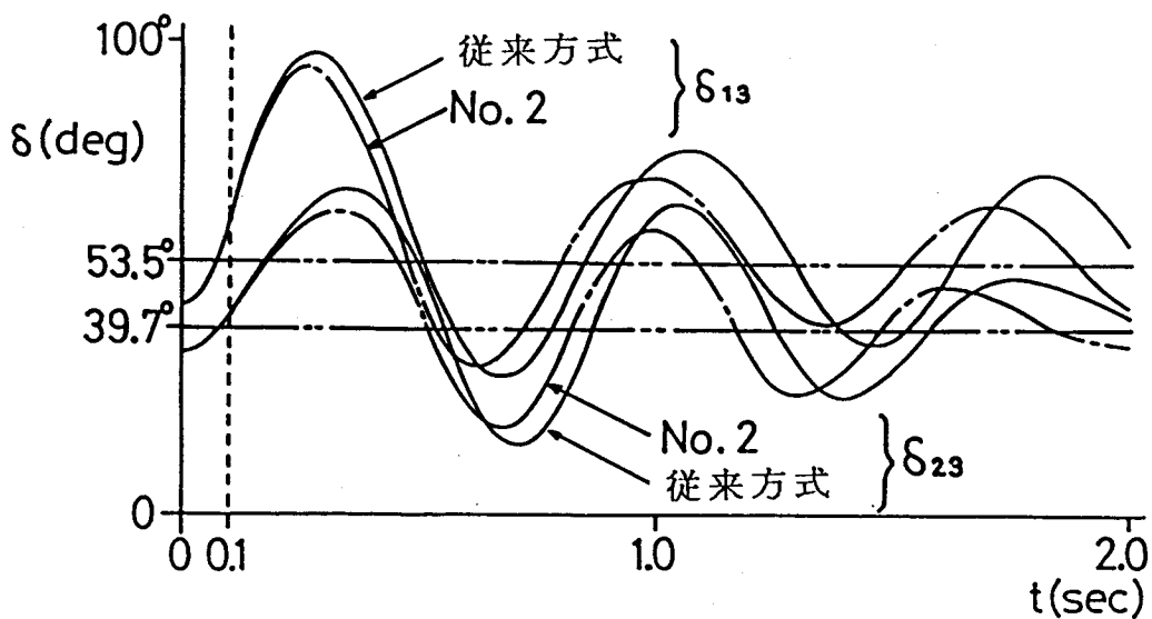
第 6 . 2 図 \delta_{13}, \delta_{23} の時間応答
