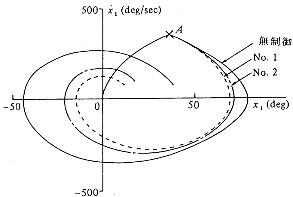
第 3 . 4 図 x_1 - \dot{x}_1 位相面軌道
