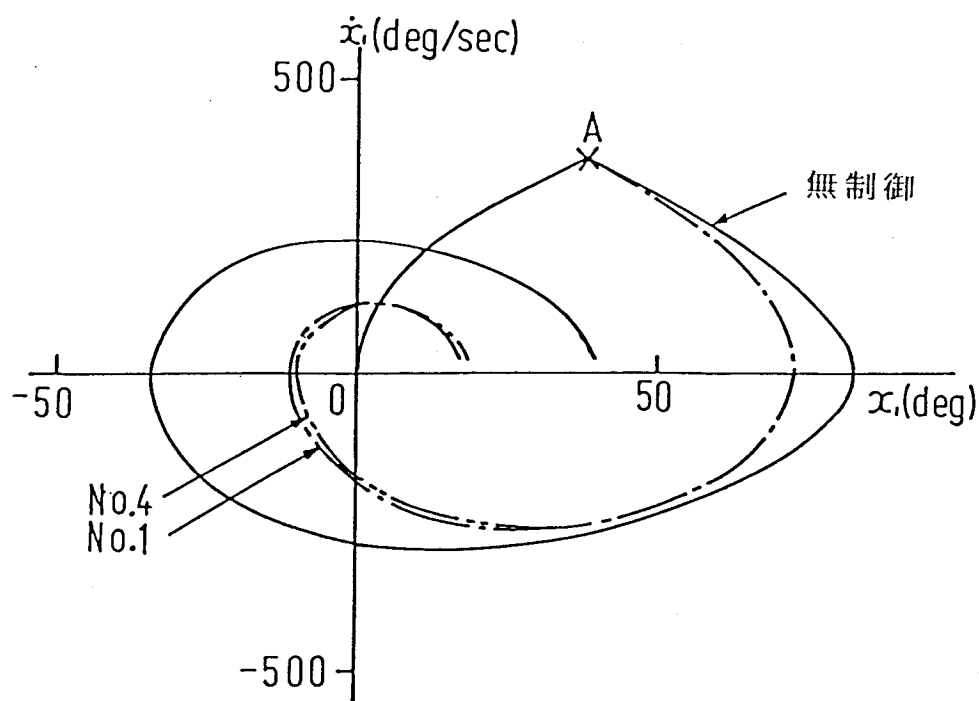
第 4 . 6 図 x_1 - \dot{x}_1 位相面軌道
