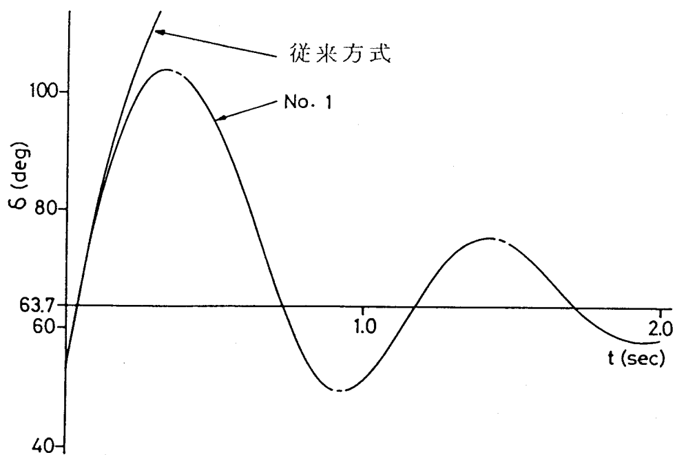
第 5 . 8 図 \delta の時間応答
