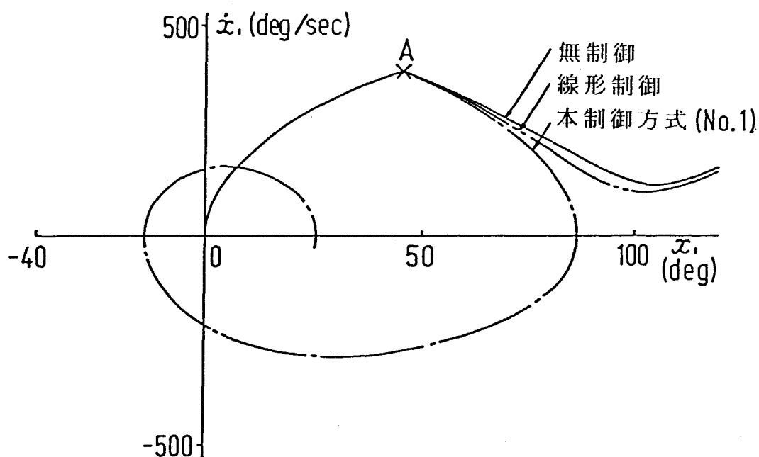
第 4 . 8 図 x_1 - \dot{x}_1 位相面軌道
