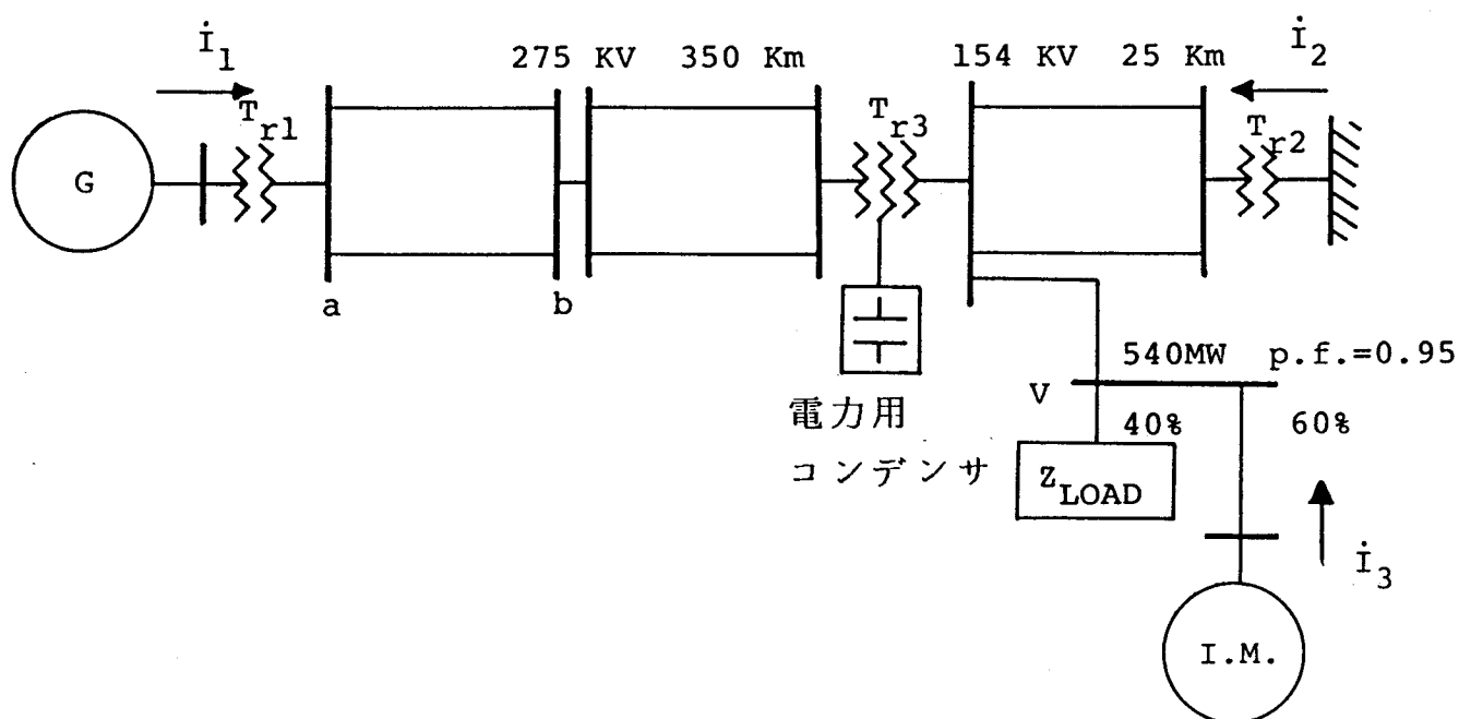
第 7. 1 図 系統負荷特性を考慮した一機—無限大母線系統
