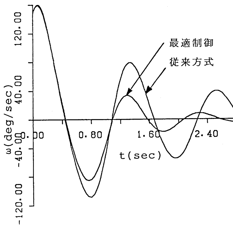
第 8 . 6 図 \omega の時間応答
