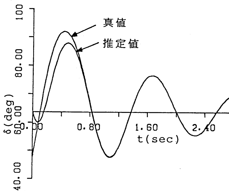
第 8. 2 図 \delta の時間応答
