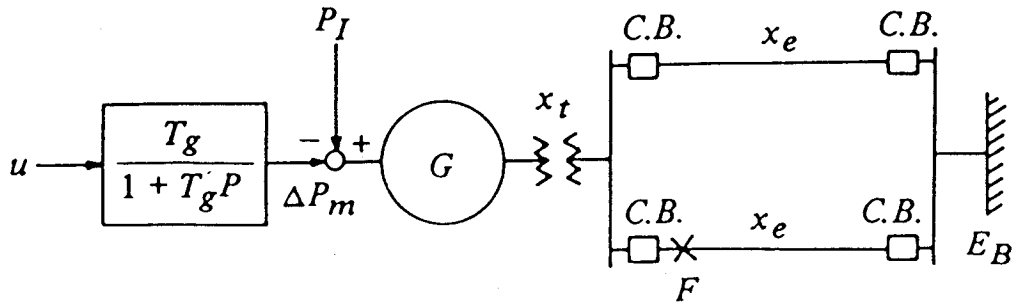
第 3. 1 図 調速機制御系を含む一機一無限大母線系統
