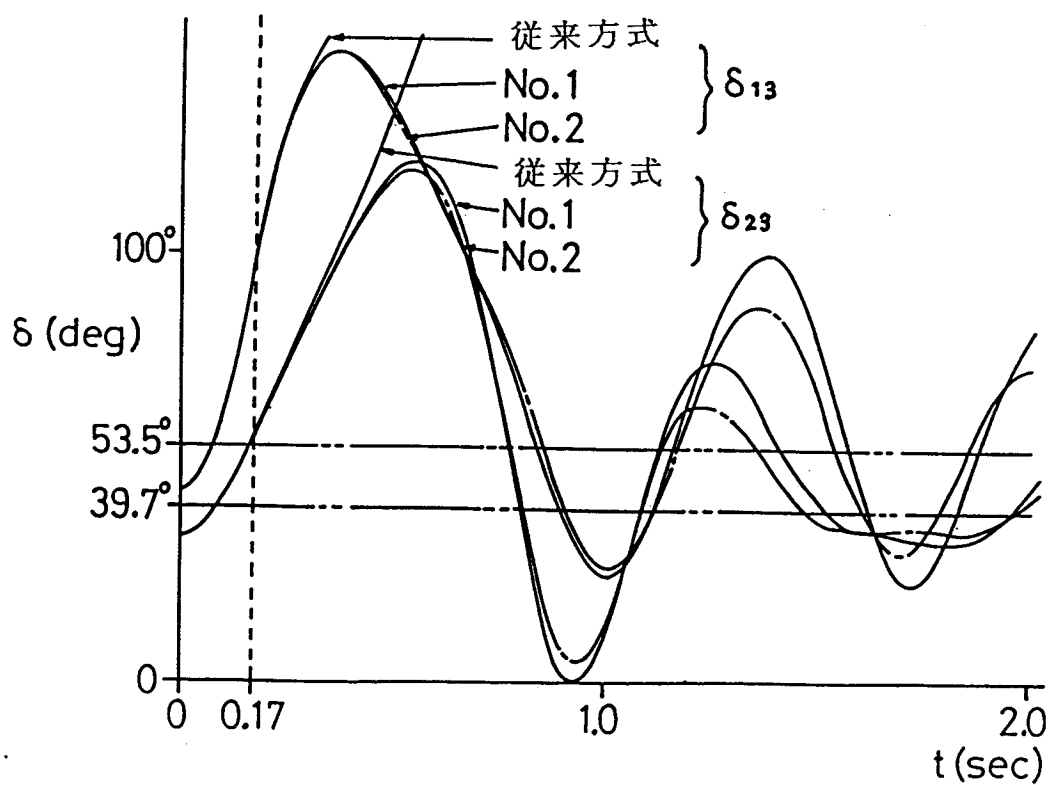
第 6 . 4 図 \delta_{13}, \delta_{23} の時間応答
