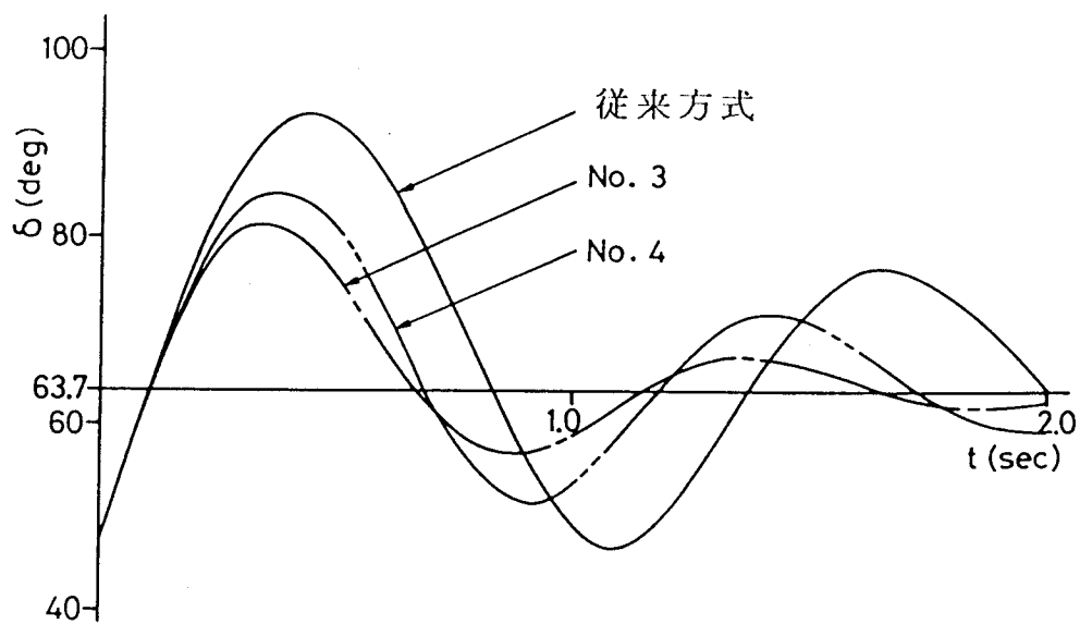
第 5 . 6 図 \delta の時間応答
