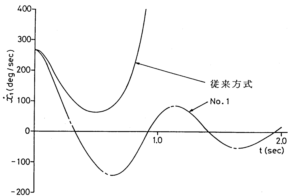
第 5 . 9 図 \dot{\delta}_1 の時間応答
