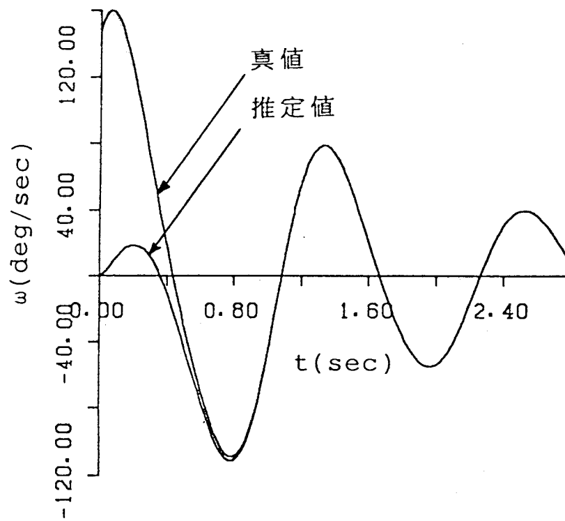
第 8 . 3 図 \omega の時間応答
