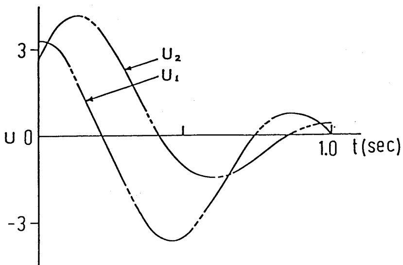
第 4 . 3 図 制御信号と時間関係
