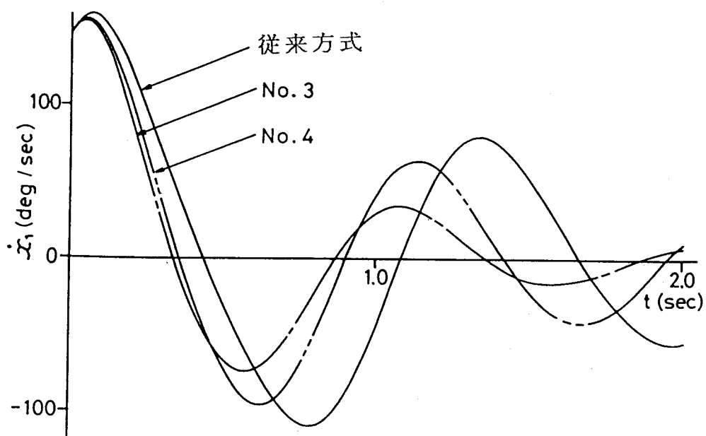
第 5 . 7 図 \dot{\delta} の時間応答
