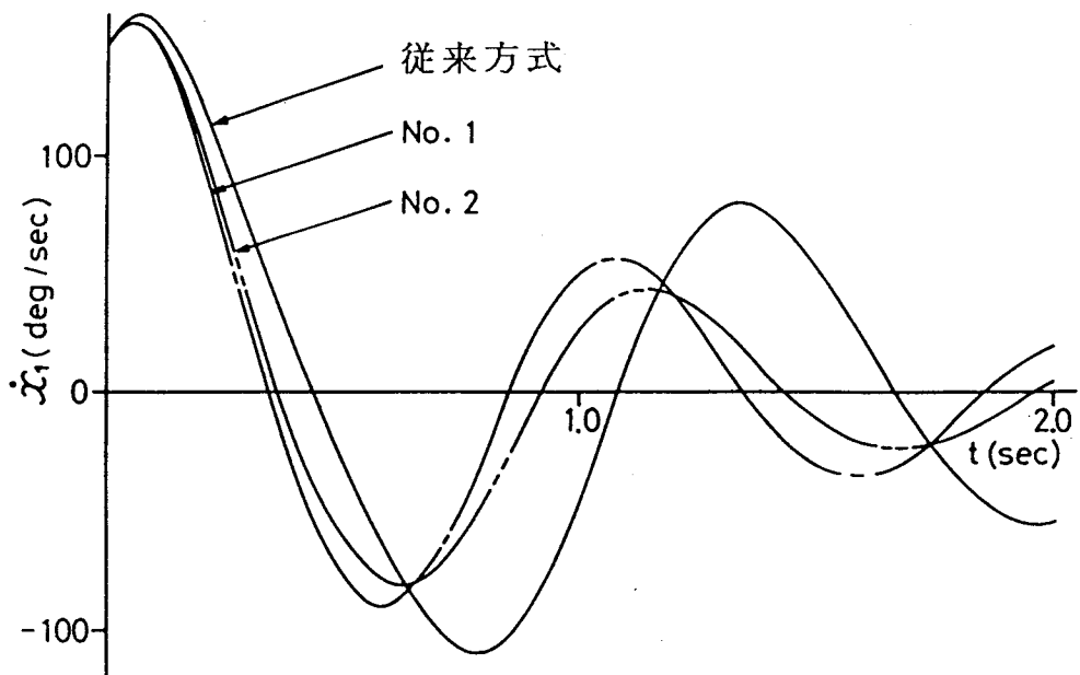
第 5 . 3 図 \dot{x}_1 の時間応答
