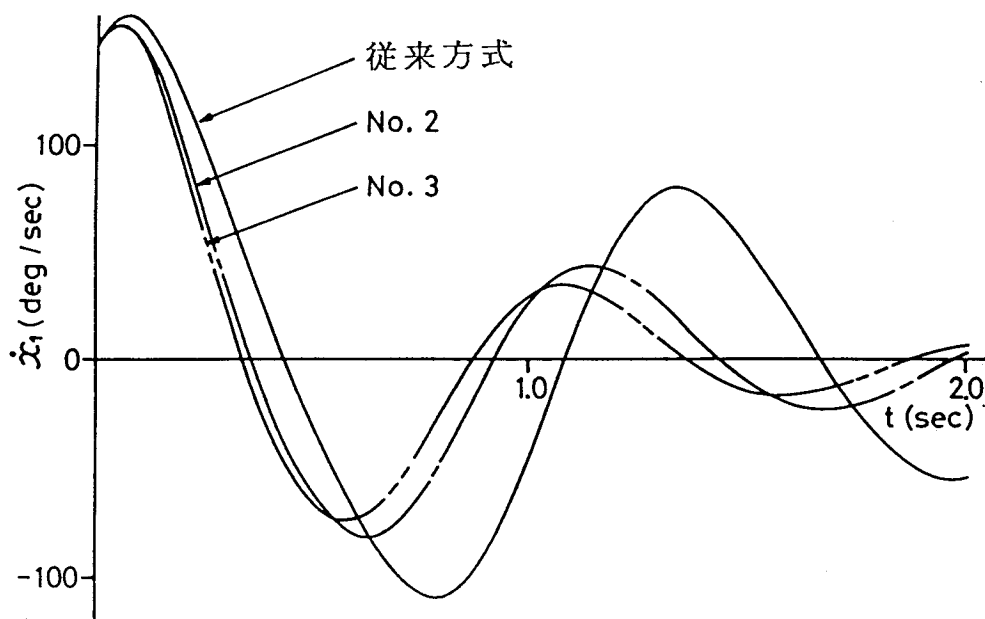
第 5 . 5 図 \dot{\delta}_1 の時間応答
