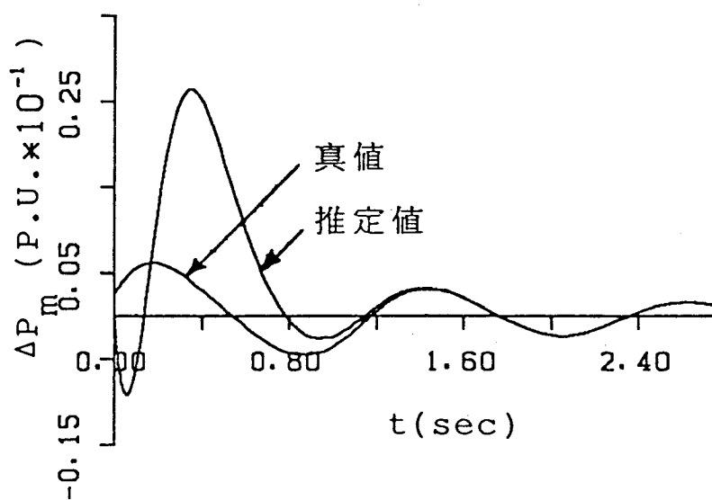
第 8 . 4 図 \Delta P_m の時間応答
