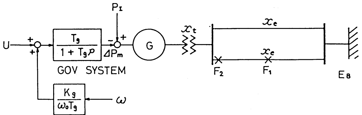
第5.1図 調速機制御系を含む一機—無限大母線系統
