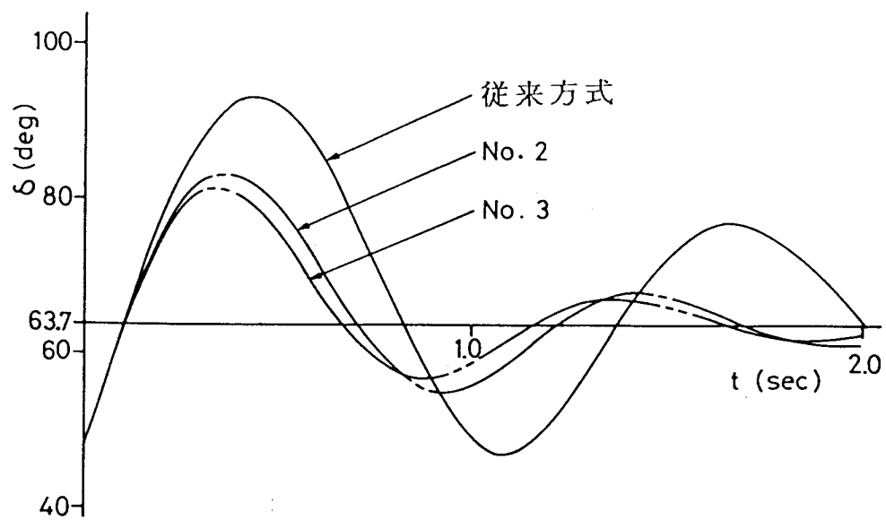
第 5 . 4 図 \delta の時間応答
