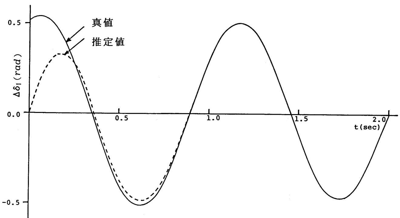
第7. 2 図 \Delta\delta_1 の時間応答
