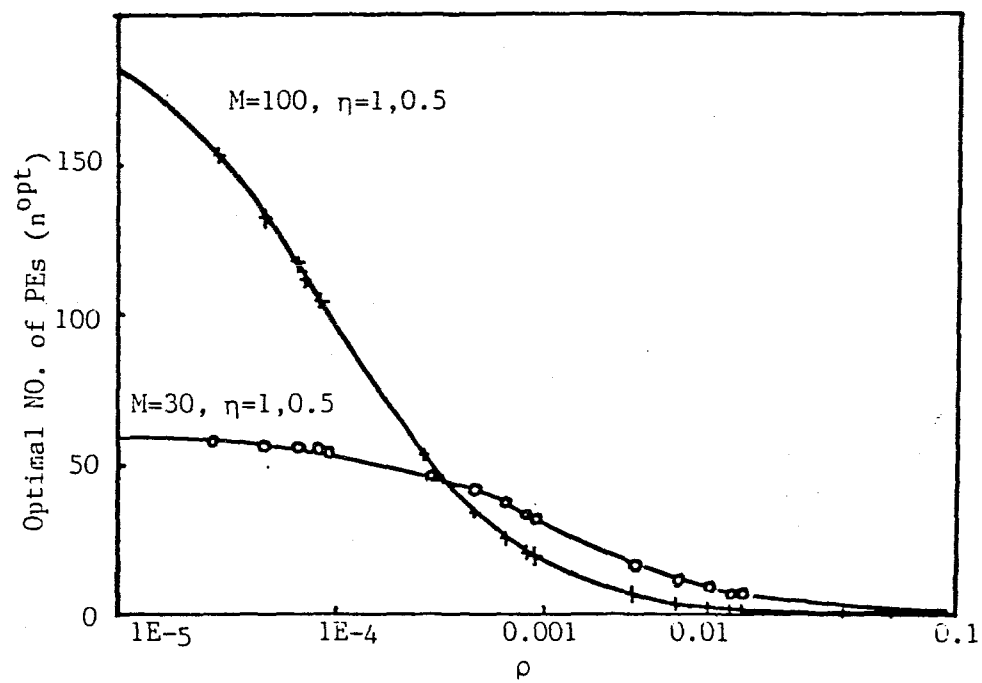
図3.5 最適PE数
