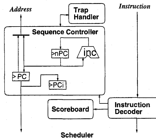
Fig. 2.9 命令解釈ユニットのブロック図
