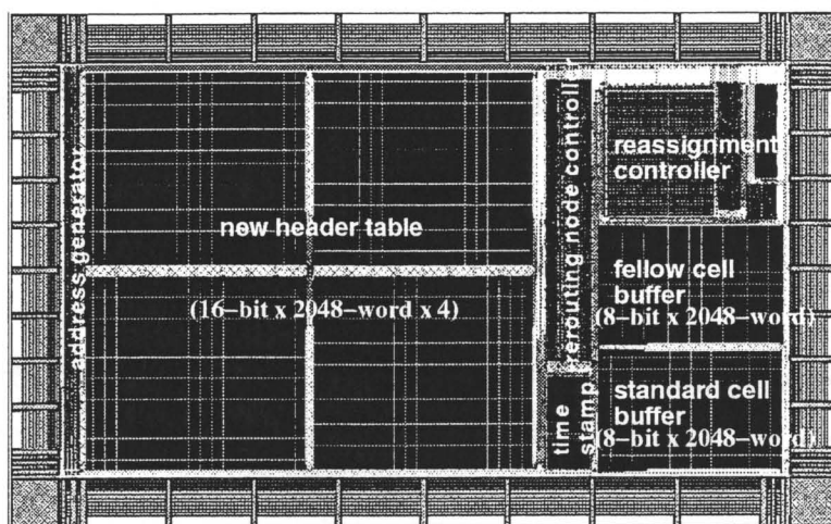
Fig. 5.4 リルートノードのレイアウト
