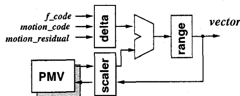
Fig. 3.19 ベクトル復号部の構成
