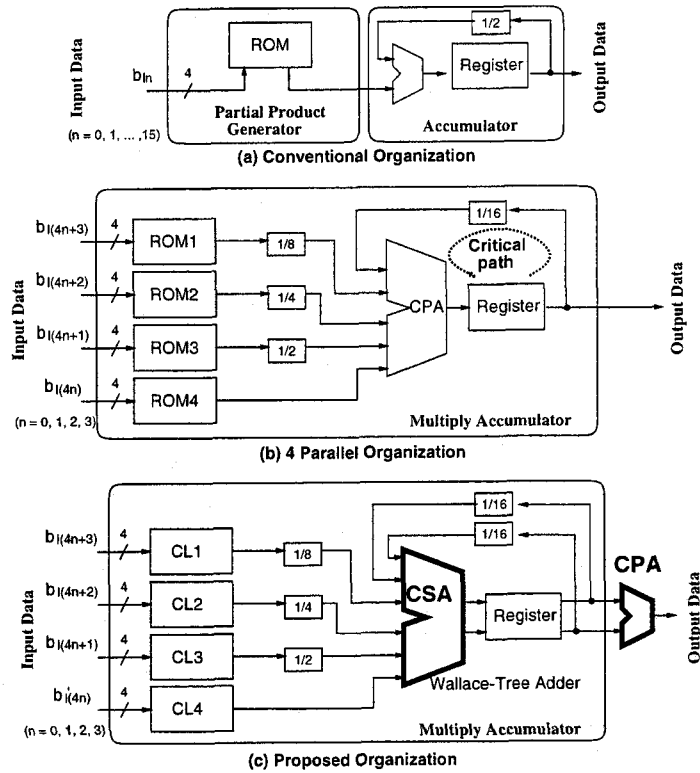
Fig. 3.15 積和演算器の構成
