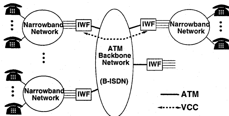
Fig. 4.5 バックボーンとしての ATM ネットワーク
