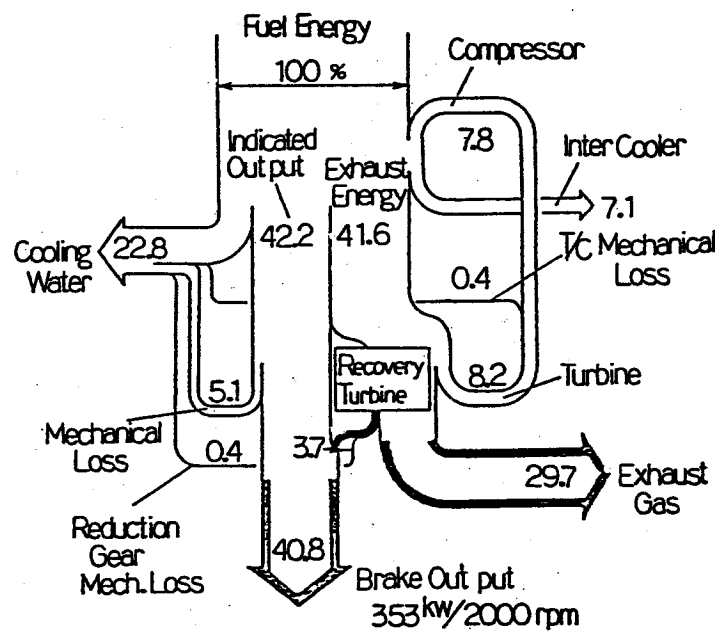
図 4.2.15 ターボコンパウンドのエネルギーフロー
