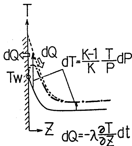
図 5.3.2 壁面近傍温度分布の非定常挙動
