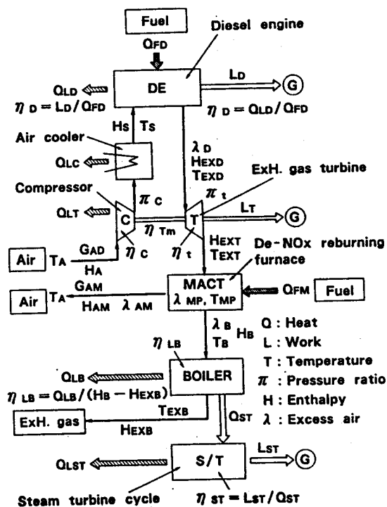
図 4.2.7 低 NOx 高効率ディーゼル複合発電システム
