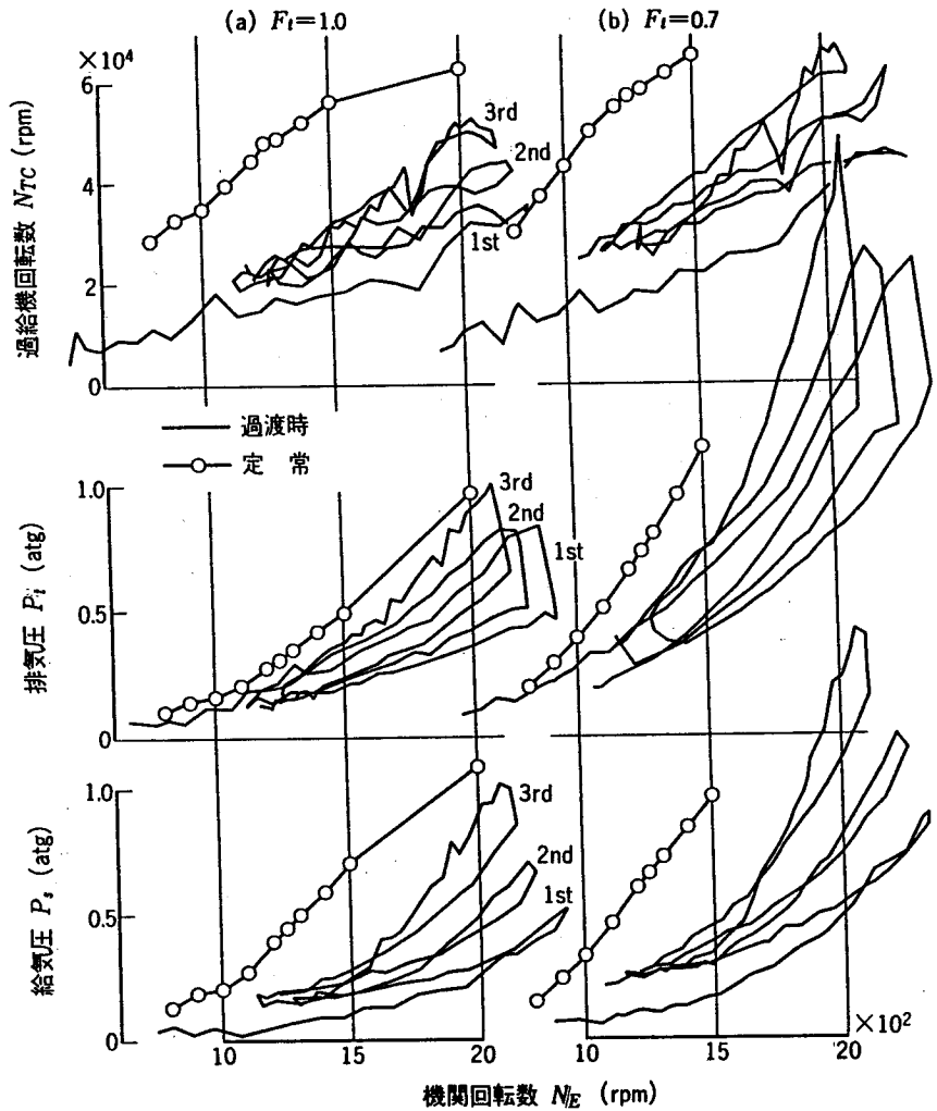
図 4.3.6 給排気系過渡特性
