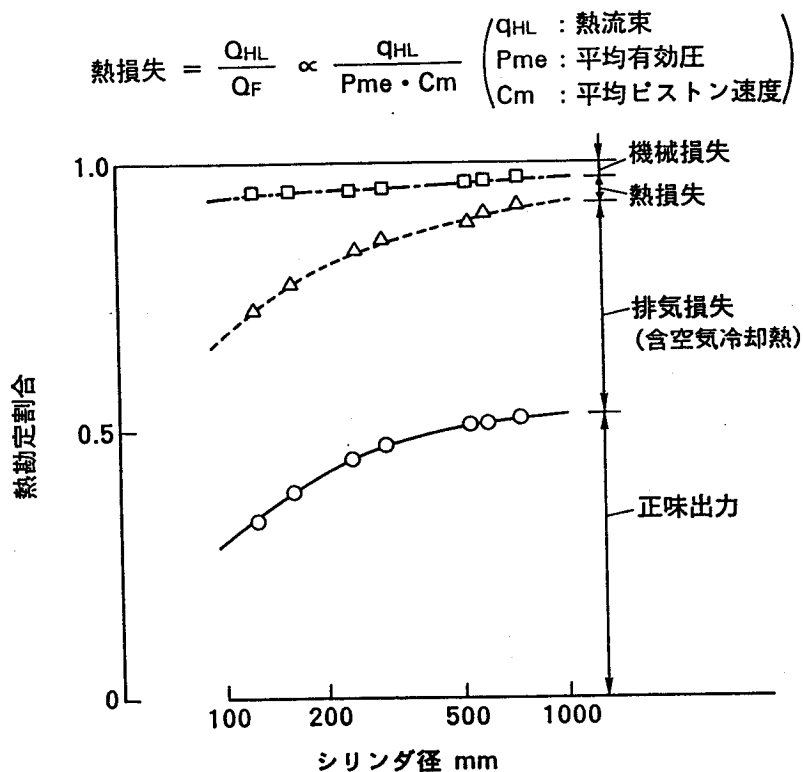
図 2.2.3 ディーゼルエンジンの熱勘定割合
