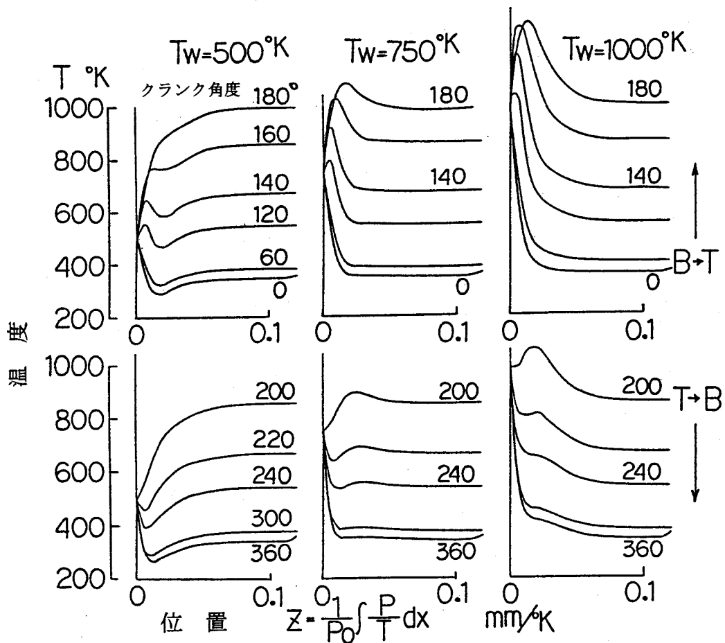
図 5. 3. 3 一次元非定常熱伝導モデル計算結果
