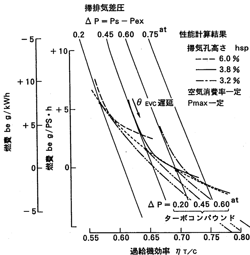
図 2.4.5 過給機効率と燃費率の関係
