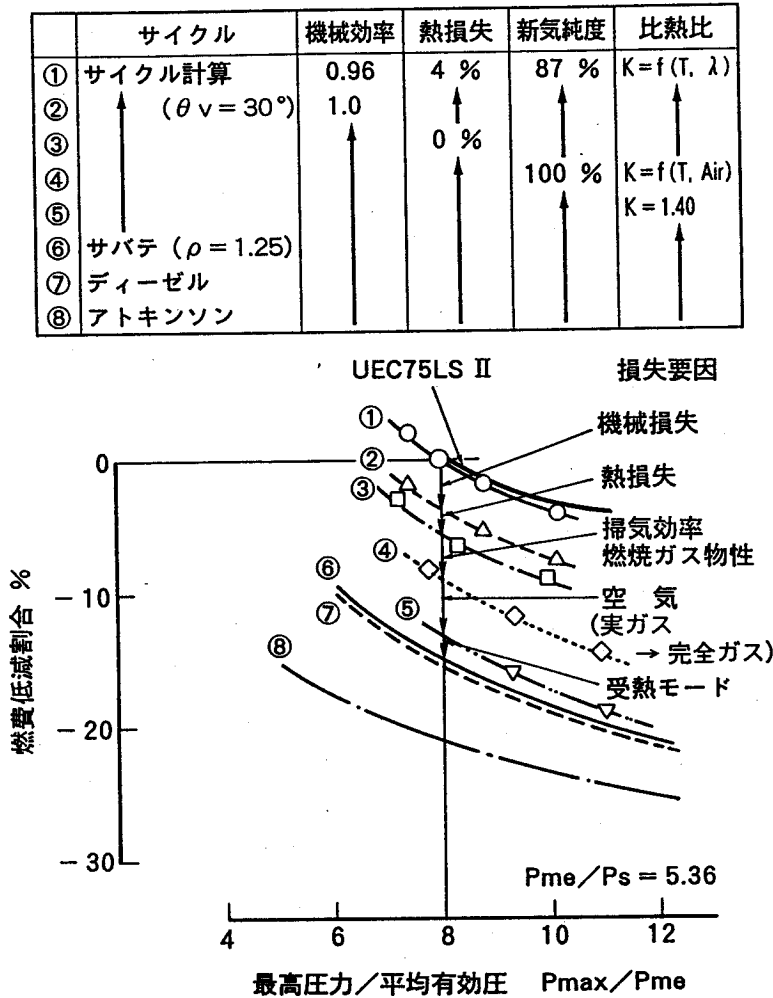
図 2.4.6 各種理想化サイクルの低燃費率化ゲイン
