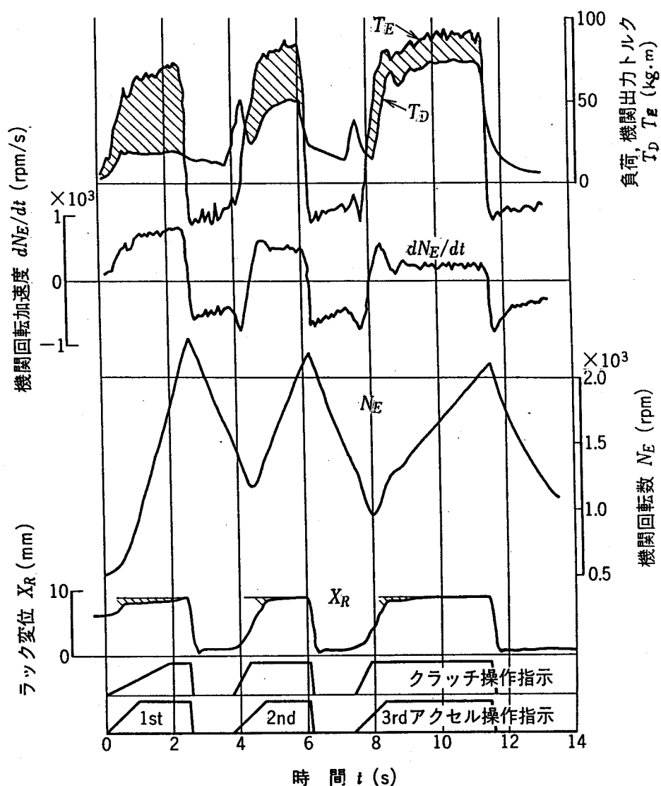
図 4.3.3 発進加速変速試験結果
