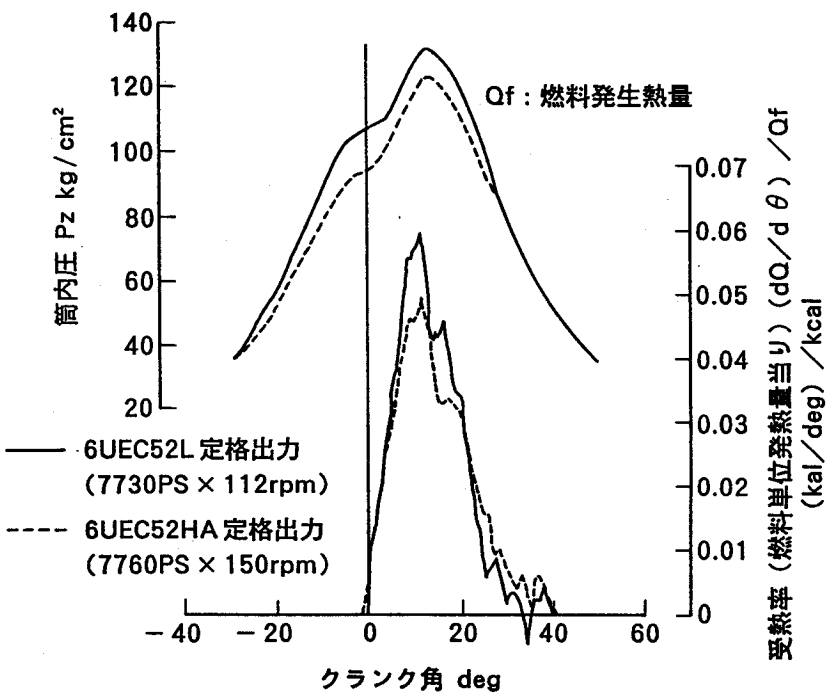
図 2.2.13 低速 2 サイクルディーゼルの受熱率
