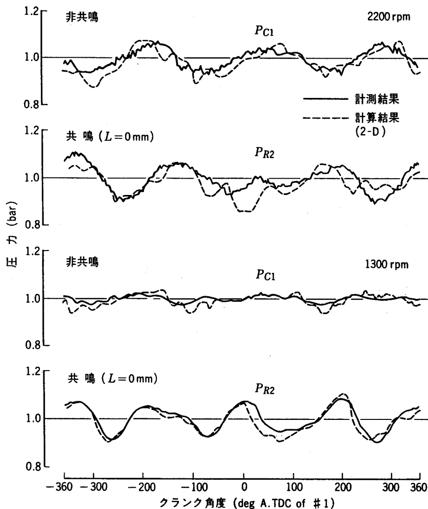
図 3.3.6 圧力変動の計測結果と計算結果の比較
