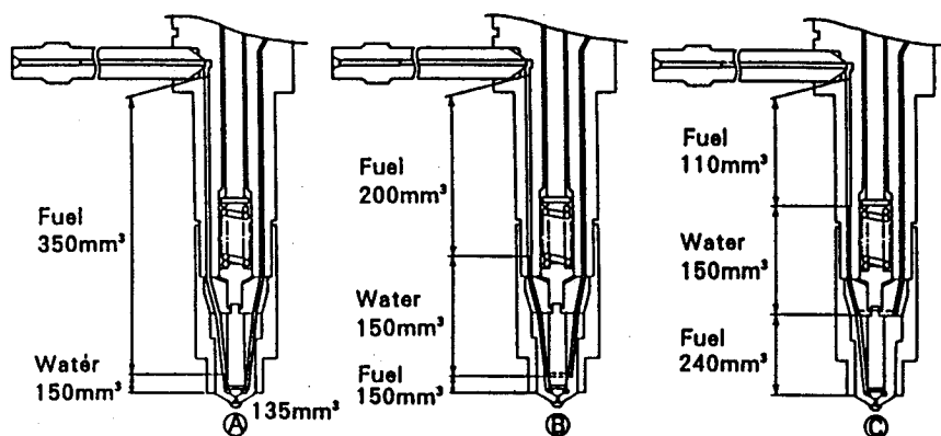
図 6.3.3 水注入位置の異なる燃料噴射弁構造の比較
