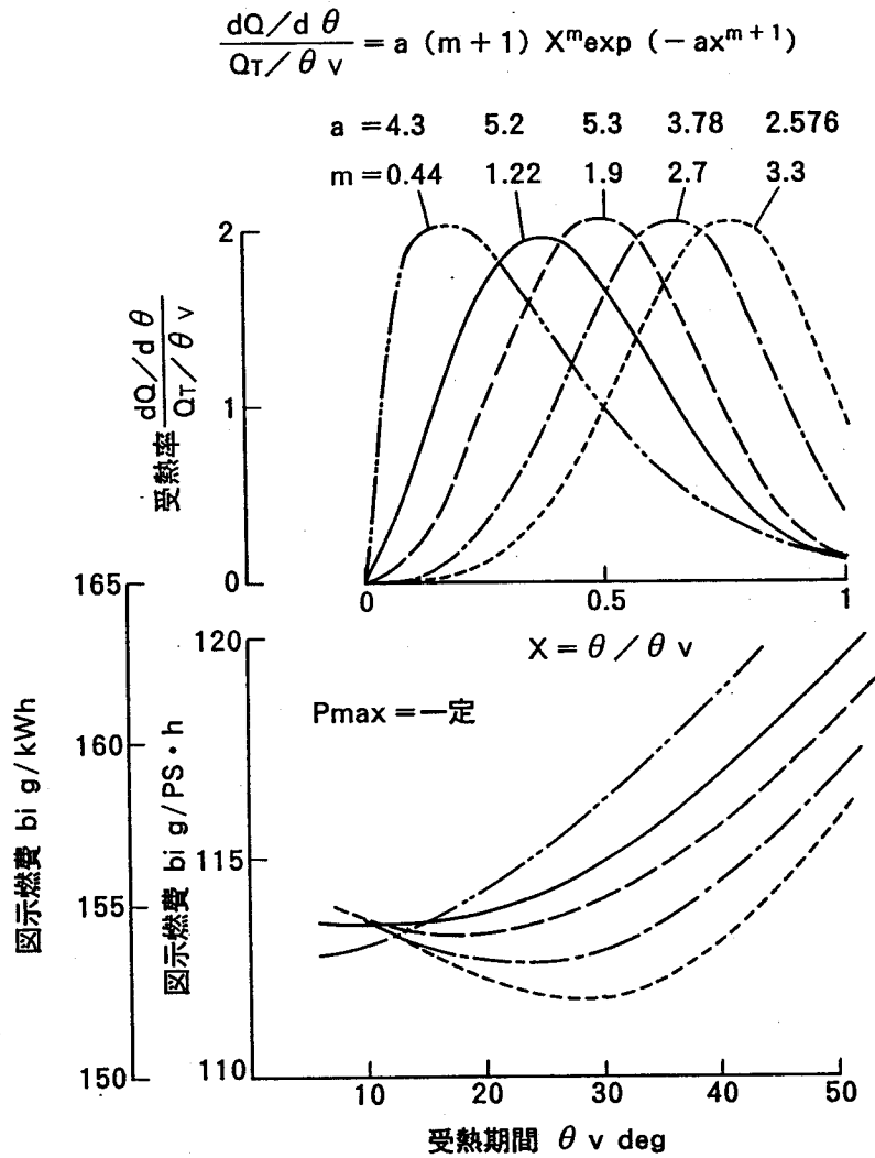
図 2.4.2 受熱モードおよび受熱期間による燃費率低減
