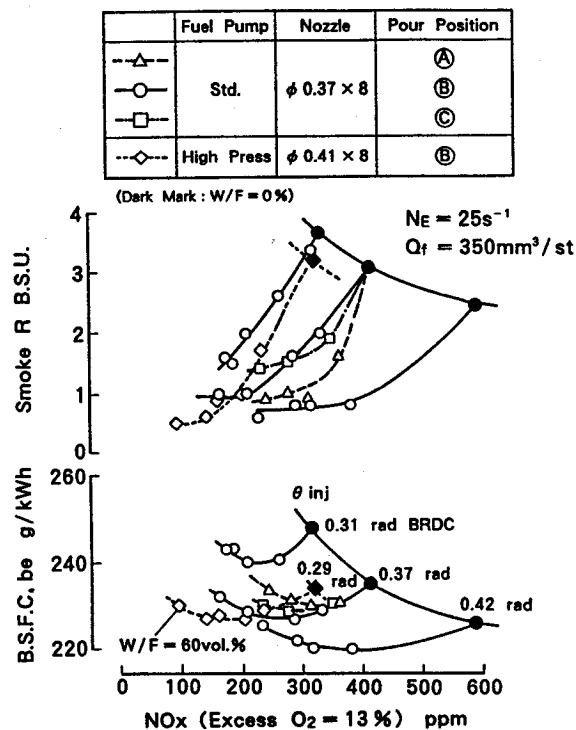
図 6.3.8 燃料・水層状噴射による NOx 低減
