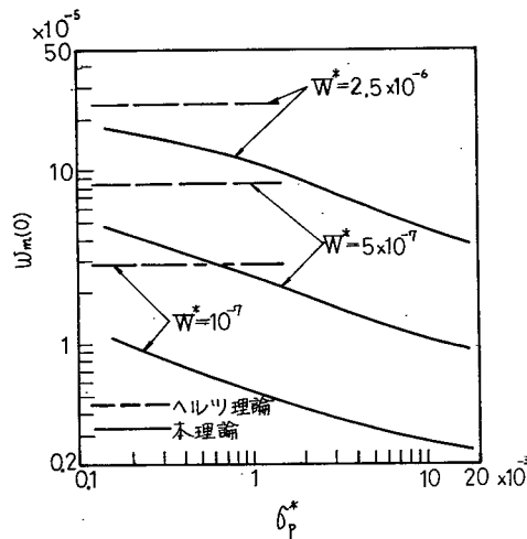
図 1.5.6 \sigma_p^* と母材の弾性変形量の関係 n_p^* = 300 \beta^* = 0.02
