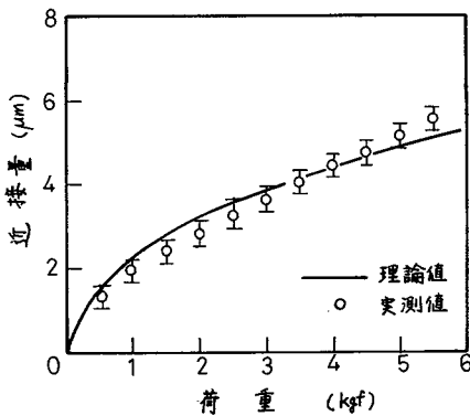
図 1.4.16 近接量に関する理論値と 実測値の比較
