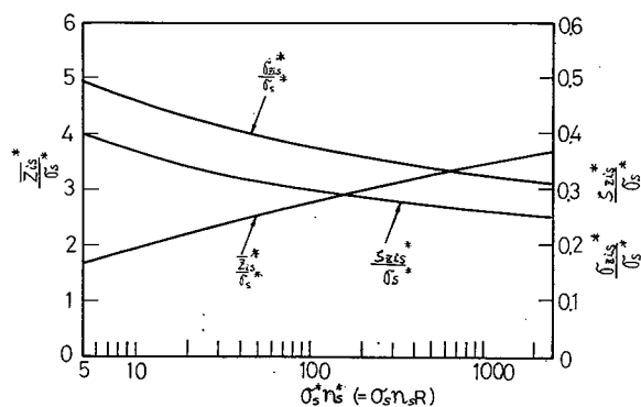
図 1.3.9 \sigma_s^* n_s^* と \bar{Z}_{is}^*/\sigma_s^* 、 \sigma_{zis}^*/\sigma_s^* 、 \zeta_{zis}^*/\sigma_s^* の関係
