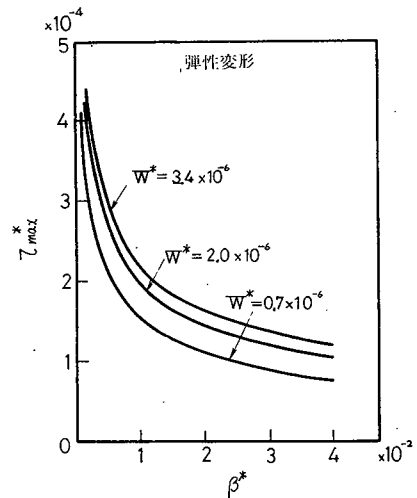
図 1.2.9 \beta^* と \tau_{\max}^* の関係 n_p^* = 120
