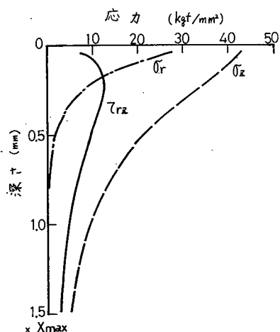
図 1.4.30 母材内部の応力分布
