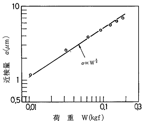
図 1.4.18 ナイロンボールの荷重と近接量の関係
