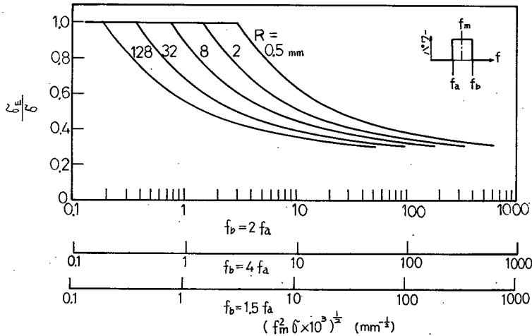
図 2.2.32 f_m と \frac{\sigma_E}{\sigma} の関係 (方向性なし)
