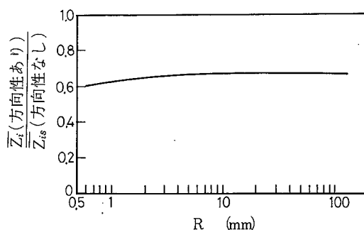
図 1.3.29 最初の接触位置の平均値に及ぼす方向性の影響
