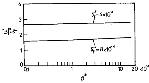
図 1.5.5 \beta^* と \frac{u^*}{\sigma_p^*} の関係 n_p^* = 250 W^* = 10^{-6}
