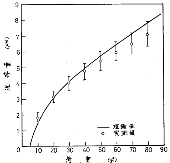
図 1.5.23 荷重と近接量の関係
