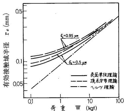
図 1.4.12 荷重と有効接触域半径の関係 \beta_s = 0.2 \text{ mm} R = 10 \text{ mm} E_1 = E_2 = 10000 \text{ kgf/mm}^2
