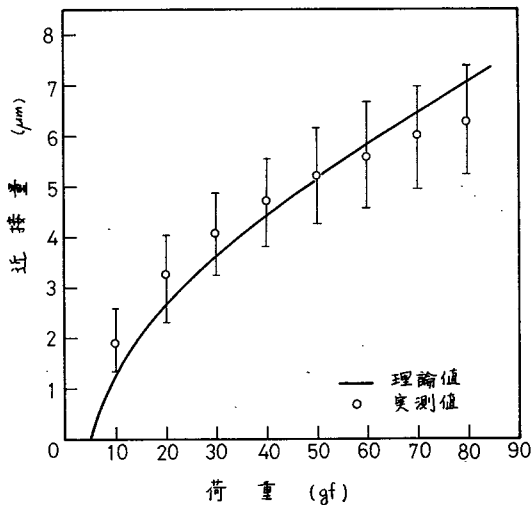
図 1.5.22 荷重と近接量の関係
