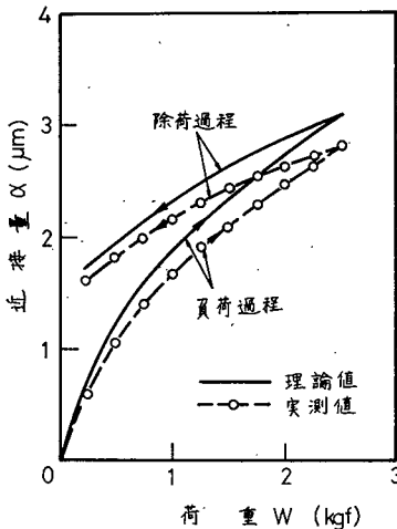
図 1.5.25 押付け実験による履歴曲線 \sigma_p = 0.9 \mu\text{m} R = 5 \text{ mm} \beta = 0.02 \text{ mm} p_m = 250 \text{ kgf/mm}^2 n_p = 34 \text{ mm}^{-1}
