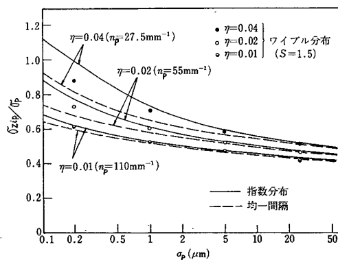
図 1.3.5 \sigma_{zip} に及ぼす突起間隔分布の影響 ( R_x = 5 \text{ mm} )
