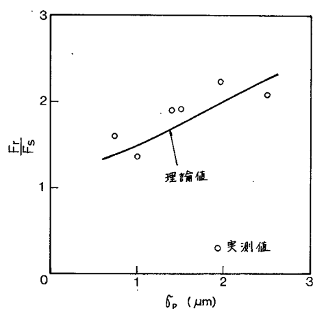
図 2.1.9 \frac{F_r}{F_s} に関する理論値と実測値の比較 W = 50 \text{ gf} R = 5 \text{ mm} E = 225 \text{ kgf/mm}^2
