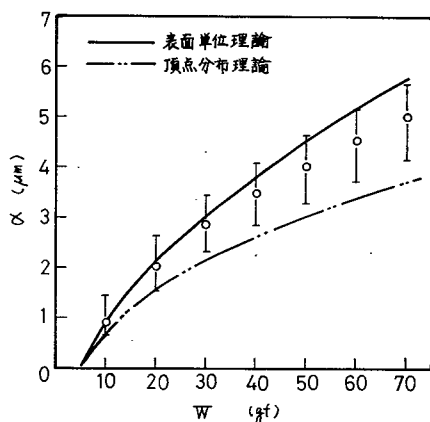
図 1.4.26 荷重と近接量の関係 R_a = 0.97 \mu\text{m} R = 5 \text{ mm}
