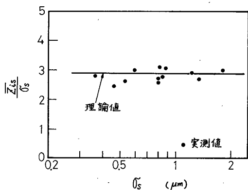
図 1.3.24 \bar{Z}_{is} の理論値と実測値の比較 R = 10 mm
