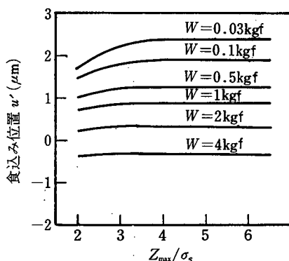
図 1.4.5 Z_{max} と食込み位置の関係 \sigma_s = 1 \mu m p_m = 500 kgf/mm^2 R = 5 mm
