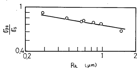
図 1.4.24 R_a と \frac{\sigma_{p3}}{\sigma_s} の関係
