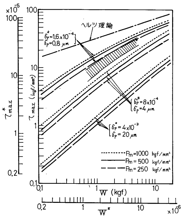
図 1.5.33 W と \tau_{max} の関係
