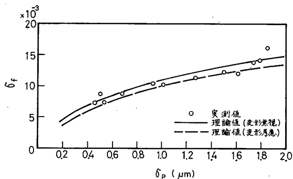
図 2.1.31 \sigma_f に関する理論値と実験値との比較
