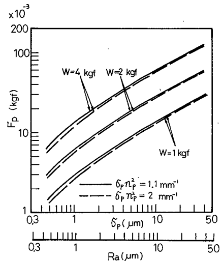
図 2.1.16 R_a と F_p の関係 (研摩布仕上面)
