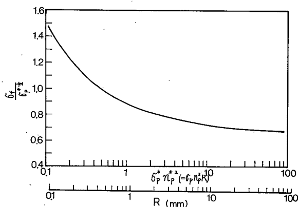
図 2.1.29 \sigma_p^* n_p^2 と \sigma_f / \sigma_p^{1/2} の関係
