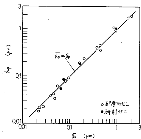
図 1.3.28 突起頂点高さの標準偏差と平均値
