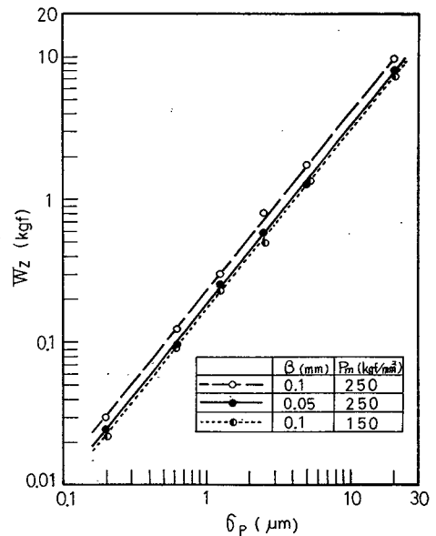
図 1.5.38 \sigma_p と W_z の関係
