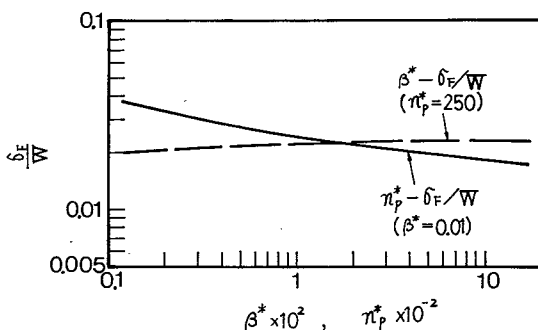
図 2.1.36 \beta^* , n_p^* と \sigma_F/W の関係
