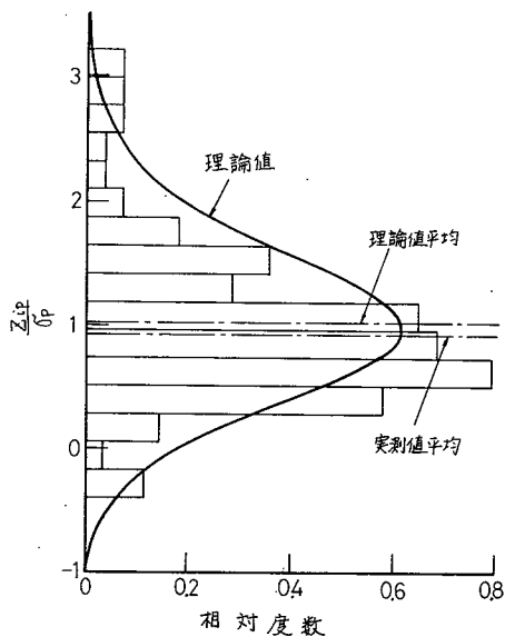
図 1.3.17 最初の接触位置の分布形
