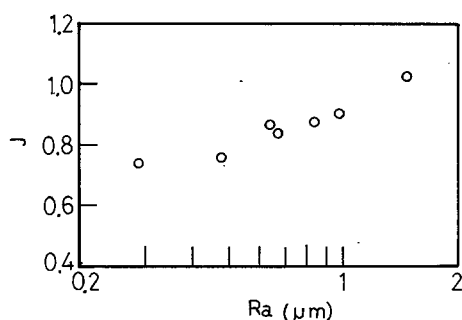
図 1.4.23 R_a と J の関係
