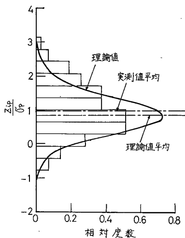
図 1.3.16 最初の接触位置の分布形
