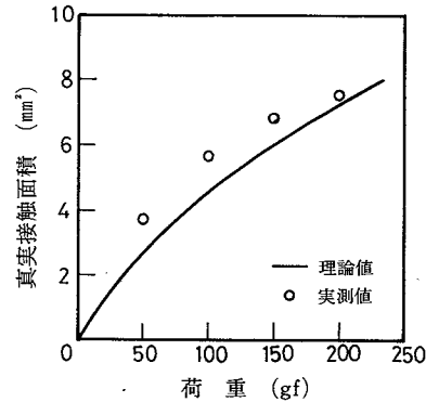
図 1.2.15 荷重と真実接触面積の関係
