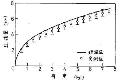
図 1.4.15 近接量に関する理論値と 実測値の比較
