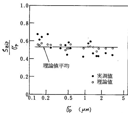
図 1.3.18 \zeta_{zip} の理論値と実測値の比較 R_x = 5 \text{ mm}
