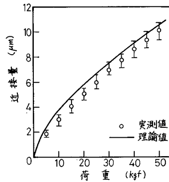
図 1.2.19 荷重と近接量の関係
