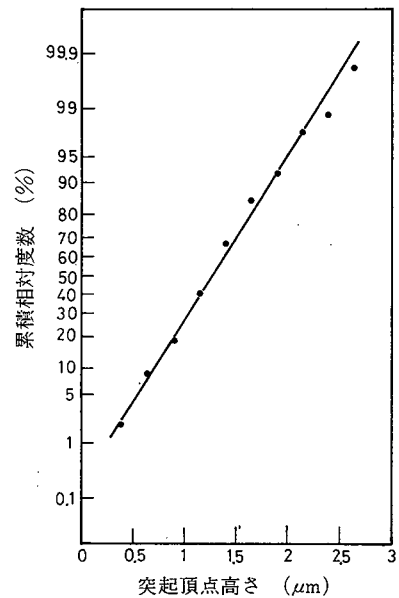
図 1.3.2 正規確率紙による分布形の推定 (研磨布仕上面)
