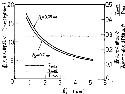
図1.4.33 \alpha_s と \tau_{max} , \frac{\tau_{max}}{p_{max}} の関係 W = 1 \text{ kgf}
