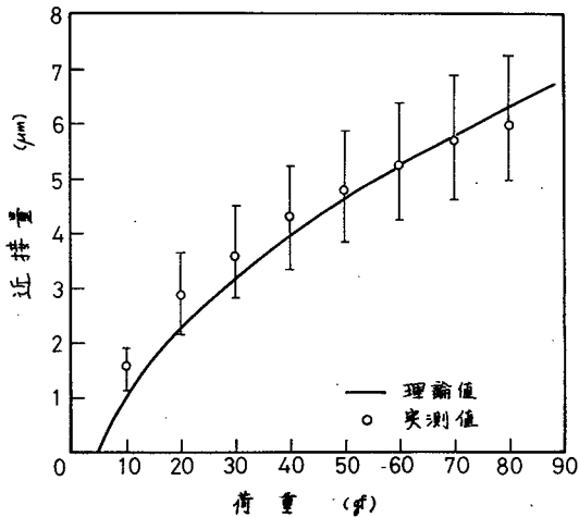
図 1.5.20 荷重と近接量の関係
