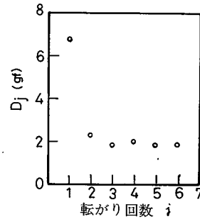
図 2.1.17 転がり回数と転がり抵抗差の関係
