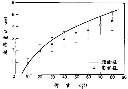
図 1.5.24 荷重と近接量の関係 R_a = 0.55 \mu\text{m} R = 5 \text{ mm}
