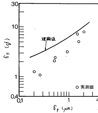
図 2.1.43 \sigma_F に関する理論値と実測値の比較
