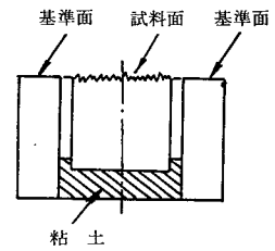
図 1.3.12 最初の接触位置測定用保持具
