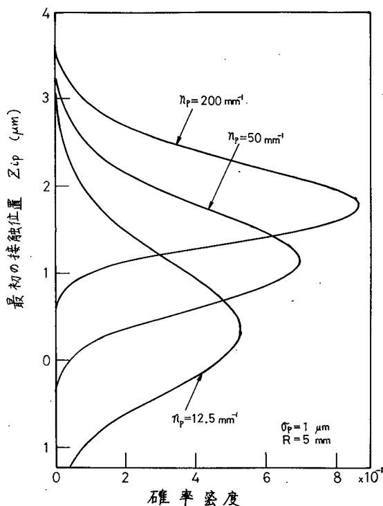
図 1.3.8 最初の接触位置の分布形
