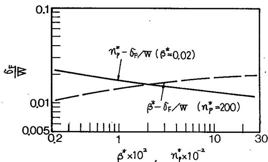
図 2.1.39 \beta^* , n_p^* と \sigma_F/W の関係
