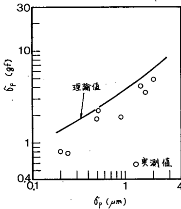
図 2.1.42 \sigma_F に関する理論値と実測値の比較
