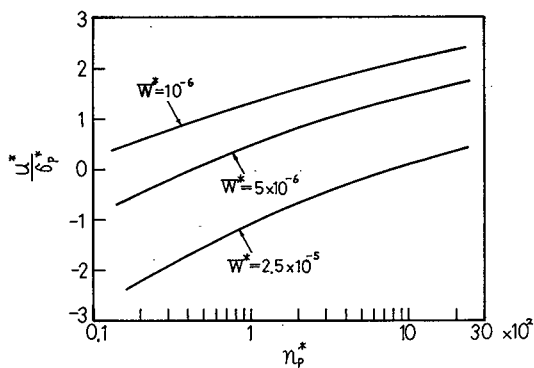
図 1.5.4 n_p^* と \frac{u^*}{\sigma_p^*} の関係 \beta^* = 0.01 \sigma_p = 8 \times 10^{-4}
