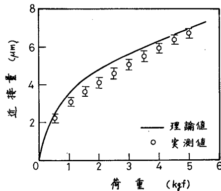
図 1.4.17 近接量に関する理論値と 実測値の比較
