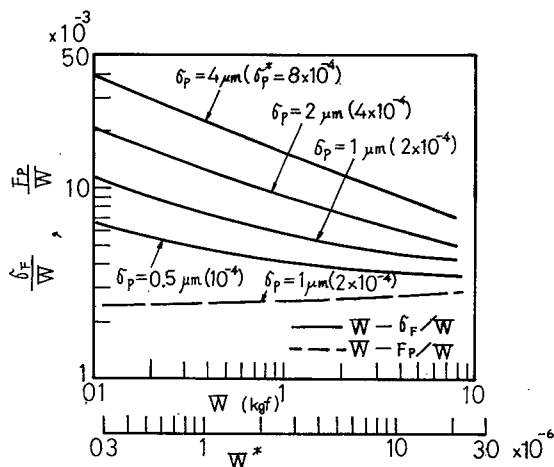
図 2.1.38 W と \sigma_F の関係
