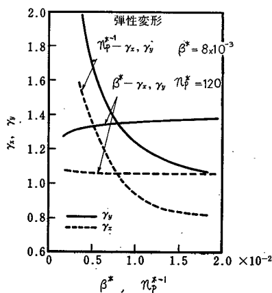
図 1.2.4 母材の弾性変形 W^* = 2 \times 10^{-6}
