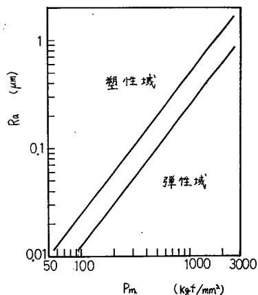
図 1.4.29 湿式ラップ仕上面における変形形態 R = 5 \text{ mm} E_1 = E_2 = 21000 \text{ kgf/mm}^2
