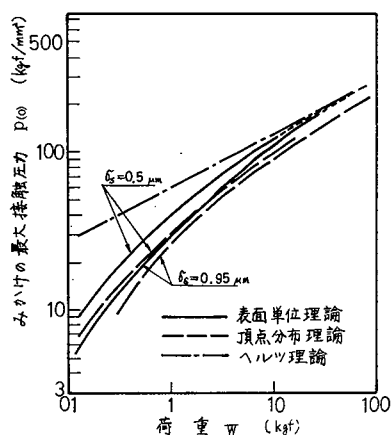
図 1.4.13 荷重とみかけの最大接触圧力の関係 \beta_s = 0.2 \text{ mm} R = 10 \text{ mm} E_1 = E_2 = 10000 \text{ kgf/mm}^2
