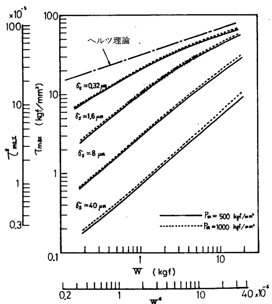
図 1.4.31 W と \tau_{max} の関係
