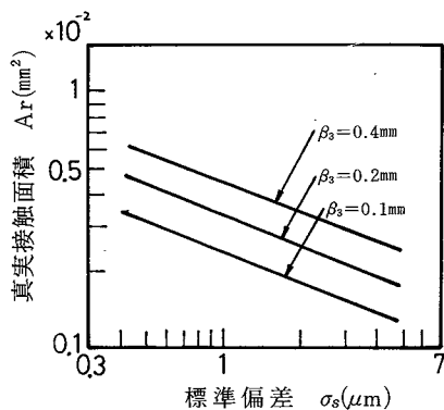
図 1.4.10 標準偏差と真実接触面積の関係 W = 1 \text{ kgf}
