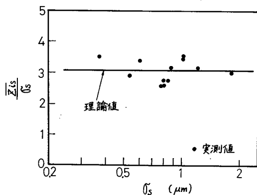
図 1.3.25 \bar{Z}_{is} の理論値と実測値の比較 R = 18 mm
