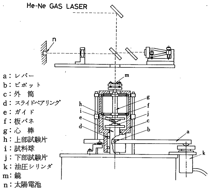
図 1.1.3 押付け実験装置
