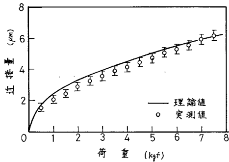
図 1.4.14 近接量に関する理論値と 実測値の比較
