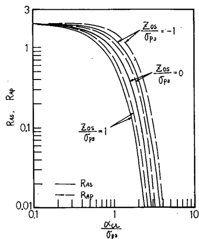
図1.4.28 R_{AS} と R_{AP} の比較
