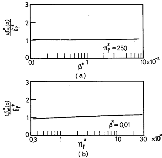
図 1.5.7 \beta^* , n_p^* と母材の弾性変形量の関係 \sigma_p^* = 8 \times 10^{-4} W^* = 2.5 \times 10^{-5}
