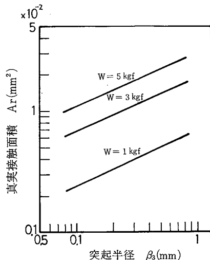
図 1.4.11 突起半径と真実接触面積 \sigma_s = 1 \mu\text{m}
