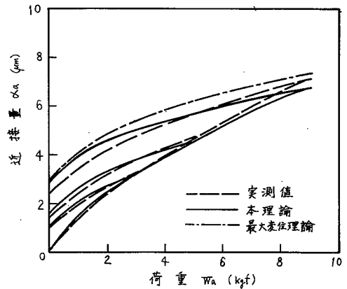
図 1.1.5 荷重と近接量の関係 (黄銅板試験片)
