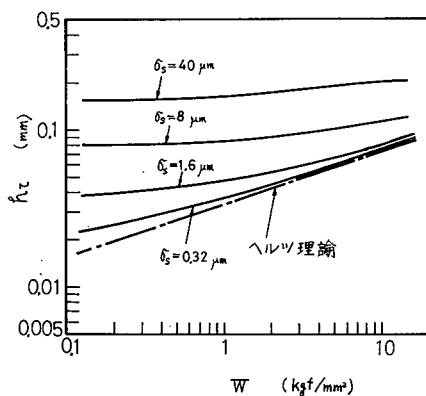
図 1.4.32 W と h_\tau の関係 p_m = 500 \text{ kgf/mm}^2
