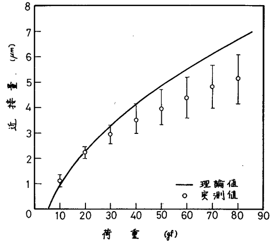
図 1.5.21 荷重と近接量の関係
