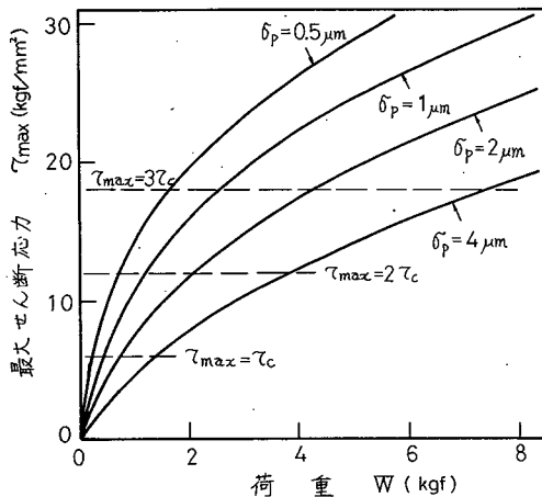
図 2.1.22 荷重と最大せん断応力の関係
