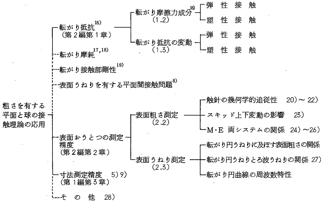
図２ 粗さを有する平面と球の接触理論の応用（本論文で扱う領域を実線で示す）
