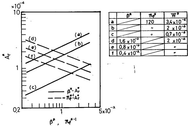
図 1.2.7 突起半径、密度と真実接触面積の関係
