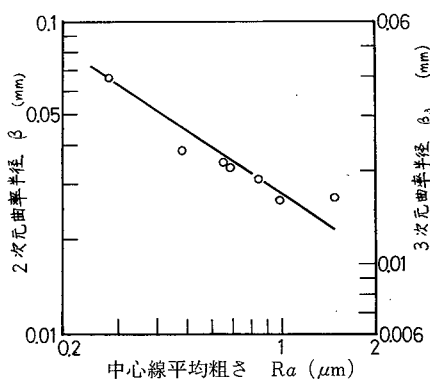
図 1.4.20 ラップ仕上面における突起先端曲率半径
