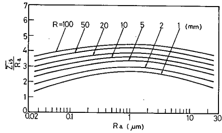
図 1.3.11 R_a と \bar{Z}_3/R_a の関係
