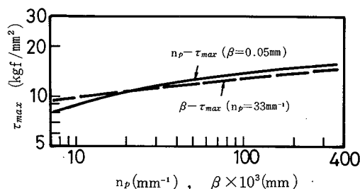
図 1.5.34 n_p , \beta と \tau_{max} の関係
