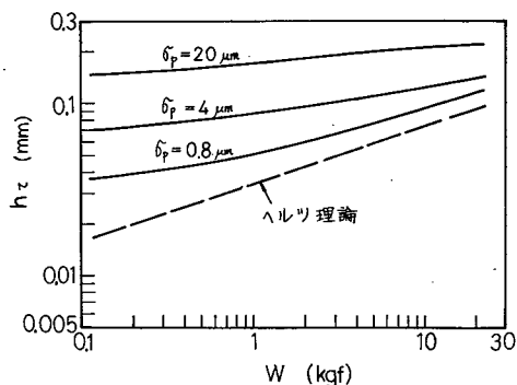
図 1.5.35 最大せん断応力が生じる深さ
