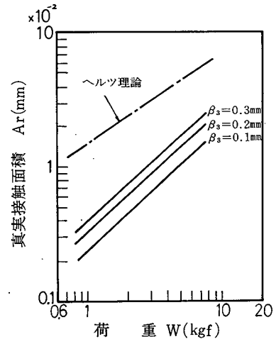
図 1.4.9 荷重と真実接触面積の関係 \sigma_s = 1 \text{ } \mu\text{m}
