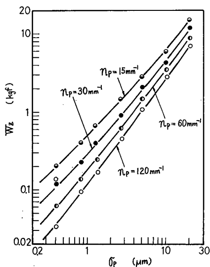
図 1.5.37 \sigma_p と W_z の関係 \beta=0.1\text{mm} R=5\text{mm} E_1=E_2=21000\text{kgf/mm}^2
