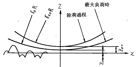
図 1.5.2 除荷過程の接触状態
