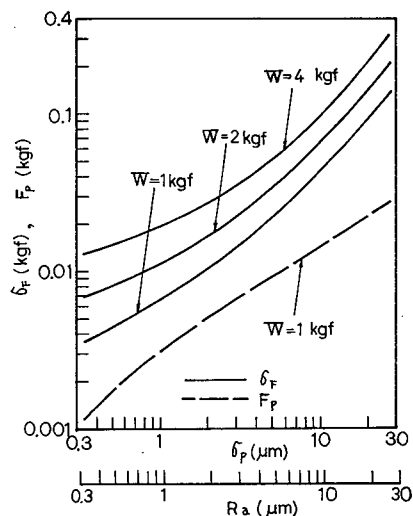
図 2.1.40 R_a と \sigma_F の関係
