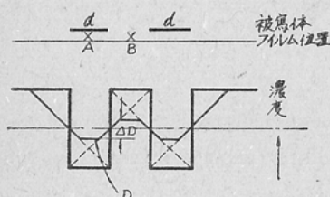
第1圖 フィルム上における分解能とぼけの大きさとの関係
