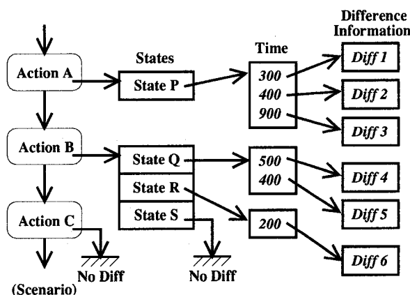
図 5.4: 差分の保存
