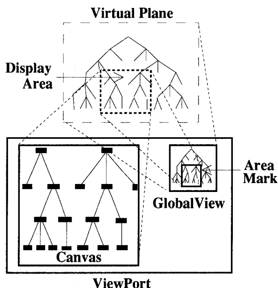
図 3.3: Canvas と GlovalView
