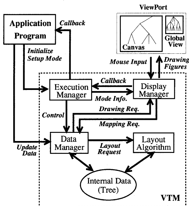
図 3.1: VTM の構成
