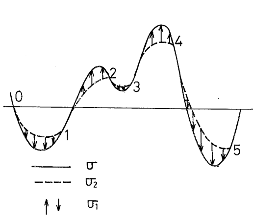
(図6.2) 外応力とバネ、スライダへの応力の変動状況
