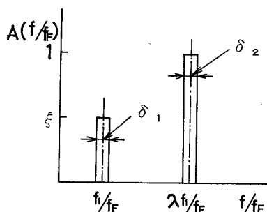
( 図 5 ・ 8 ) 二個の狭帯域スペクトルのある場合
