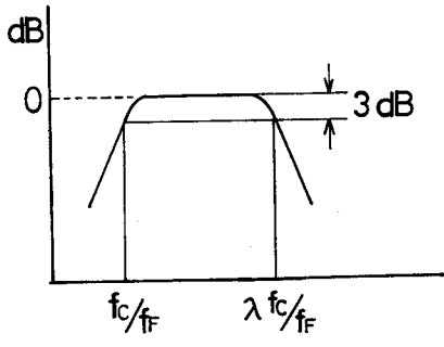
(図 5・4) -12 \text{ dB/oct} のカットのパワースペクトル
