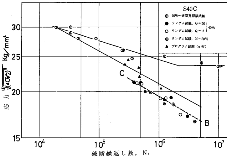
（図3・5） 応力レンジペアの \bar{m}a 乗平均値で整理した試験結果 （S40C）
