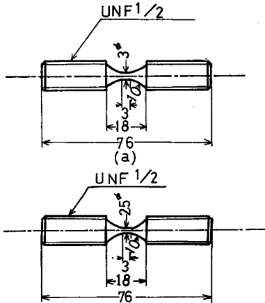
(図3・6) 試験片の形状 寸法
