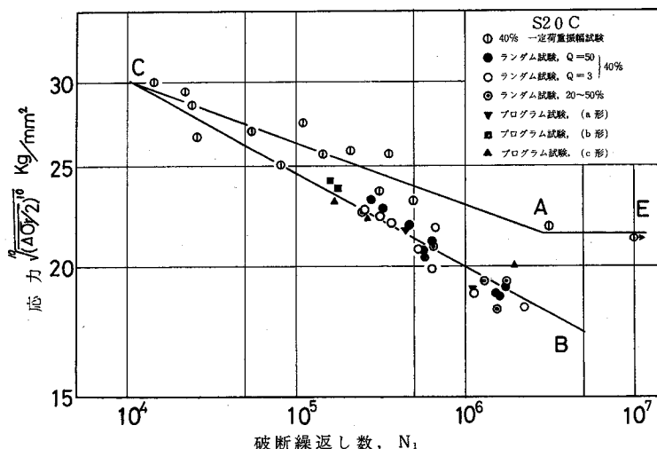
（図3・3） 応力レンジペアの \bar{m}a 乗平均値で整理した試験結果 （S20C）
