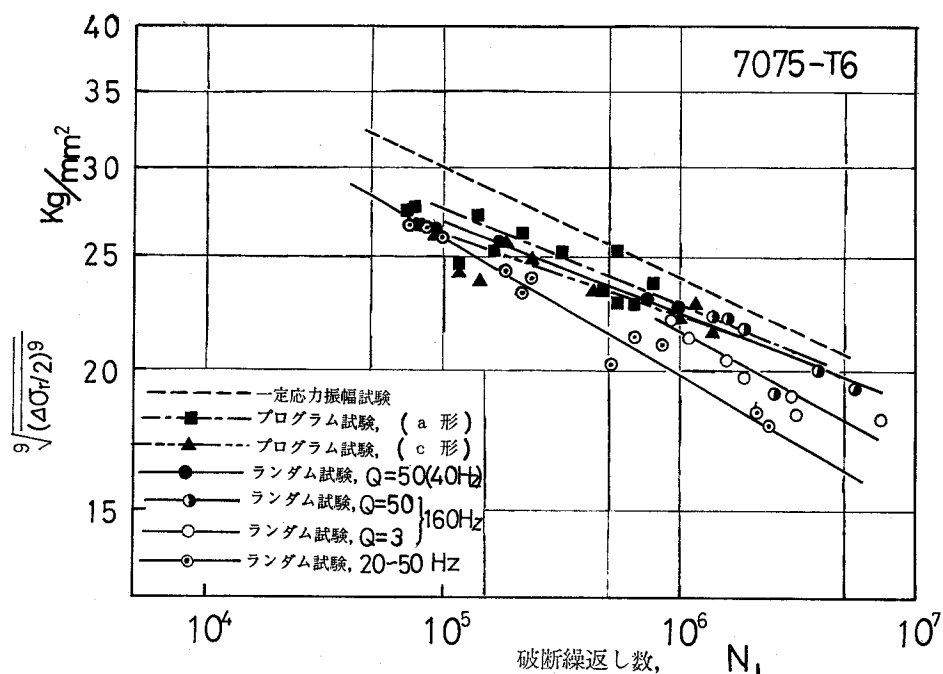
(図3・10) 応力レンジペアの \overline{ma} 乗平均値で整理した試験結果(7075-T6)
