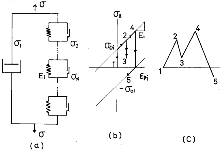
(図 6・1) バネ、スライダモデル
