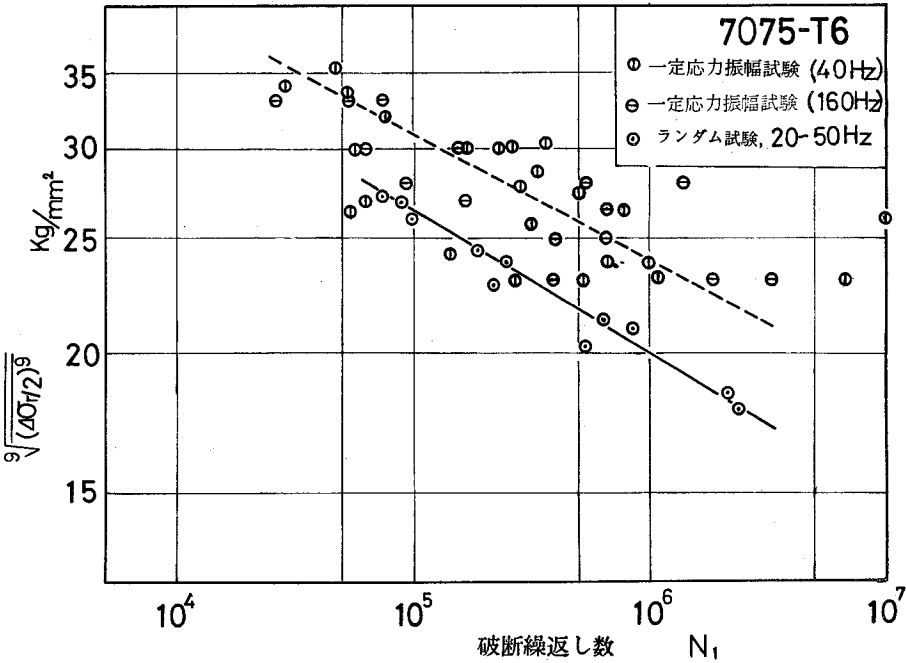
(図3・9) 応力レンジペアの \bar{ma} 乗平均値で整理した試験結果(7075-T6)
