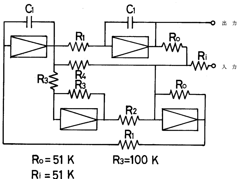
（図2・4） バンドパスフィルタ
