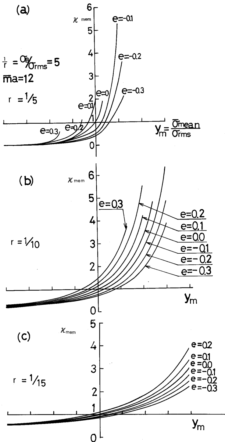
( 図 5 ・ 2 4 ) レーレ分布のとき非対称性が \chi_{mem} におよぼす影響
