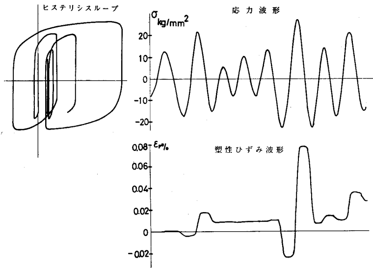
( 図 6 ・ 8 a , b ) ランダム 応力 対 する ヒステリシスループ ( 計 算 例 )
