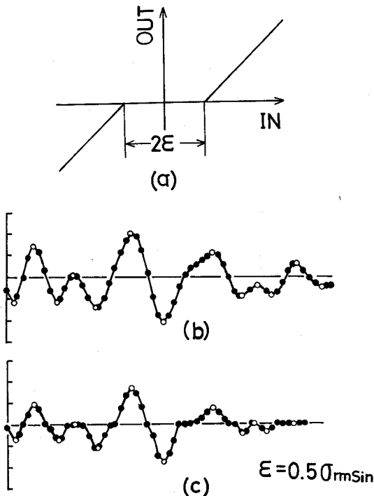
( 図 4 ・ 7 a , b , c ) 折線非線形系を通過した波形
