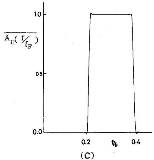
(図4・4, a, b, c) Gibbs の現象と収束係数の効果
