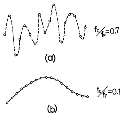
(図4・5 a, b) しゝ断周波数の上限と波形
