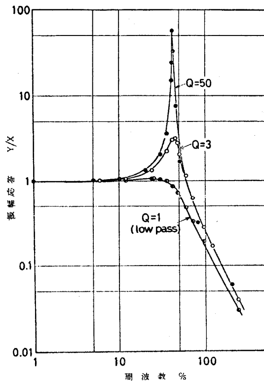
( 図 2 - 5 ) フィルタ周波数特性
