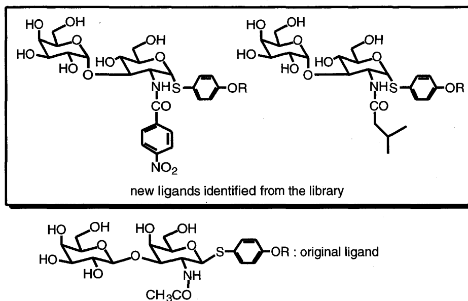
Fig. 1-1 Kahne のエンコード糖鎖ライブラリーから見出された Bauhinia purpurea レクチンの新リガンド
