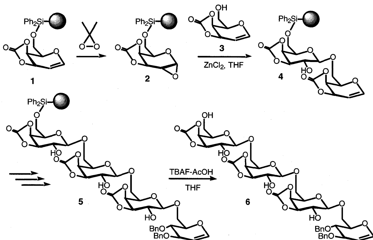
Scheme 1-1 1,2-アンヒドロ糖を糖供与体にした糖鎖固相合成
