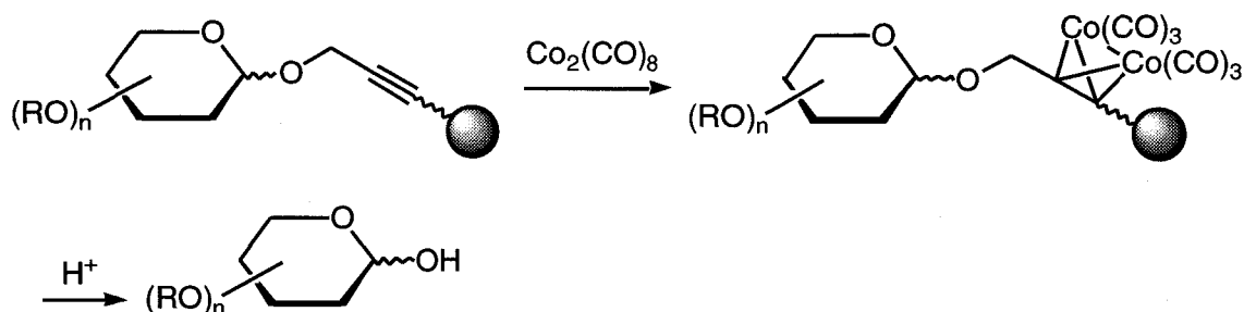
Fig. 3-1 新しいアルキン型リンカー
