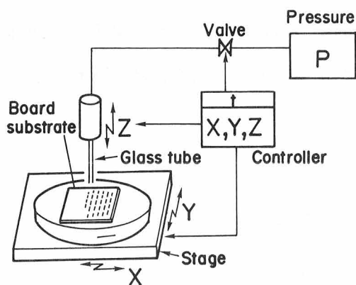
図3.16 製作した自動水銀注入装置
