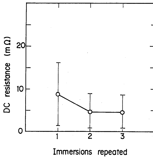
図3.48 コネクタ直流抵抗値の測定結果例
