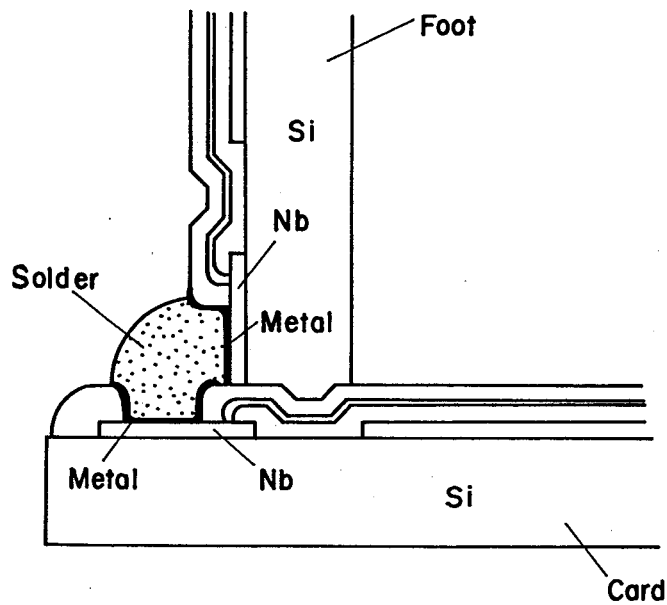
図4.8 フィレの構成断面図
