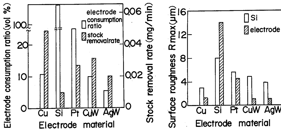
図3.35 シリコン基板の放電加工特性
