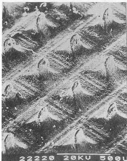
図3.25 ワイヤカット放電加工によるマイクロピン
