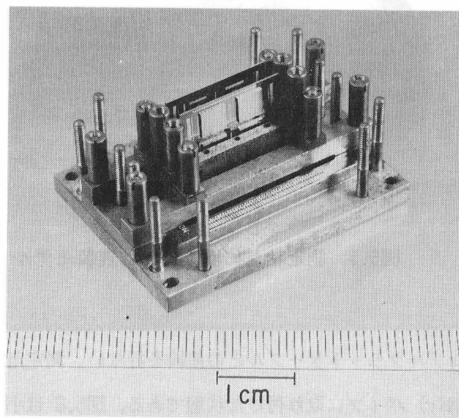
図5.4 ホルダに組み立てた実装モデル
