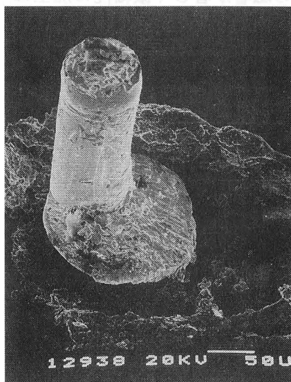
図3.23 塑性加工によるマイクロピン
