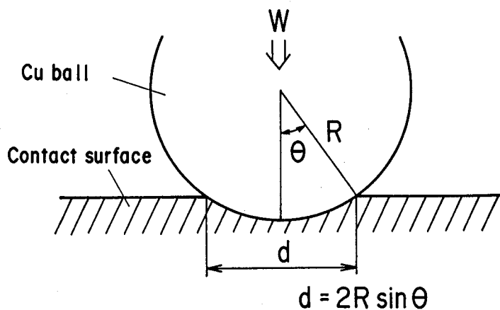
図4.10 ケーブルとボールの接続部における接触モデル
