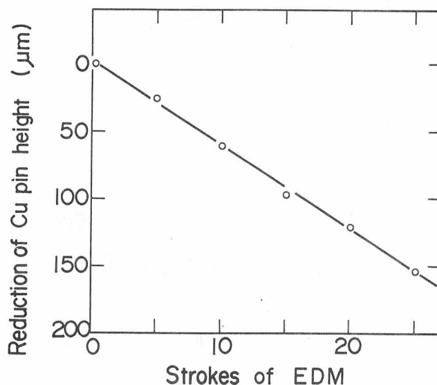
図3.41 シリコン基板の放電加工における電極高さの変化
