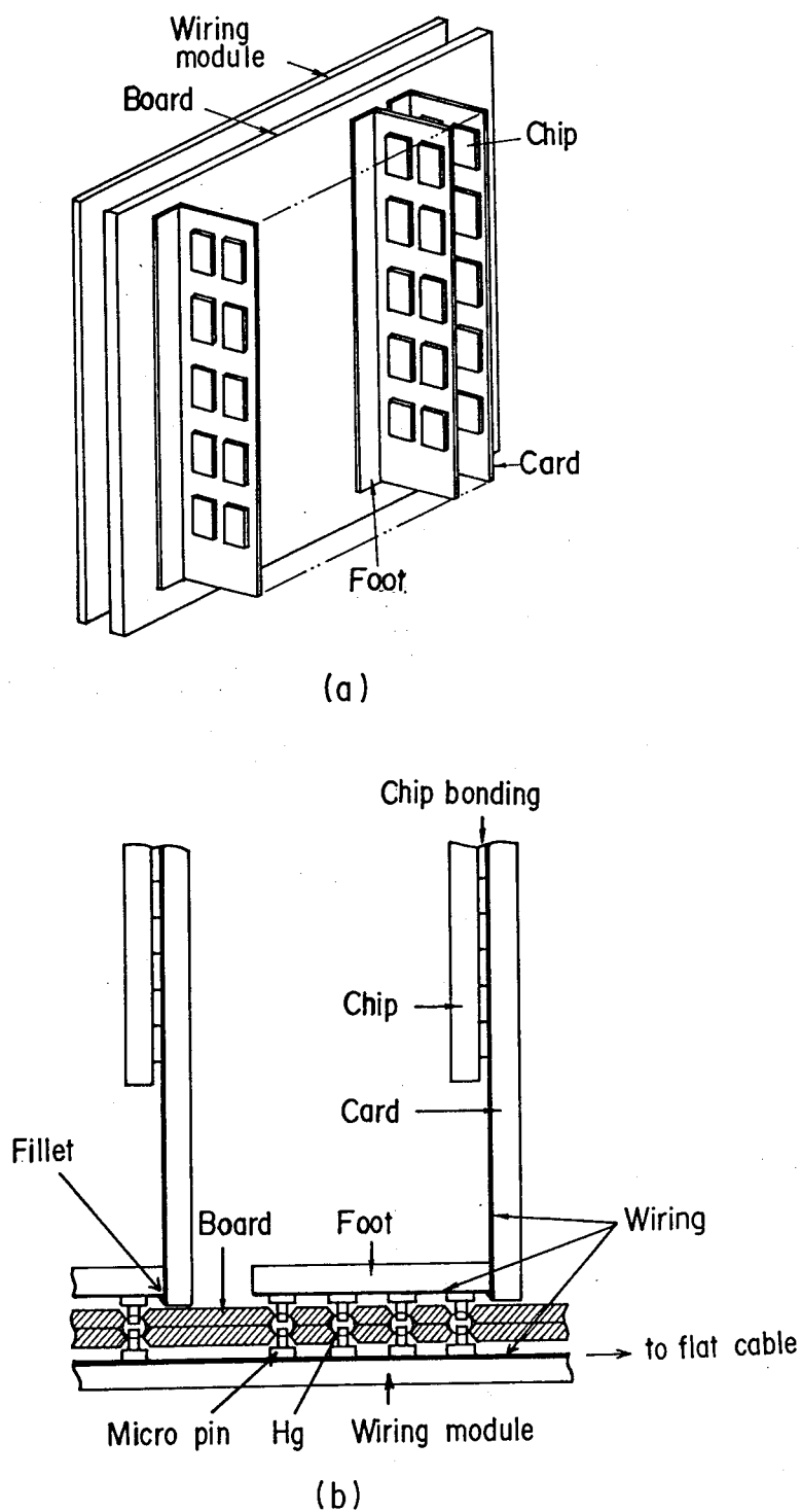
図4.1 マイクロコネクタによる超伝導素子の実装構成法
