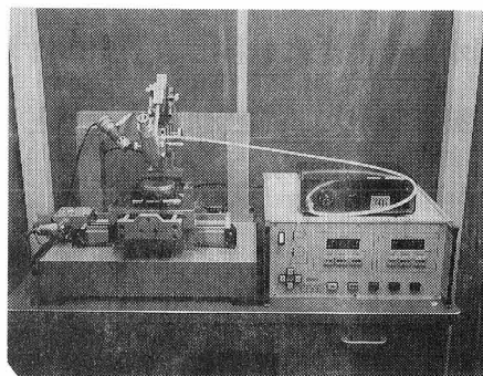
図3.16 製作した自動水銀注入装置
