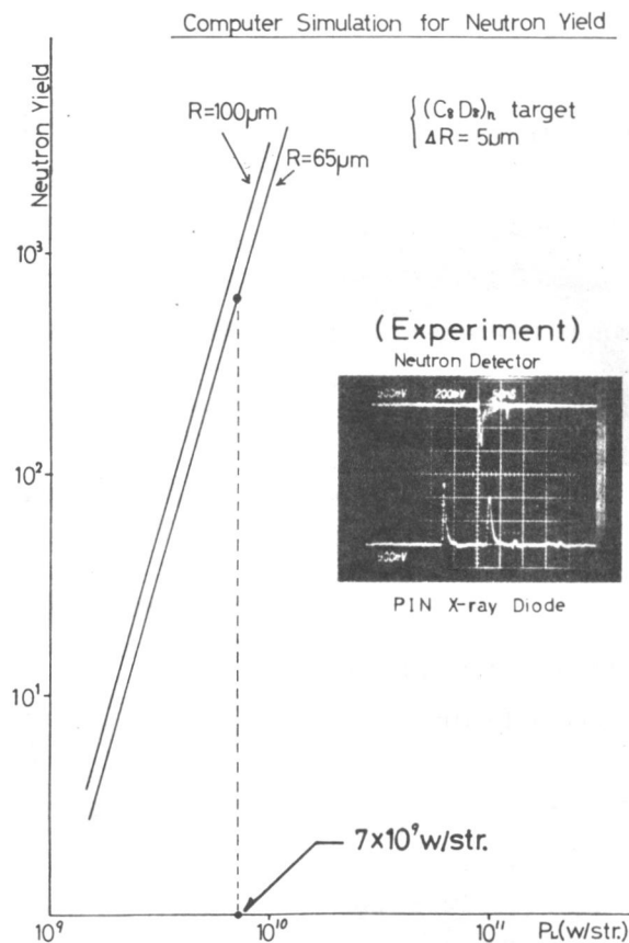
図3-18 中性子検出器から得られた信号(上)とタイムマーカー用の2ch X線信号 レーザー照射時に発生高エネルギー電磁波(X線もしくは \gamma 線)から64 nsec遅れて中性子信号が得られている。グラフは (\text{C}_8\text{D}_8)_n シェルタ ターゲットに対するシミュレーション結果で、生成中性子数は観測値と一致 している。
