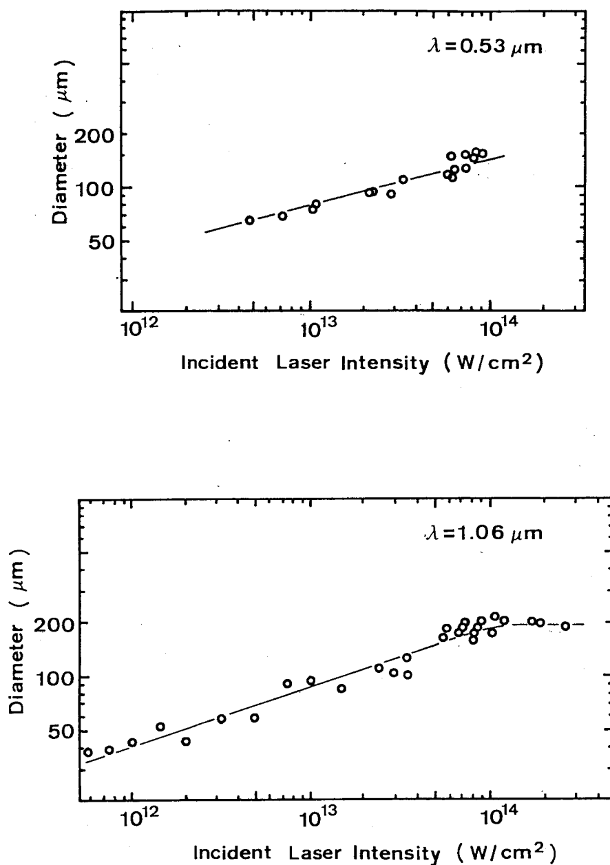
図4-17 入射レーザー強度に対する輻射領域のプラズマの直径，X線ダイオードの信号比から求めた輻射温度を与える平均的なプラズマ規模に相当する。1.06 μm レーザーの場合，プラズマ径の増加に飽和傾向が見られる。
