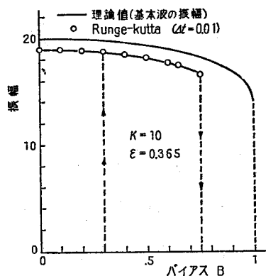
図2.13 バイアスによる振幅の変化
