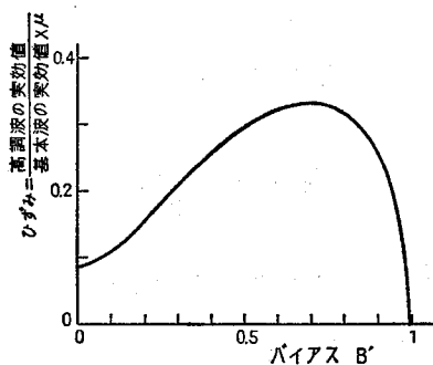
図 2.20 バイアスによる歪の変化 (小振幅動作)
