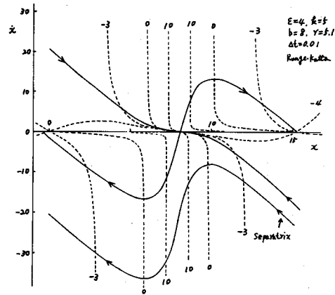
図 2.28 3安定マルチバイブレータの位相面軌跡
