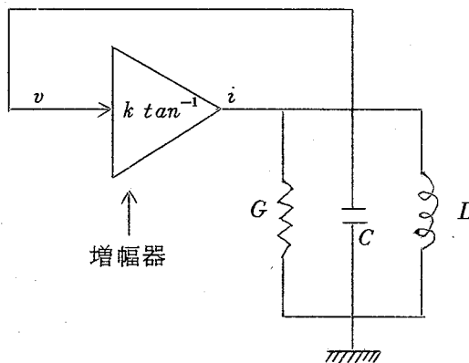
図 2.6 発振回路
