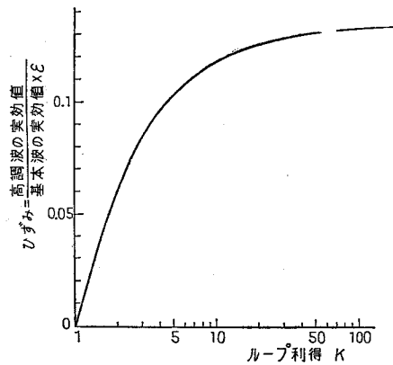
図 2.10 ループ利得による歪の変化
