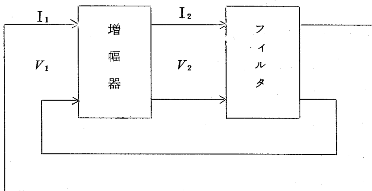
図2.1 一般的な発振回路
