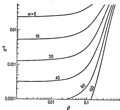
図 4.13 AM 検波器の位相誤差の分散
