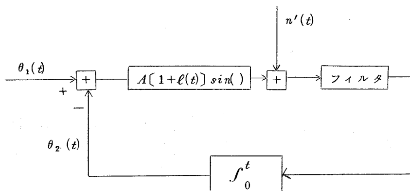
図 4.2 リミッタの無い位同期ループ
