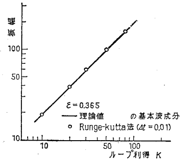
図 2.8 ループ利得による振幅の変化
