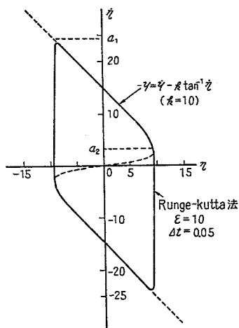
図 2.11 マルチバイブレータの位相面軌跡
