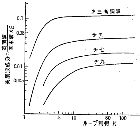
図 2.9 ループ利得による高調波の変化
