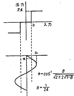
図2.21 プッシュプル発振器の入出力特性
