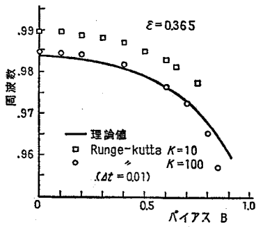
図 2.15 バイアスによる周波数の変化
