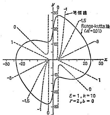
図 2.26 リミットサイクルの軌跡
