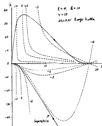
図2.25 双安定MVの位相面軌跡
