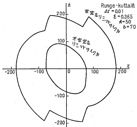
図 2.22 安定と不安定のリミットサイクルの軌跡
