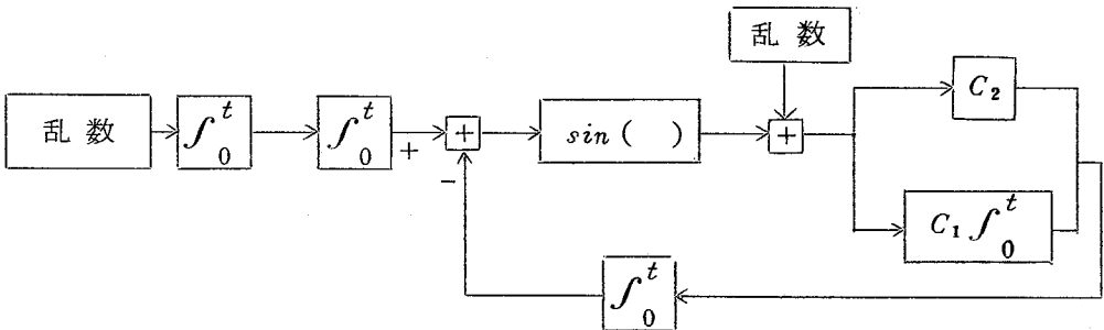
図4.5 デジタル計算機のシミュレーションモデル
