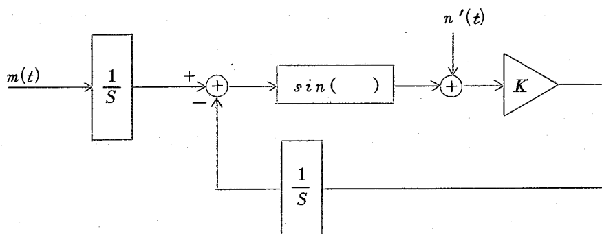
図 4.4 一次の位相同期ループ
