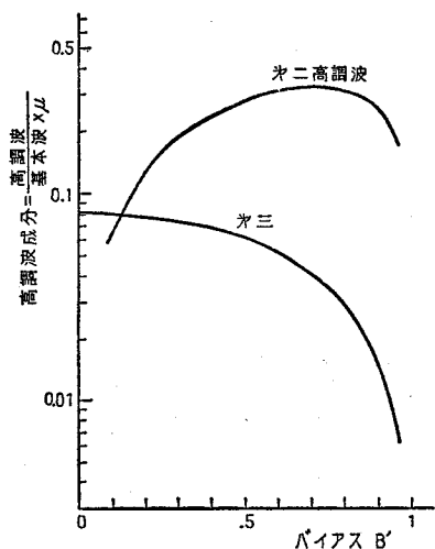
図 2.19 バイアスによる高調波の変化 (小振幅動作)
