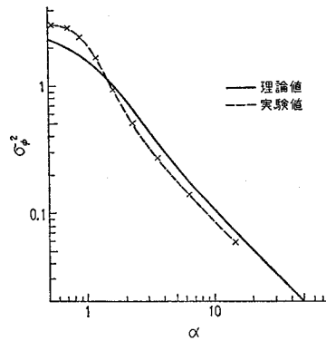
図 4.7 Kalman-filter による計算機シミュレーション
