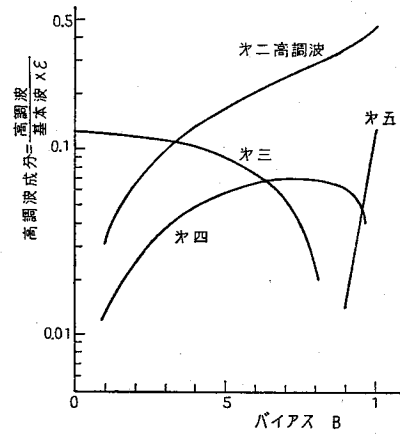
図 2.16 バイアスによる高調波の変化 (大振幅動作)
