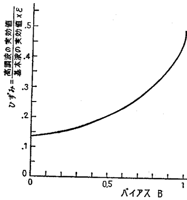
図 2.17 バイアスによる歪の変化 (大振幅動作)
