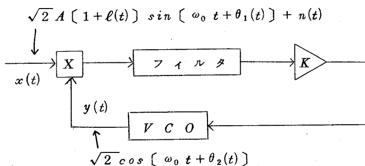
図 4.1(a) 位相同期ループ
