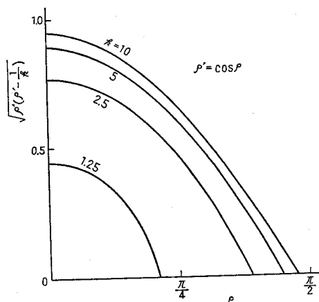
図 2.24 位相遅れ対振幅特性
