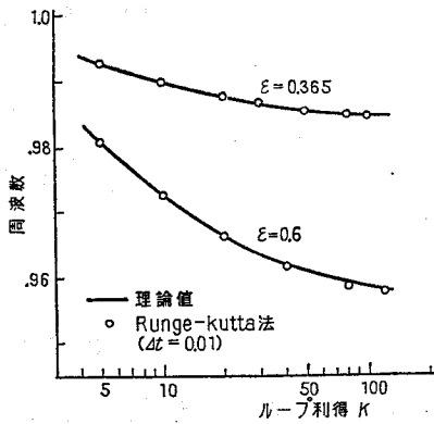
図 2.7 ループ利得による周波数の変化
