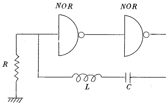
図 2.5 DICを使った発振器
