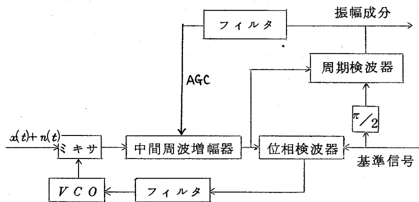
図 4.10 AGC ループを持った位相同期ループ
