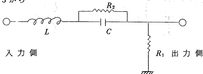
図2.3 フィルタ
