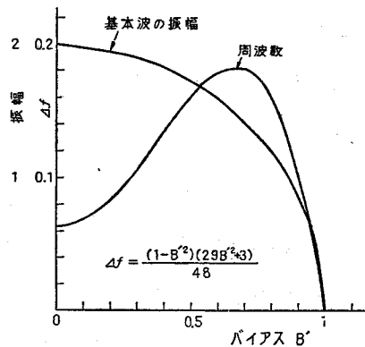
図2.18 バイアスによる振幅と周波数（小振幅動作）
