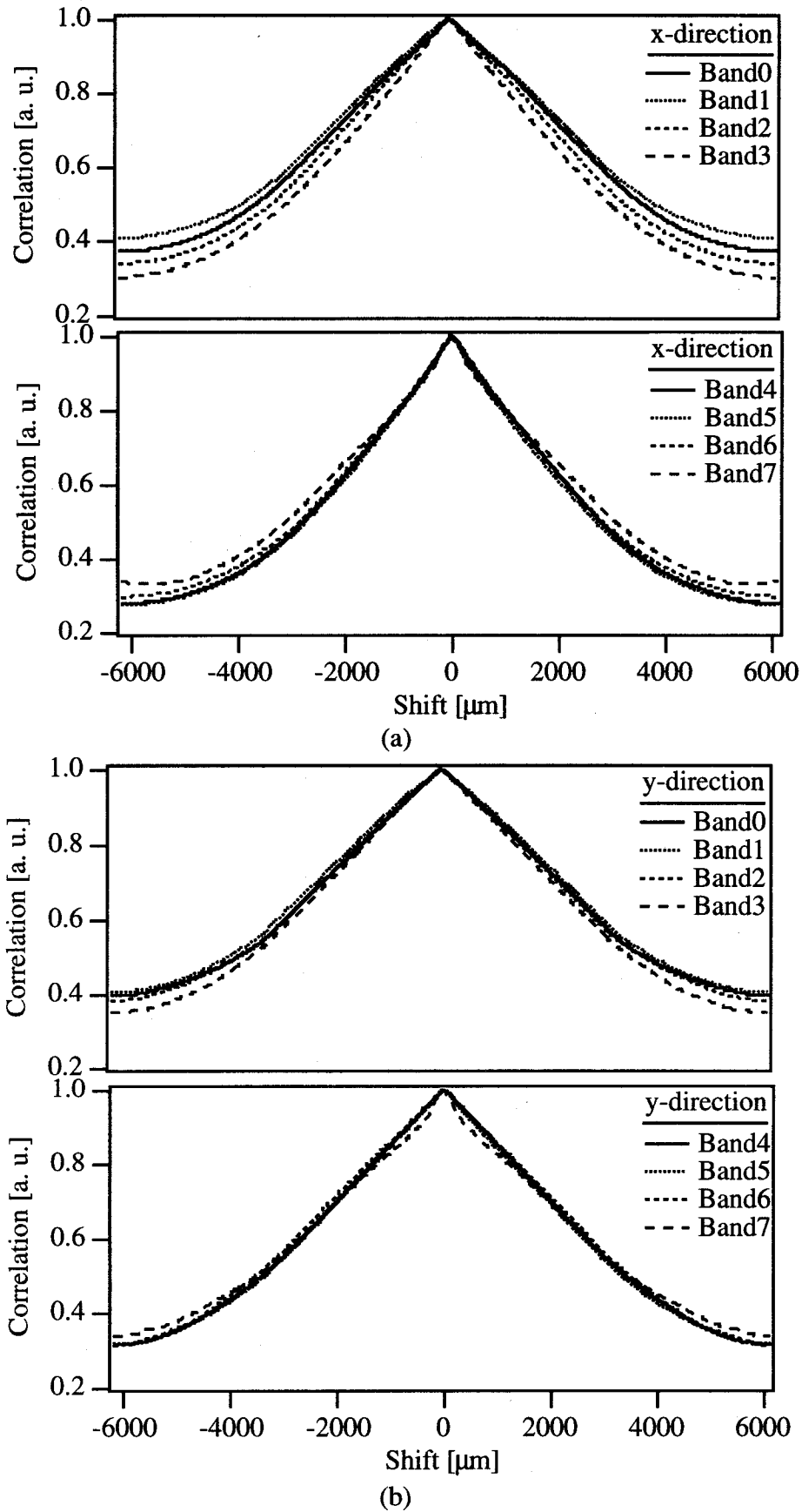
図 4.21 ファーフィールドの端付近の分光画像の 2 次元相関関数： (a) 横方向の断面 (b) 縦方向の断面
