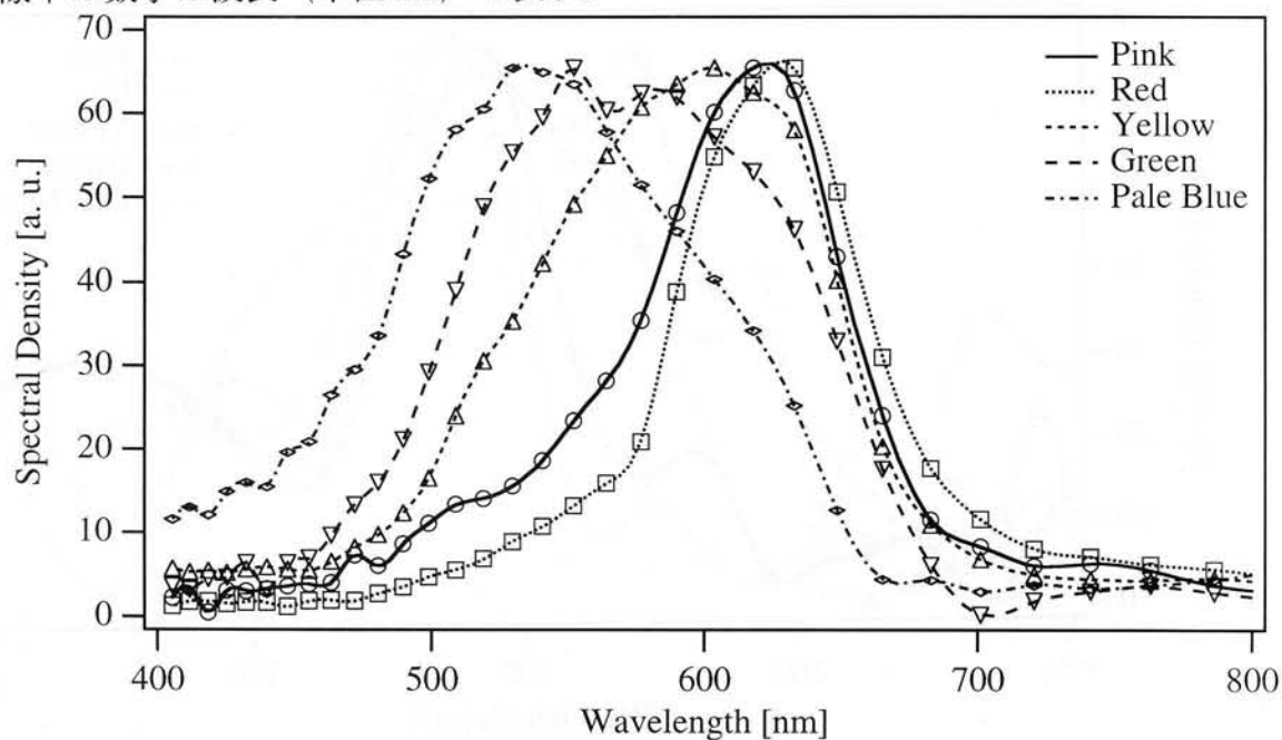
図 2.20 像面フーリエ分光映像法により測定された多色物体（図 2.14）のスペクトルの例
