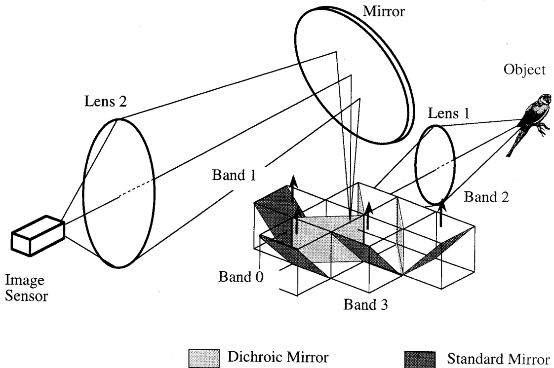
図4.4 ダイクロイックミラーを用いたマルチチャネル分光映像装置
