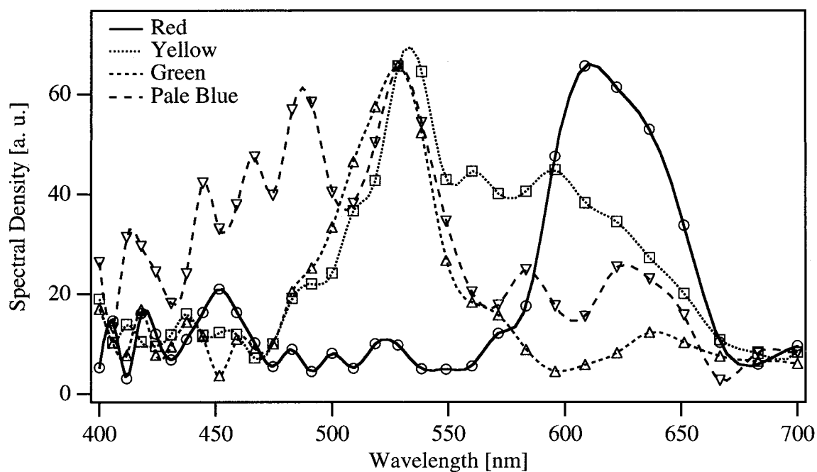
図 2.24 多重像フーリエ分光映像法により測定された 多色物体（図 2.21）のスペクトルの例
