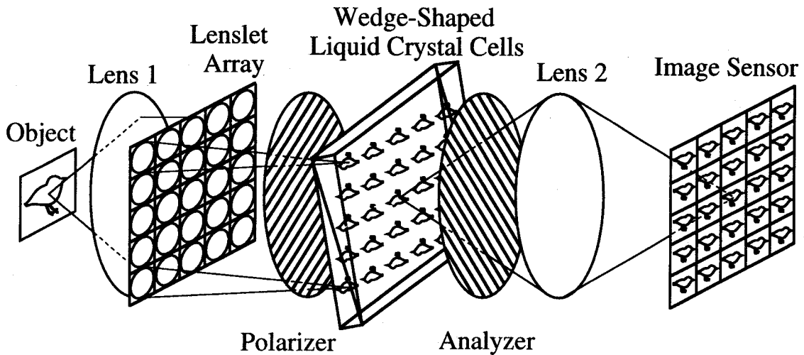
図3.2 くさび型液晶偏光干渉計を用いた多重像フーリエ分光映像法の光学系
