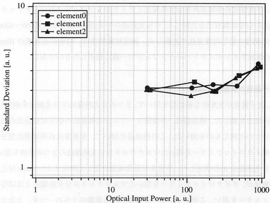
図 5.6 検出器の雑音特性
