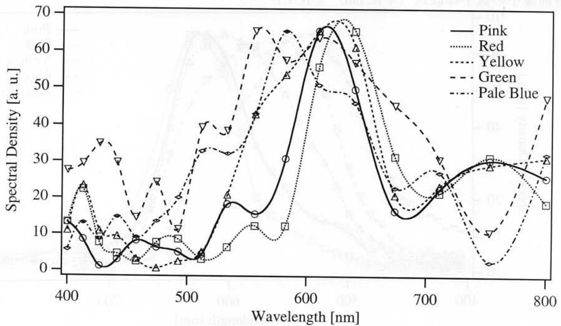
図 2.18 多重像フーリエ分光映像法により測定された多色物体（図 2.14）のスペクトルの例
