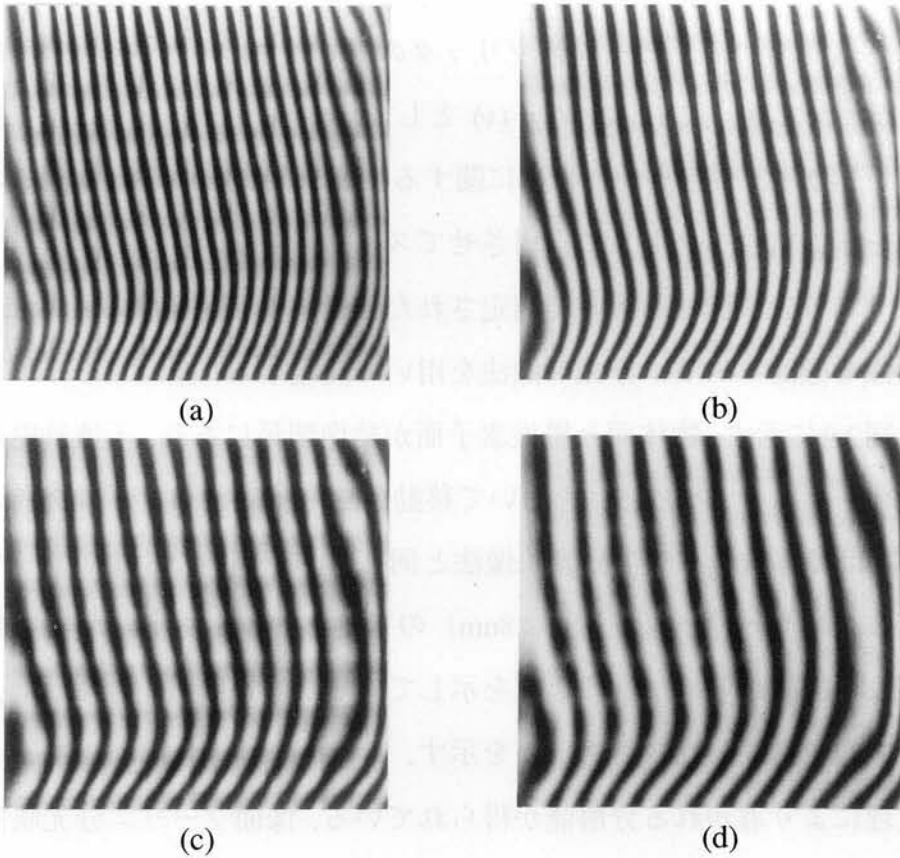
図2.7 干渉フィルターによる単色光の干渉縞（干渉計の全面）： 干渉フィルターの中心波長はそれぞれ，(a) 450nm, (b) 500nm, (c) 550nm, (d) 600nm
