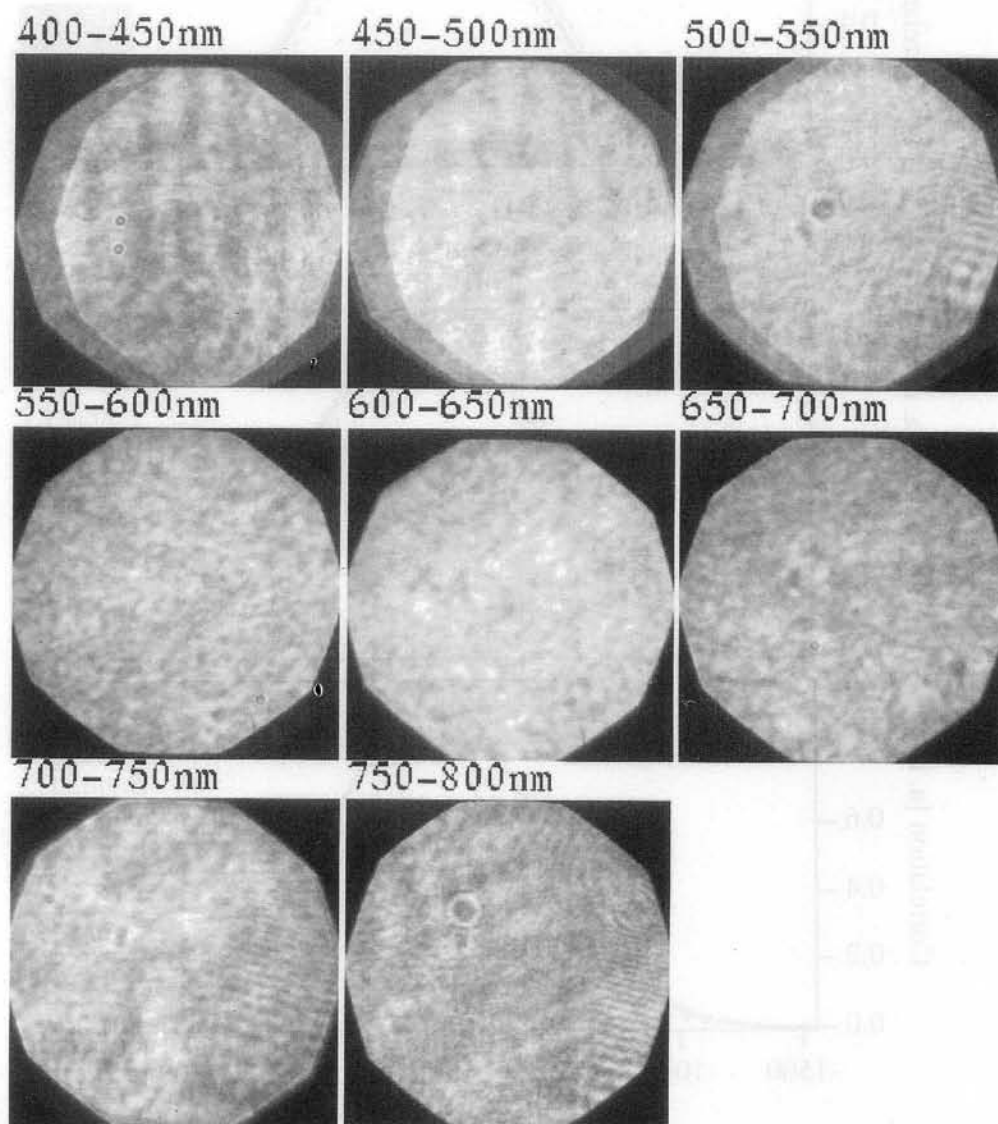
図4.18 ファーフィールドの中心付近の分光画像
