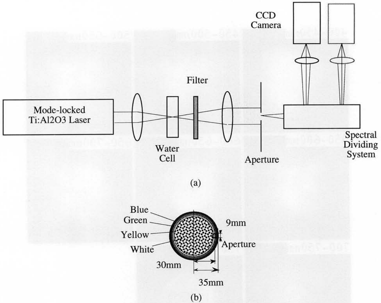
図4.15 ファーフィールド観察光学系：(a) 光学系， (b) ファーフィールドパターンと開口の位置
