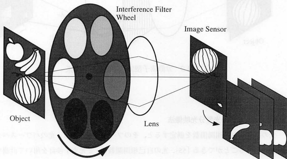
図1.1 波長帯域選択型分光映像法の光学系
