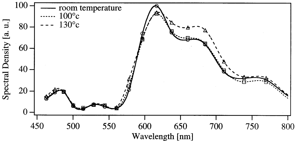
図 3.9 スペクトルの温度変化
