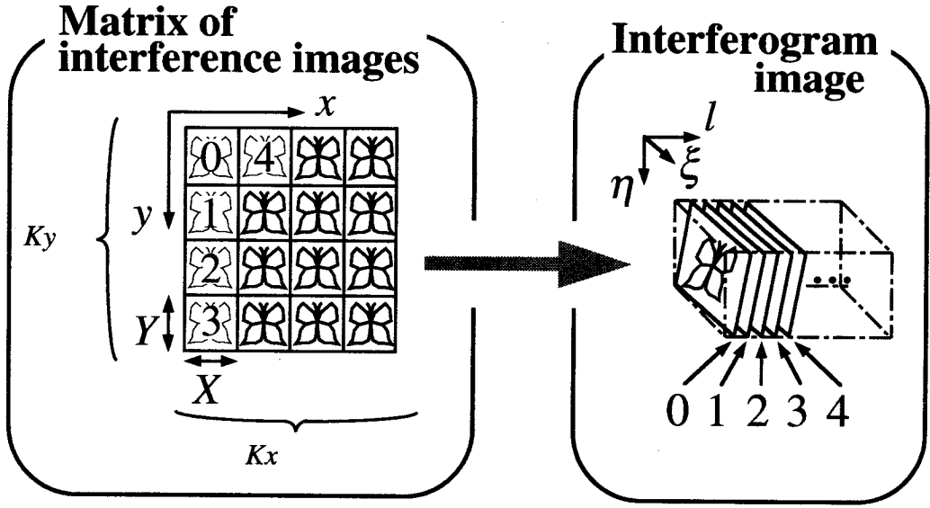
図2.2 干渉像マトリクスとインターフェログラム画像
