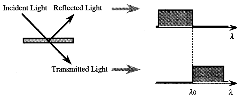
図4.1 ダイクロイックミラー
