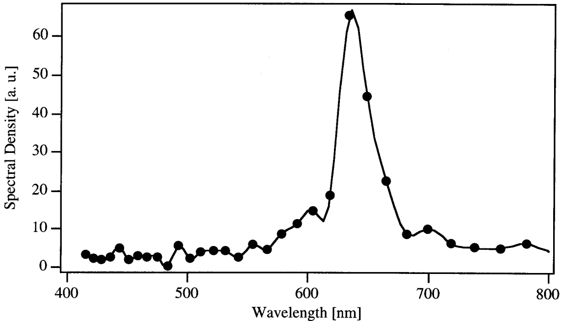
図 2.10 像面フーリエ分光映像法により測定された He-Ne レーザーのスペクトル
