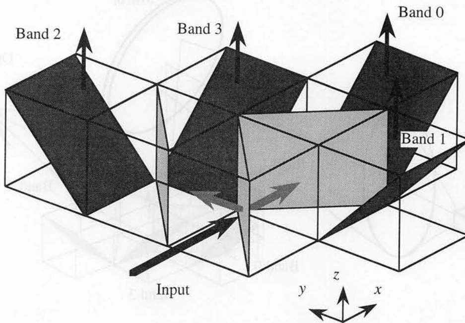
図4.3 ダイクロイックミラー配置例
