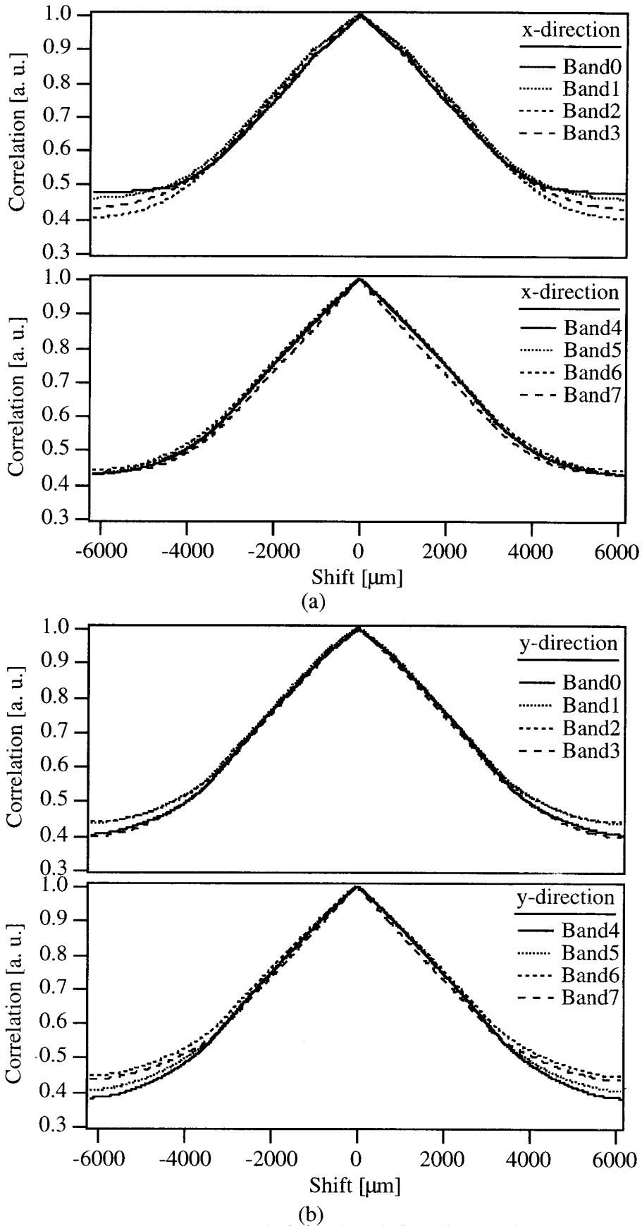
図4.19 ファーフィールドの中心付近の分光画像の2次元相関関数： (a) 横方向の断面 (b) 縦方向の断面
