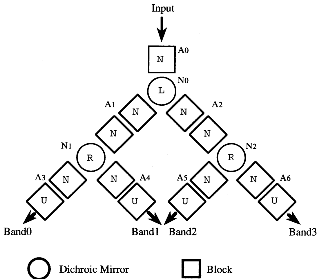
図4.5 木構造
