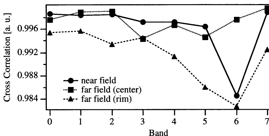
図4.22 相互相関値
