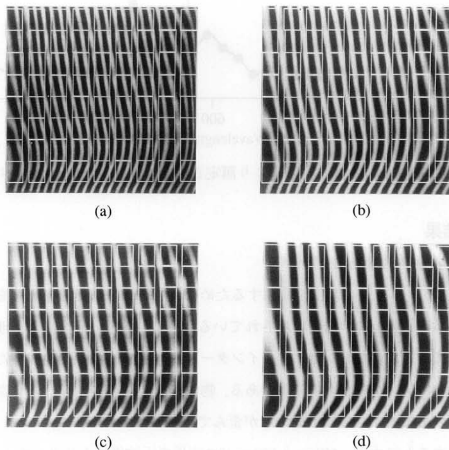
図 2.11 干渉フィルターによる単色一様物体の干渉像マトリクス (8×9 個の干渉像)：干渉フィルターの中心波長はそれぞれ、(a) 450nm, (b) 500nm, (c) 550nm, (d) 600nm
