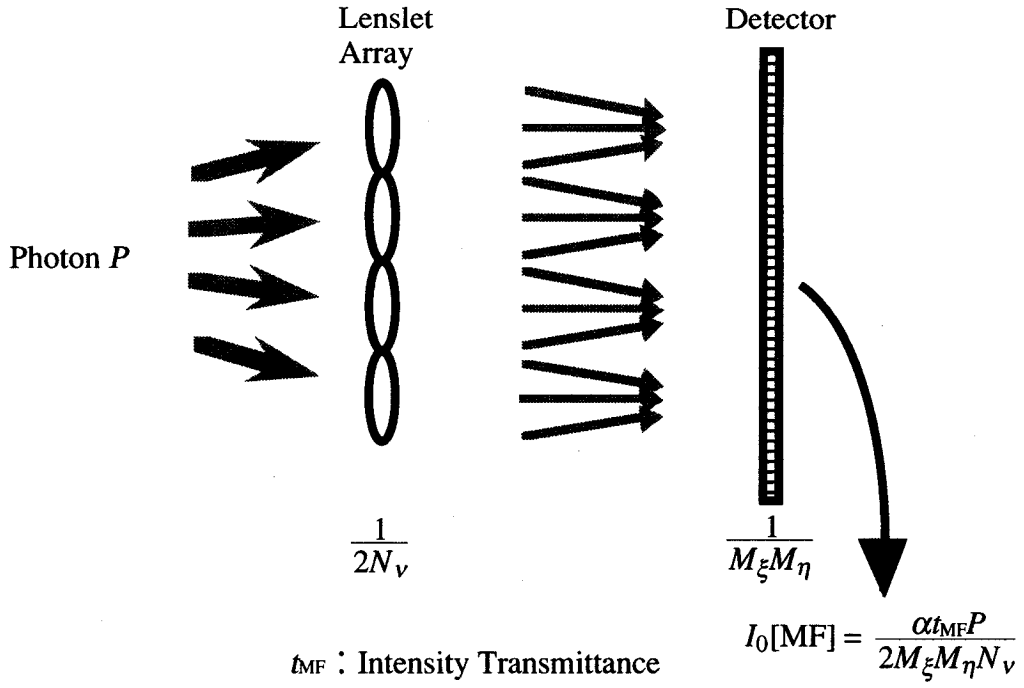
図5.2 多重像フーリエ分光映像法
