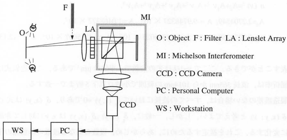
図2.3 多重像フーリエ分光映像システム
