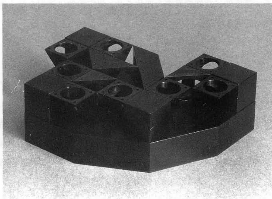
図 4.13 波長分割部分（ダイクロイックミラー装着前）
