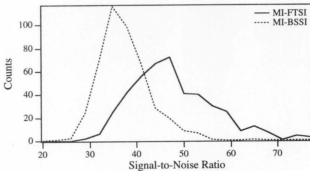
図 5.5 光子雑音が支配的な場合の分光画像の信号対雑音比のヒストグラム
