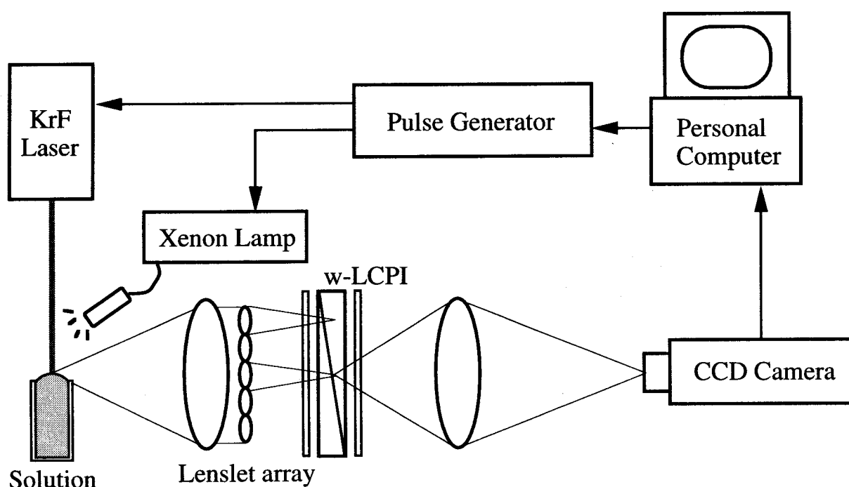
図3.3 液体のレーザーアブレーション測定システム
