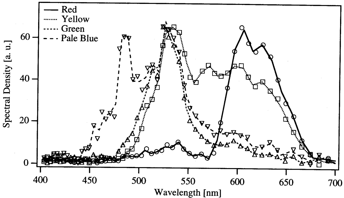
図 2.26 像面フーリエ分光映像法により測定された 多色物体（図 2.21）のスペクトルの例
