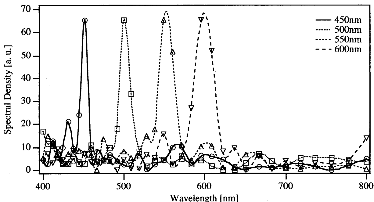
図 2.13 単色一様物体のスペクトルの例
