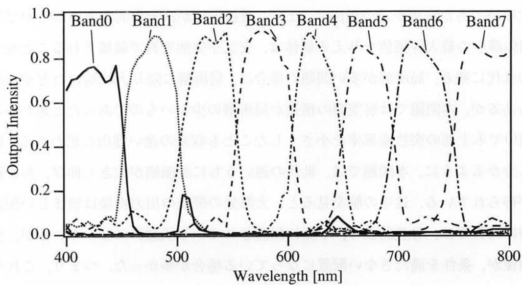
図 4.12 各出力画像の波長帯域
