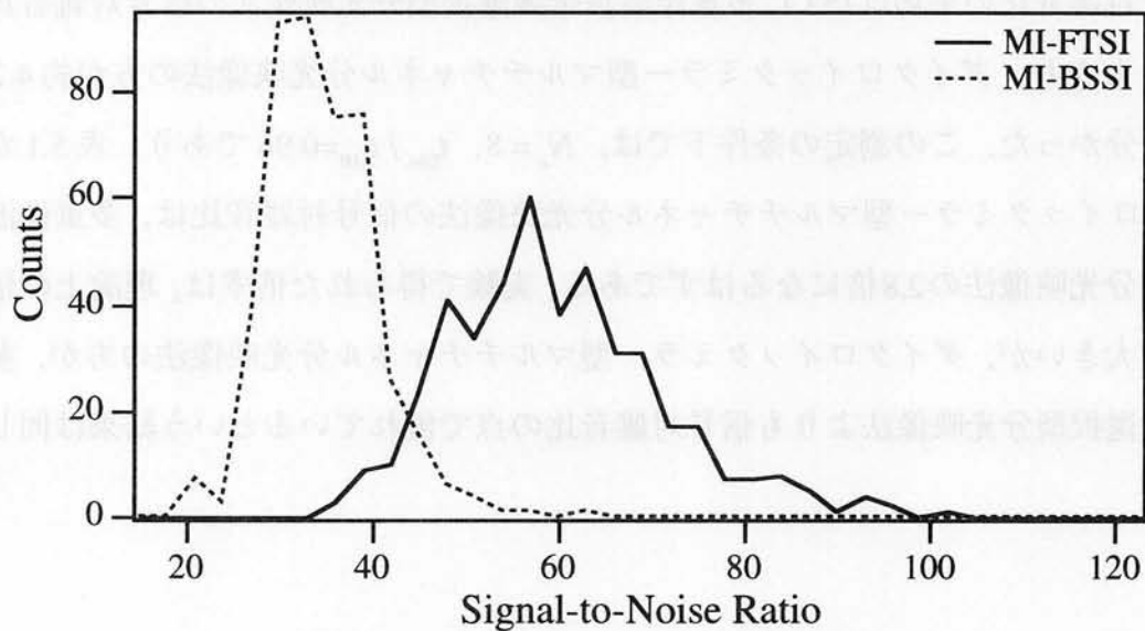
図 5.7 検出器雑音が支配的な場合の分光画像の信号対雑音比のヒストグラム
