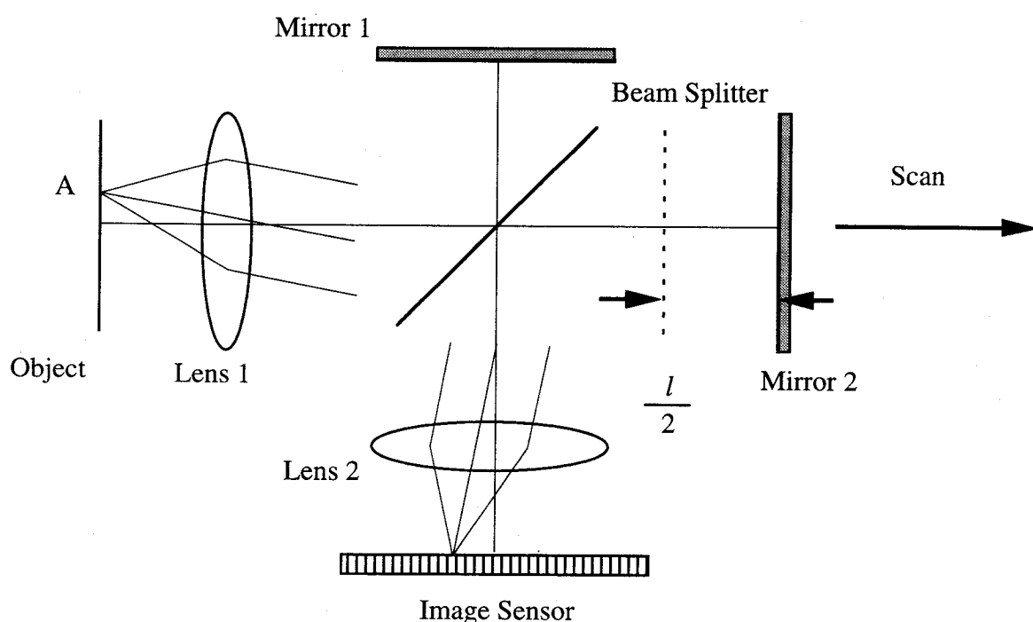
図1.3 フーリエ分光型分光映像法の原理
