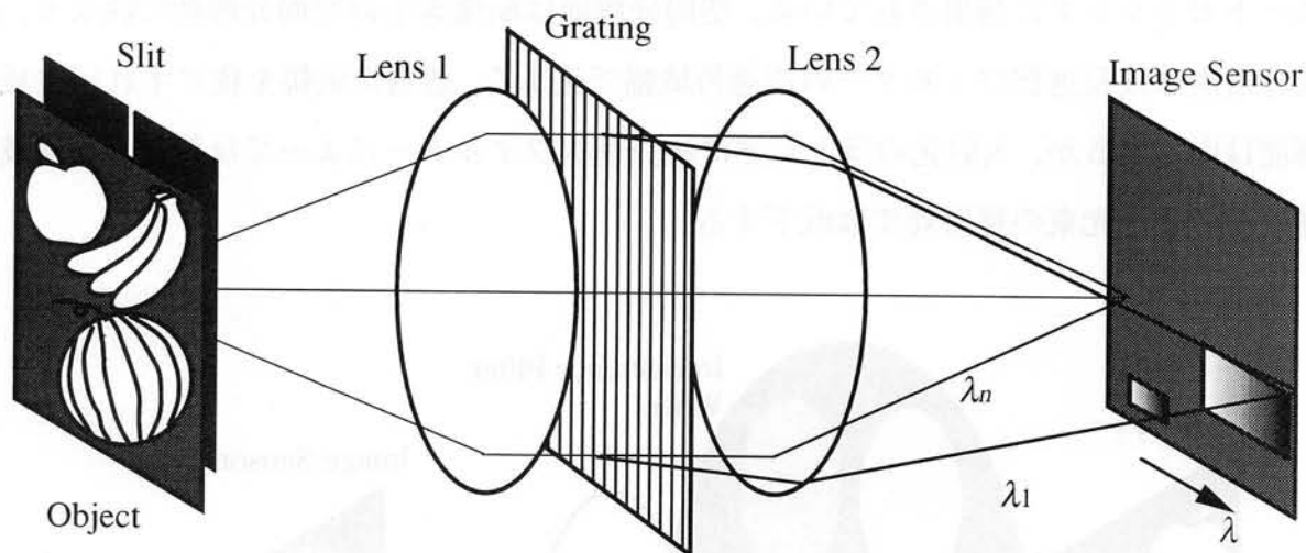
図1.2 分散素子型分光映像法の光学系
