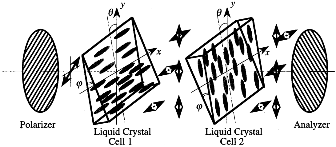
図3.1 くさび型液晶偏光干渉計
