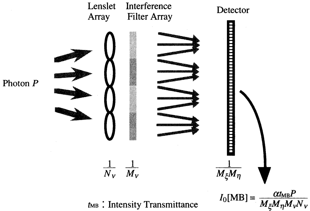
図5.1 多重像波長帯域選択型分光映像法
