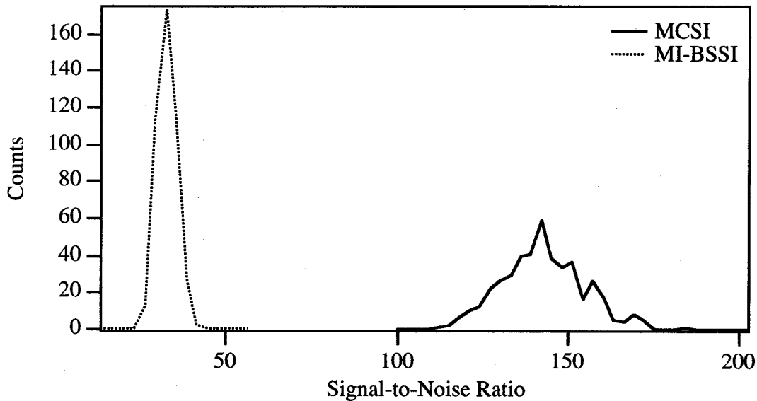
図 5.8 光子雑音が支配的な場合の分光画像の信号対雑音比のヒストグラム
