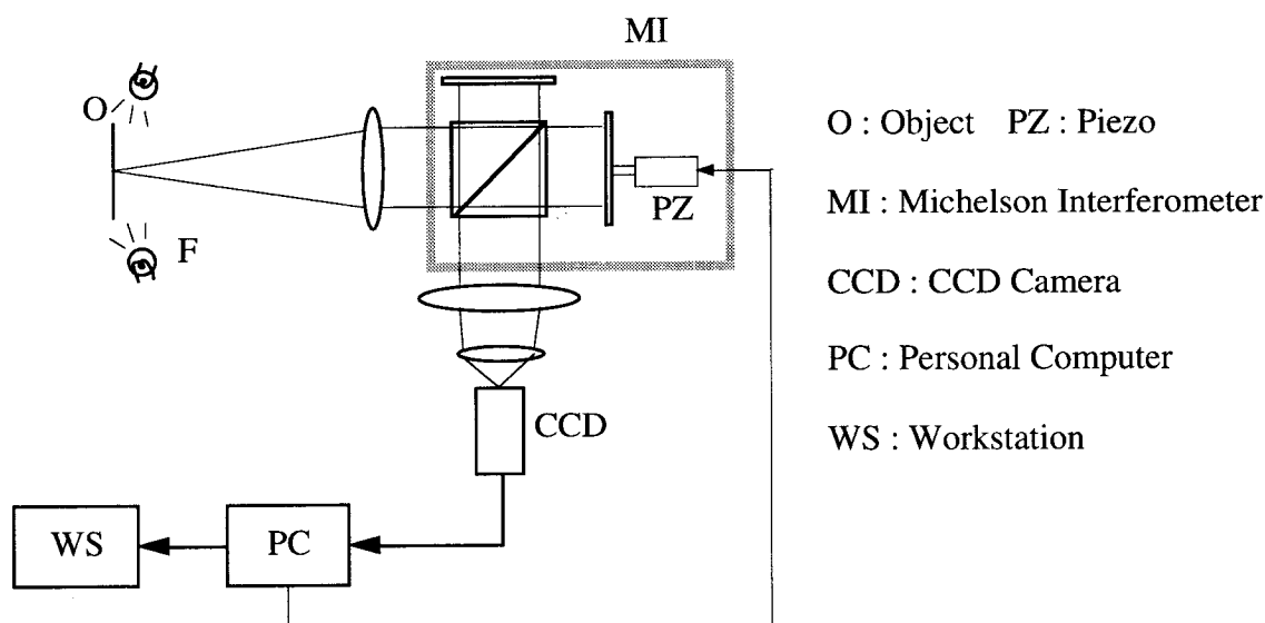
図2.9 像面フーリエ分光映像システム
