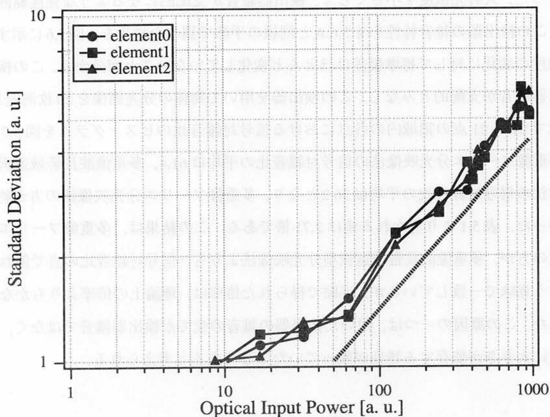
図 5.4 検出器の雑音特性
