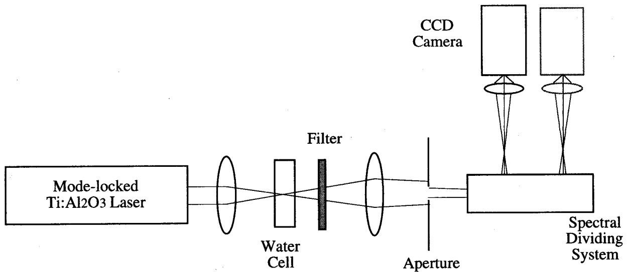
図4.14 ニアフィールド観察光学系
