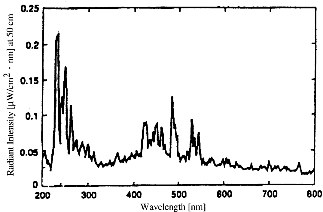
図 2.25 フラッシュランプのスペクトル
