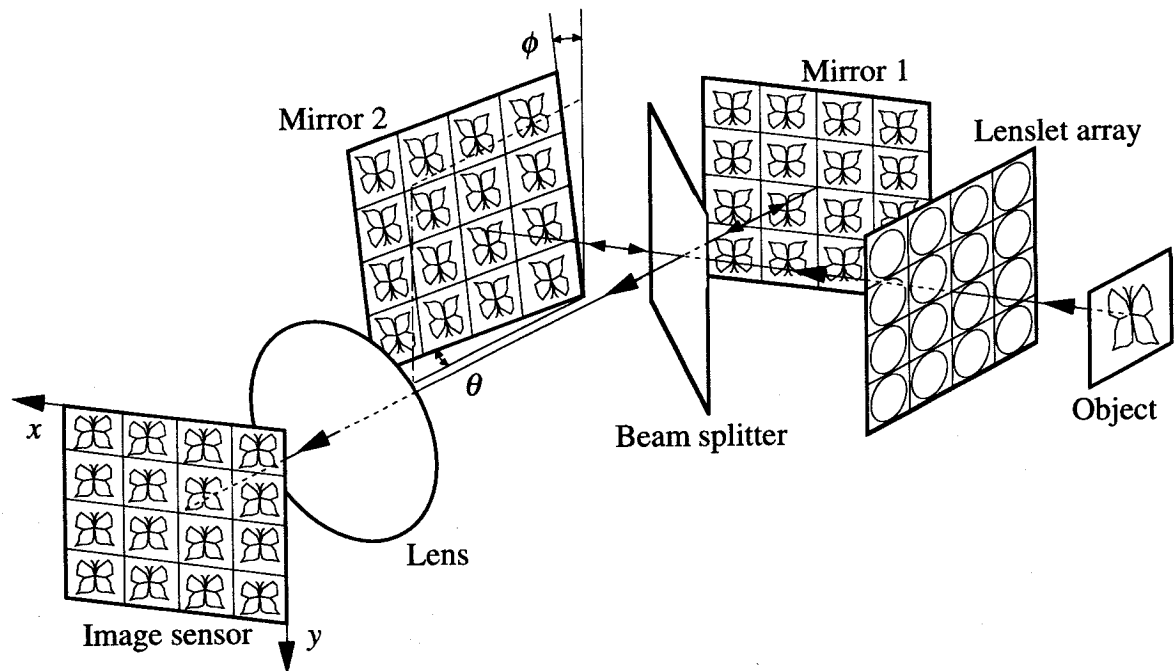
図2.1 多重像フーリエ分光映像法の原理光学系
