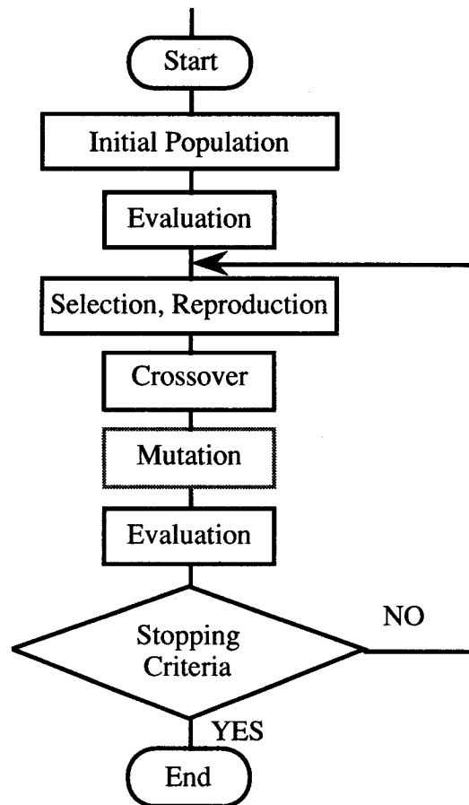
図4.7 遺伝的アルゴリズムの流れ図
