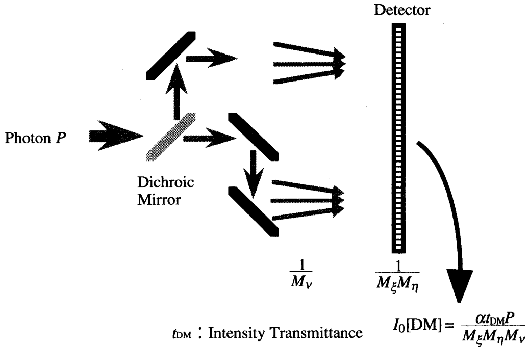
図5.3 ダイクロイックミラー型マルチチャネル分光映像法
