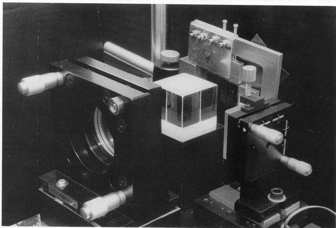
図 2.4 マイケルソン干渉計部分
