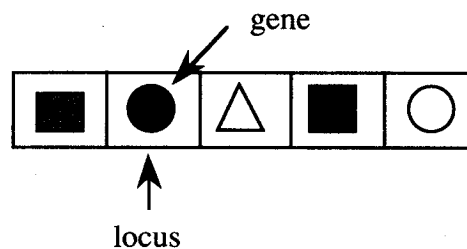
図4.6 染色体
