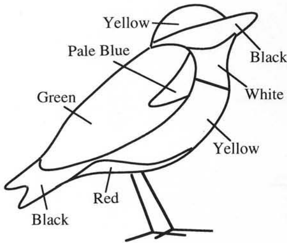
図2.21 多色物体（鳥）
