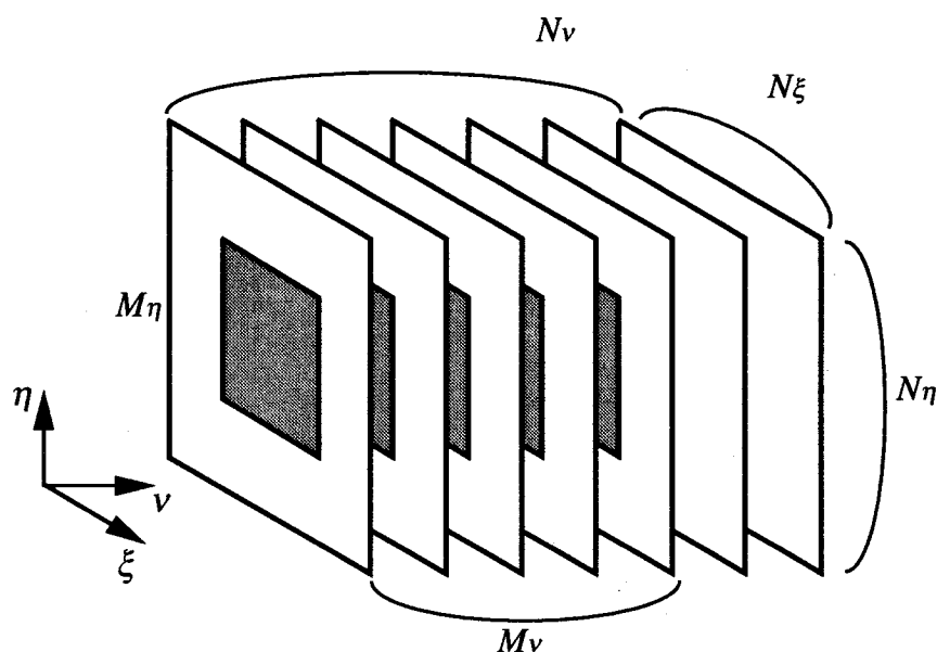
図1.4 測定される分光画像のモデル
