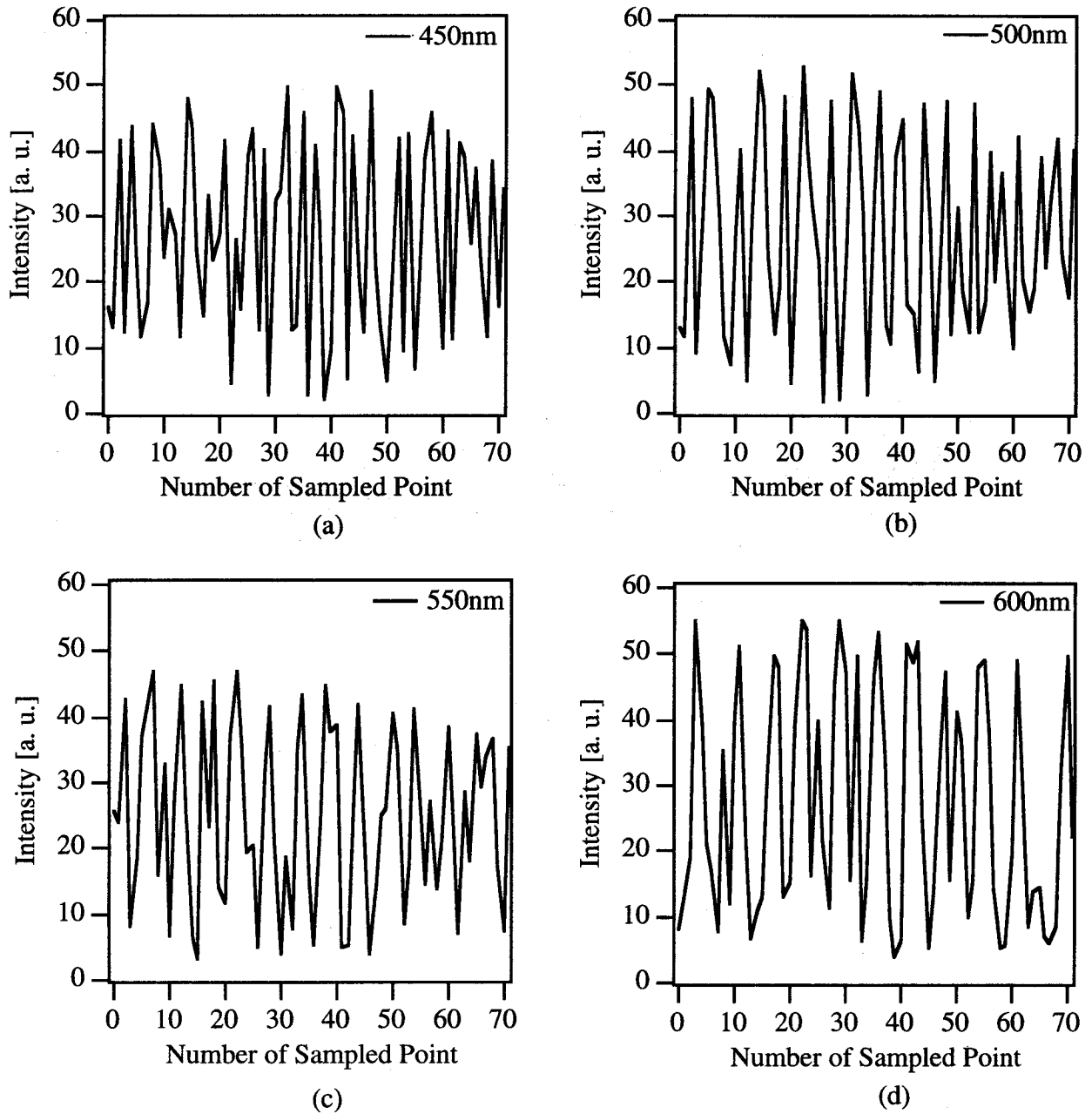
図 2.12 干渉フィルターによる単色一様物体の干渉信号の例：干渉フィルターの中心波長はそれぞれ、(a) 450nm, (b) 500nm, (c) 550nm, (d) 600nm
