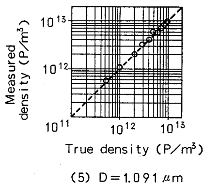
図6. 5 ポリスチレン粒子の粒子密度の測定結果と真の値の比較 (真の値と測定値が一致すると、破線上に測定点(○)が並ぶ。 図中Pは個数を意味する。)
