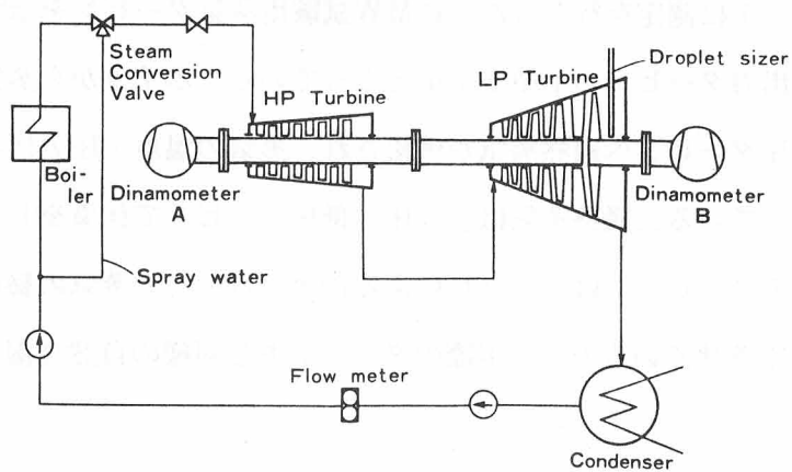
図5. 7 10MW試験用蒸気タービンと測定位置
