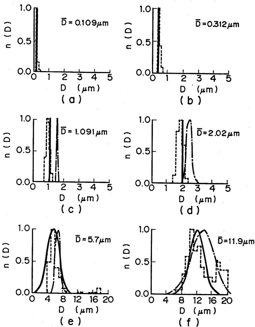
図3. 5 光ファイバを用いた粒径測定装置（実験装置） によるポリスチレン粒子の測定結果
