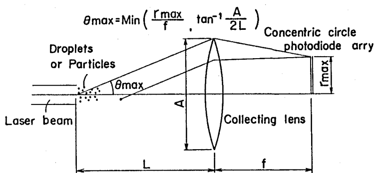
図3. 3 前方微小角散乱法を用いた従来装置の 散乱光強度分布の測定系
