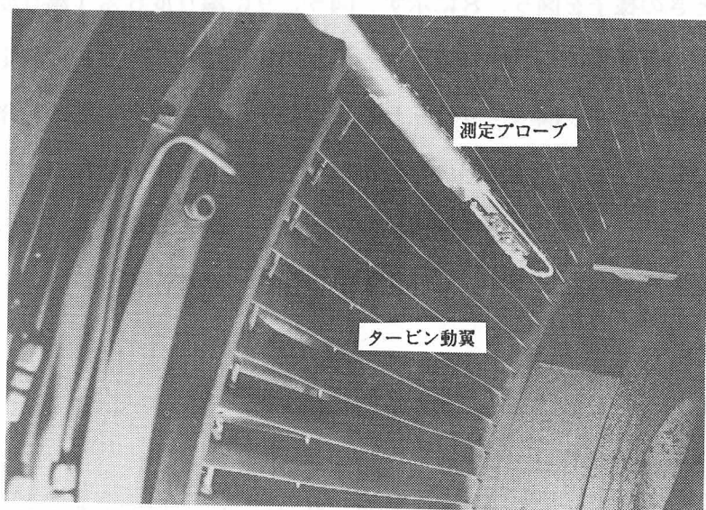
図5. 8 測定プローブをタービン内に挿入したときの様子
