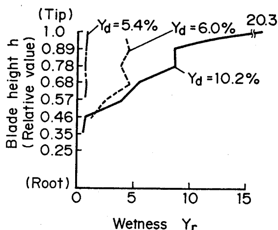
図6.8 試験用蒸気タービン動翼 半径方向の湿り度の分布
