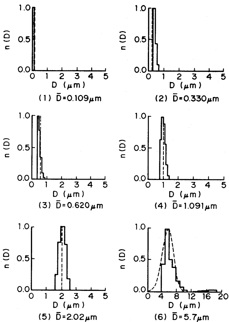
図5.6 試験用蒸気タービン中の水滴を測定するための 粒径測定装置によるポリスチレン粒子の測定結果
