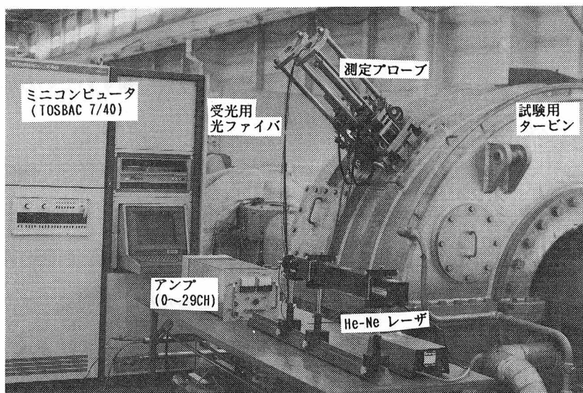
図5. 2 装置全体の写真
