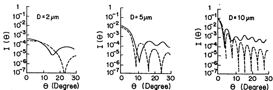
図3. 2 Mie 散乱理論に基づいて計算した i(D, \theta) （実線）とFraunhofer回折理論に基づいて計算した i(D, \theta) （破線）の比較
