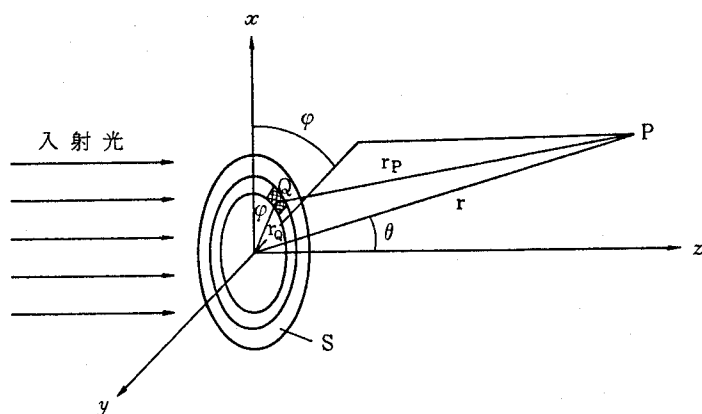
図2.4 Fraunhofer回折理論の考え方
