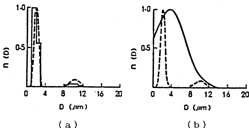
図4. 2 ピークが2つある粒径分布を求める場合の比較
