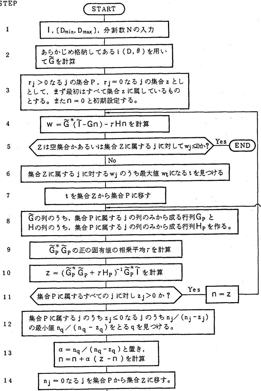
図4. 1 対数束縛積分方程式法を計算機プログラムで実行するときのアルゴリズムの流れ
