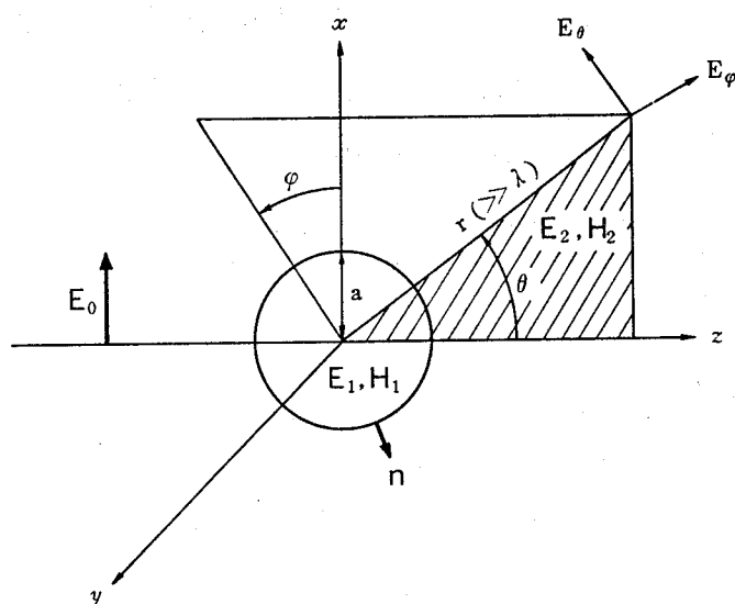
図2.3 Mie 散乱理論により求める光の電場
