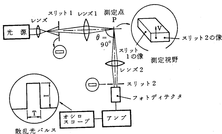
図2. 7 フォトカウント法の測定原理
