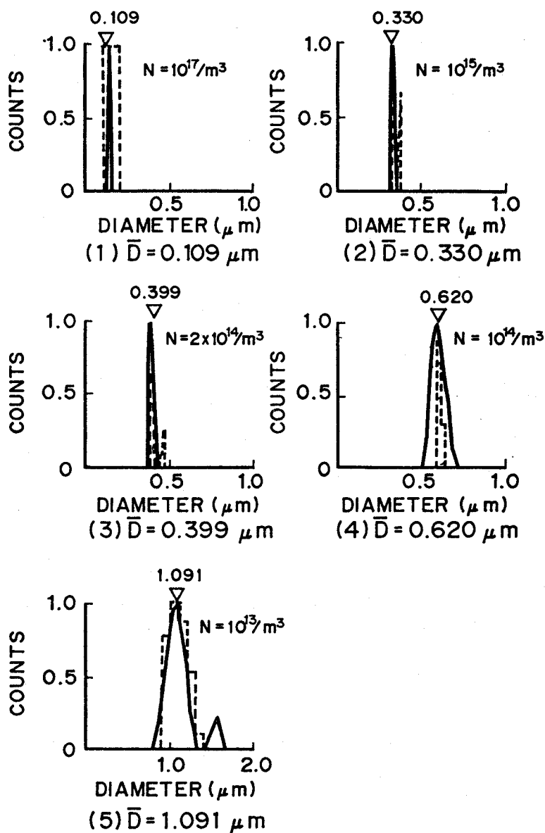
図7. 2 比較的粒子密度が大きい場合のポリスチレン粒子の粒径分布(相対値)を測定した結果
