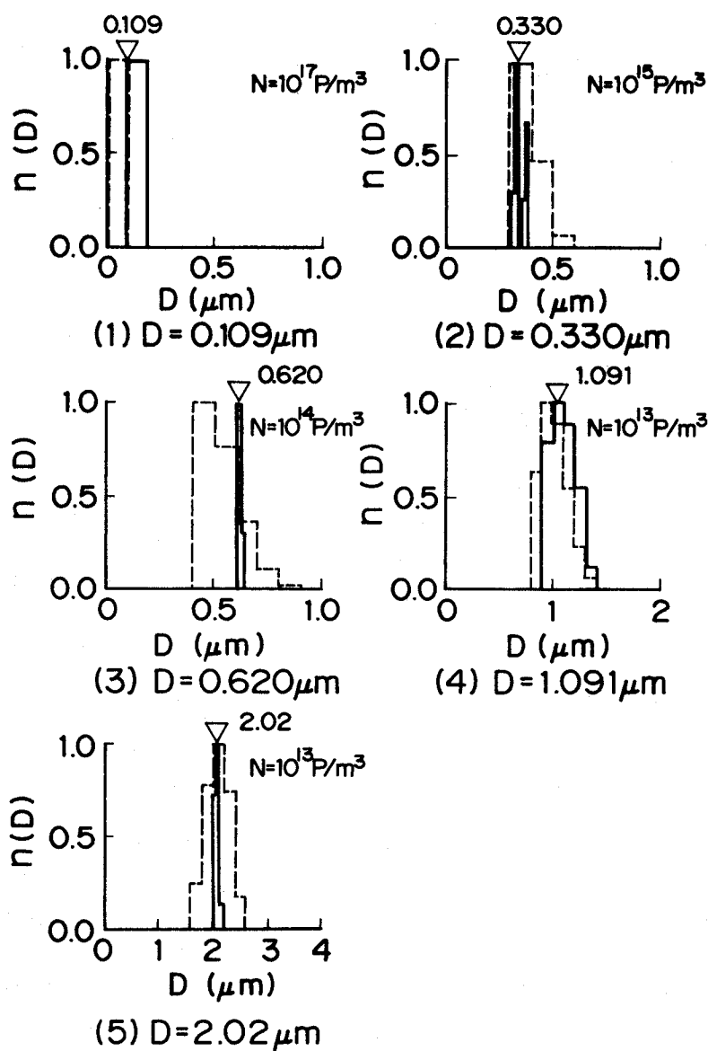
図5.11 \text{Ar}^+ レーザを用いた粒径測定装置によるポリスチレン粒子の測定結果。Pは個を表している。
