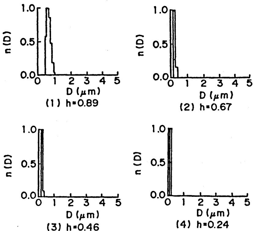
図5. 9 試験用蒸気タービン中の水滴の測定結果 (平均湿り度6%, ここで平均湿り度とは 動力計で測定したタービン出力より求めた 湿り度のことである。)
