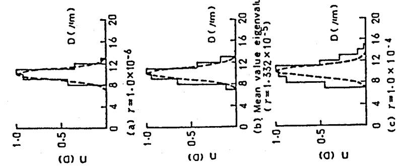
図4.4 \gamma の与え方の妥当性 I 平均 10.0 \mu\text{m} , 標準偏差 1.0 \mu\text{m} , \theta が 0.5 \sim 15^\circ の場合 (----- 仮定した分布) (—— 変換して求めた分布)
