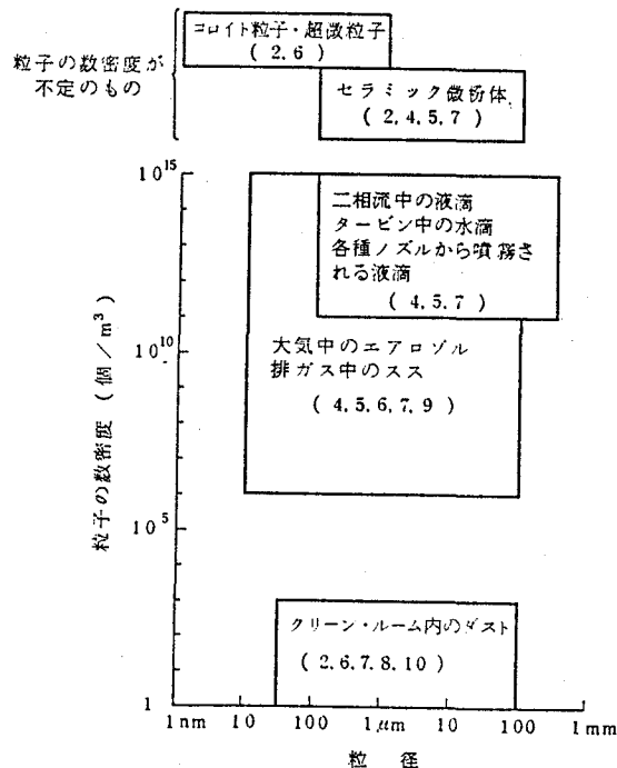
図2. 1 いろいろな微小粒子の大きさ及び粒子密度
