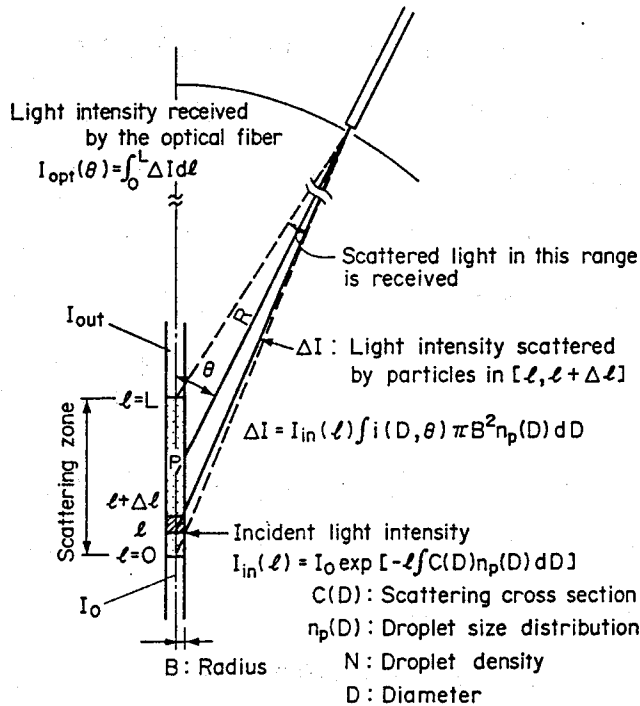
図6. 2 粒子による照射ビームの減衰を考慮した場合の散乱光強度
