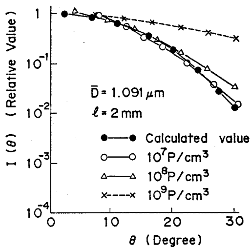
図3. 8 粒子密度が 10^7 \sim 10^9 個/ cm^3 の場合の散乱光強度分布。 10^9 個/ cm^3 になると明らかに多重散乱の影響が現れ、理論値との差が大きくなっている。
