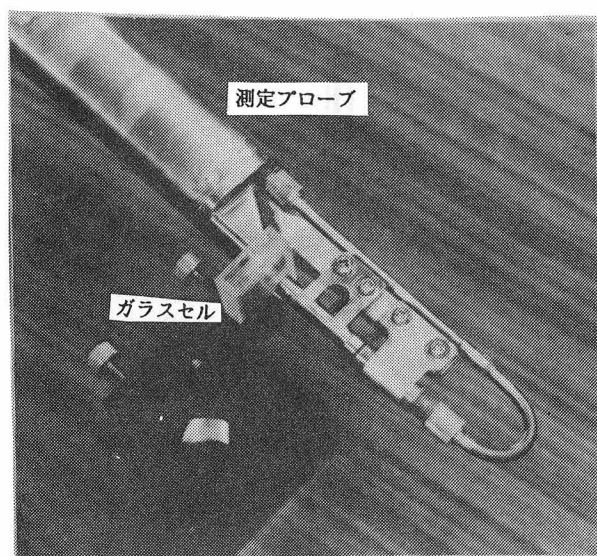
図5. 5 ポリスチレン粒子を測定しているときの様子
