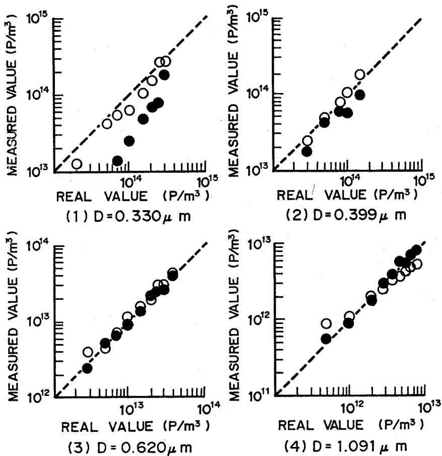
図7. 5 測定した粒子密度より計算した湿り度と真の値の比較
