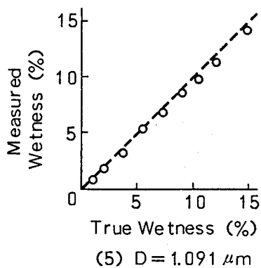
図6. 6 測定した粒子密度から計算した湿り度と真の値の比較 (真の値と測定値が一致すると、破線上に測定点(○)が並ぶ。)
