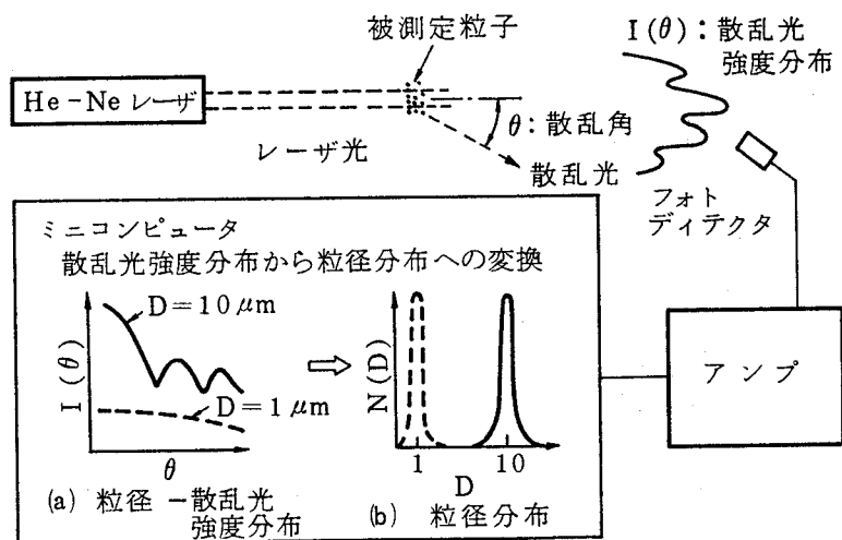
図2. 5 前方微小角散乱法の測定原理
