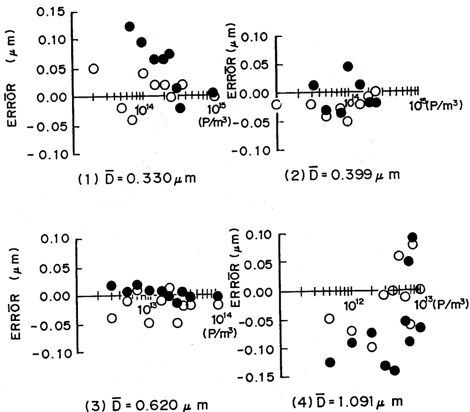
図7. 3 ポリスチレン粒子の粒子密度を変えた場合の平均 粒径の測定誤差
