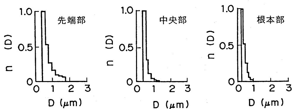
図6.7 試験用蒸気タービン中の水滴の粒径分布 (平均湿り度 Y_d = 10.2\% の場合)
