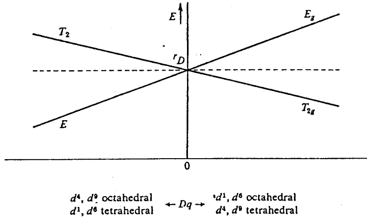
Fig. 1-9 Energy levels of (d)^1 , (d)^4 , (d)^6 and (d)^9 electronic configurations.
