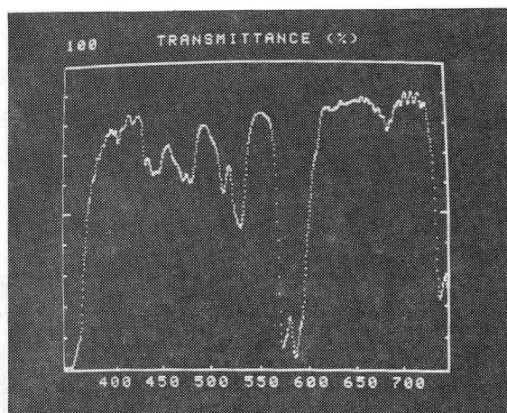
図2.29 ディスプレイ・モジュールに出力した吸収スペクトン
