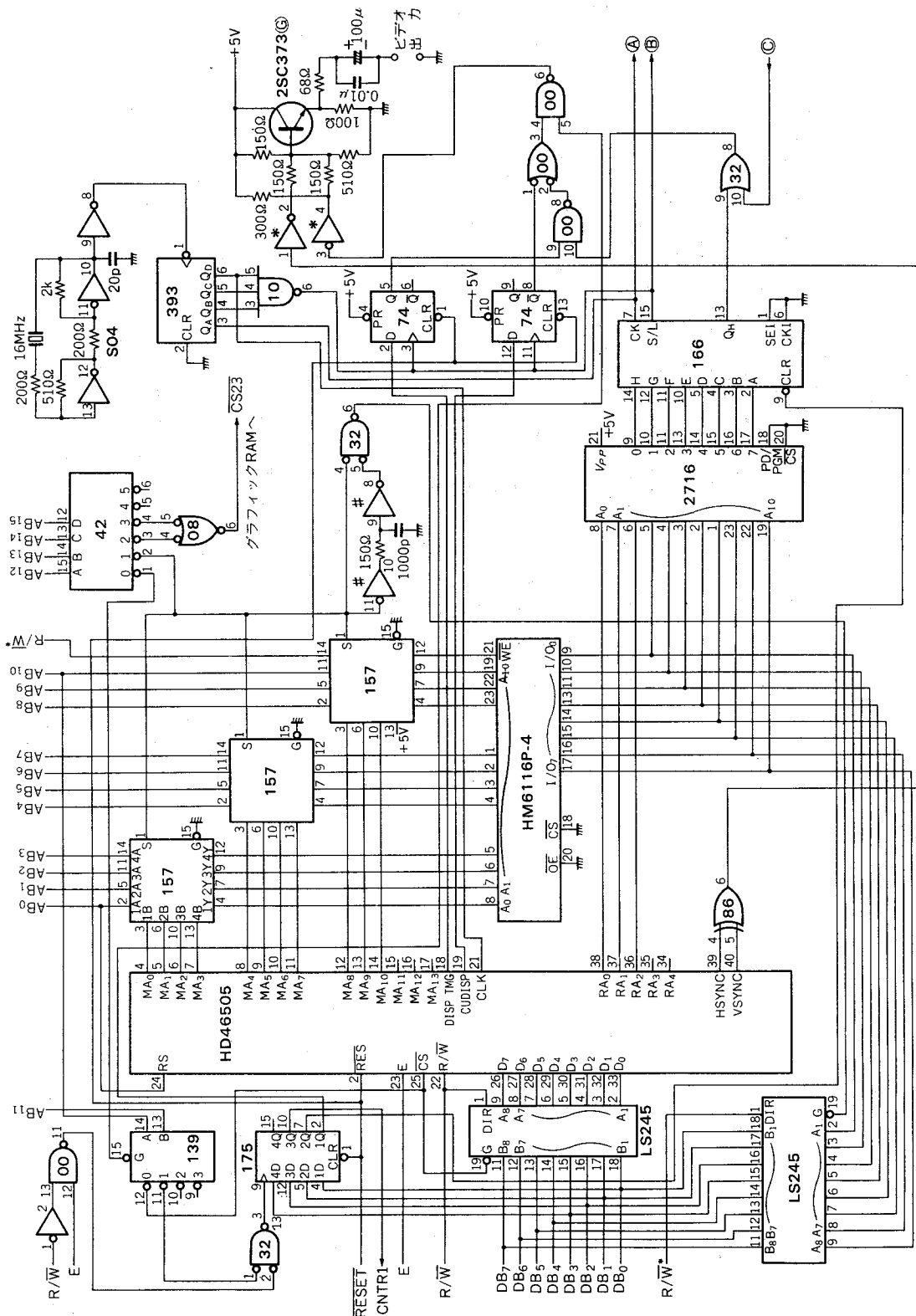
図 5.3 ディスプレイ制御回路 (I)
