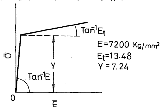
図 4-2 単軸引張りの相当応力 \sigma -対数ひずみ \bar{\epsilon} 関係
