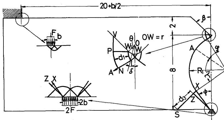
図Ⅱ-1 切欠き試験片形状と深い切欠きのすべり線場
