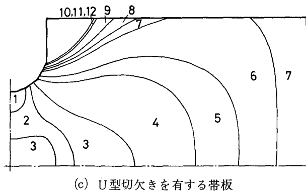
図4-16 弾塑性境界の進展状態
