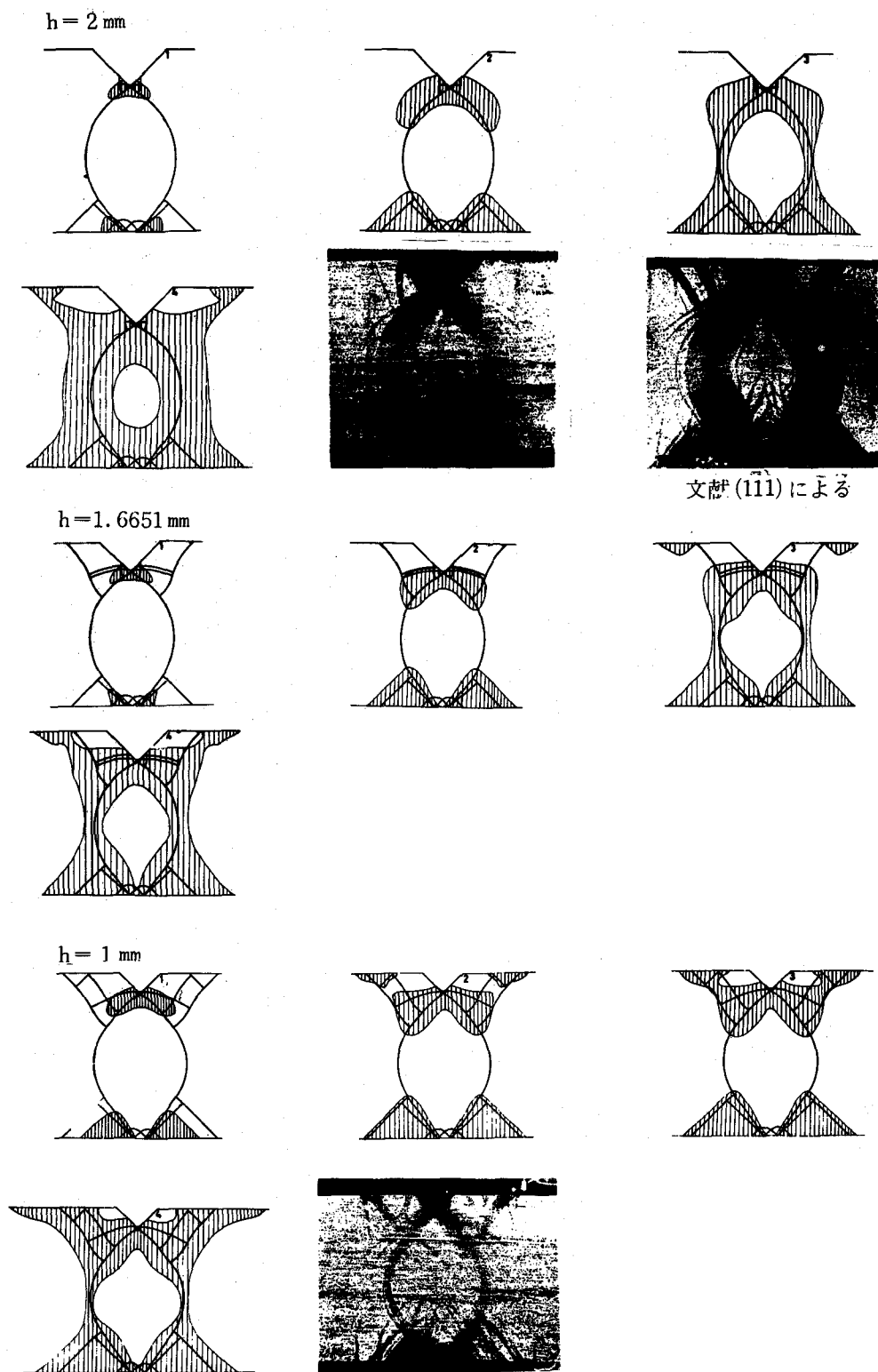
図Ⅱ-7 塑性域の進展状態
