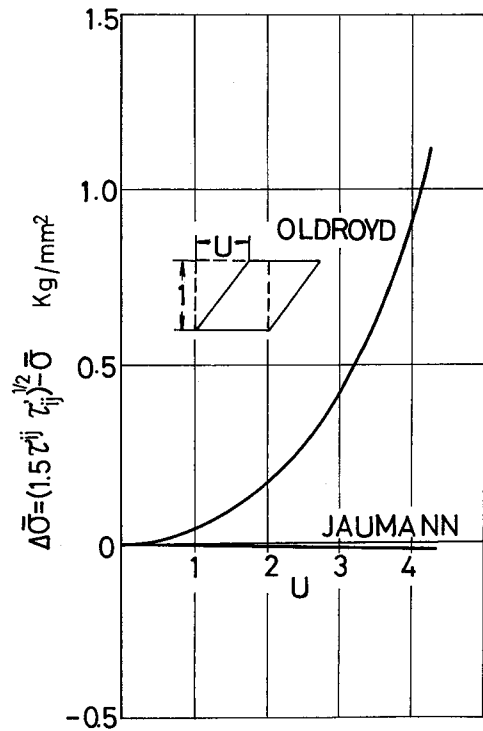
図4-3 相当応力の誤差
