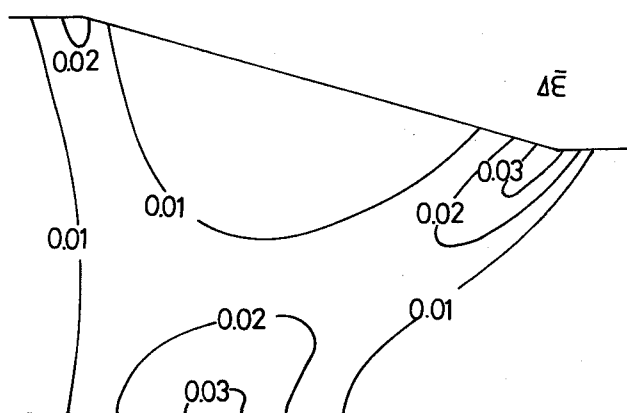
図 5-14 相当ひずみ増分の分布
