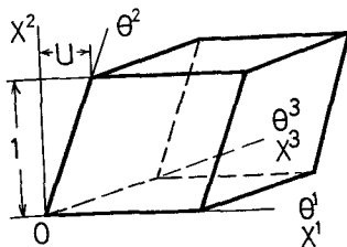
図 4-1 単純せん断変形
