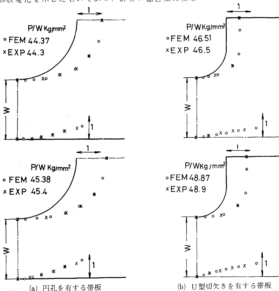
図4-20 円孔および切欠きに沿う軸方向の変位 U^2 の分布, (U^2/W) \times 10 FEMは厳密法, EXPは実験による結果を示す
