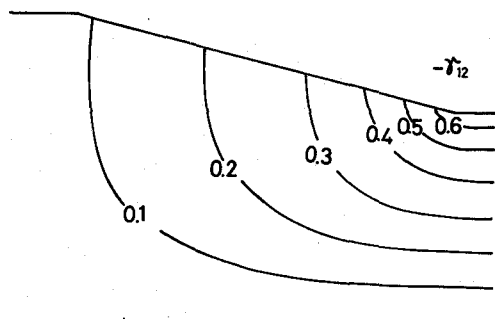
図 5-16 Green のひずみ分布
