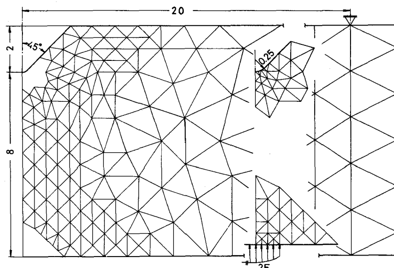
図Ⅱ－５ 要素分割
