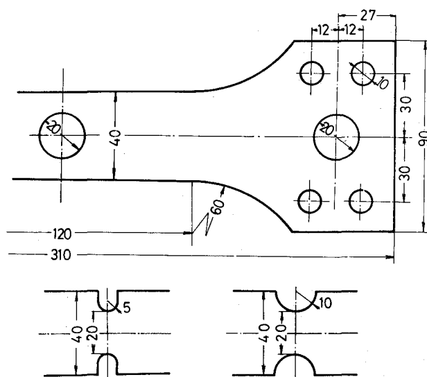
図5-7 試験片
