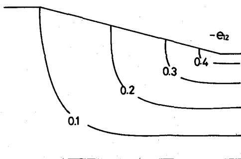
図 5-17 Almansi のひずみ分布
