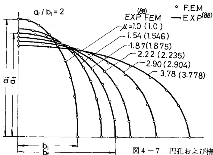
(b) 楕円孔
