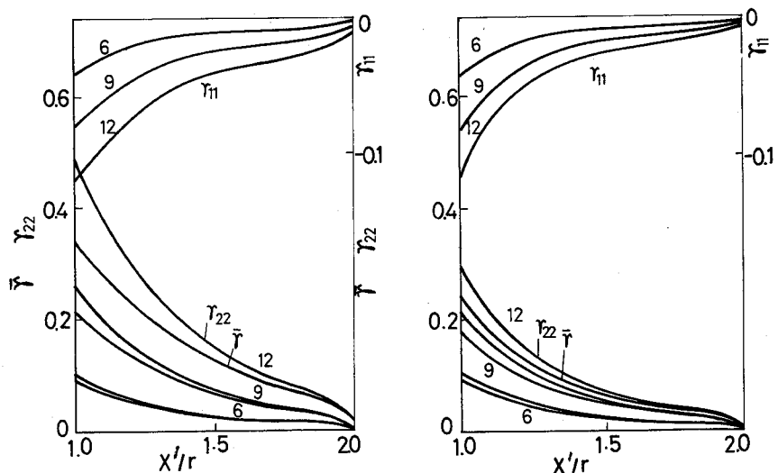
(a-1) 厳密法 円孔を有する帯板
