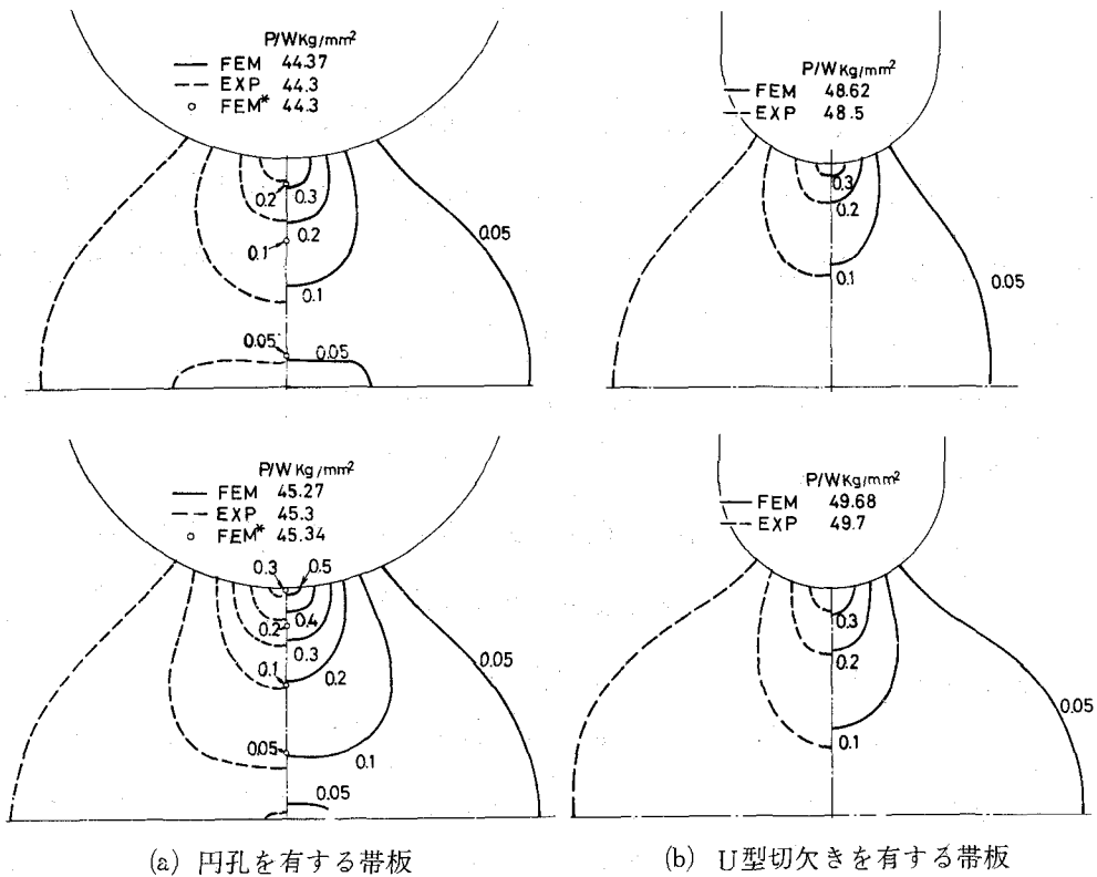
図4-22 最小断面付近の Green のひずみ分布 FEM は厳密法, FEM* は従来法, EXP は実験による結果を示す
