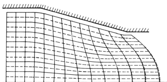
図5-13 流線 ——物体点の軌跡 -----モアレじまから求めた流線
