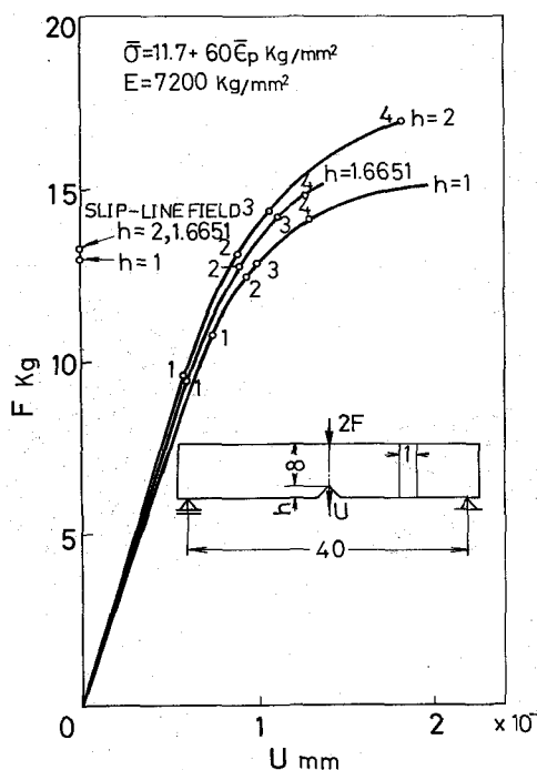
図Ⅱ-6 荷重変位関係
