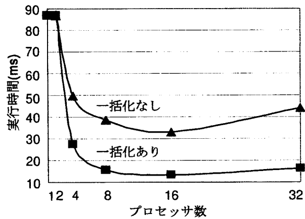
図 3.7: 通信の一括化の効果 (問題サイズ 128 のヤコビ法を AP1000 で解く場合)
