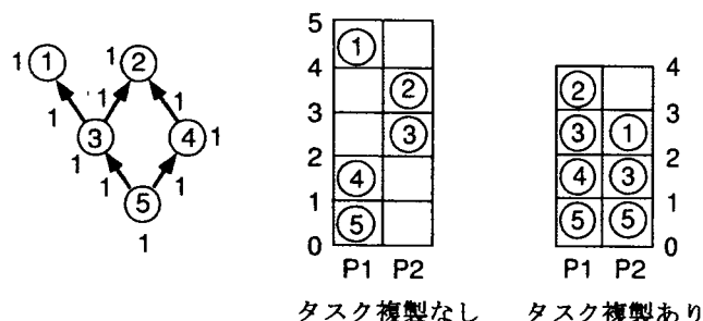
図 2.4: タスク複製の例 [4]
