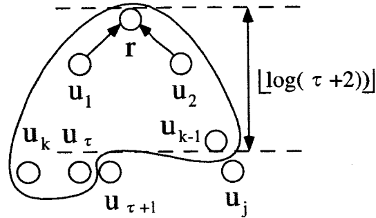
図 4.12: r, u_\tau, u_{\tau+1} の関係
