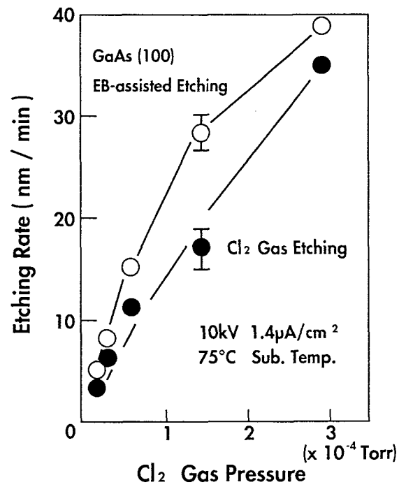
図 2 - 5 塩素ガスおよび電子ビーム励起ドライエッチング速度の塩素圧依存
