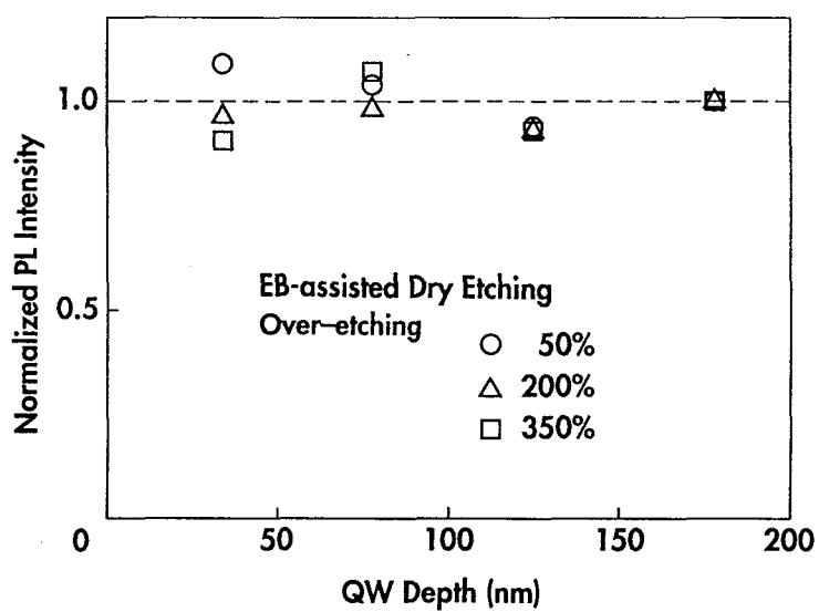
図 5 - 2 2 オーバーエッチングを行った試料の規格化発光強度
