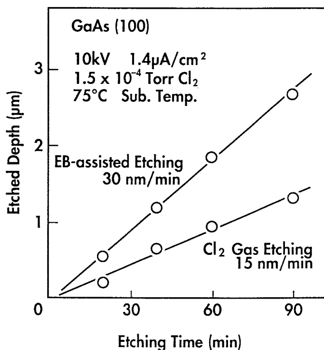
図 2 - 3 塩素ガスエッチングおよび電子ビーム励起ドライエッチング結果
