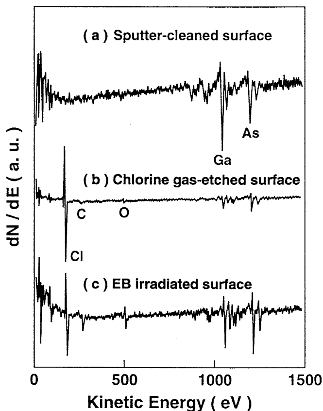
図 4 - 2 GaAs試料のその場 AES 測定結果
