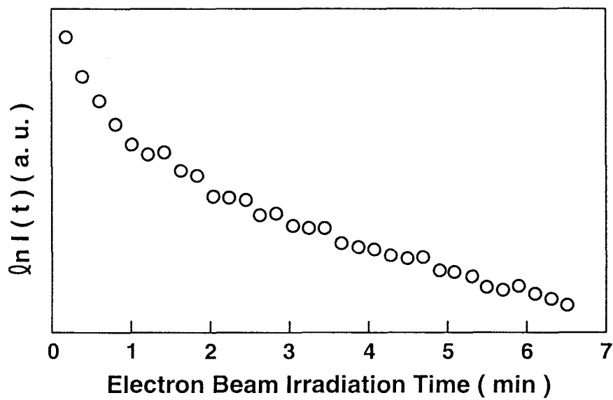
図 4 - 6 吸着塩素脱離特性の対数プロット
