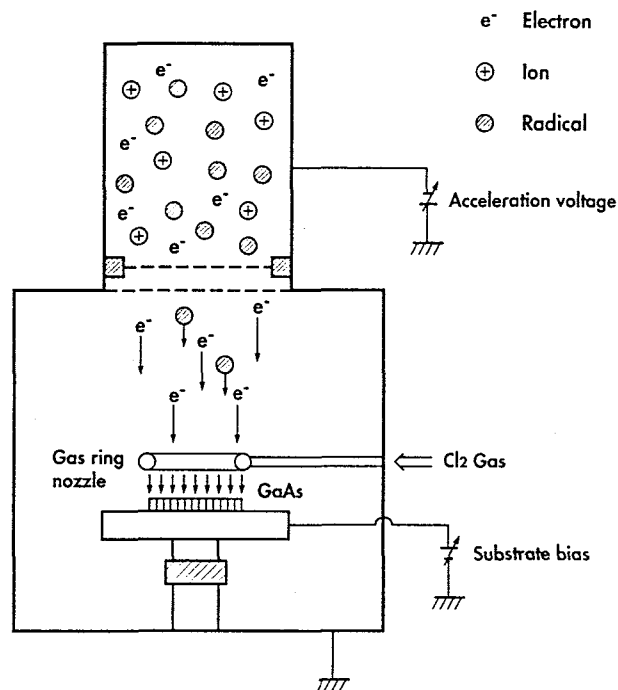
図5-1 ECRプラズマを電子線源としたエッチング法の概念
