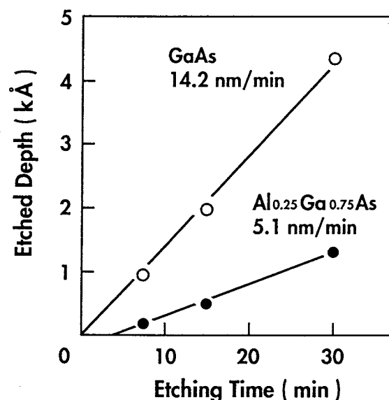
図 5 - 1 4 GaAsおよびAlGaAsの電子ビーム励起ドライエッチング
