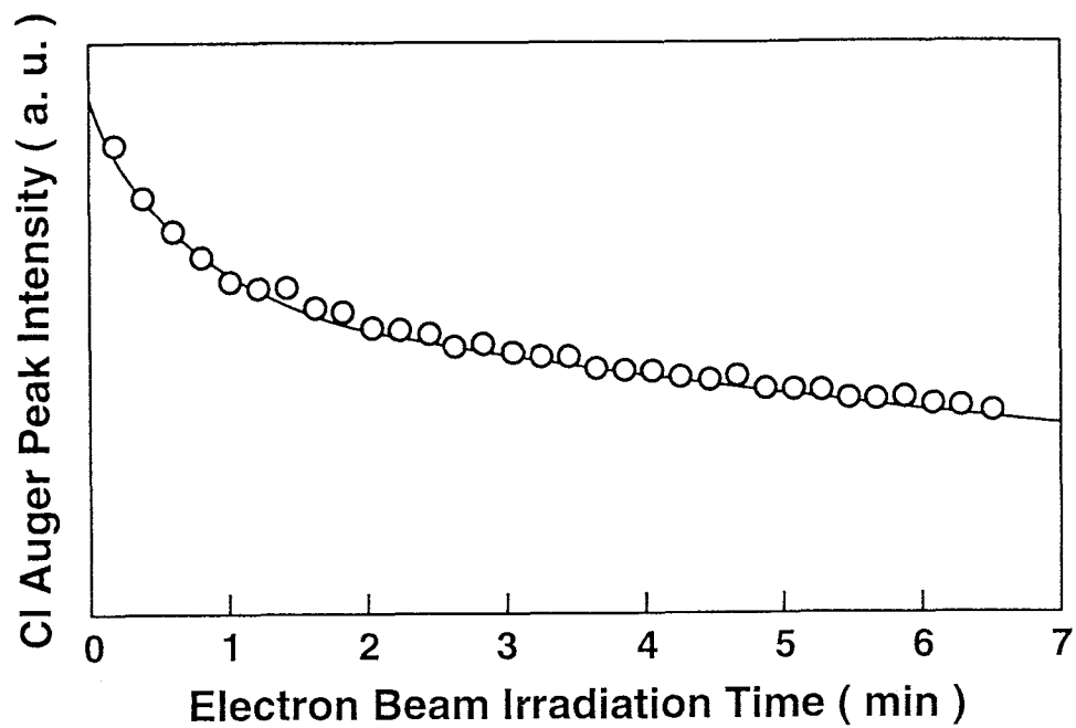
図 4 - 5 塩素吸着GaAs表面からの電子衝撃脱離過程のAES測定結果
