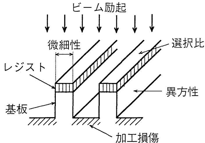
図 1 - 1 微細構造形成におけるエッチング技術への要求
