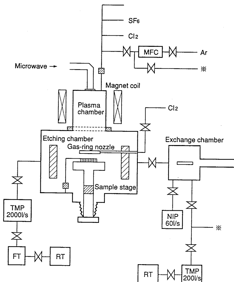
図 5 - 2 ECR電子ビーム励起ドライエッチング装置の構成
