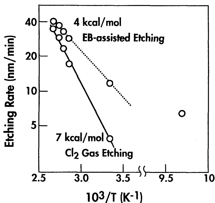
図 3 - 6 エッチング速度の基板温度依存性のアレニウスプロット
