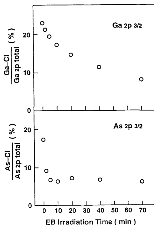
図 4 - 8 電子衝撃脱離に伴うXPSスペクトル中のケミカルシフト成分の変化
