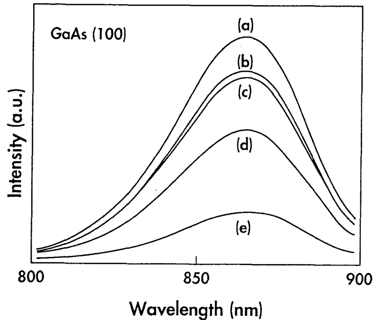
図 2 - 9 GaAs基板および各種エッチング試料のPL測定結果 (a)GaAs基板, (b)塩素ガスエッチング, (c)電子ビーム励起ドライエッチング, (d)Cl-RIBE, (e)Ar-IBE
