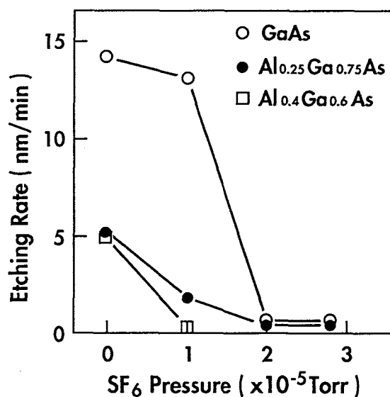
図 5 - 1 5 フッ素ラジカルによるGaAs/AlGaAs選択エッチング結果
