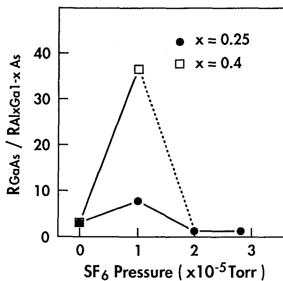
図 5 - 1 6 GaAs/AlGaAs選択比のSF 6 ガス圧依存性
