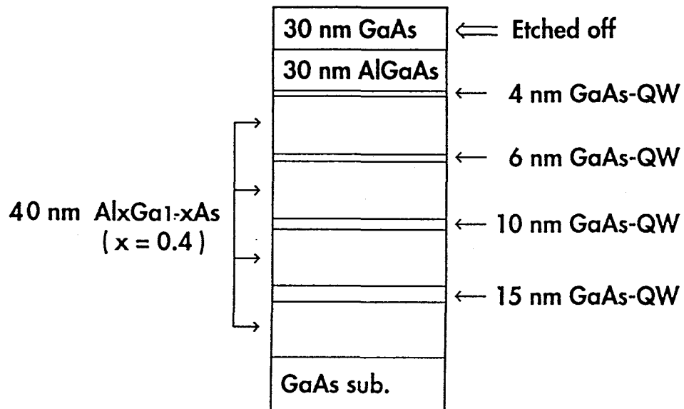
図 5 - 1 7 光学的損傷評価に用いた量子井戸試料の構造
