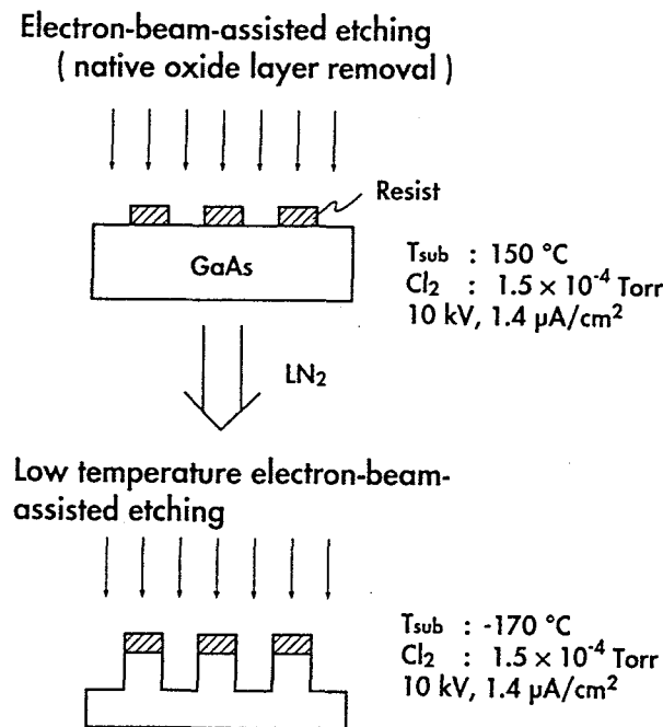
図3-1 低温電子ビーム励起ドライエッチングのプロセス
