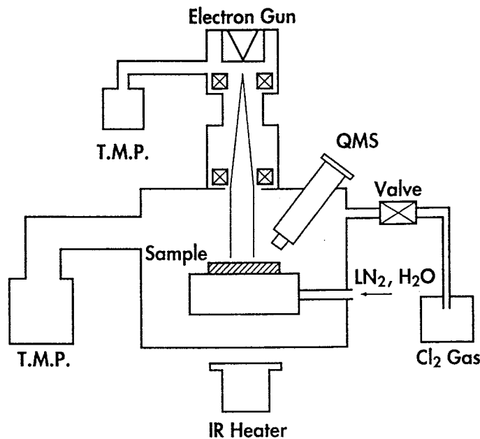
図 2 - 2 RHEED用電子銃を備えた電子ビーム励起ドライエッチング装置
