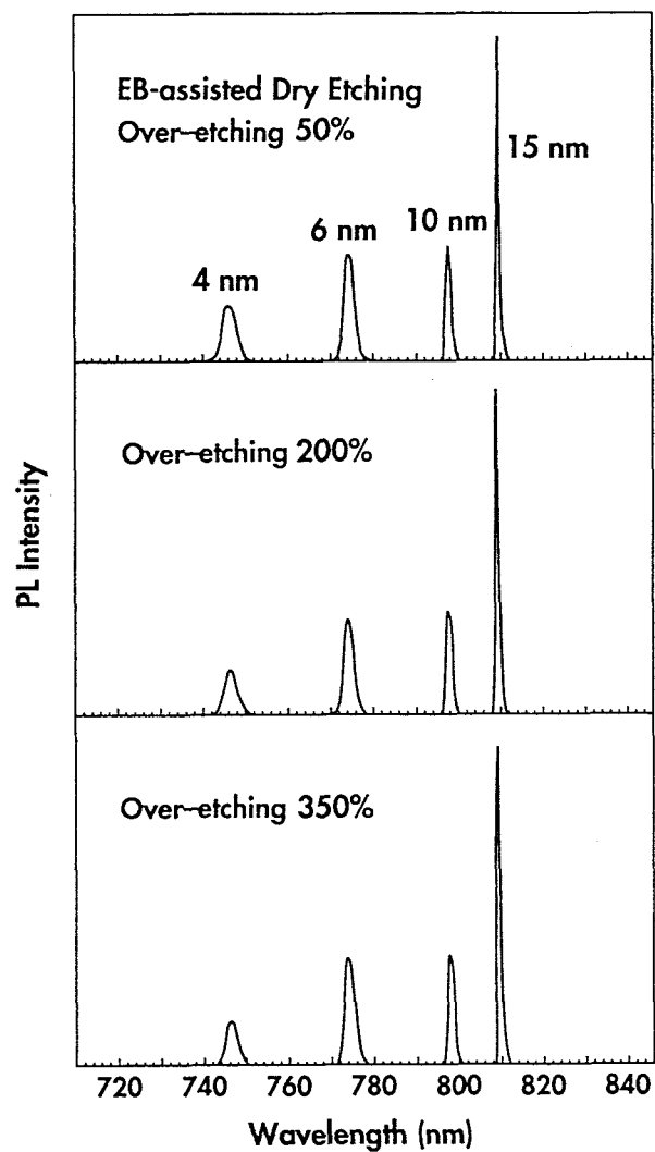
図 5 - 2 1 オーバーエッチングを行った試料からの PL測定結果
