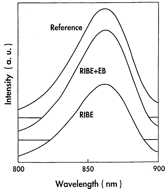
図 5 - 5 GaAs基板および各種エッチング試料のPL測定結果
