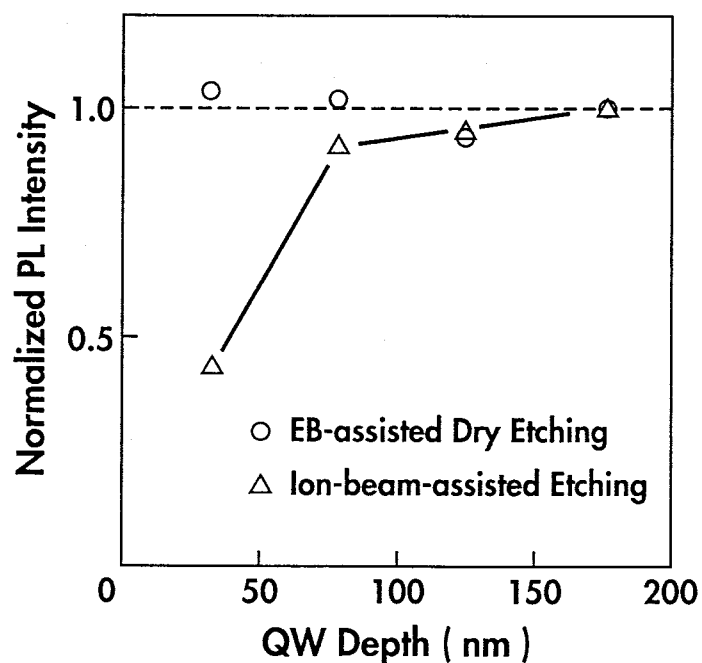
図 5 - 2 0 エッチング試料の規格化発光強度の量子井戸深さ依存性
