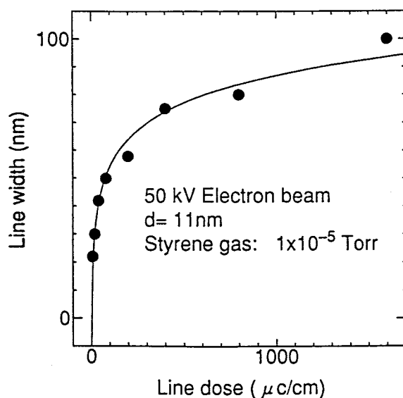
図5-10 カーボン堆積層の線幅とラインドーズの関係
