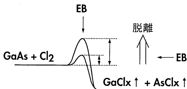
図 3 - 5 エッチングの反応機構の模式図
