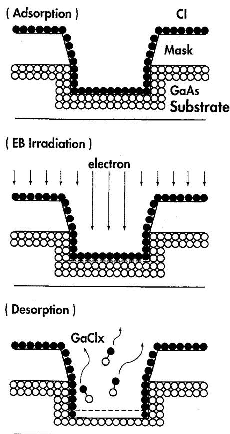
図 2-1 電子ビーム励起ドライエッチングの概念
