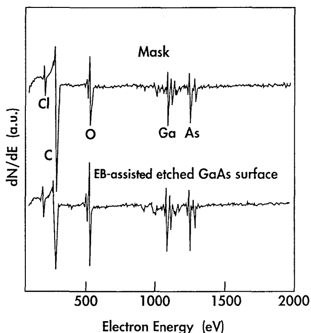
図 2 - 1 6 反転エッチング試料のAES測定結果
