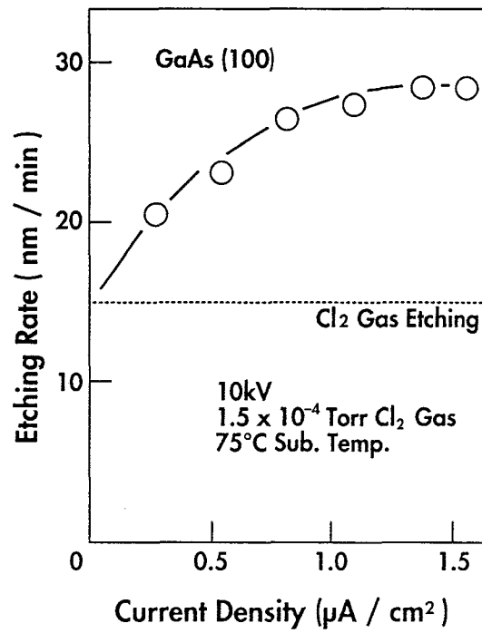
図 2 - 4 電子ビーム励起ドライエッチング速度の電流密度依存
