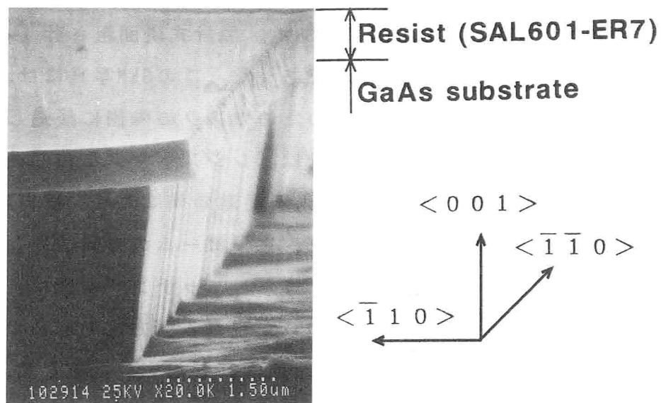
図 2 - 6 レジストマスク付き(100)GaAsエッチングパターンの断面観察結果
