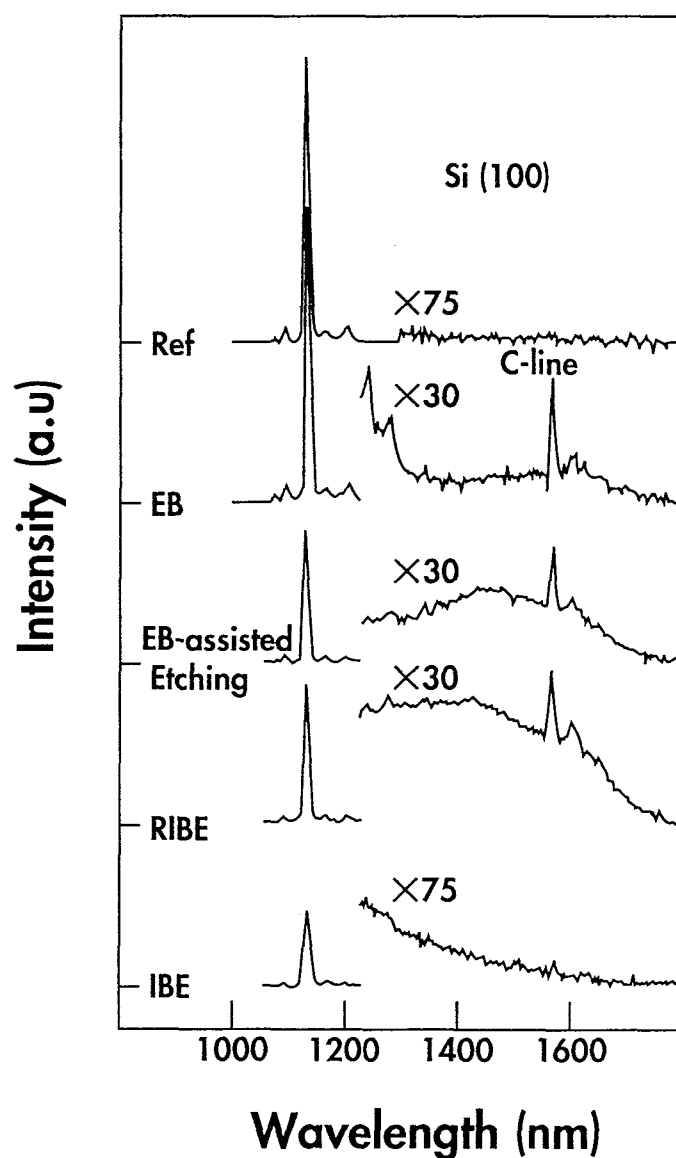
図 2 - 1 1 Si基板および各種エッチング試料の極低温PL測定結果
