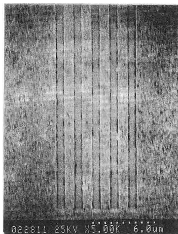
図 2 - 1 5 微細反転パターン転写結果
