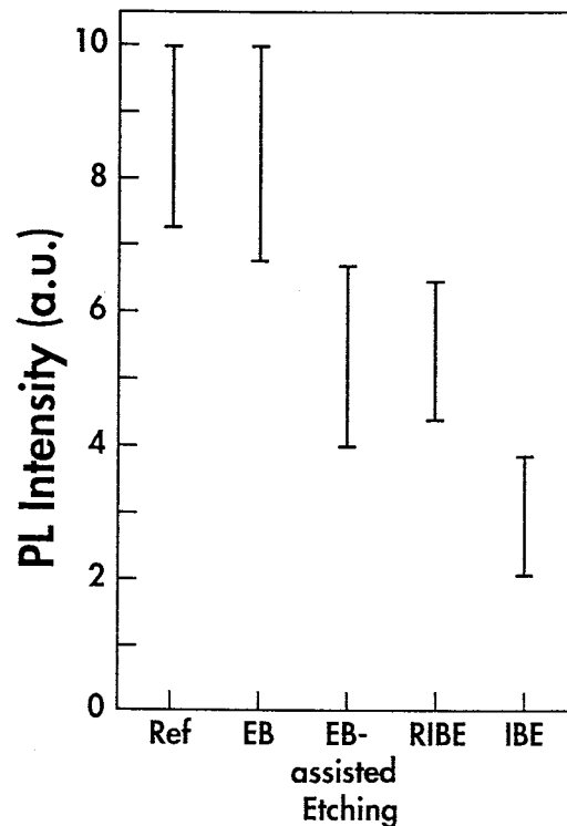
図 2 - 1 2 Si基板および各種エッチング試料のバンド端発光強度
