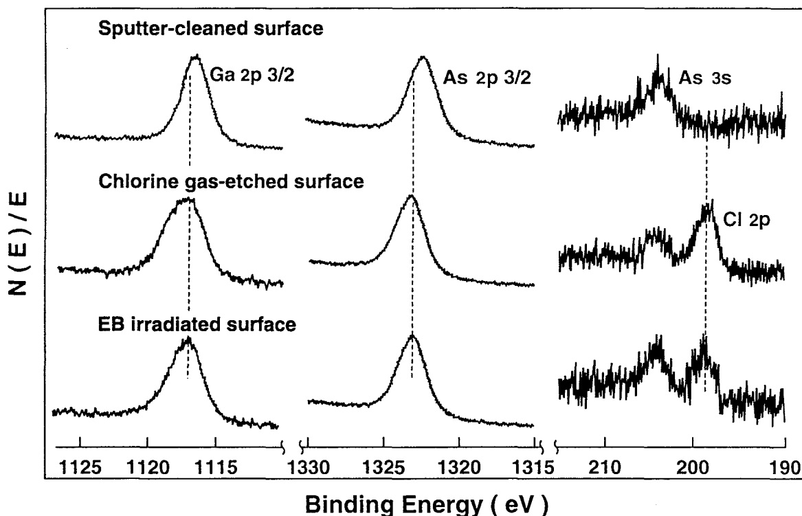
図 4 - 3 GaAs試料のその場 XPS 測定結果
