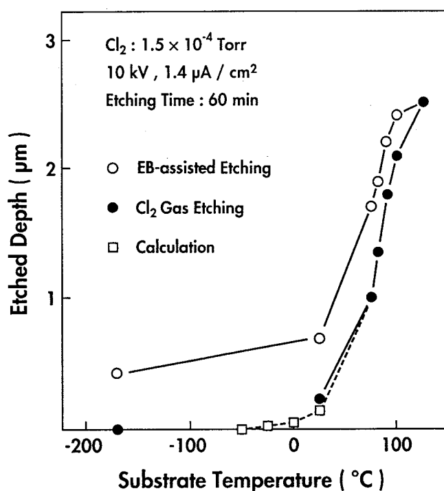
図 3 - 2 エッチング速度の基板温度依存性
