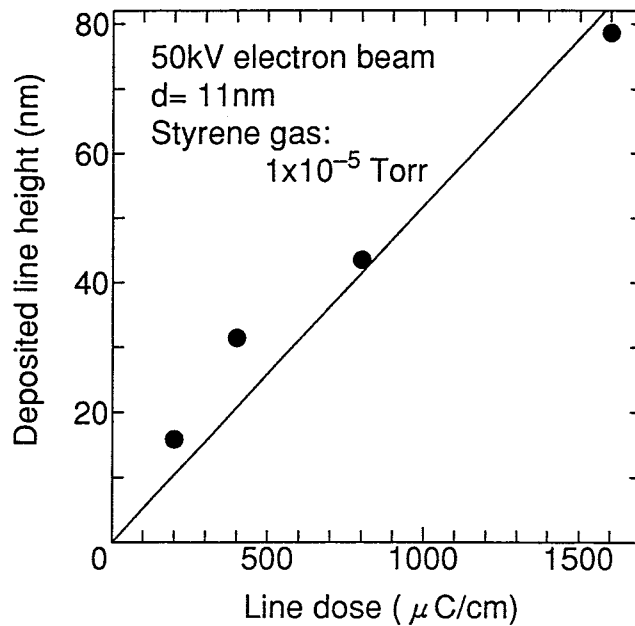
図 5 - 1 1 カーボン堆積層の厚さとラインドーズの関係
