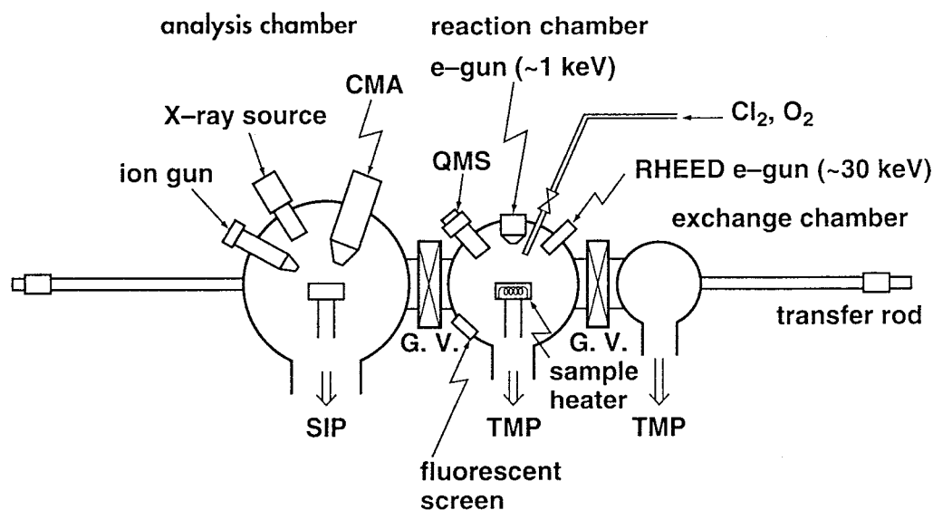
図4-1 ビーム励起表面反応評価装置の構成
