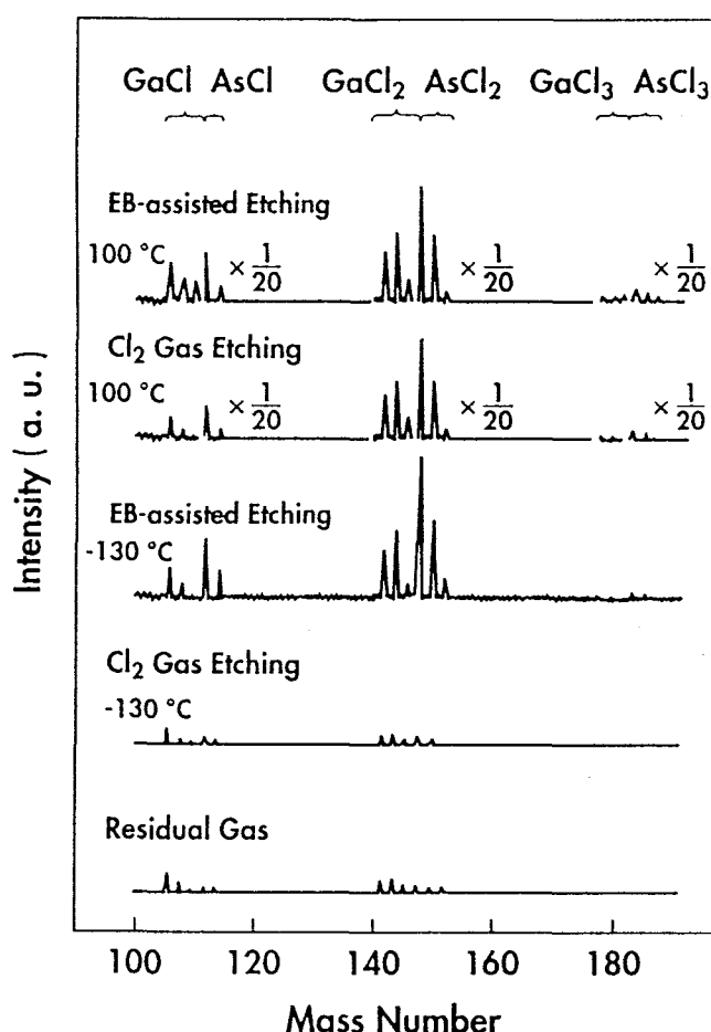
図 3 - 4 エッチング中の反応生成物の質量分析結果
