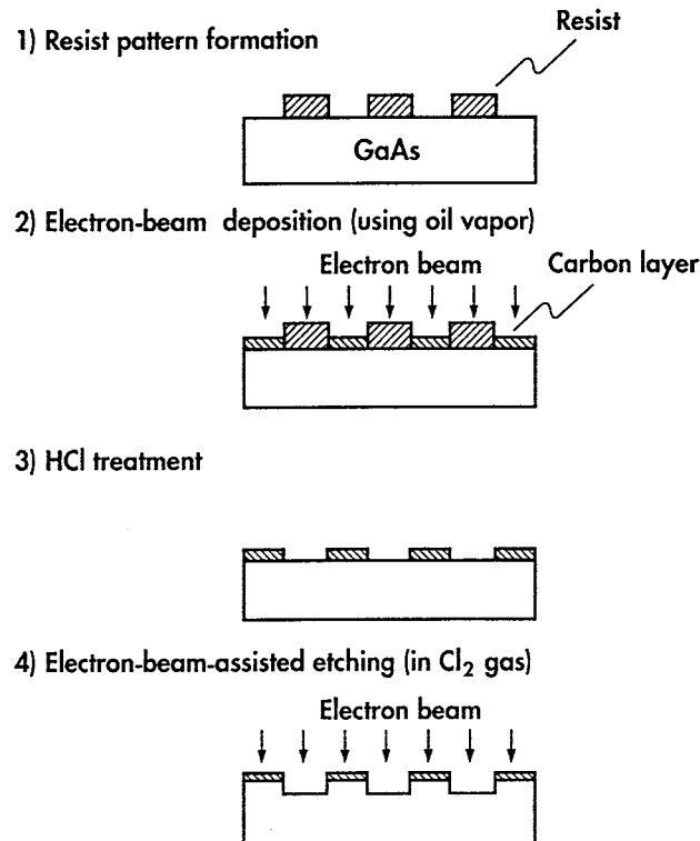
図 2 - 1 3 カーボン堆積層をマスクとした反転エッチングのプロセス
