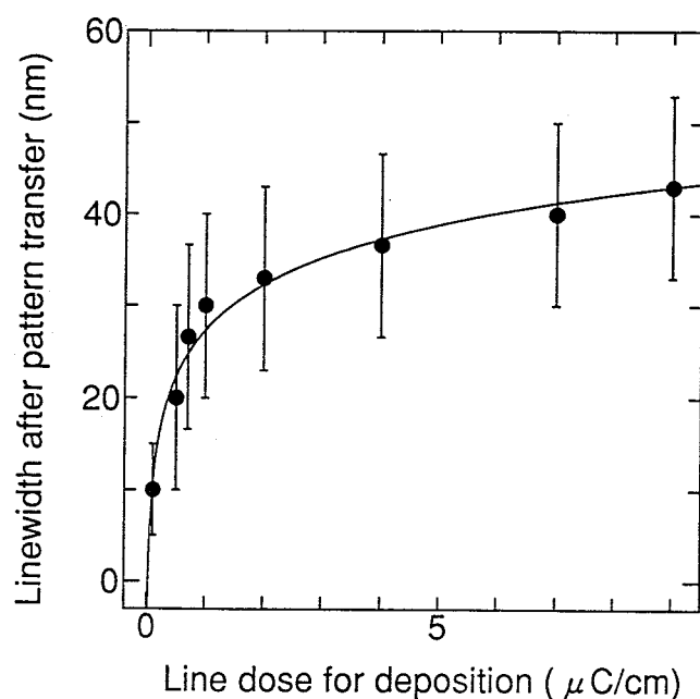
図 5 - 1 3 エッチングパターン線幅のラインドーズ依存性
