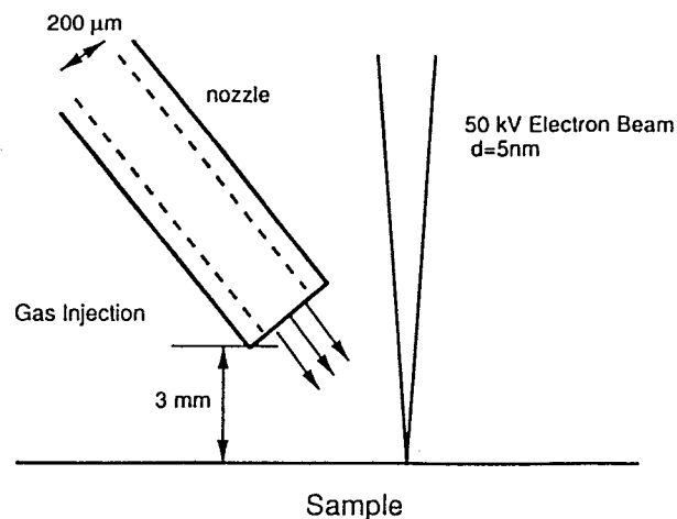
図 5-8 原料ガス導入系の構成
