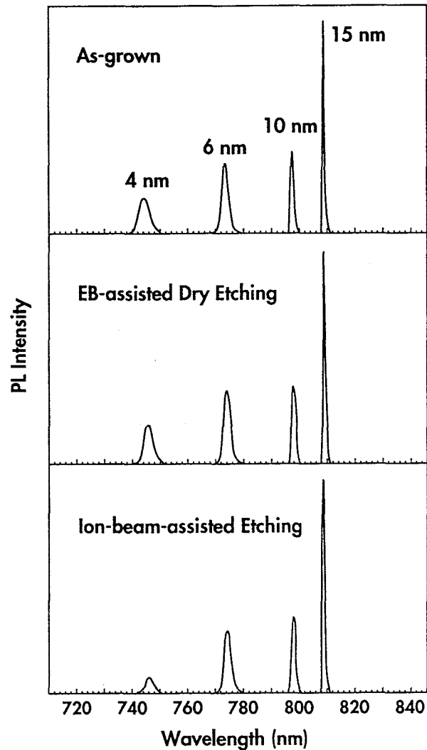
図 5 - 1 9 量子井戸試料のPL測定結果
