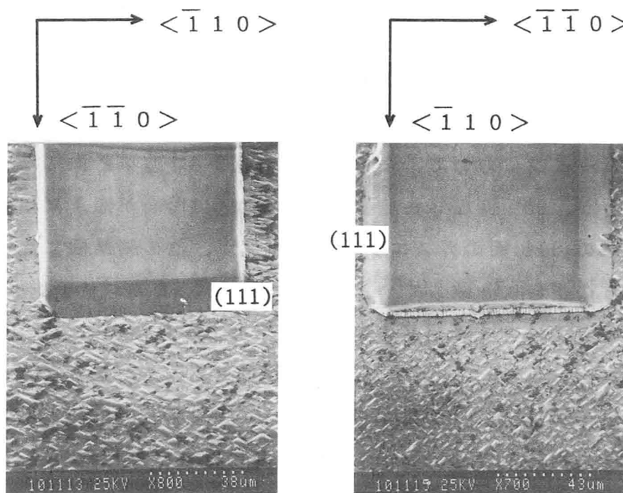
図 2 - 7 (100)GaAsエッチングパターンの観察結果
