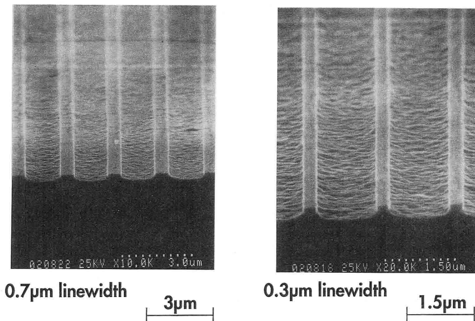
図 2-8 電子ビーム励起ドライエッチングによるGaAs微細パターン転写結果 (ラインパターン方向は \langle 011 \rangle に沿っている)
