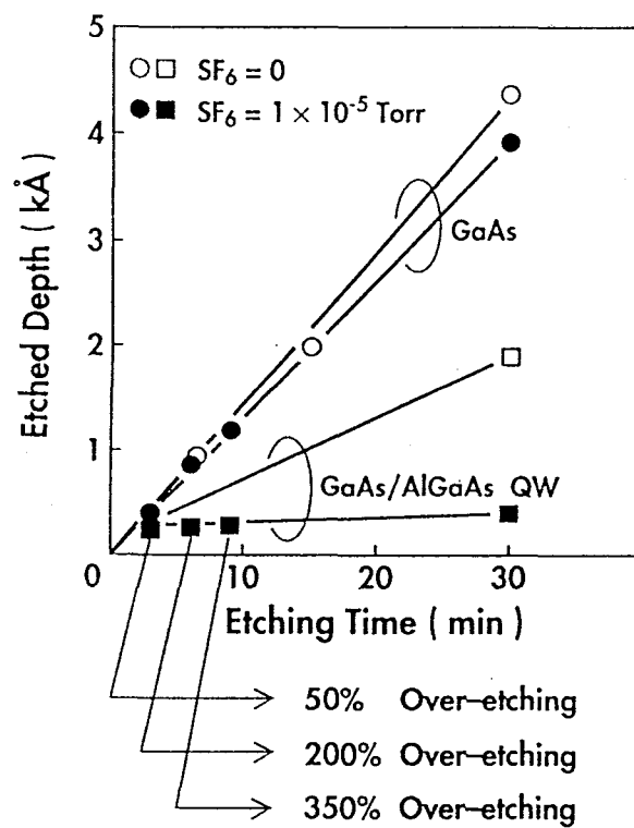
図 5 - 1 8 GaAs/AlGaAs積層構造試料の選択エッチング
