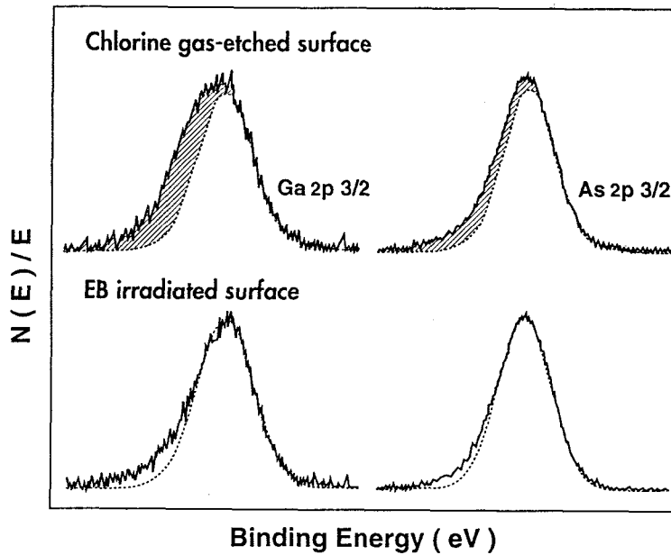
図 4 - 4 塩素吸着に伴う Ga および As スペクトルのケミカルシフト
