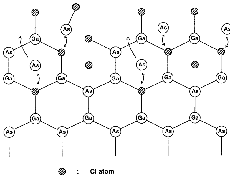
図 4 - 1 0 塩素吸着GaAs表面の反応モデル
