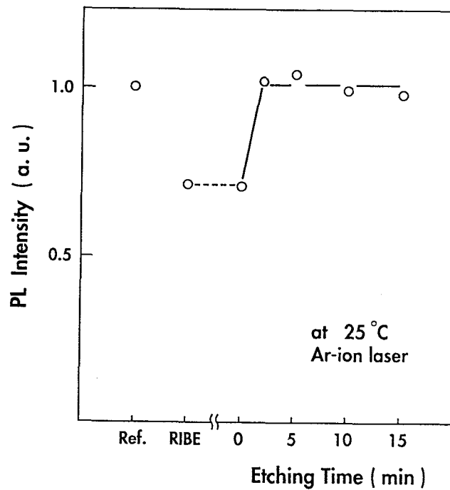
図 5 - 6 損傷層除去に伴う PL 強度の回復
