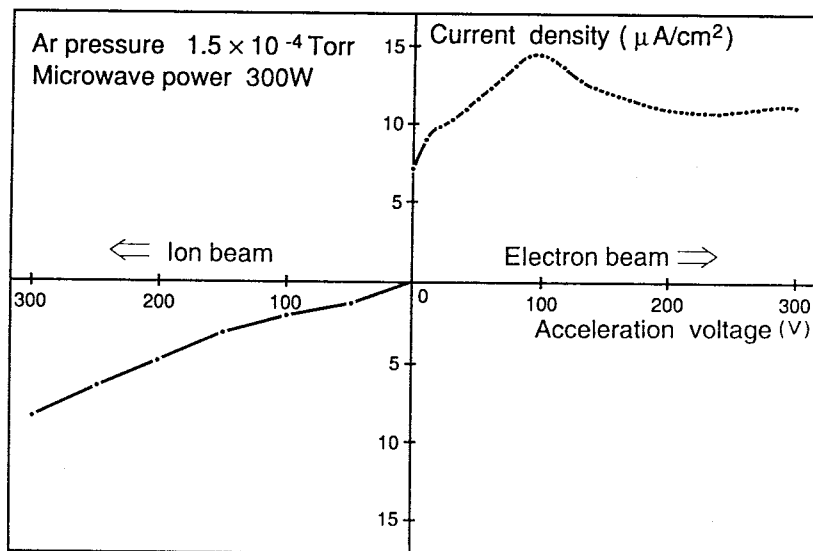
図 5 - 3 アルゴン ECR プラズマからの電子・イオンビーム引き出し特性
