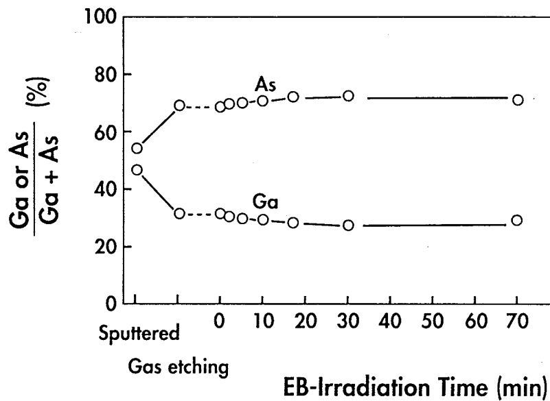
図 4 - 9 電子線照射に伴う Ga/As 組成の変化
