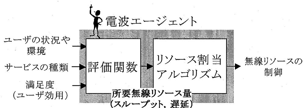
図 2.1: ユーザセントリック無線リソースマネジメントの概念
