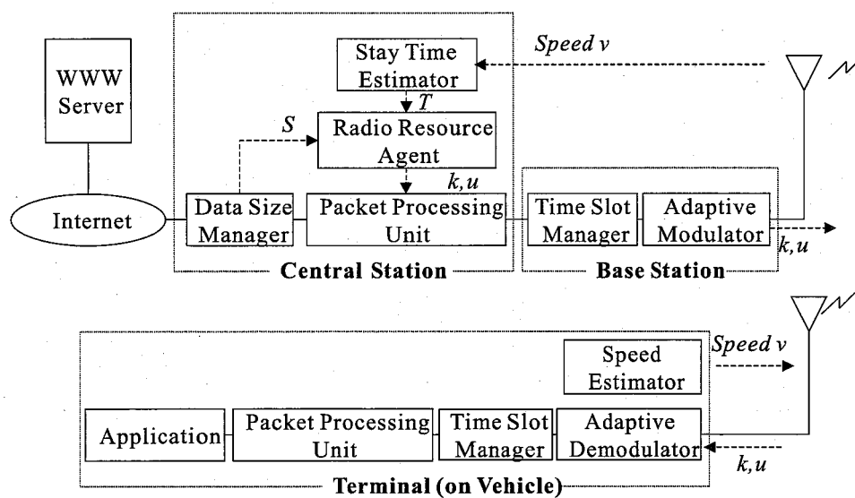
図 3.2: システム構成図
