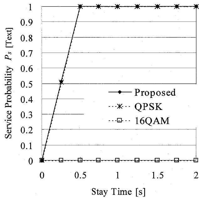
(b) 平均受信 CNR = 15[dB] の場合
