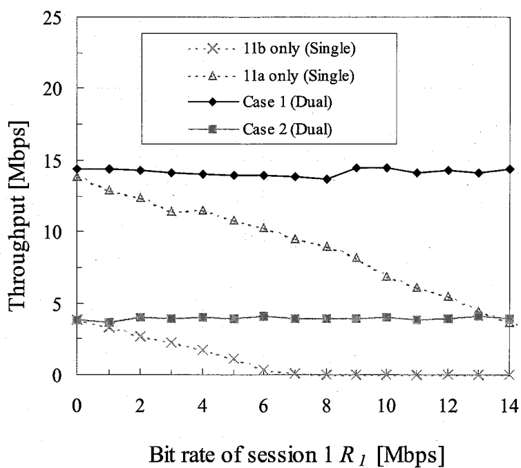
(b) セッション 2 (ファイル転送) の特性
