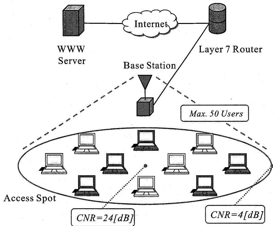
図 5.5: シミュレーションモデル
