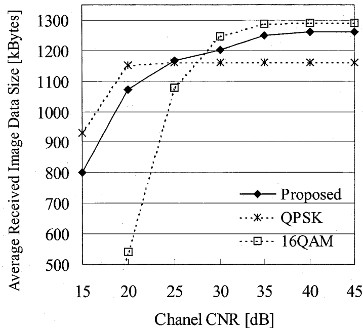
図 3.8: 平均受信 CNR に対する受信データ量特性 ( S = 1500 [KBytes])
