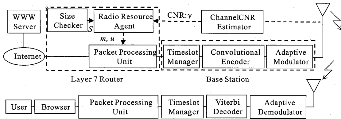
図 5.3: システム構成図
