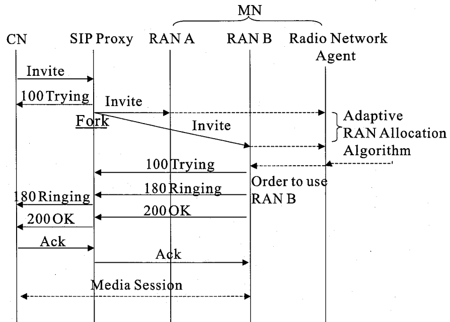
(a) CN が MN に対して接続要求する場合
