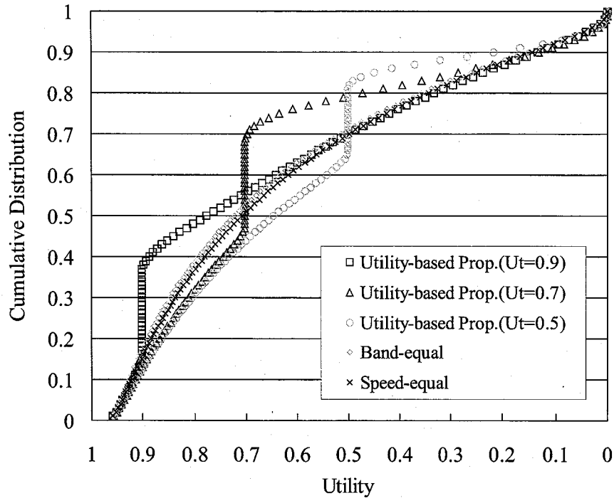
図 5.6: ユーザ効用の累積分布特性
