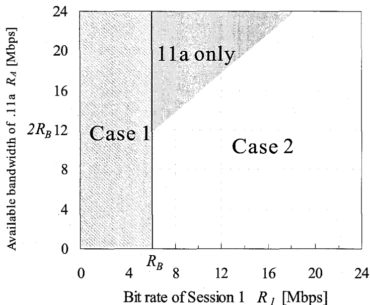
図 6.11: シナリオ 1 における RAN 適応割当の基準 (UDP 重視シナリオ)
