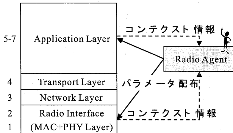
図 2.4: 電波エージェントの階層モデル
