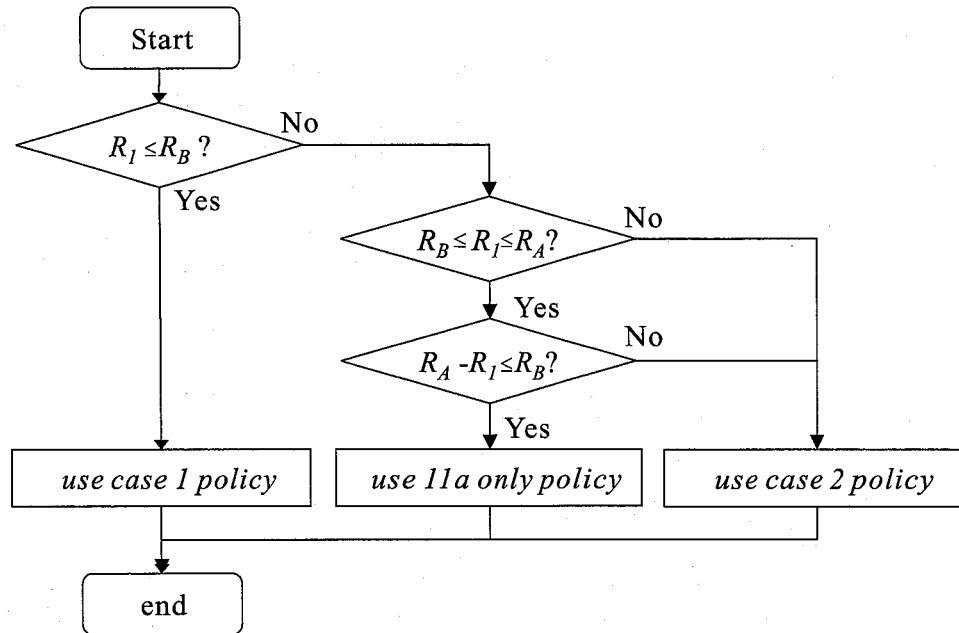
図 6.10: シナリオ 1 の場合の RAN 適応割当アルゴリズム
