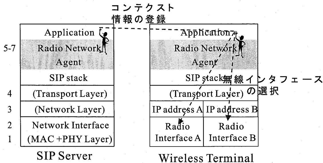
図 2.6: 無線ネットワークエージェントのレイヤ構造
