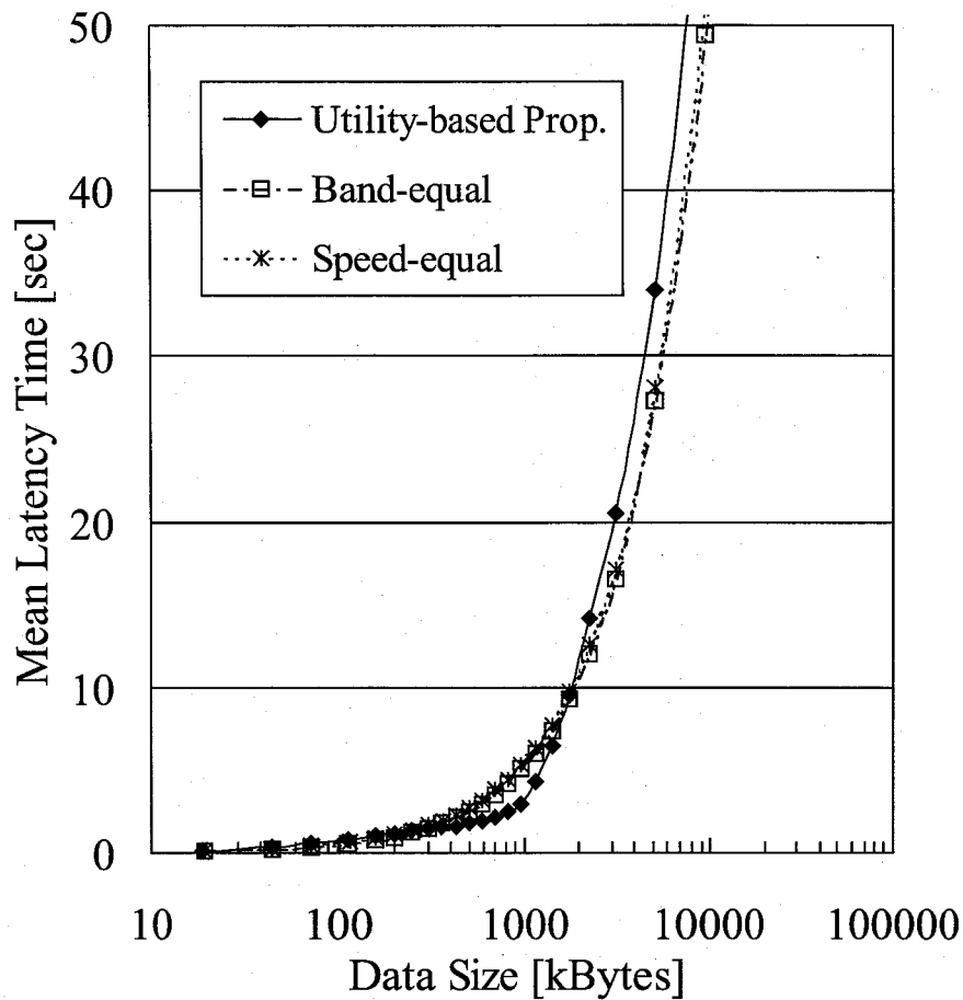
図 5.8: 要求データサイズに対する待ち時間特性
