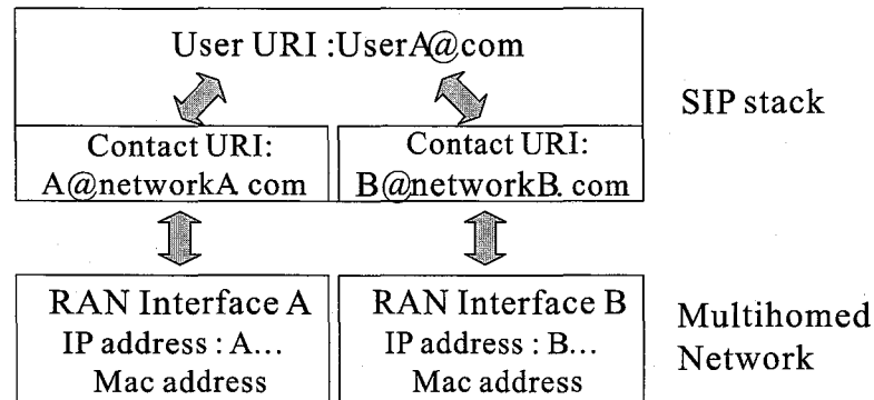
図 6.4: Contact URI と無線インタフェースの対応関係
