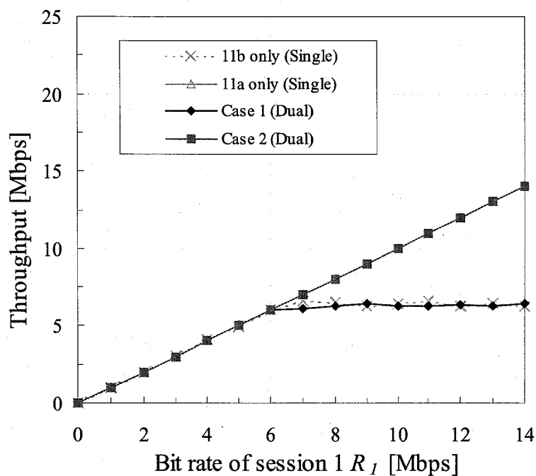
(a) セッション 1 (UDP ストリーム) の特性
