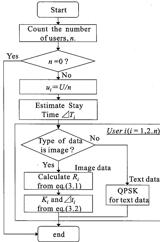
図 3.3: 提案方式のフローチャート
