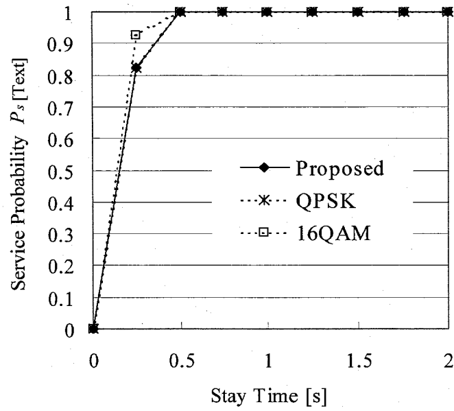
(a) 平均受信 CNR = 35[dB] の場合
