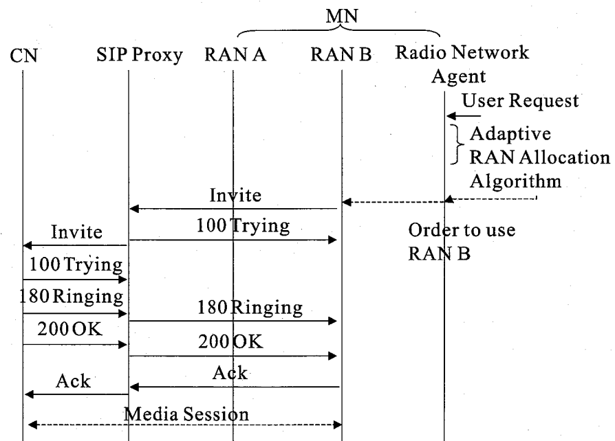
(b) MN が CN に対して接続要求する場合
