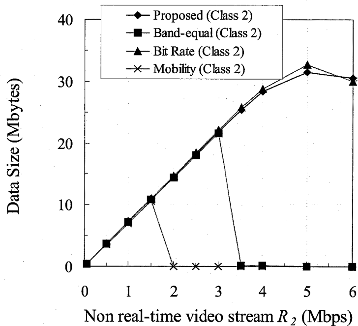
(b) 静止ユーザ (Class 2)
