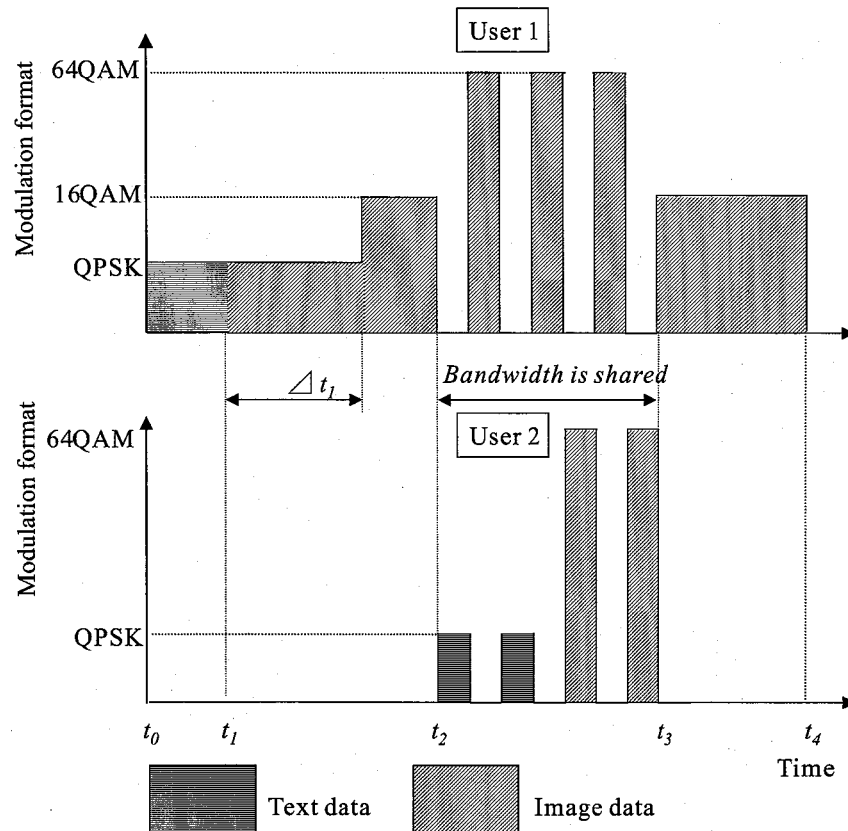
図 3.4: 提案アルゴリズムの適用例
