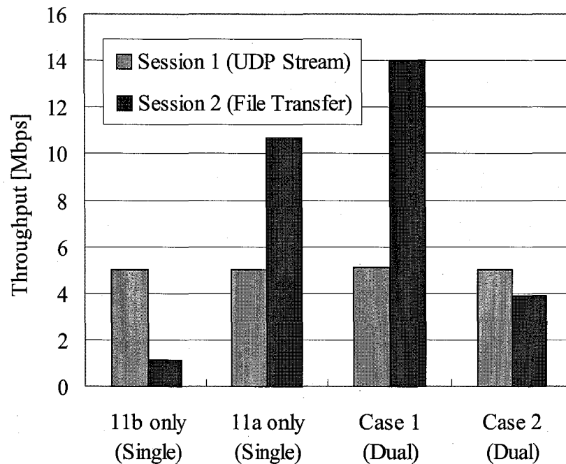
図 6.7: 各サービスに対するスループット特性 ( R_1=5\text{Mbps} )
