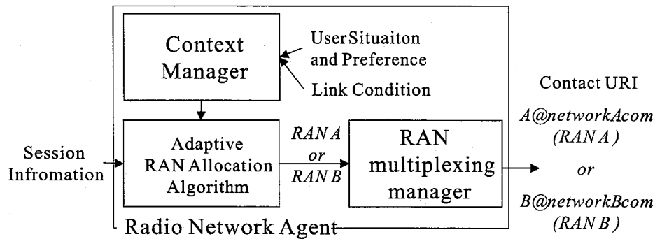
図 6.3: 無線ネットワークエージェントの構成
