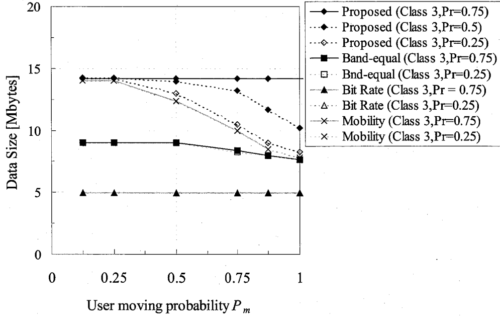
(a) 移動ユーザ (Class 3)
