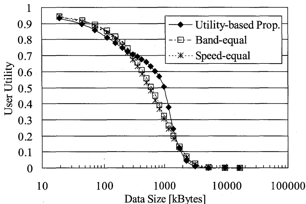
図 5.7: 要求データサイズに対するユーザ効用
