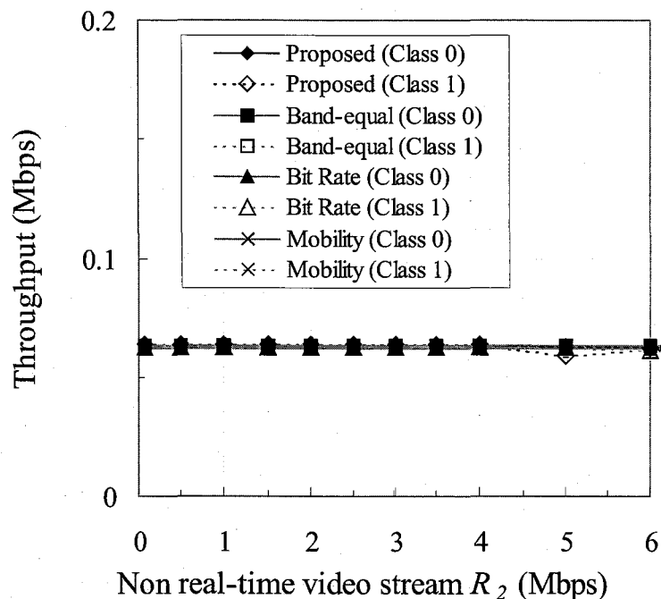
図 4.5: リアルタイムストリーム R_2 に対する Class 0 と Class 1 ユーザのスループット特性 ( R_1 = 64\text{Kbps} ).
