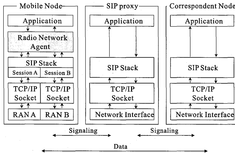
図 6.2: システム構成図
