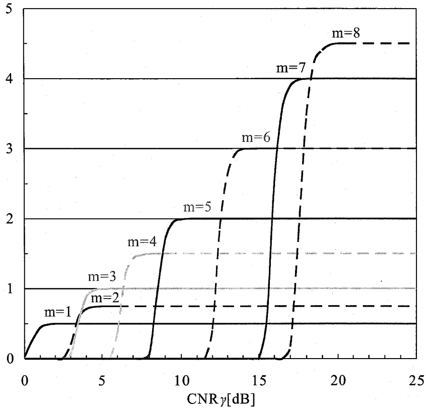
図 5.4: AWGN 環境下における各伝送モードの周波数利用効率
