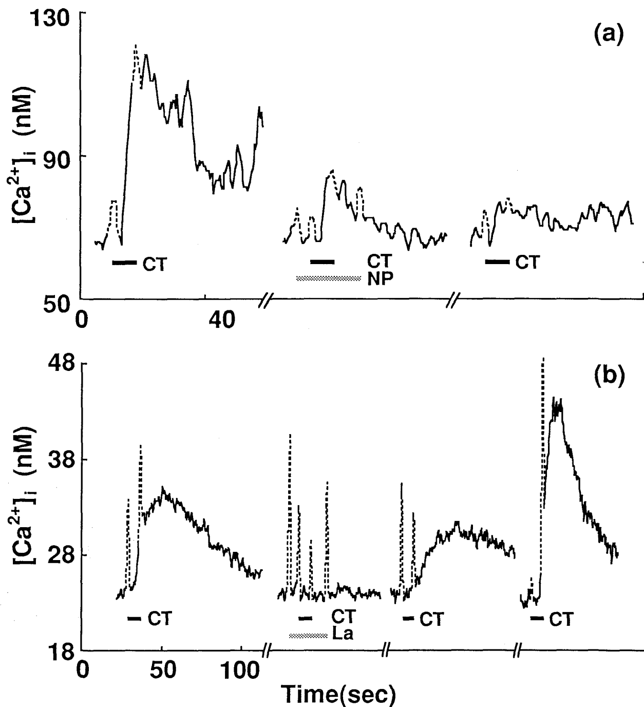
図27 Ca^{2+} チャネルブロッカーのニオイ誘起 [Ca^{2+}]_i 上昇への効果 1)
