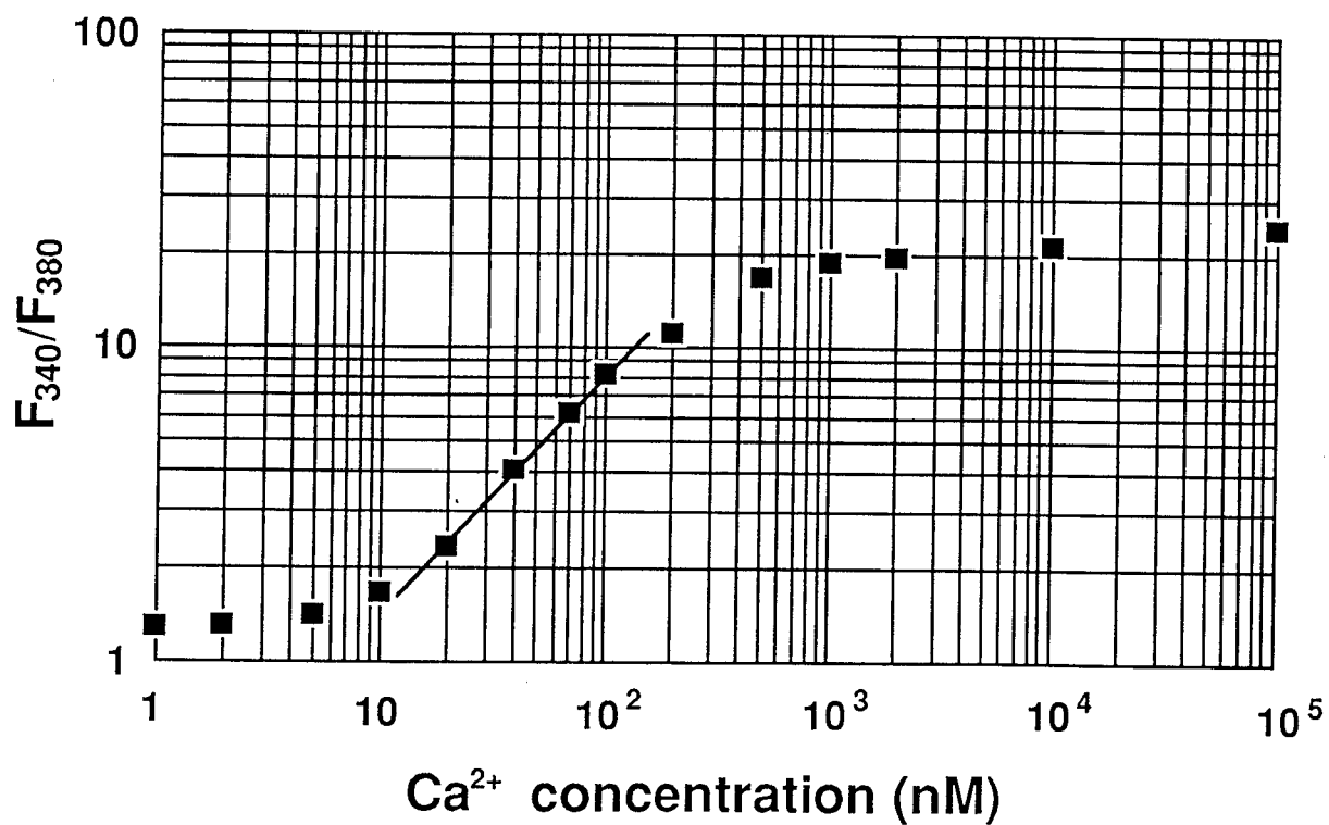
図12 マウス嗅細胞の [\text{Ca}^{2+}]_i 測定における蛍光強度比と [\text{Ca}^{2+}]_i 校正曲線
