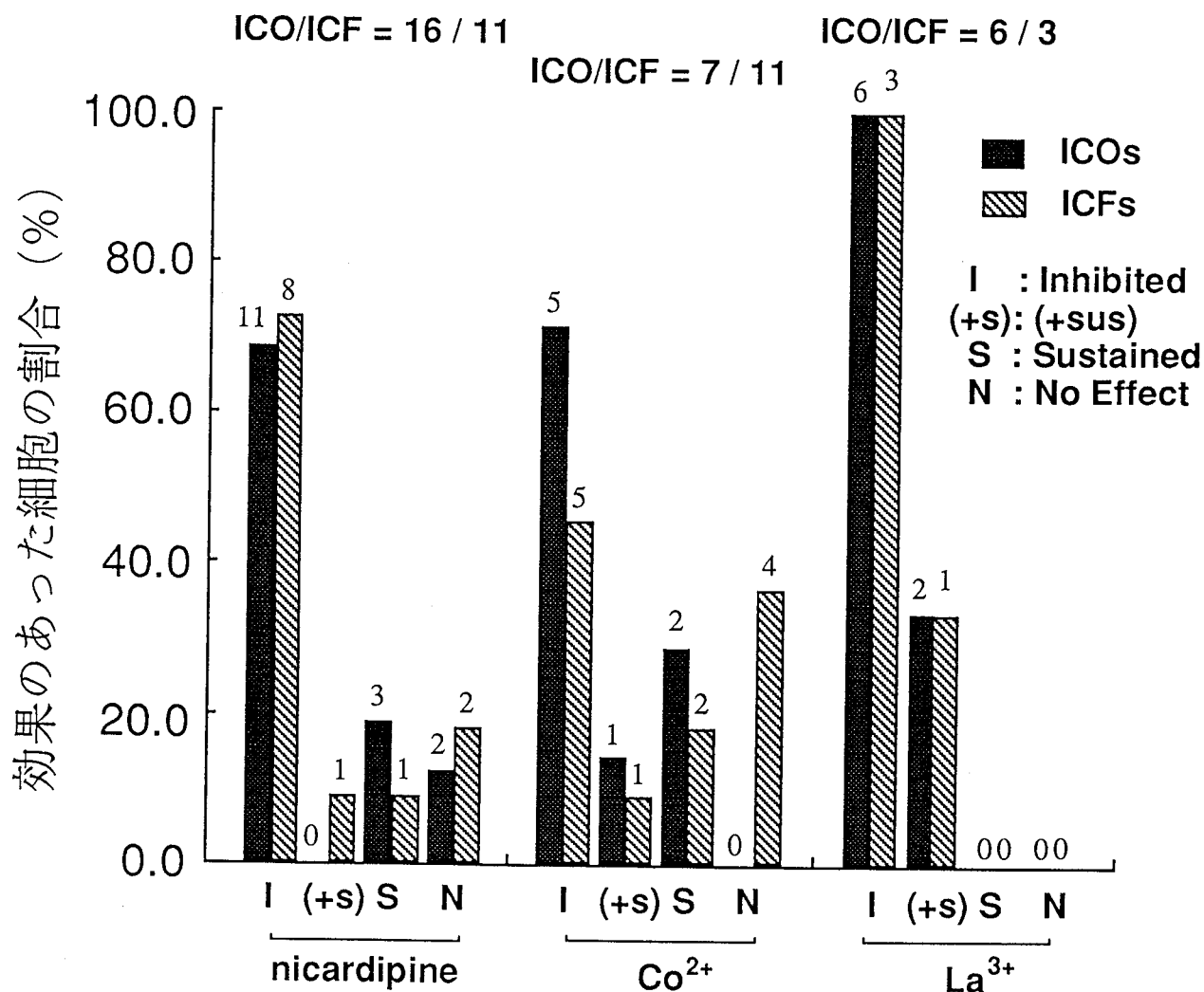
図26 \text{Ca}^{2+} チャンネルブロッカーによる [\text{Ca}^{2+}]_i 上昇の抑制効果 1)
