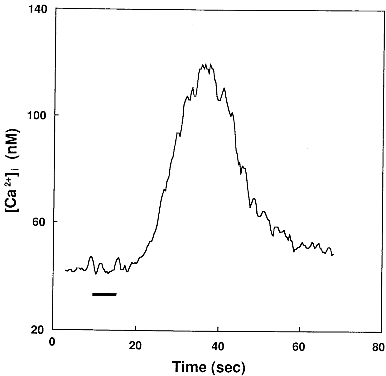
図16 ニオイ刺激終了後に [Ca^{2+}]_i 上昇が生じる応答例
