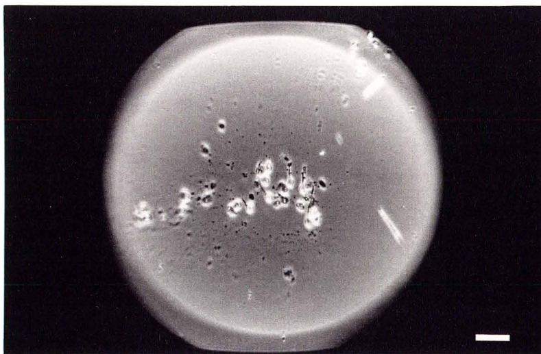
図10 Tissue-printing法によって得た単離嗅細胞の例
