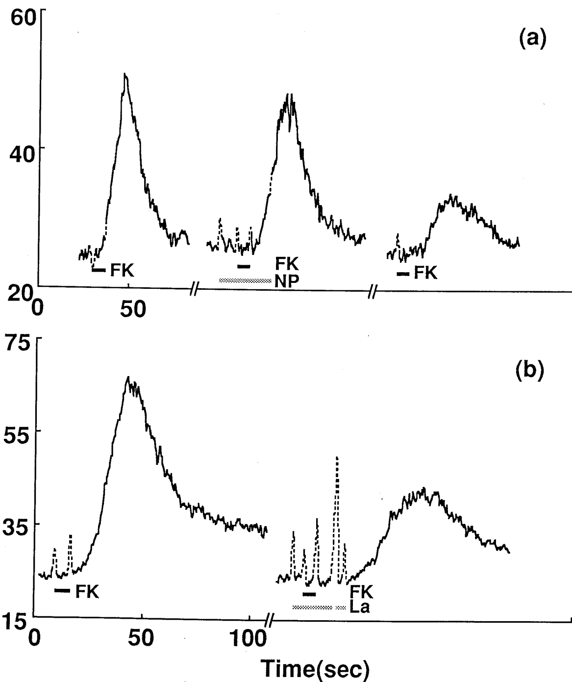
図28 Ca 2+ チャネルブロッカーのforskolin誘起[Ca 2+ ] i 上昇への効果 1)
