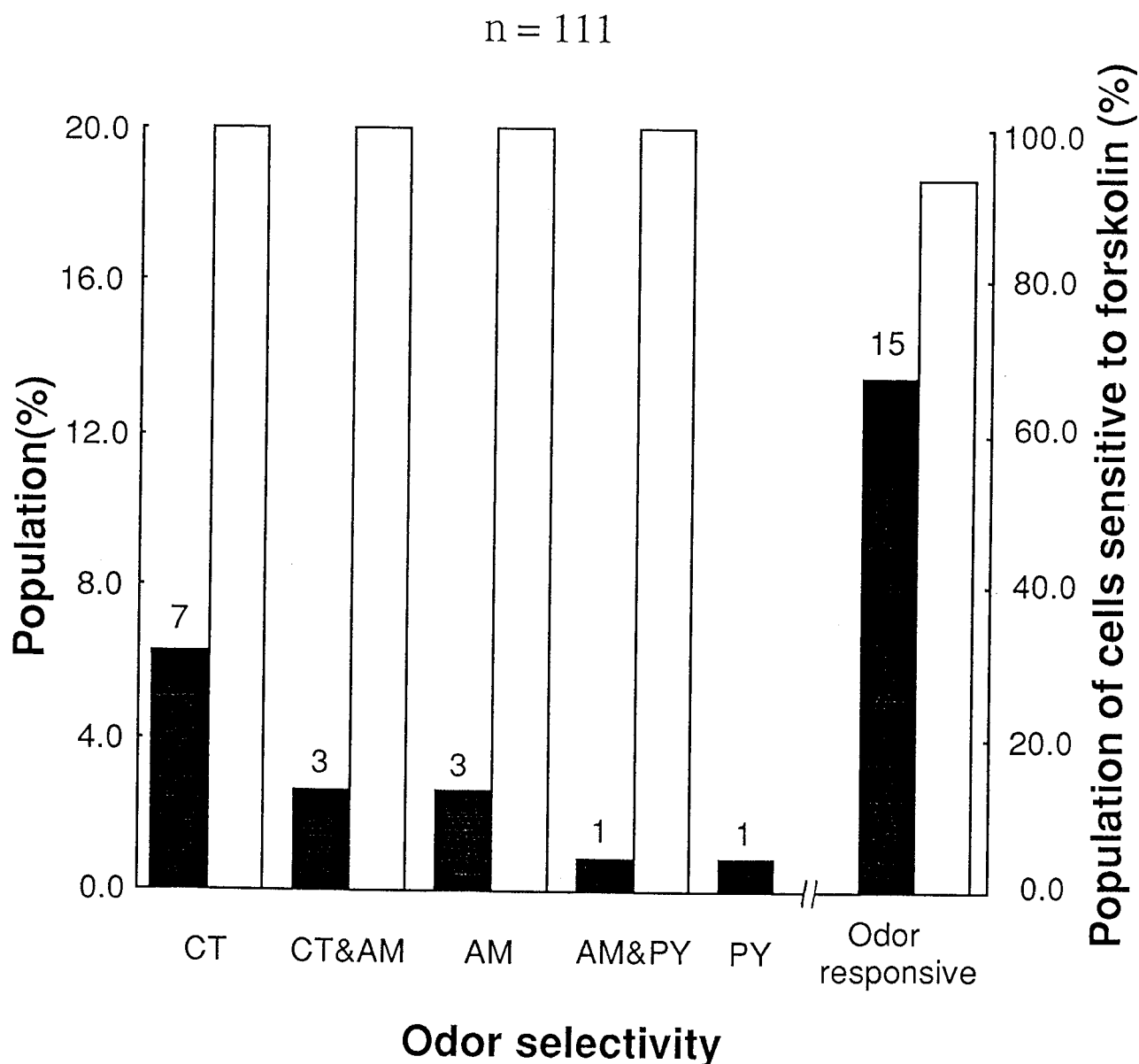
図22 tissue-printing法で得たマウス嗅細胞のニオイ応答性
